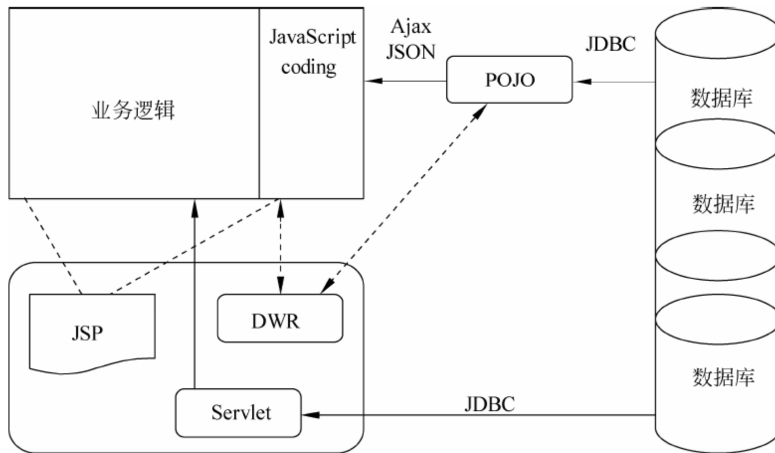
图 6-4 基于 DWR 的具体应用结构
