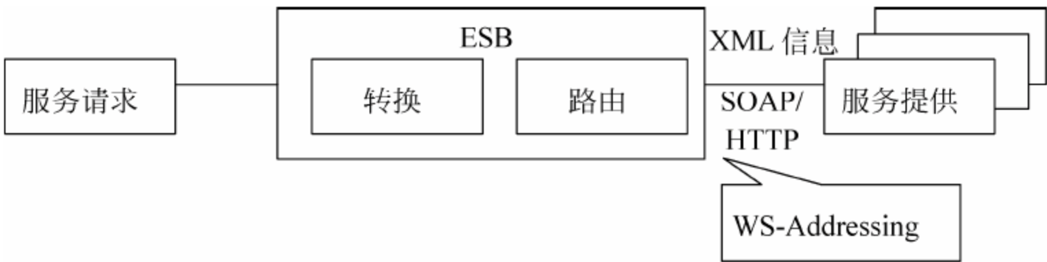
图 3-53 ESB 互操作的路由
