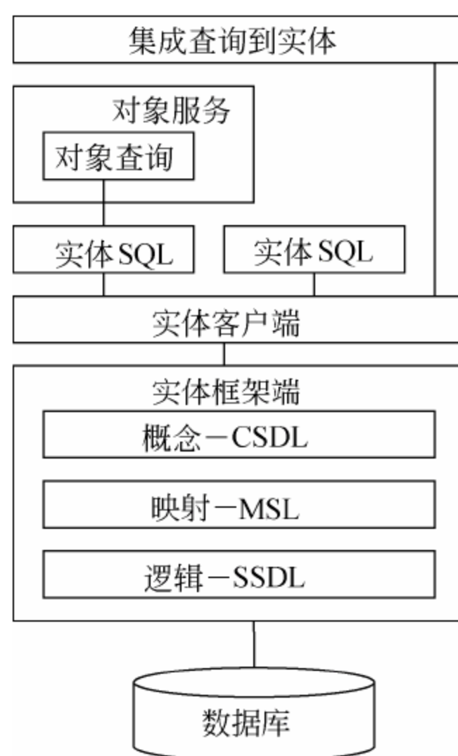
图 5-56 ADO.NET 实体框架
