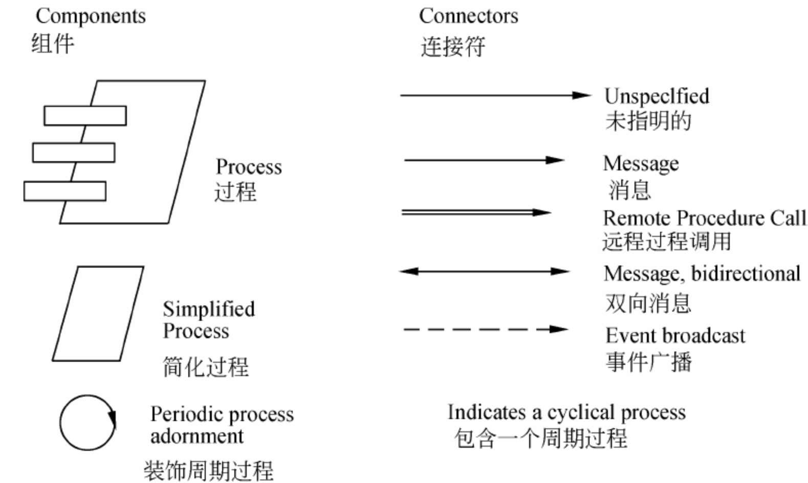
图 2-9 面向 Booch 的过程视图标记法
