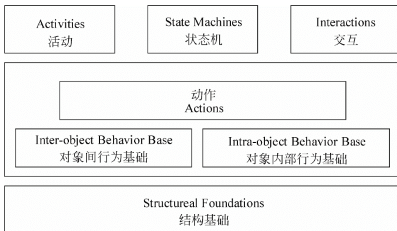
图 3-5 UML 2.0 语义框架
