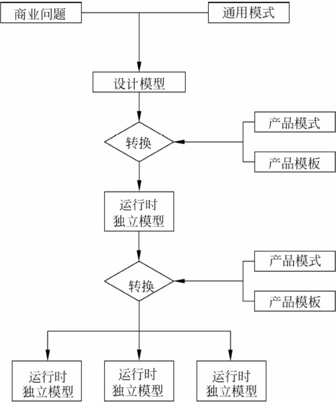
图 3-9 MDD 工具开发
