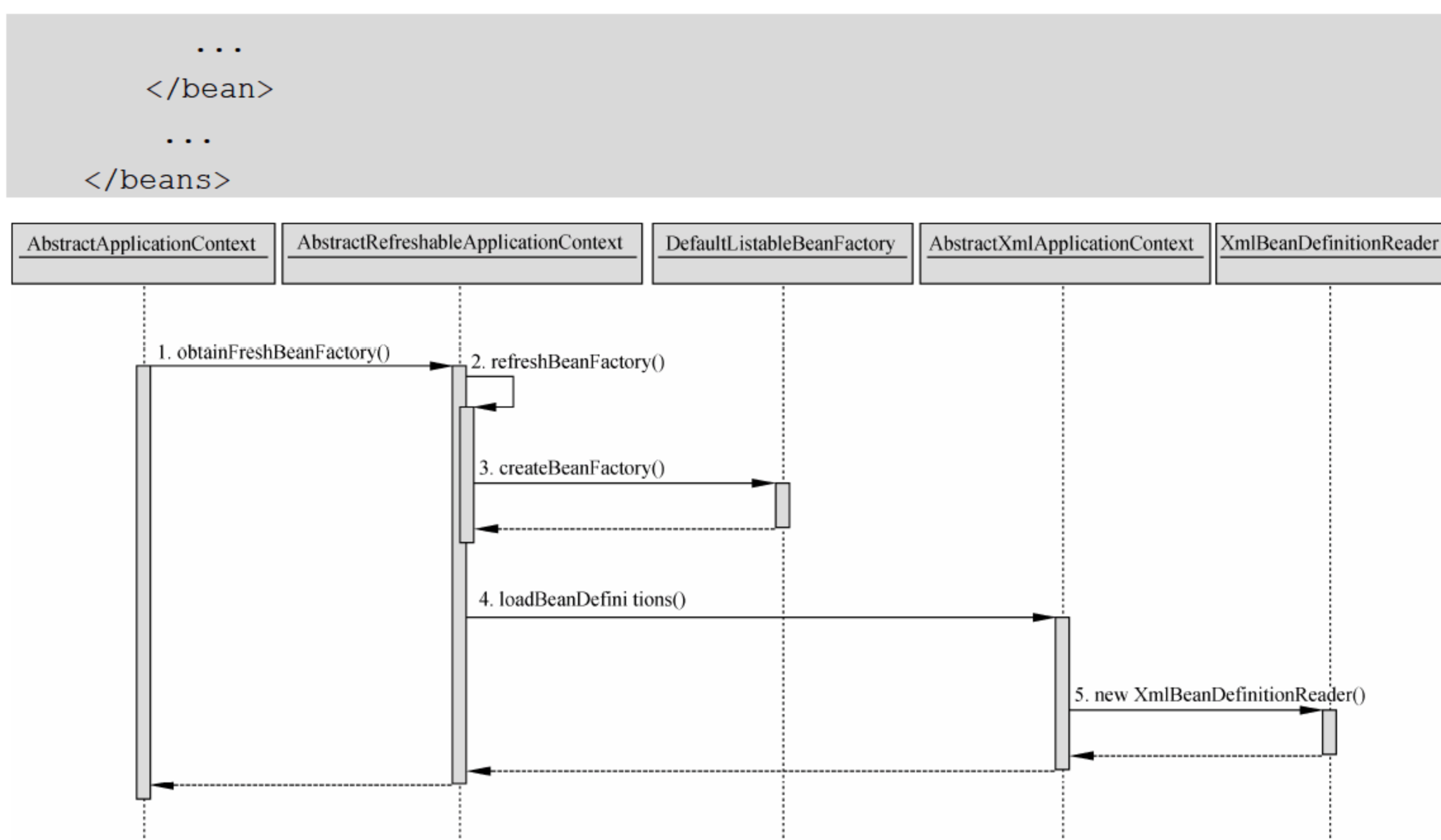
图 6-24 创建 Bean 的时序图
