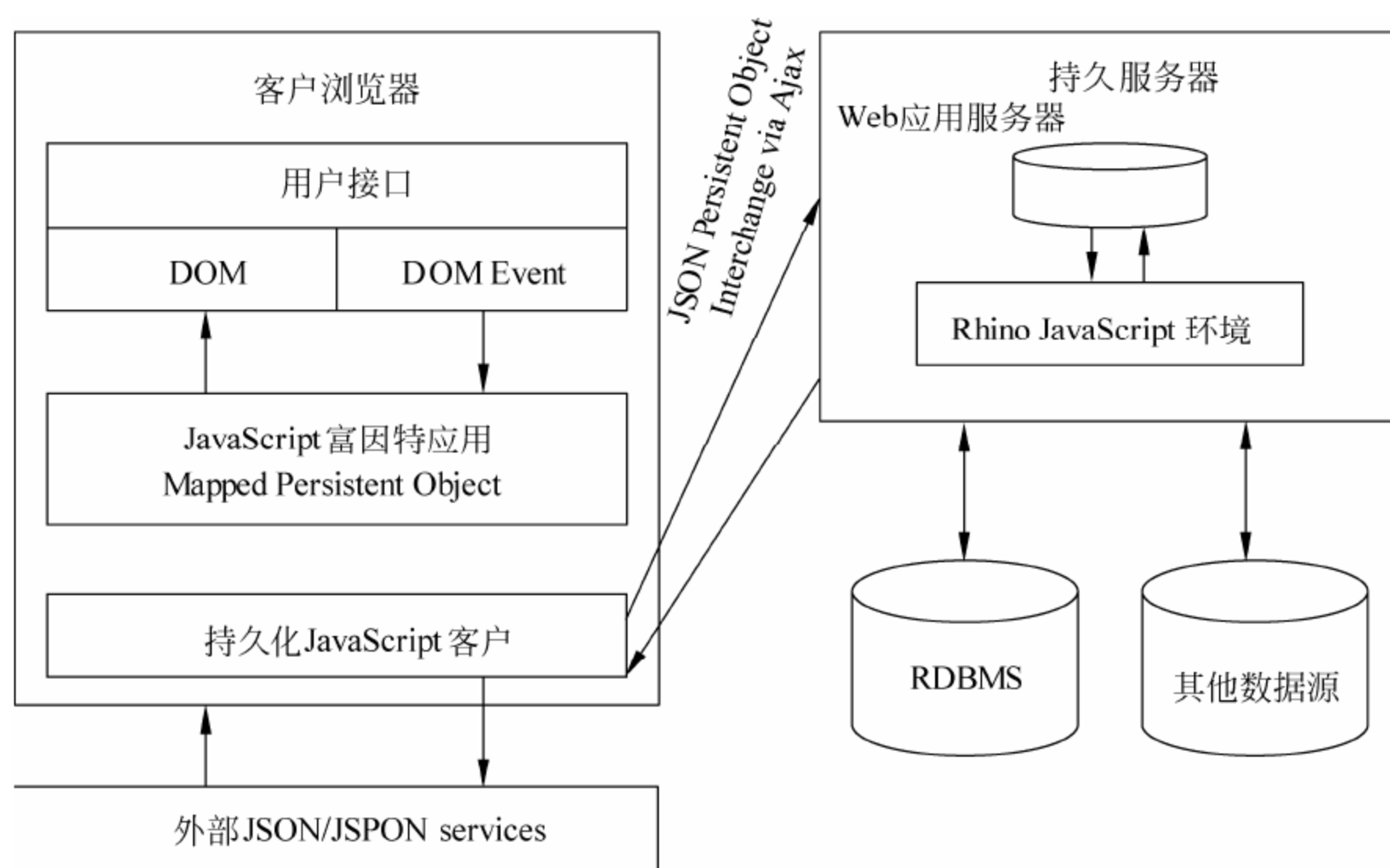
图 6-2 Persevere 持久 JSON SOA
