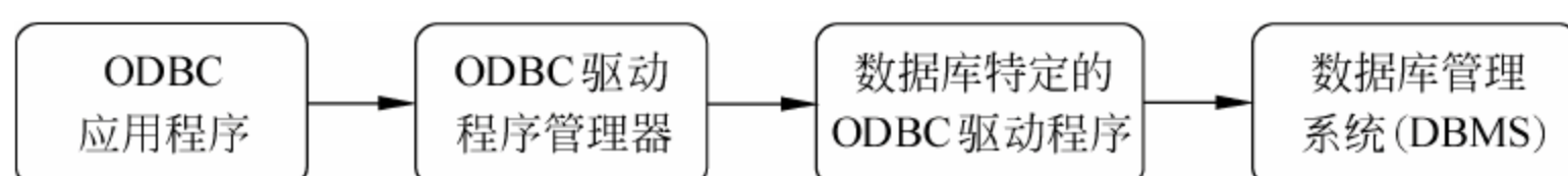
图 5-49 ODBC 体系结构
