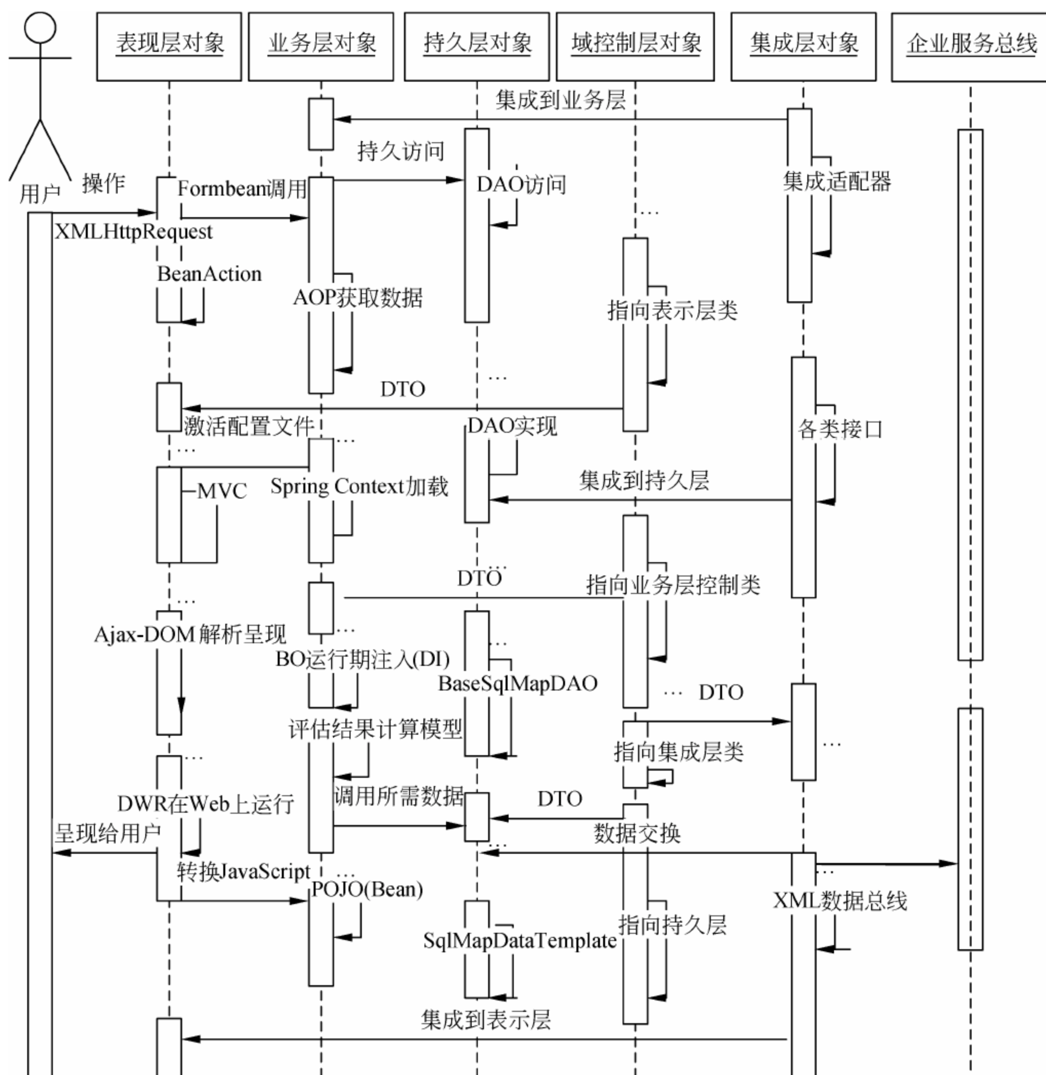
图 2-42 面向轻量级的开源技术整合的时序运行图
