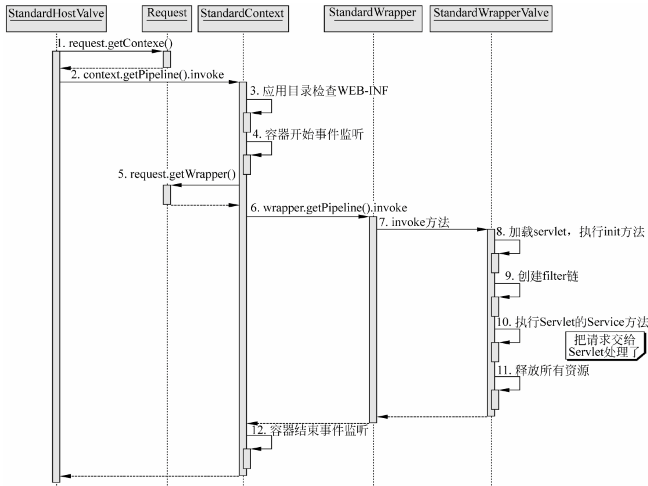
图 5-11 Context 和 wrapper 的处理请求时序图
