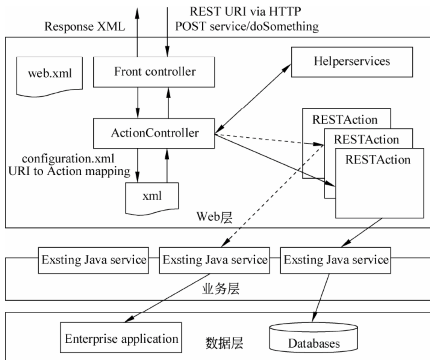
图 5-25 一种 REST 架构实现
