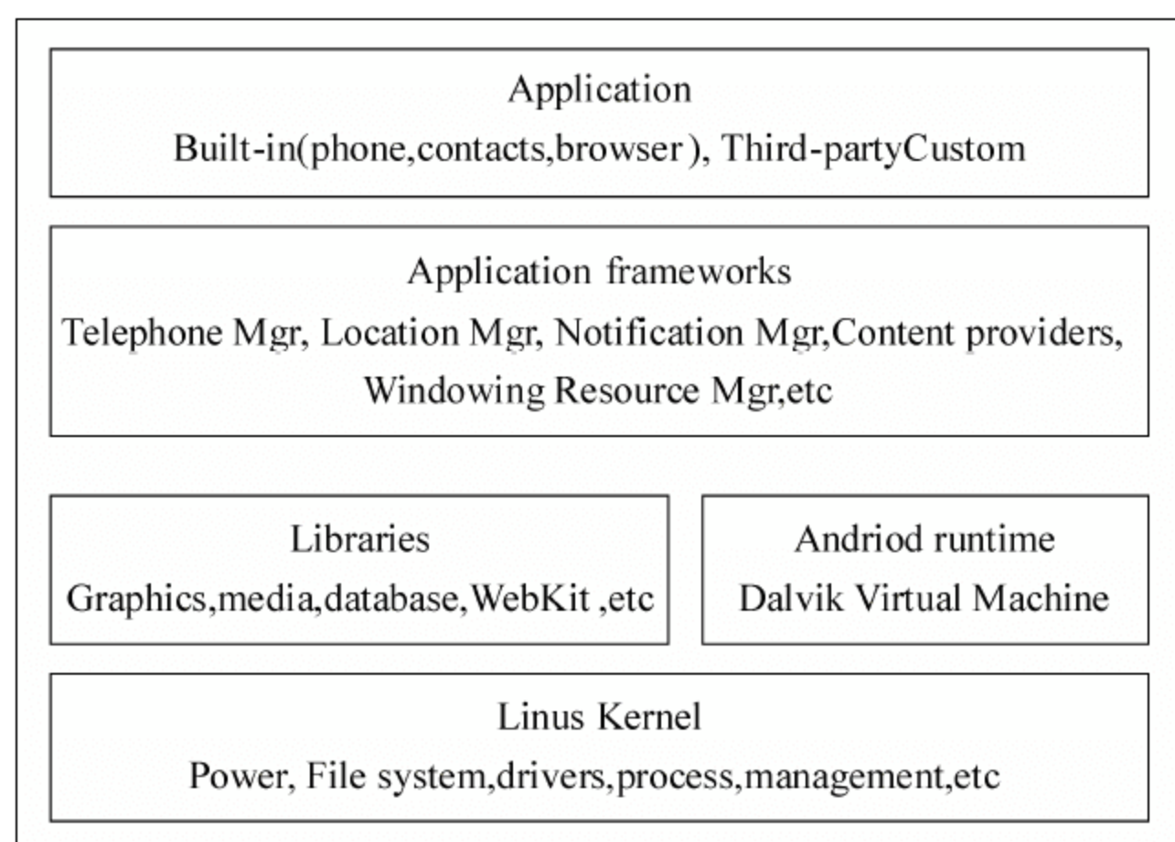
图 5-3 Android 层次结构
