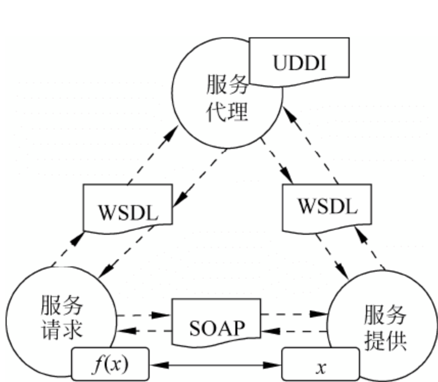
图 3-26 Web 服务基本结构
