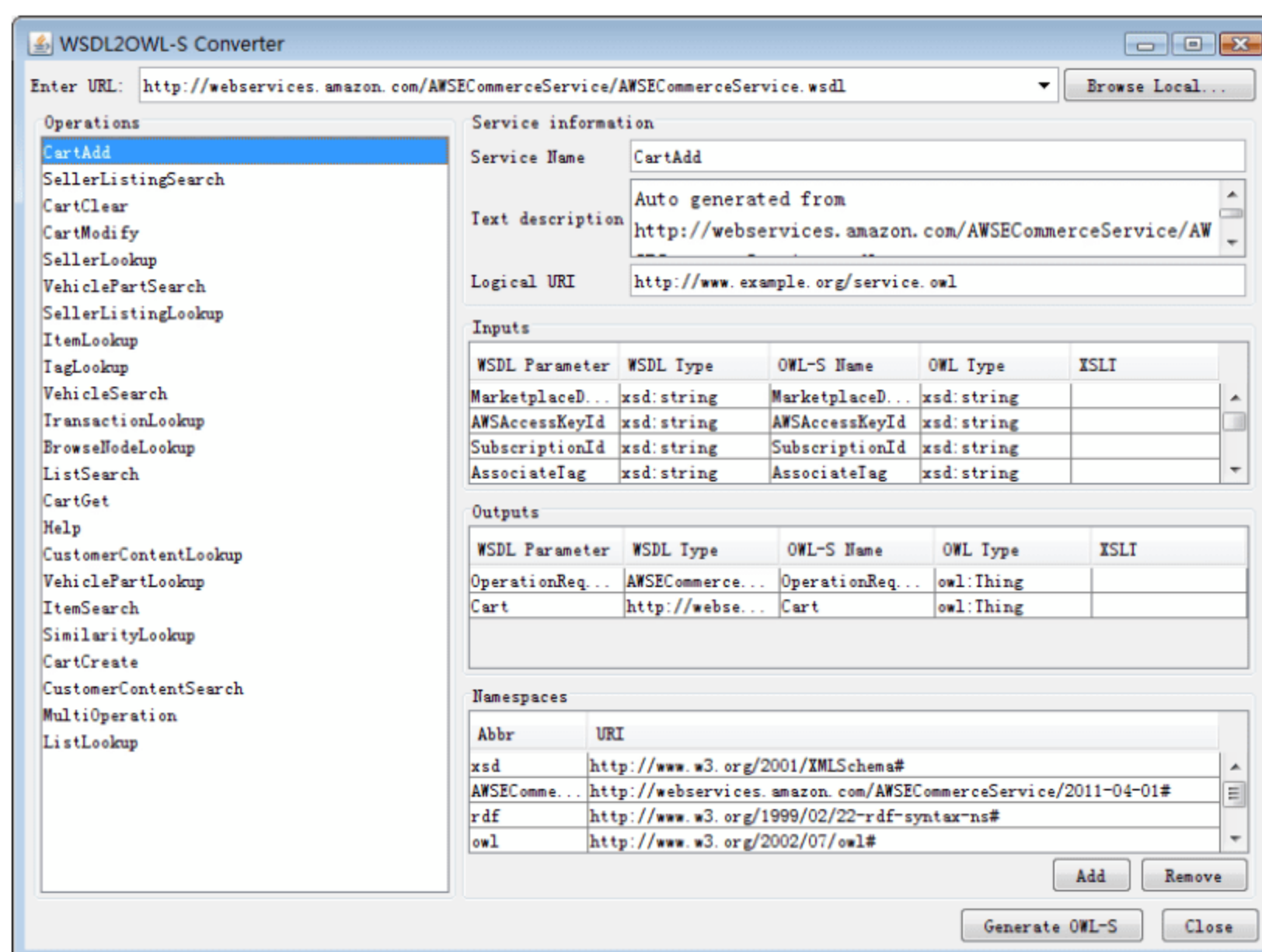
图 6-40 基于 WSDL2OWL-S 的语义 Web 服务结果
