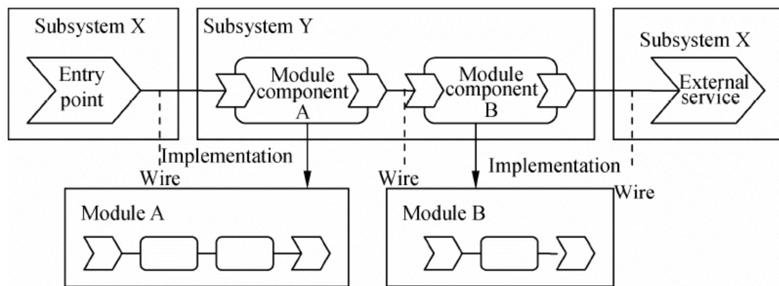
图 2-57 服务组件体系结构
