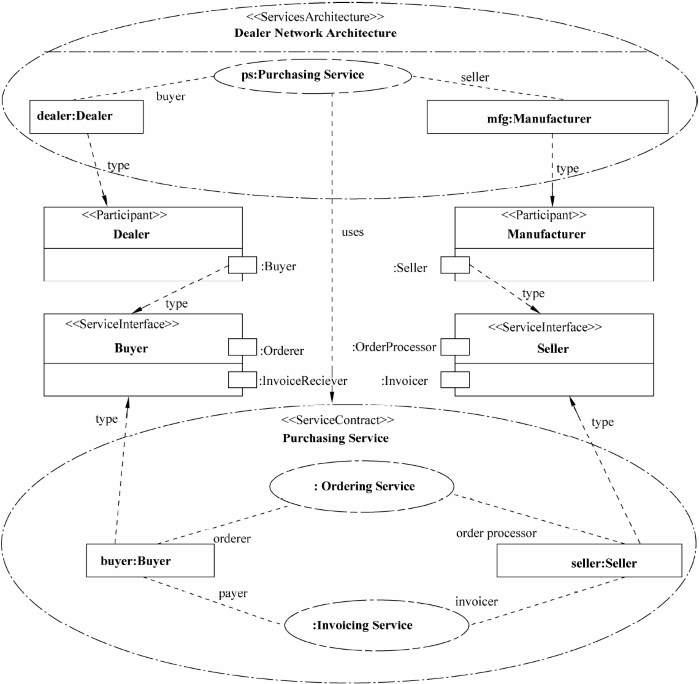
图 3-69 作为服务合约的相关服务体系结构
