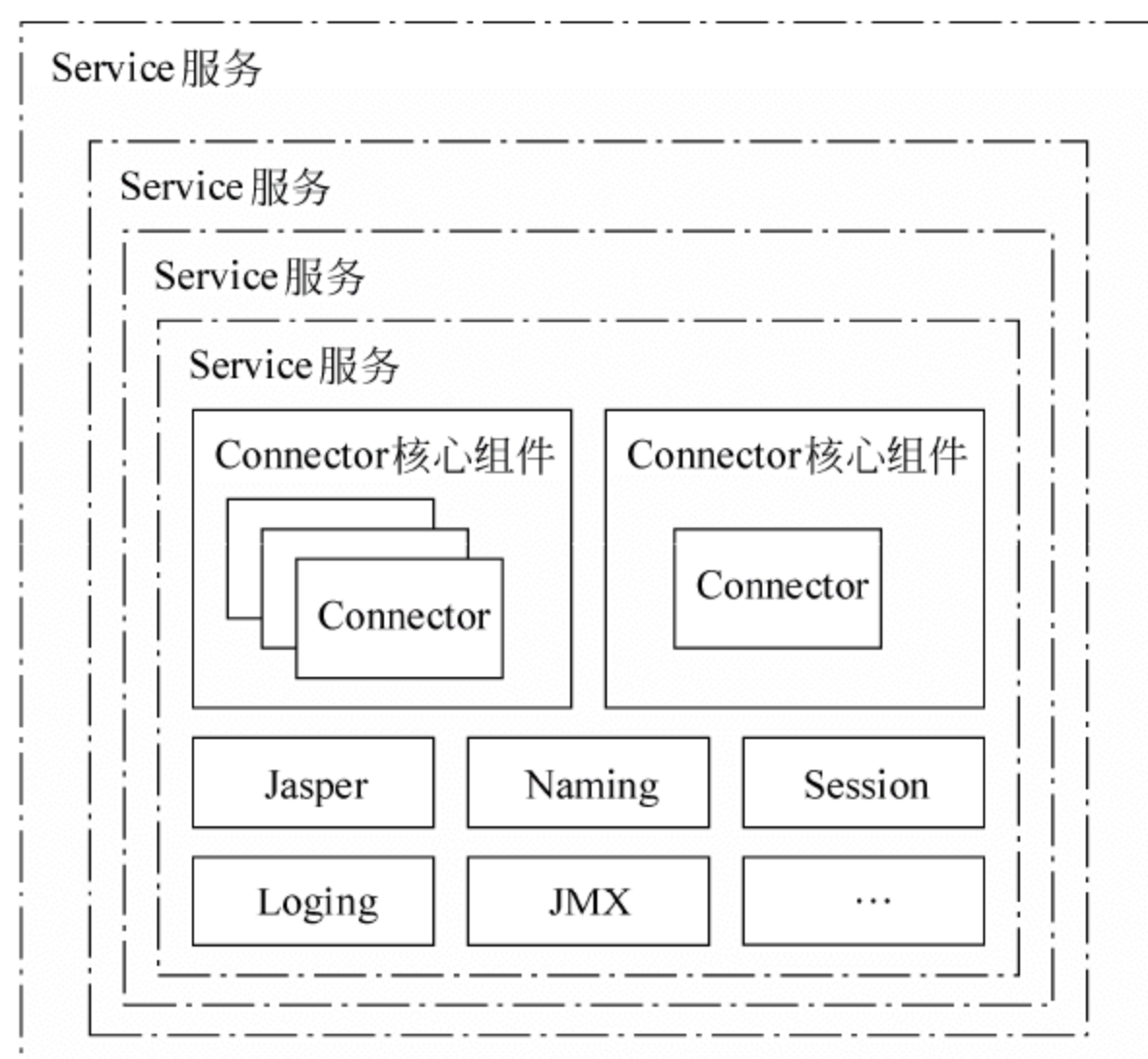
图 5-7 Tomcat 结构
