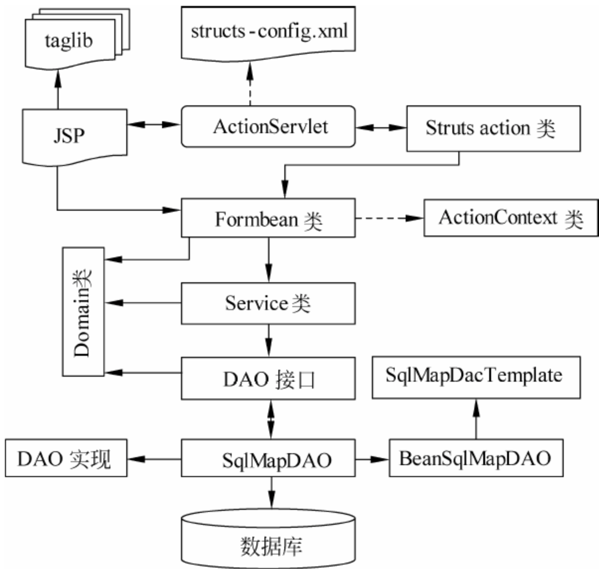
图 6-36 JpetStore 实现
