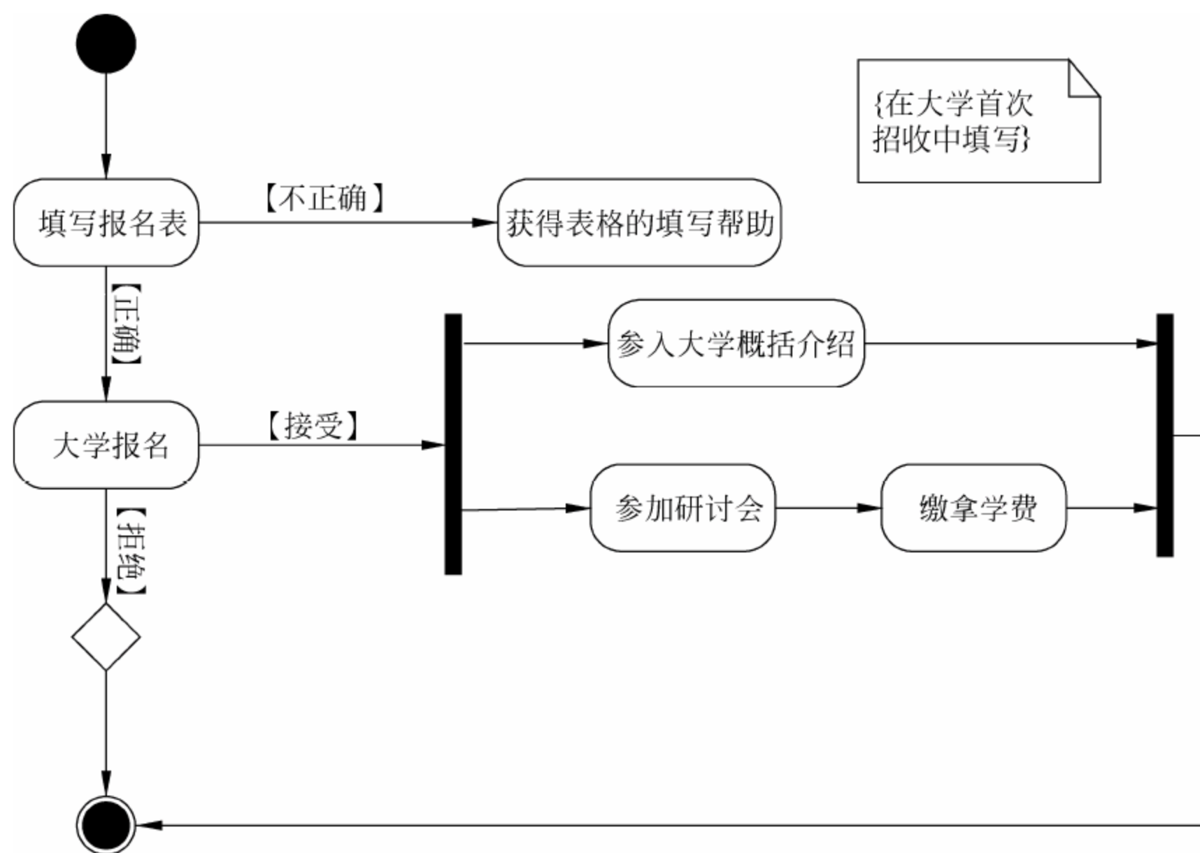
图 3-23 活动图
