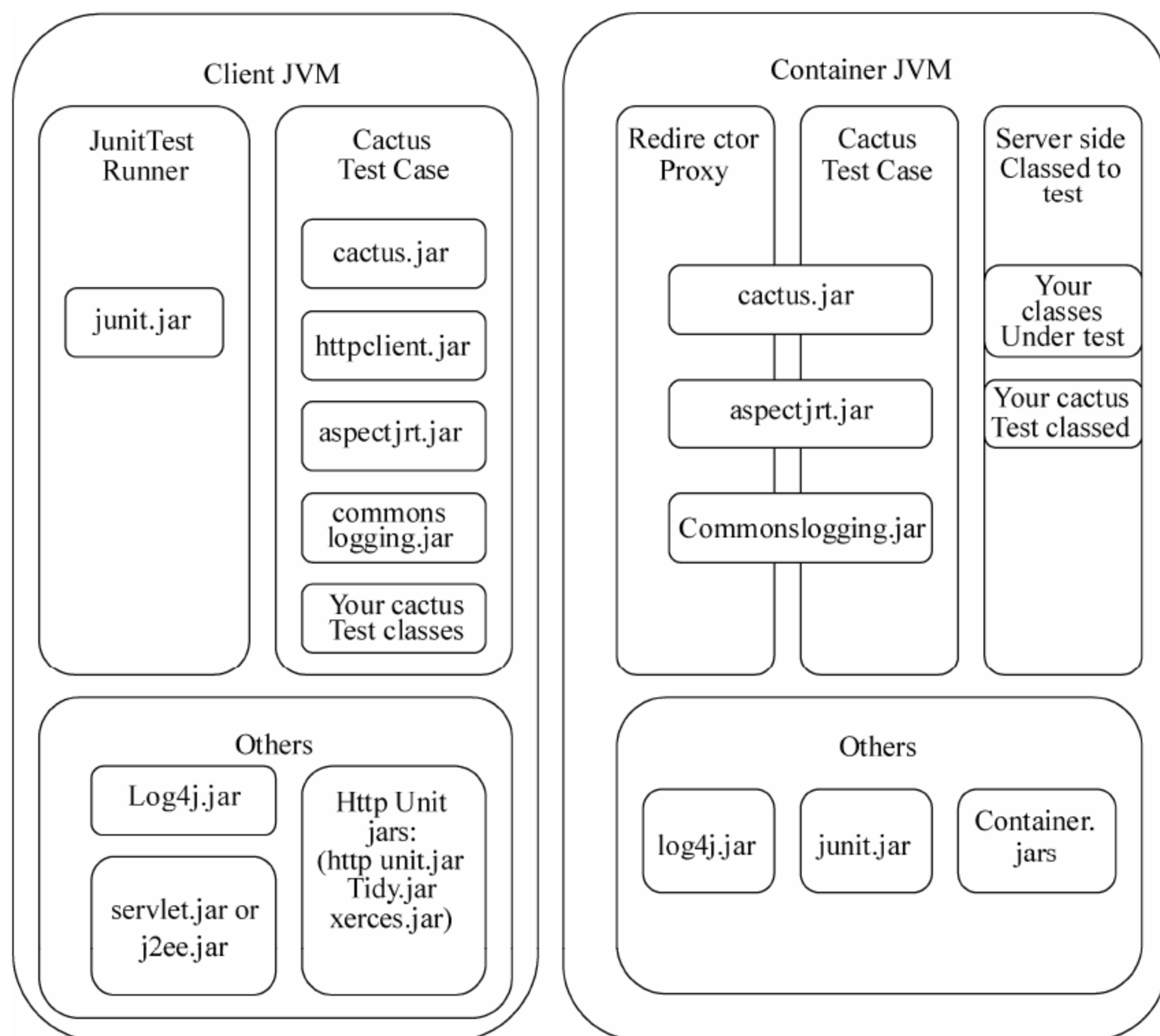
图 5-6 JUnit 结构
