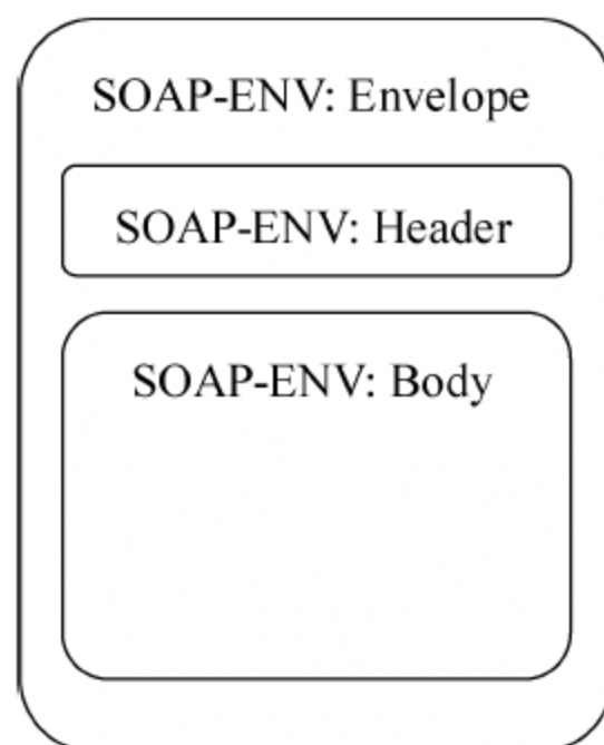
图 5-20 SOAP 结构
