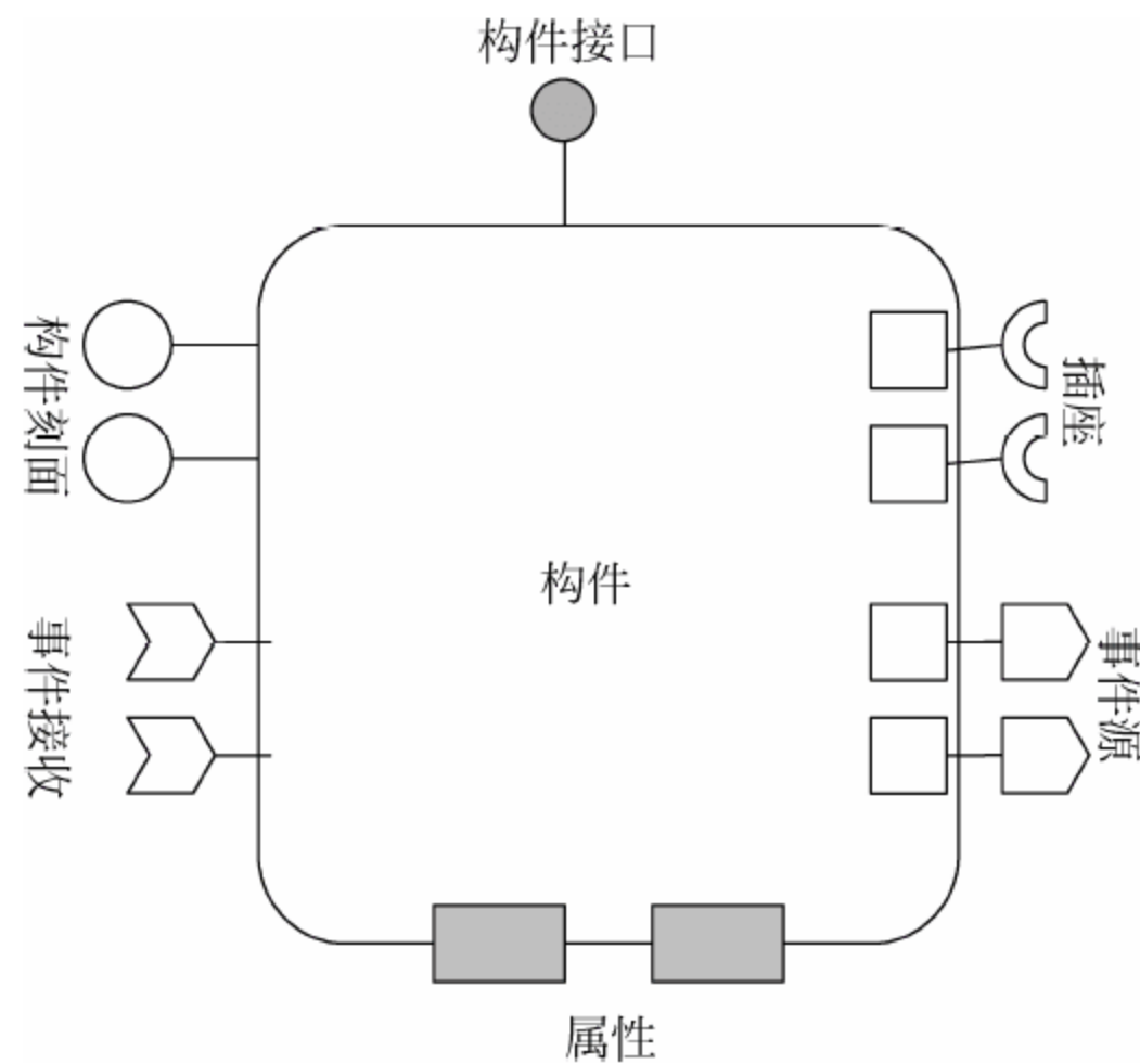
图 3-1 构件定义
