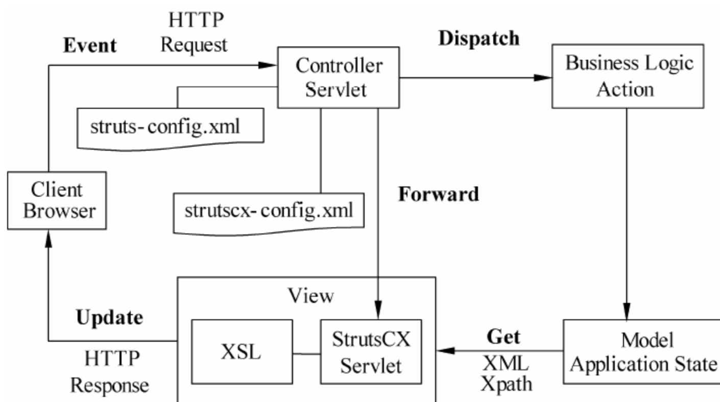
图 6-17 StrutsCX 概览
