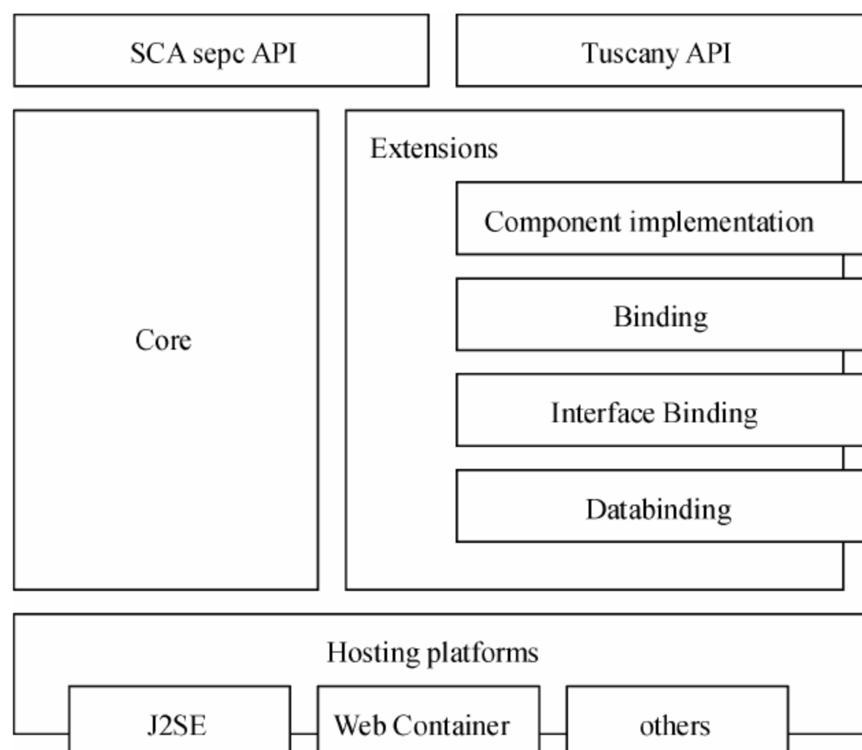
图 6-49 Tuscany 结构
