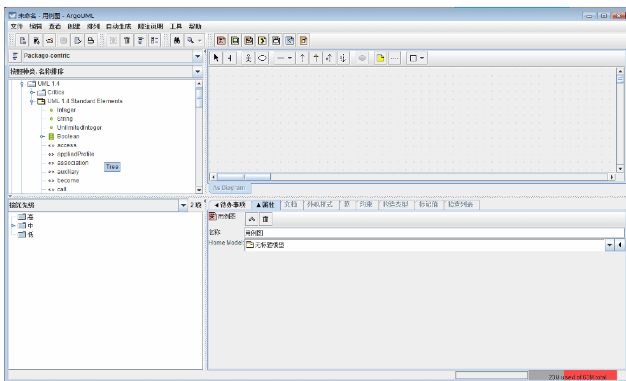
图 3-6 ArgoUML 运行图
