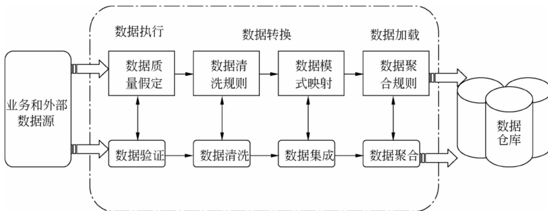
图 6-57 ETL 过程
