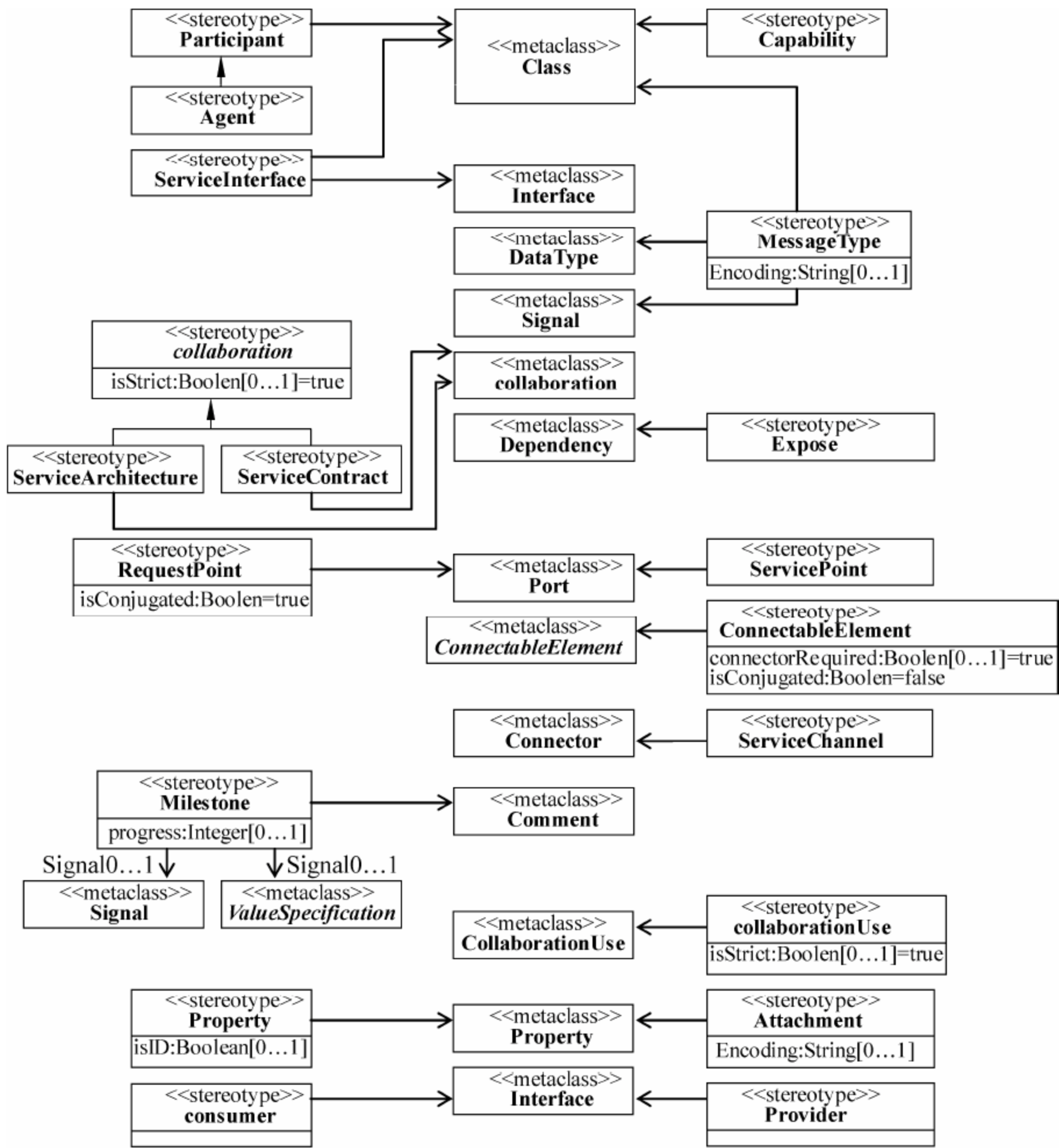
图 3-60 SoaML Profile
