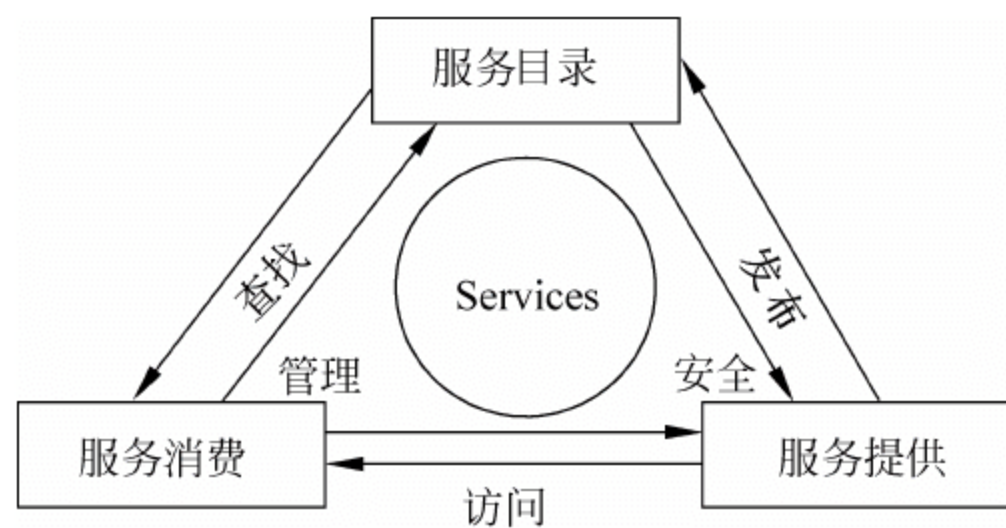
图 3-28 SOA 结构图
