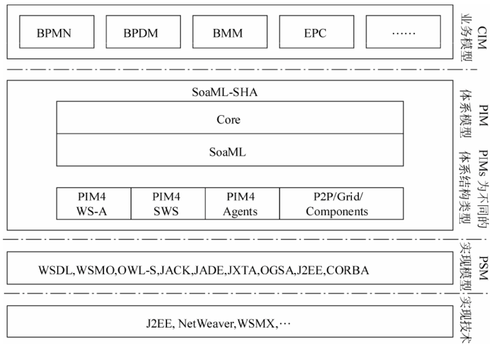
图 3-62 SOAML 结构
