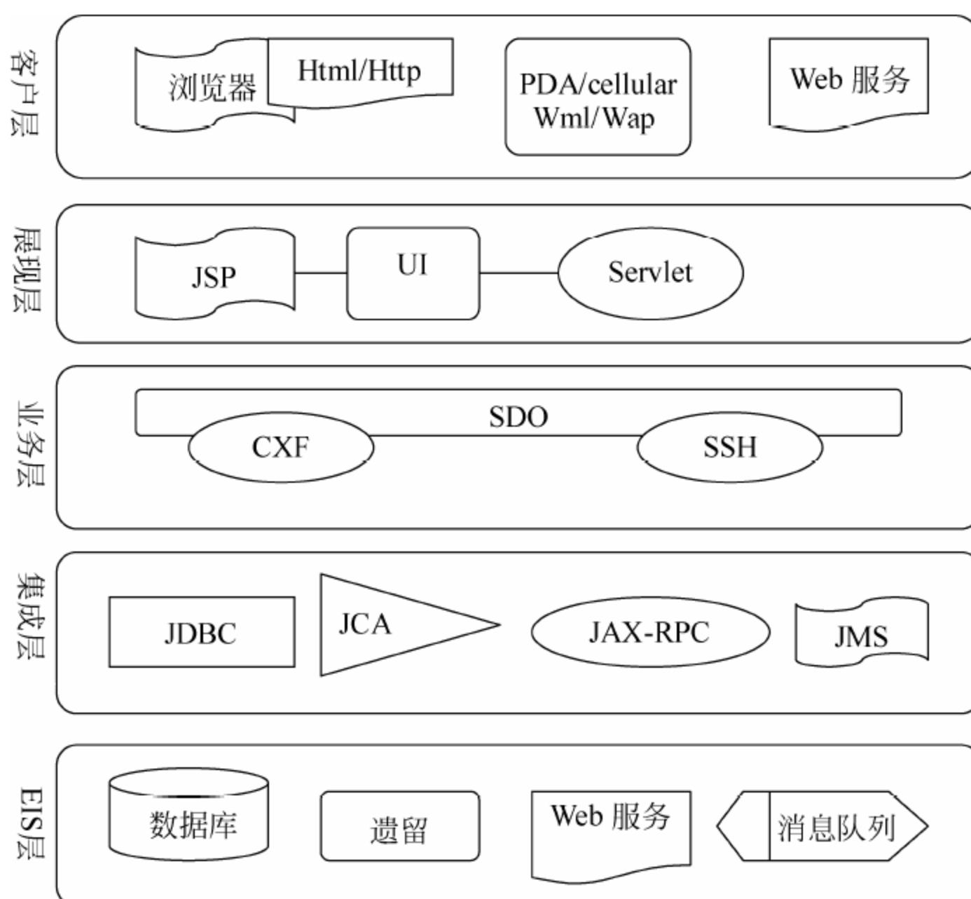
图 5-37 基于 SDO 的应用体系结构
