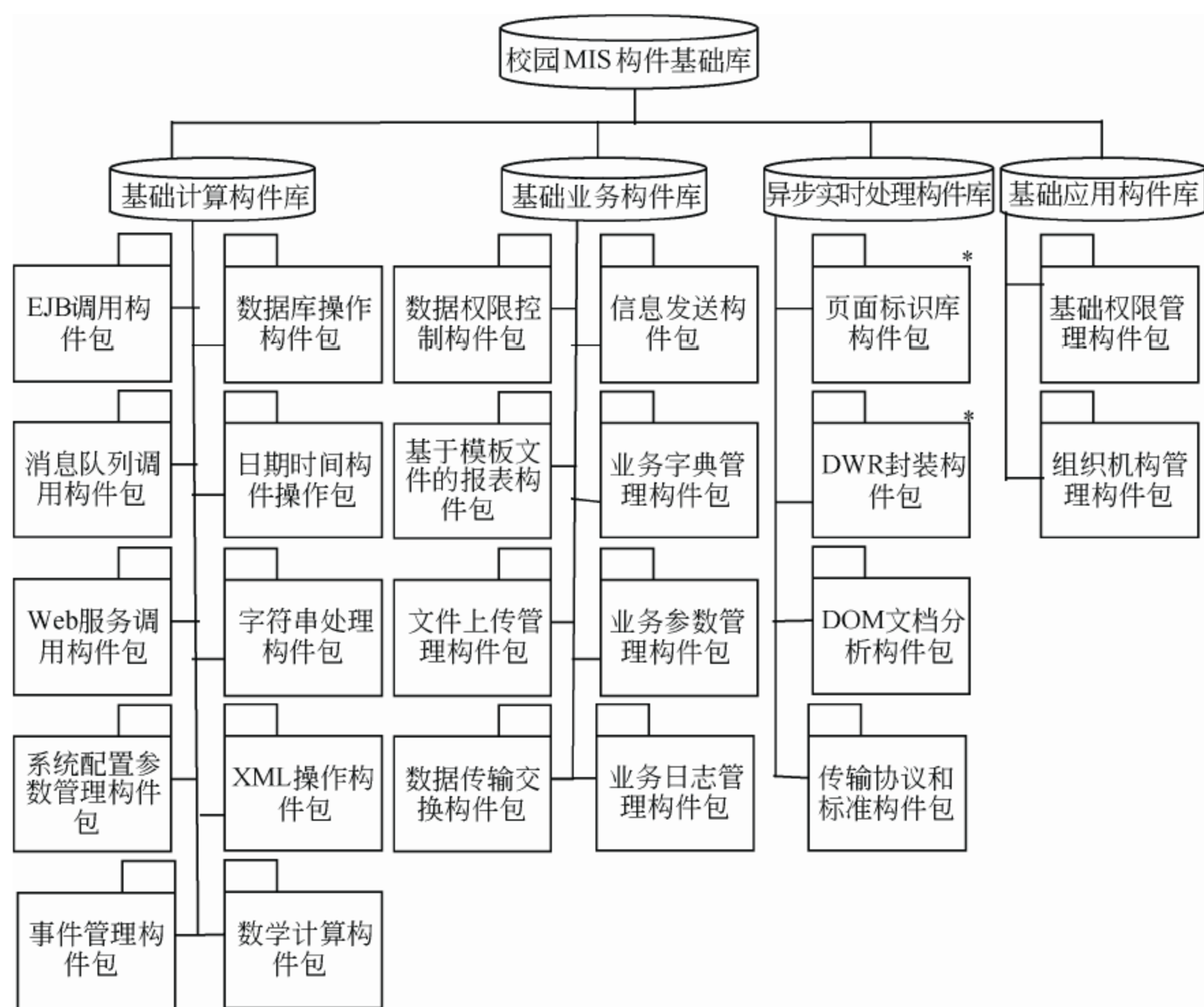
图 2-26 校园 MIS 基础构件
