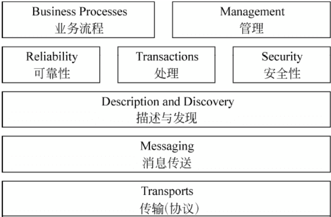
图 3-27 Web 服务规范结构
