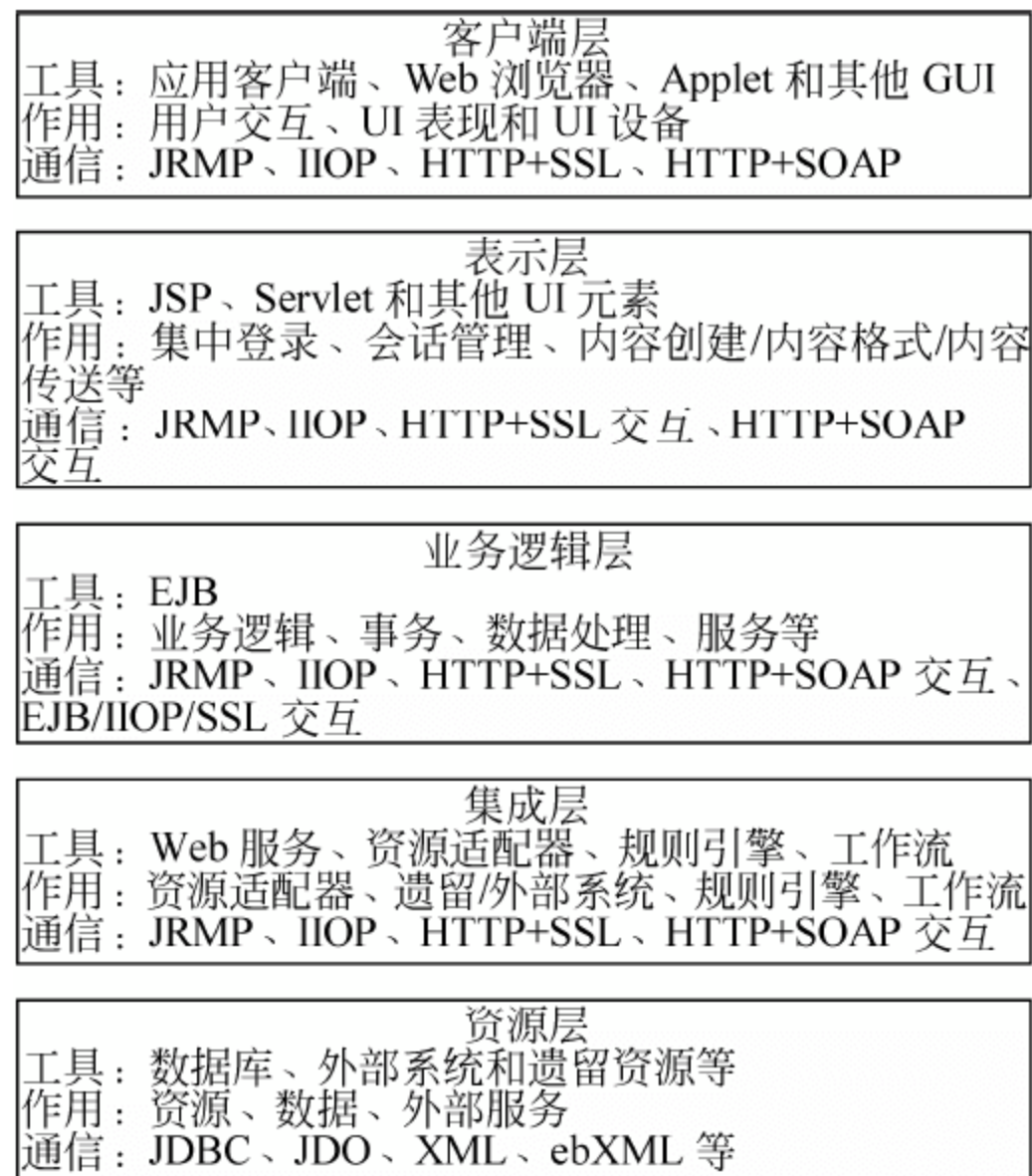
图 2-30 J2EE 核心分层模式
