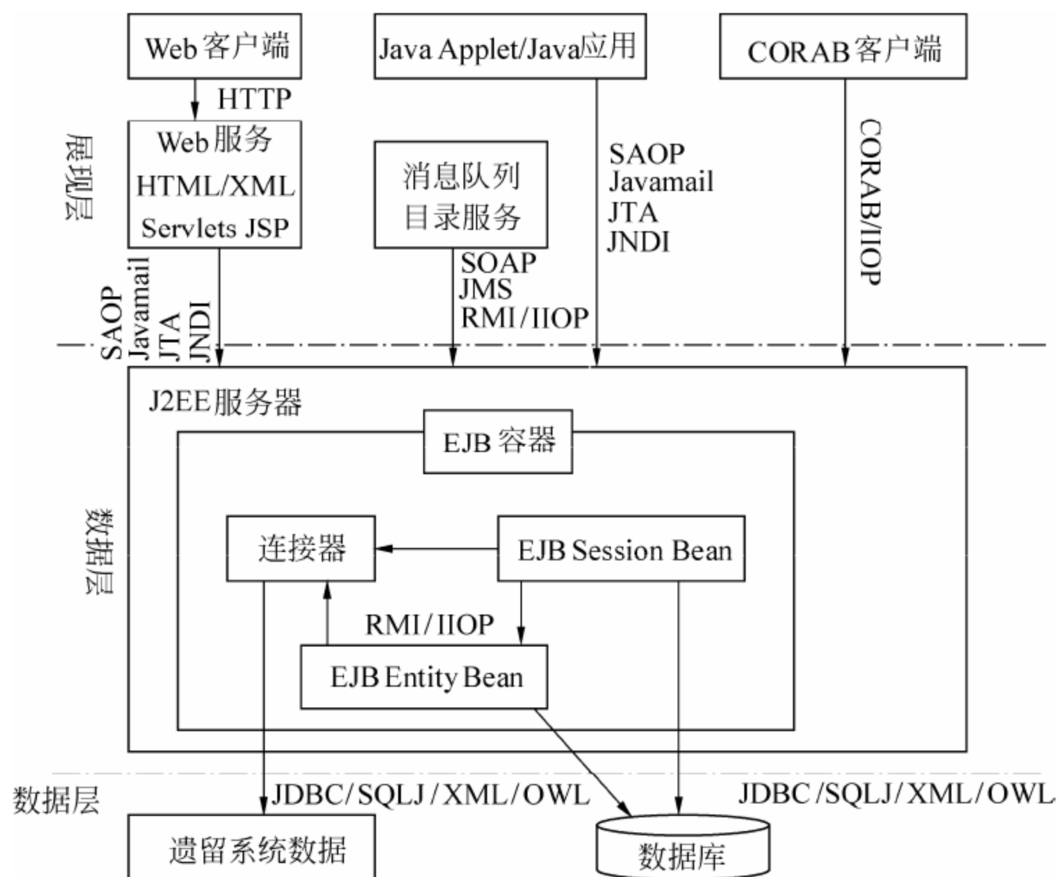
图 2-29 简化了的 J2EE 体系结构
