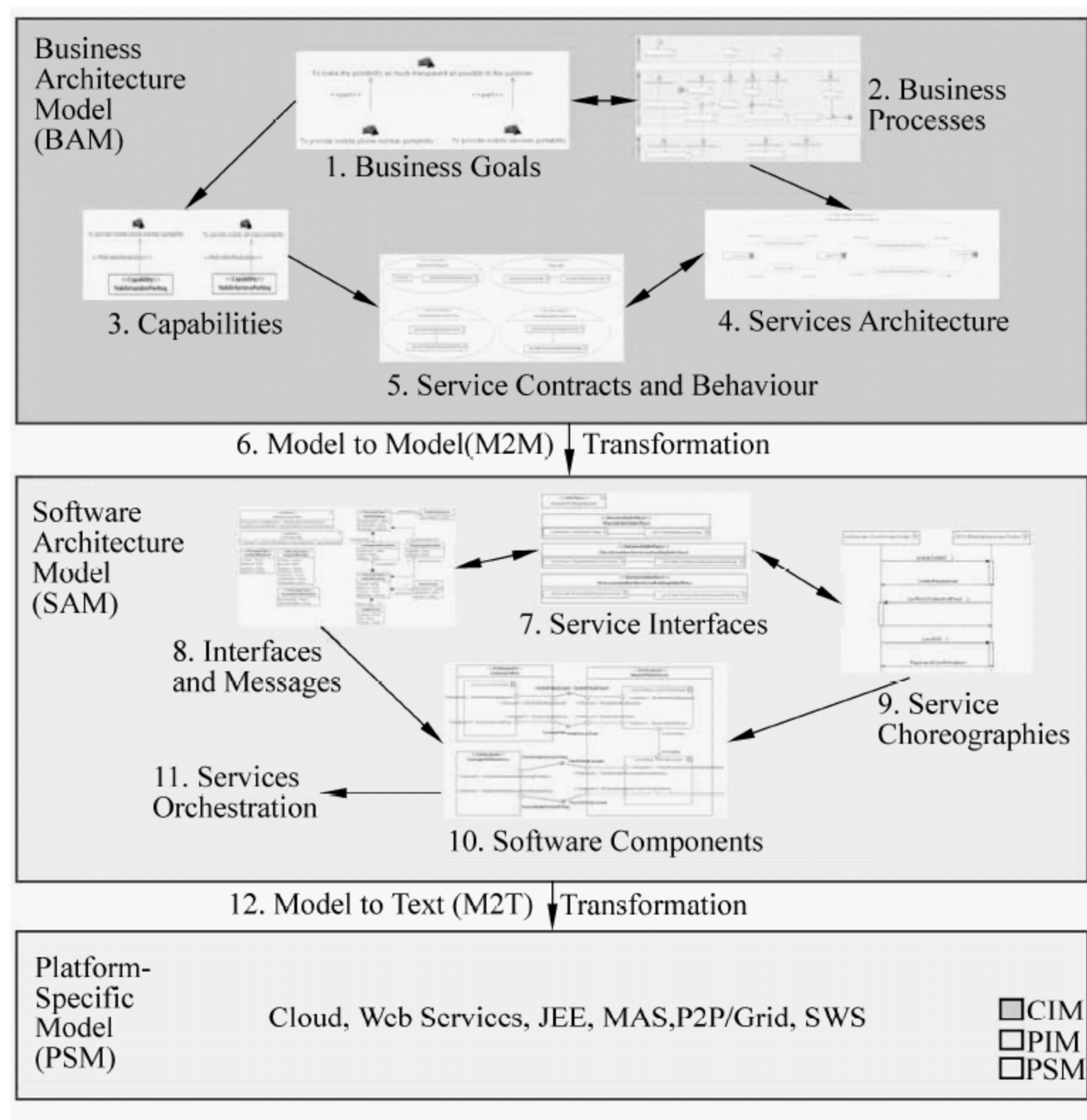
图 3-63 面向 SoaML 的 MDA 方法
