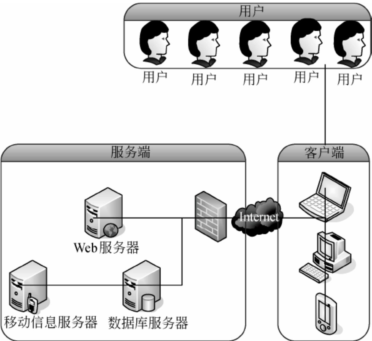
图 2-13 简化后的某项目档案管理系统网络拓扑图
