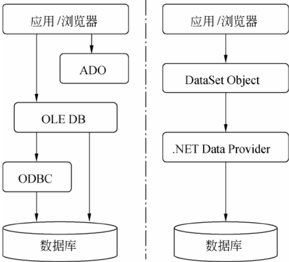
图 5-54 ADO 与 ADO.NET 结构比较
