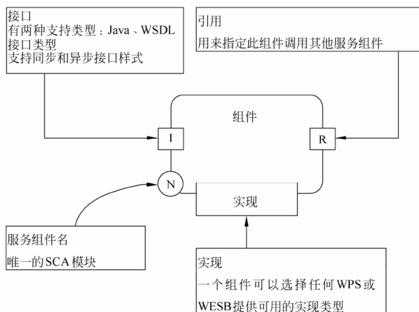
图 3-37 服务组件结构
