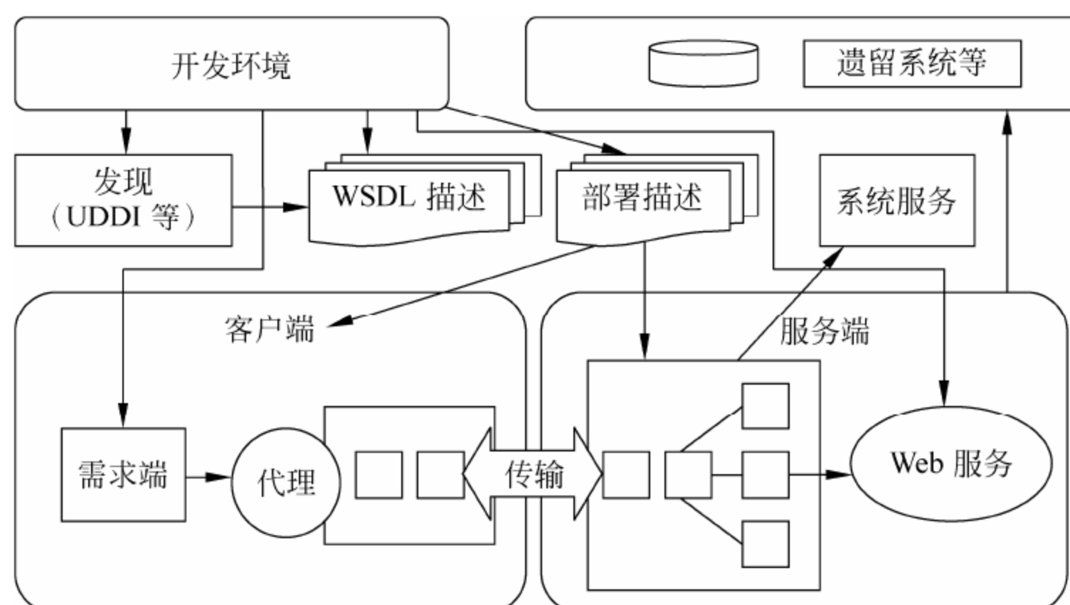
图 5-18 Web 服务体系结构
