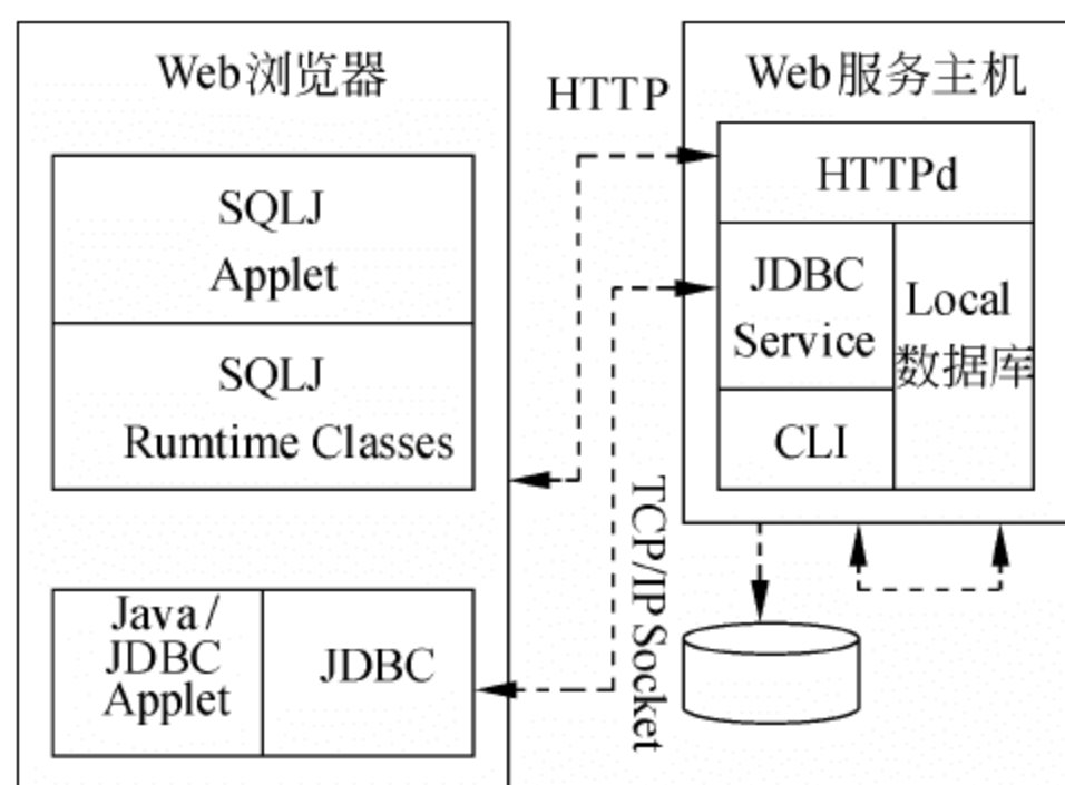
图 5-50 网络协议的驱动结构
