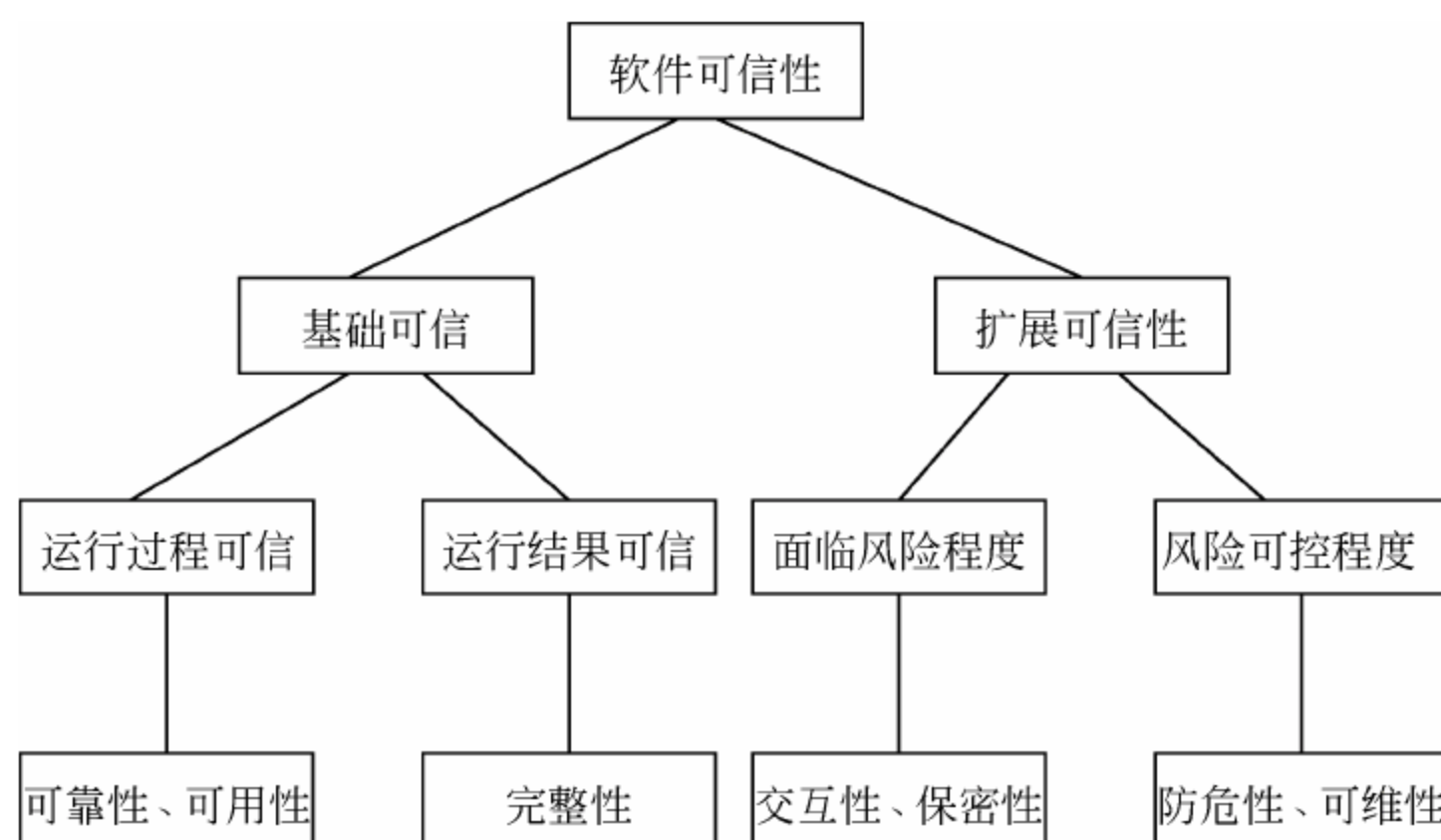
图 2-53 软件可信性结构模型图
