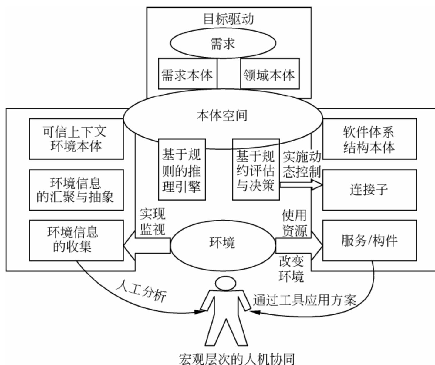
图 2-52 基于本体的可信软件动态演化框架
