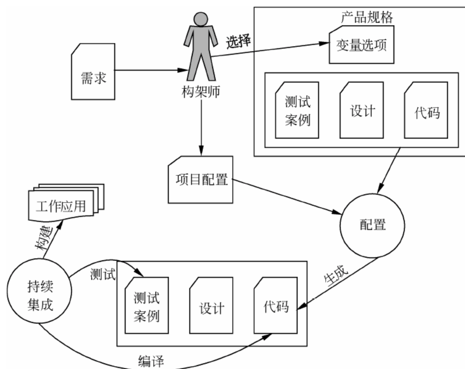
图 2-22 面向需求定制的构件组装模式
