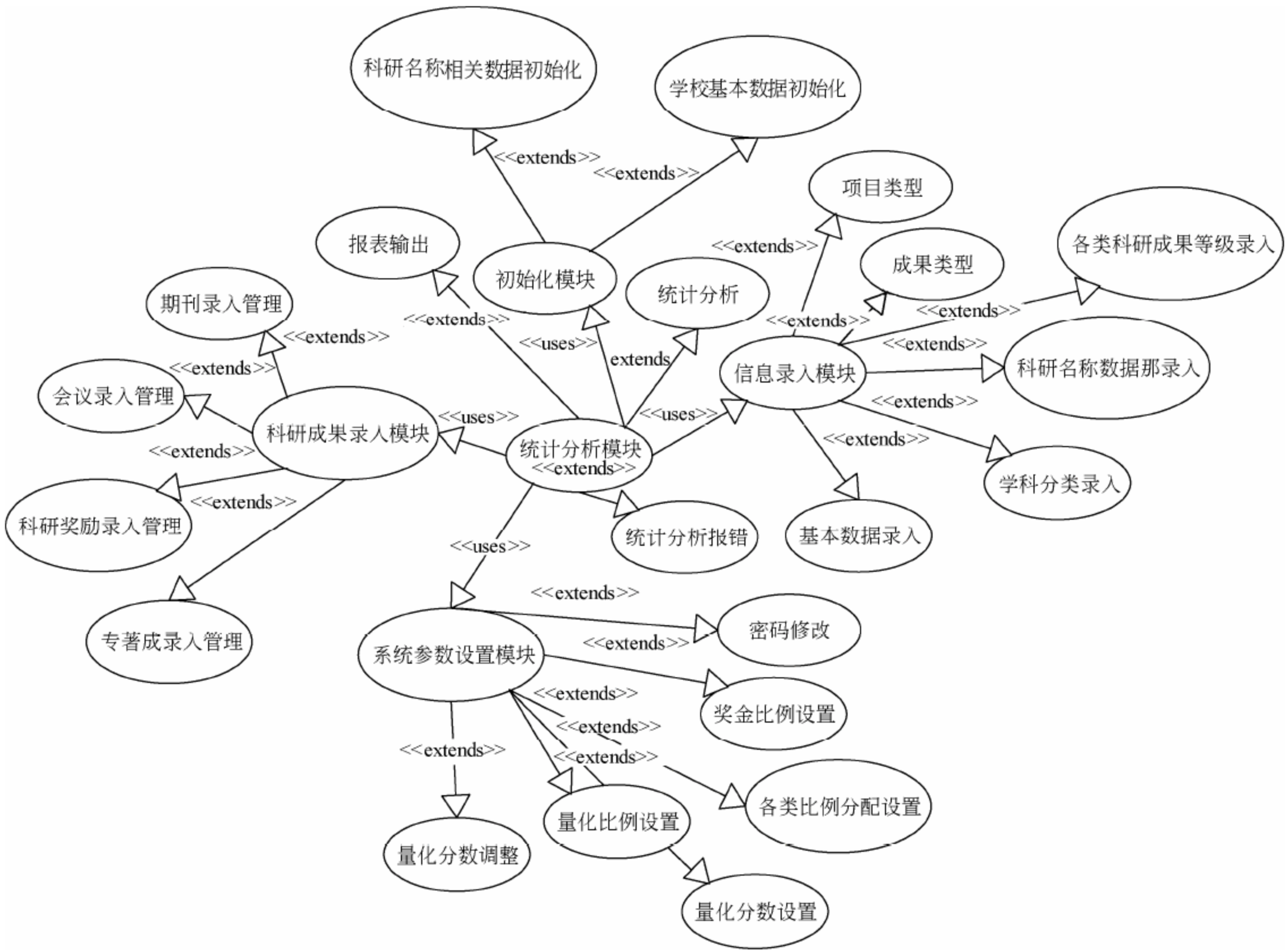
图 9-5 科研绩效统计分析功能用例图
