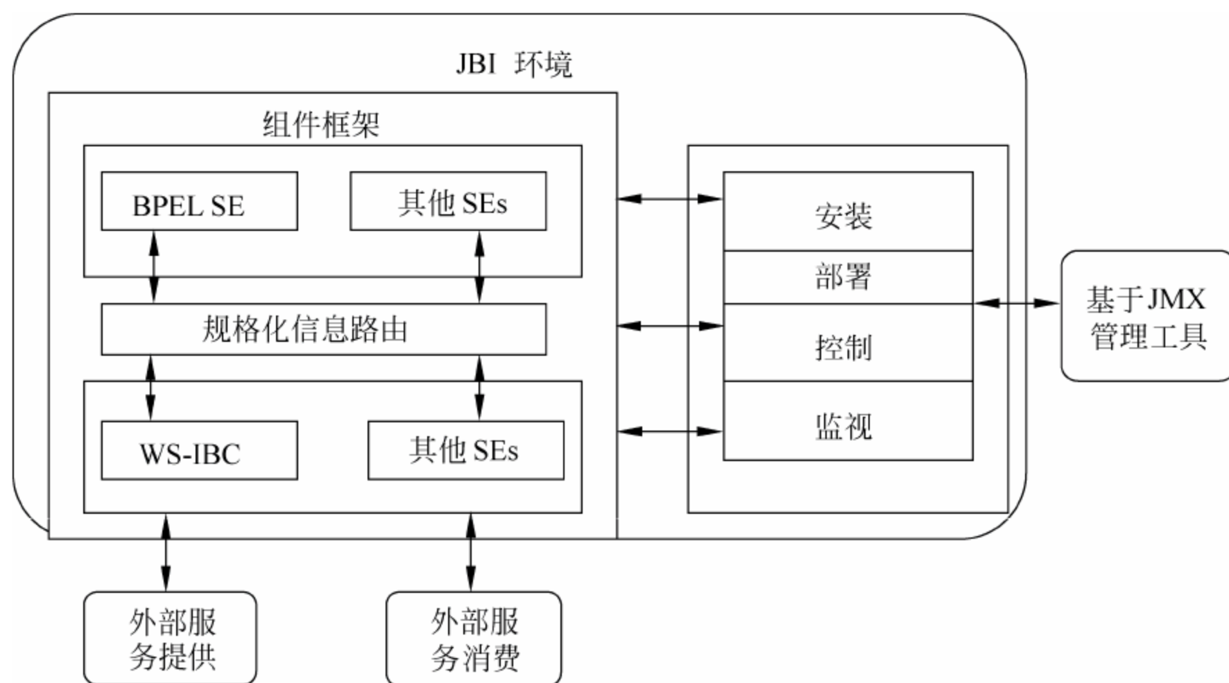
图 3-48 JBI 顶层结构图
