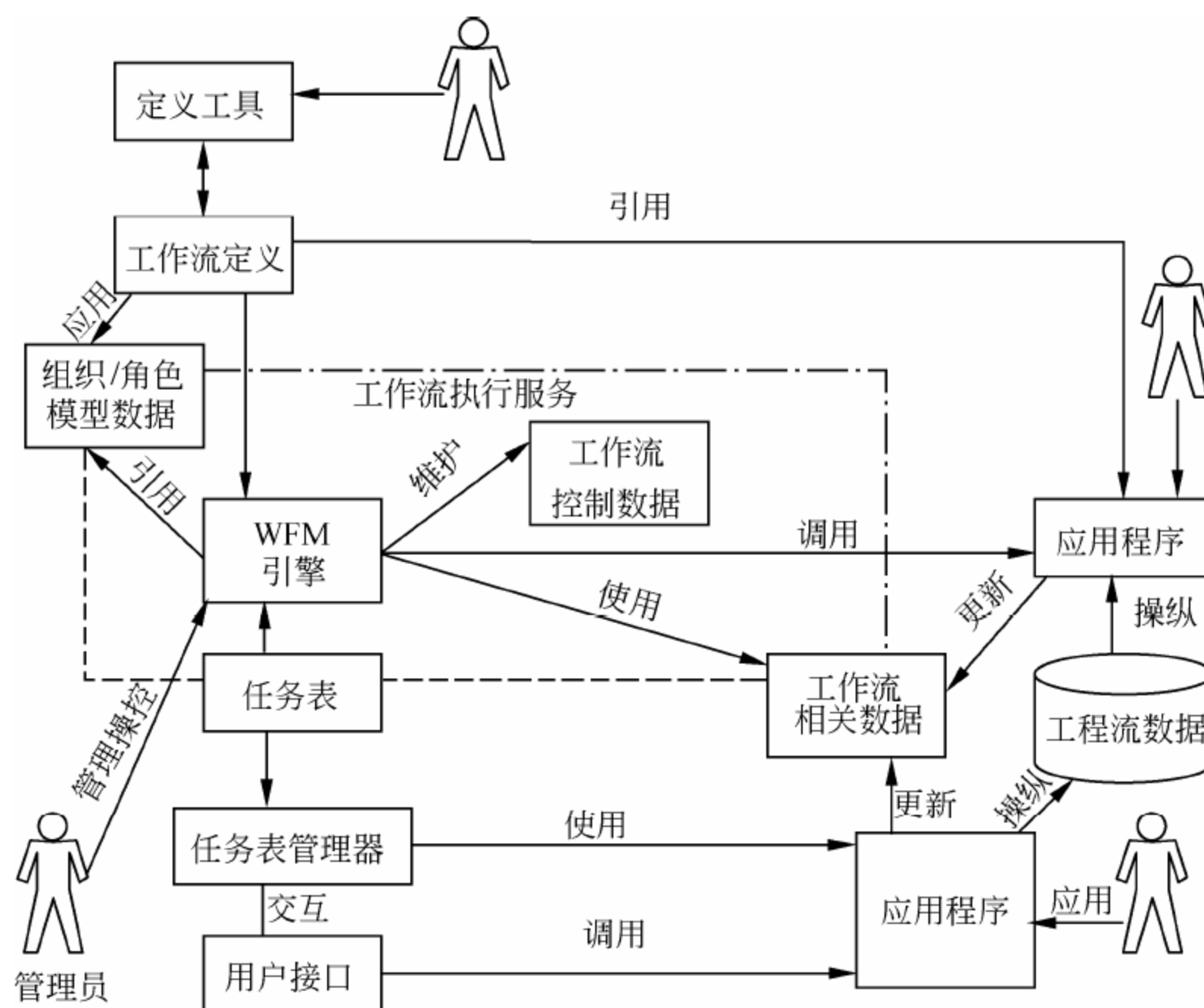
图 2-65 工作流实现模型
