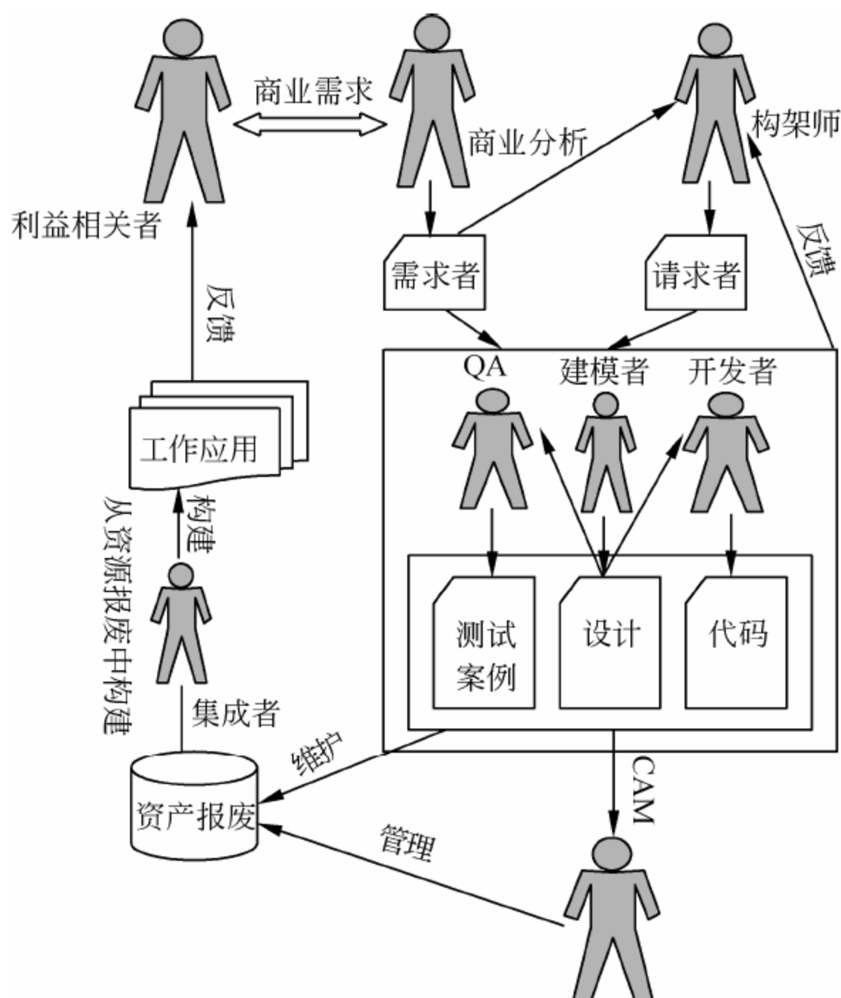
图 2-21 面向正式的方法的构件组装模式
