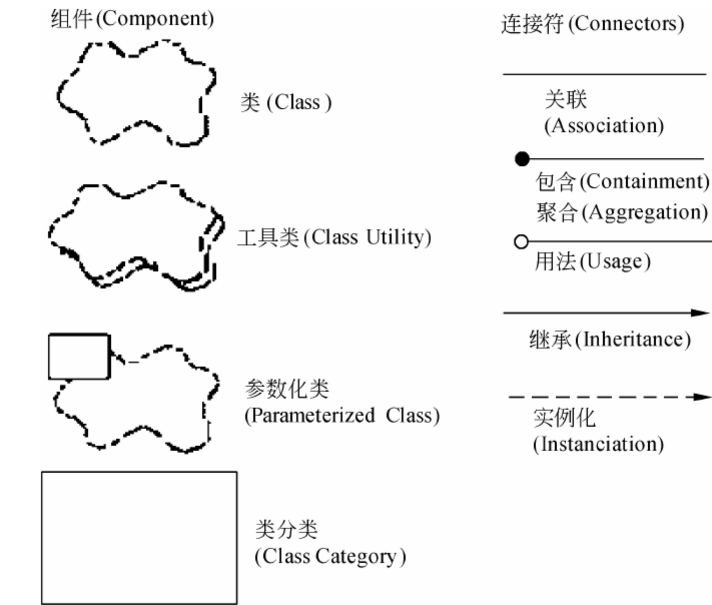
图 2-8 面向 Booch 的逻辑视图的标记法
