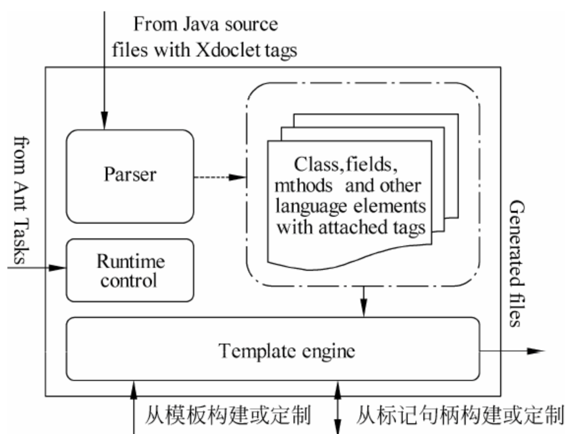
图 6-32 XDoclet 内部的功能块
