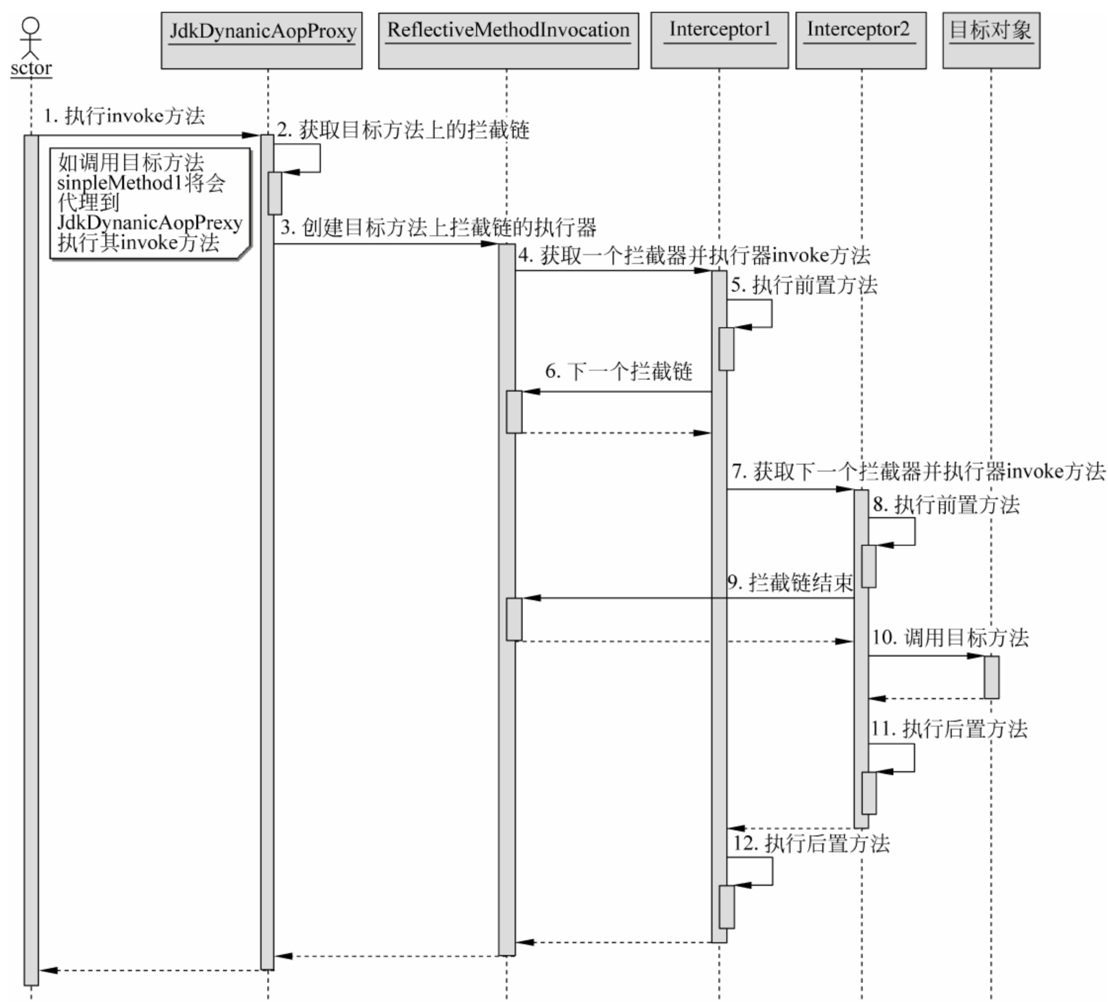
图 6-29 Spring 调用拦截器序列图
