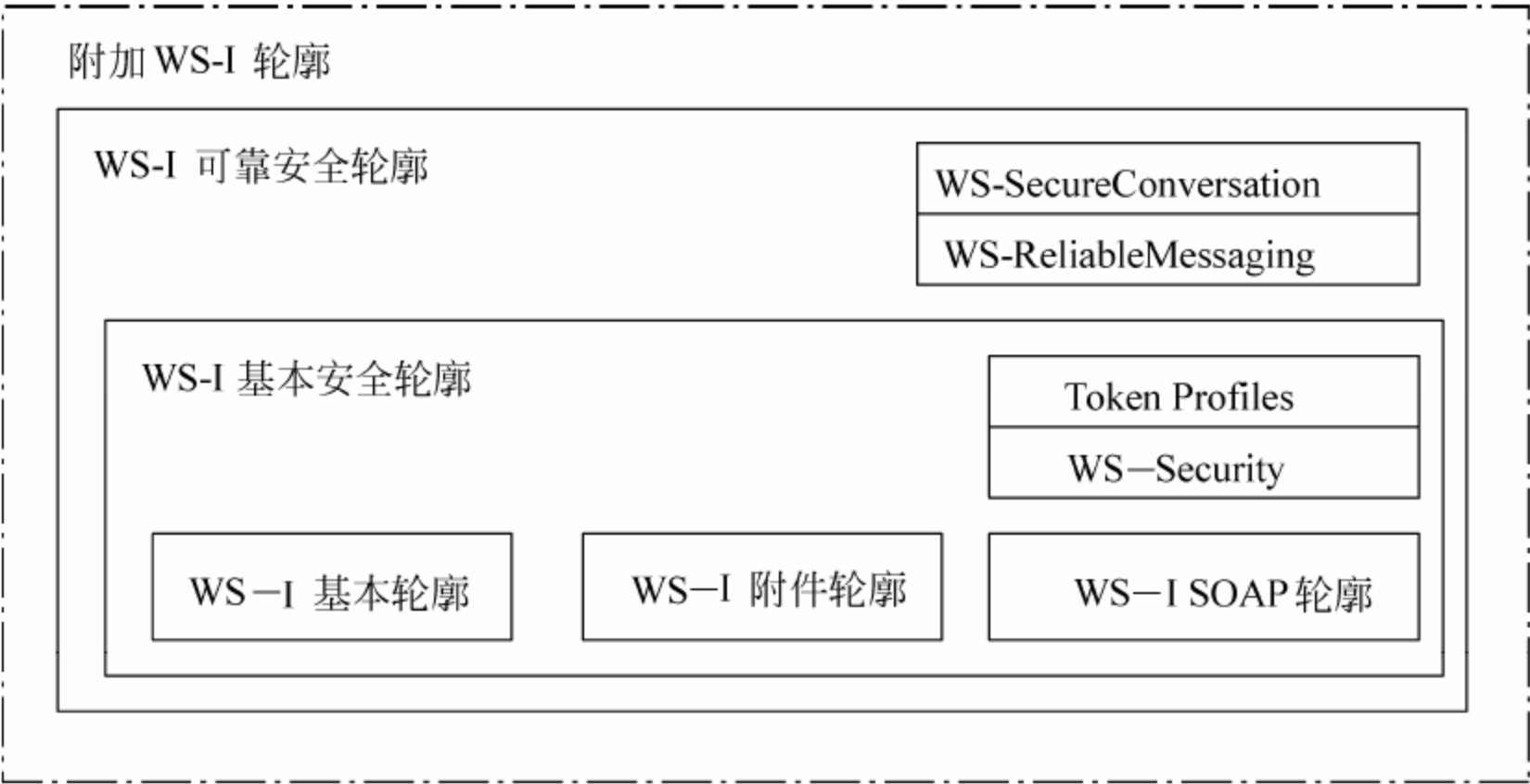
图 3-52 ESB 互操作轮廓图
