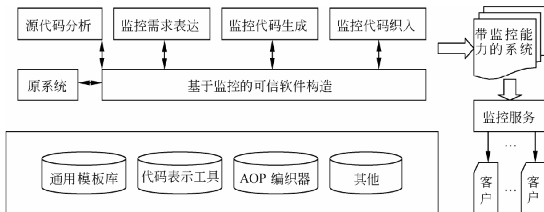
图 2-54 基于监控的可信软件构造模型 TSCM
