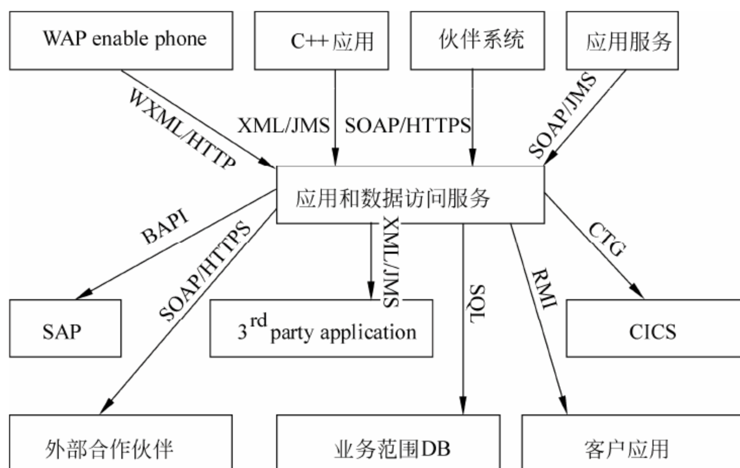
图 3-36 应用程序和数据访问服务
