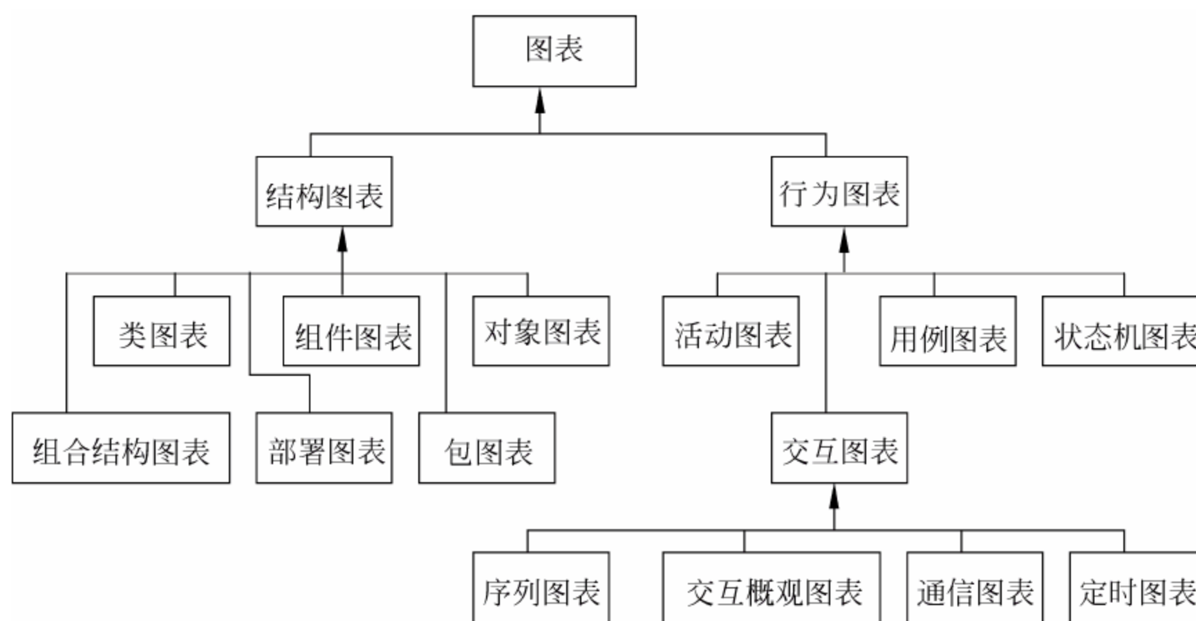
图 3-19 UML 图示结构
