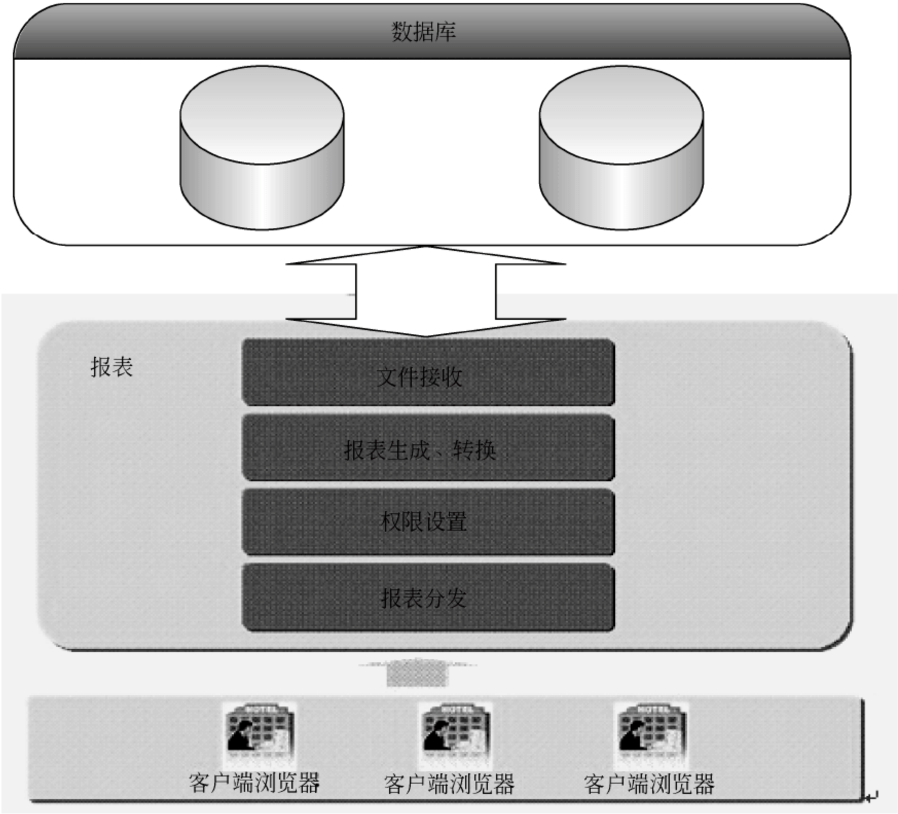
图 2-17 某项目档案管理系统报表输出结构图
