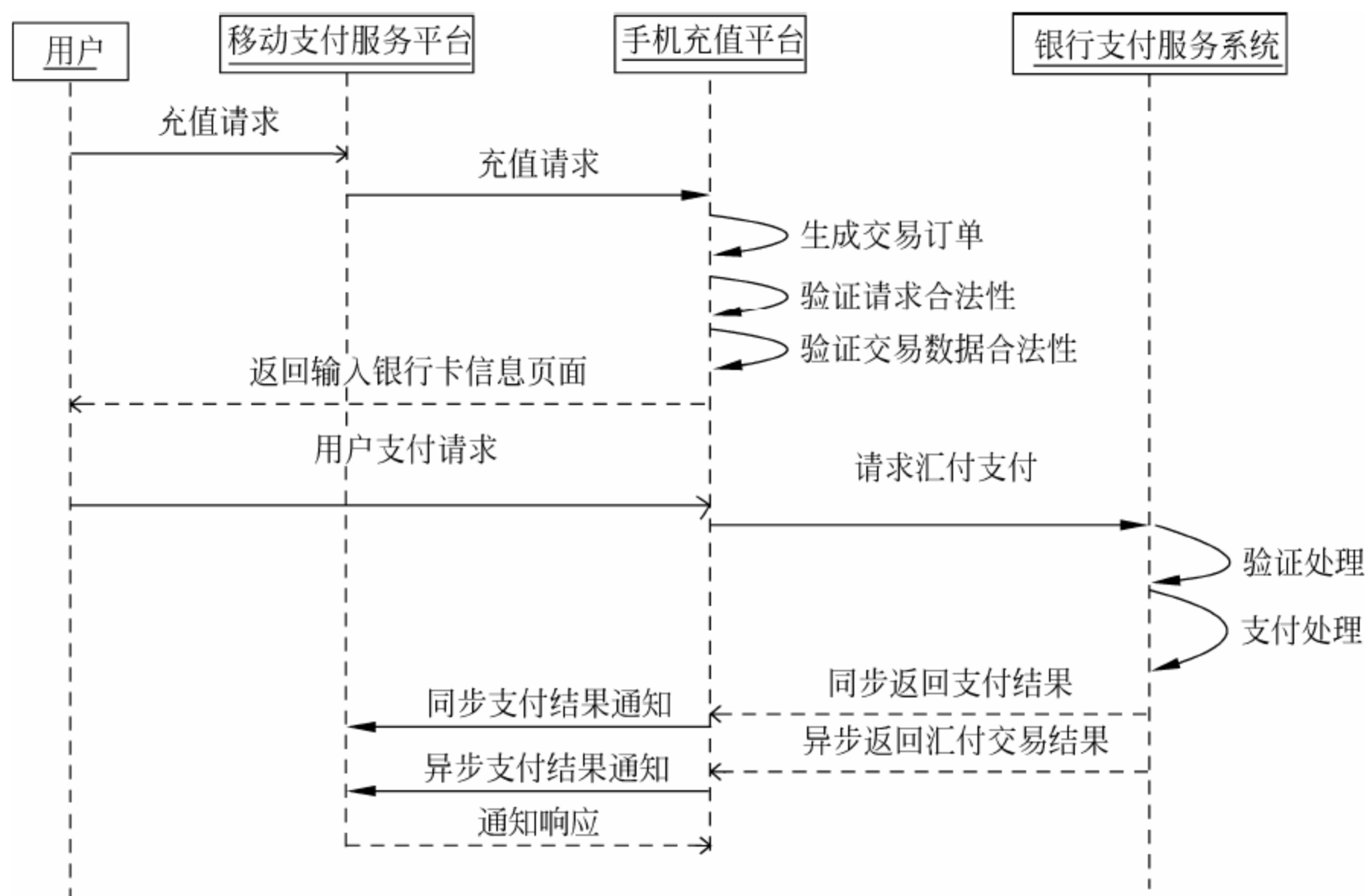
图 3-22 面向手机支付平台的时序图
