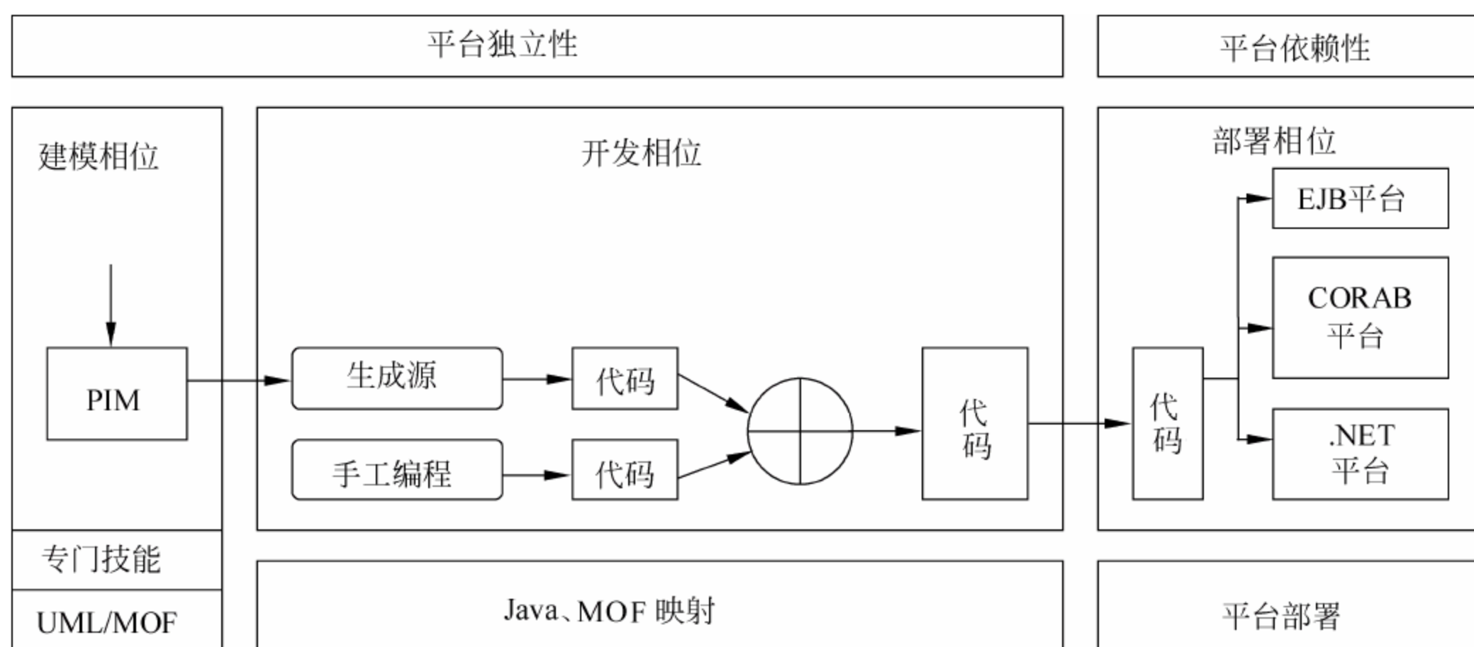
图 3-17 OpenMDX 开发流程
