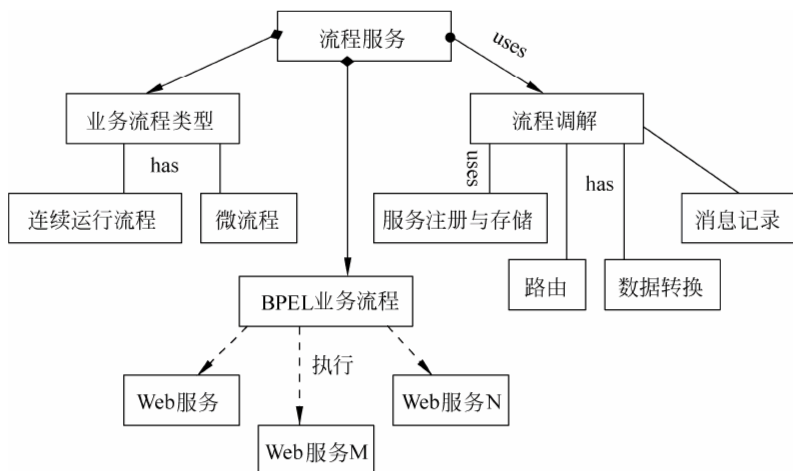
图 3-32 流程服务
