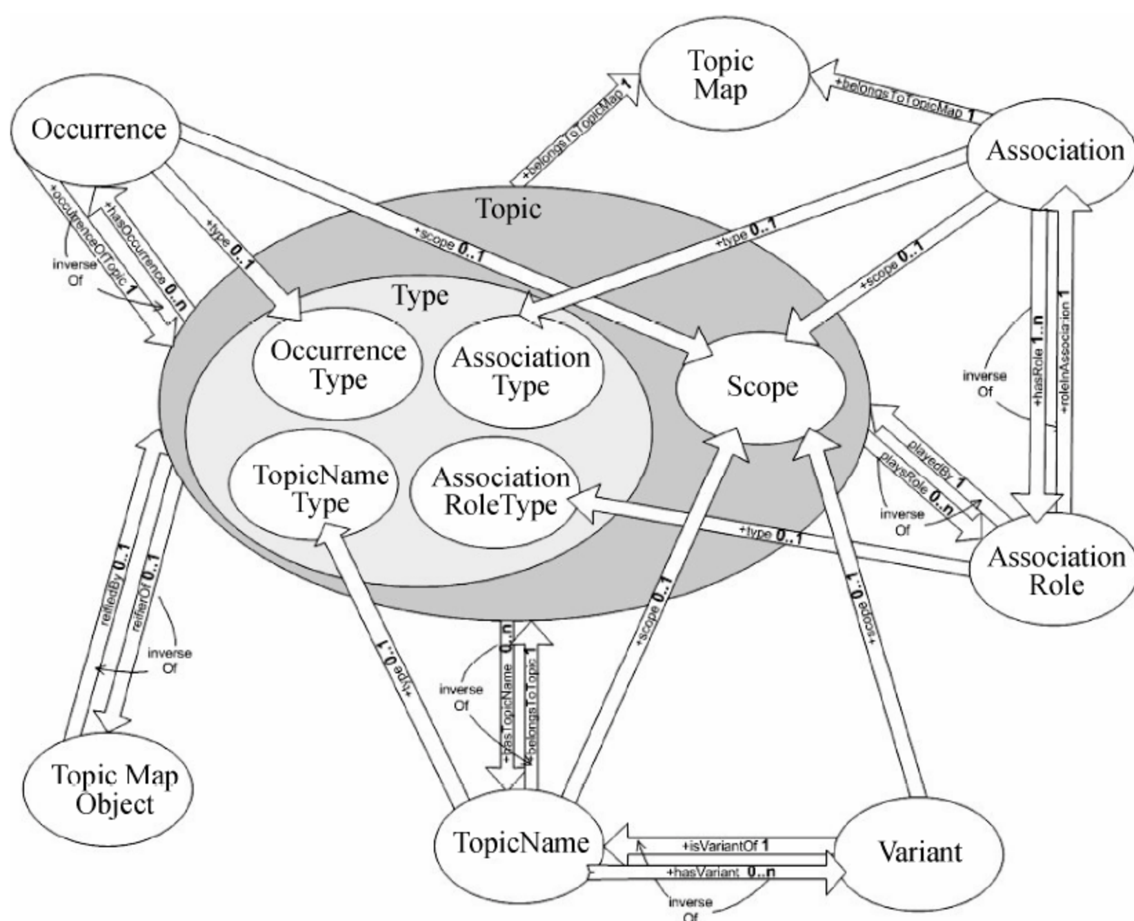
图 3-76 TMDM 结构图
