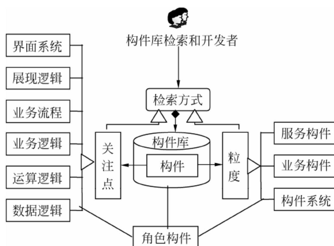
图 2-31 构件组织图
