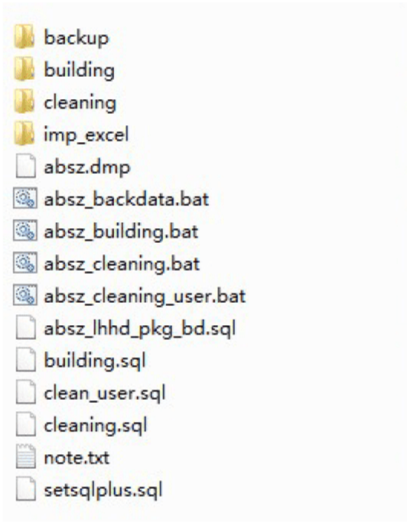
图 9-8 数据库结构
