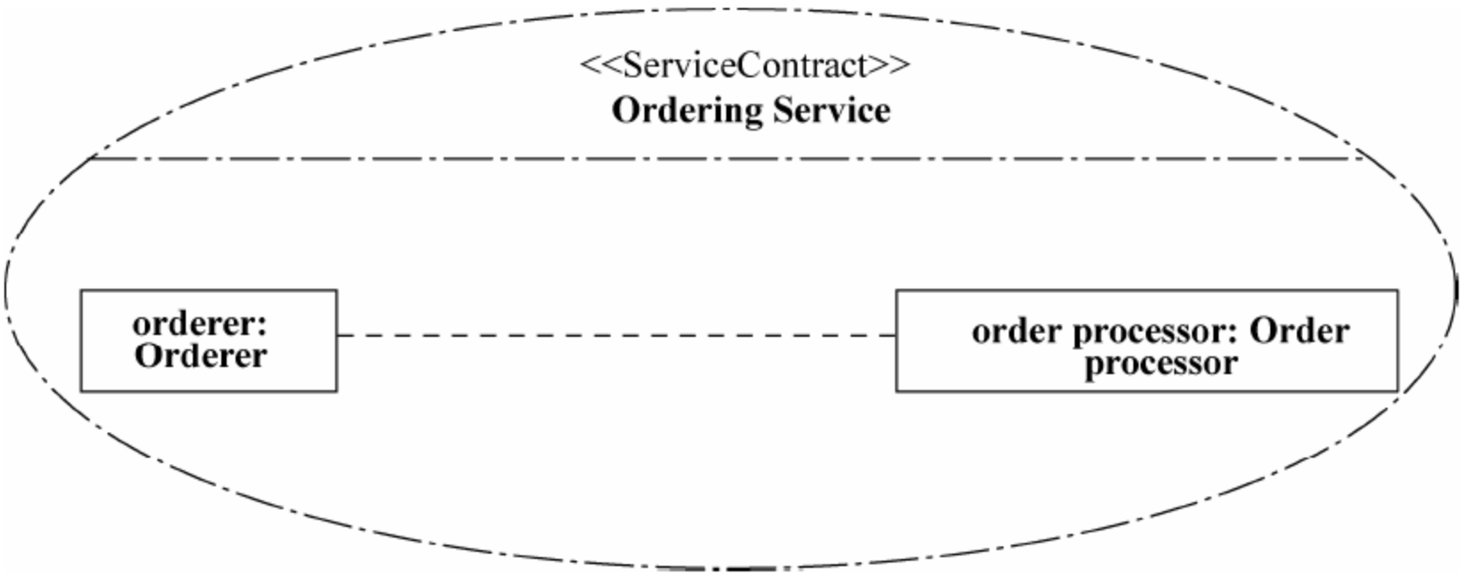
图 3-66 订购商服务
