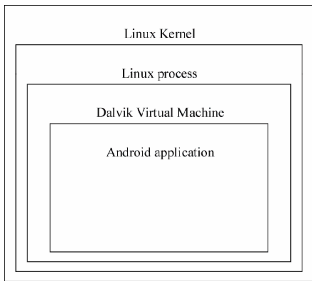
图 5-4 Dalvik VM
