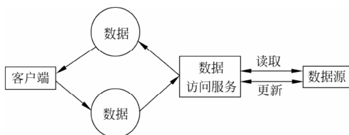
图 5-31 SDO 结构
