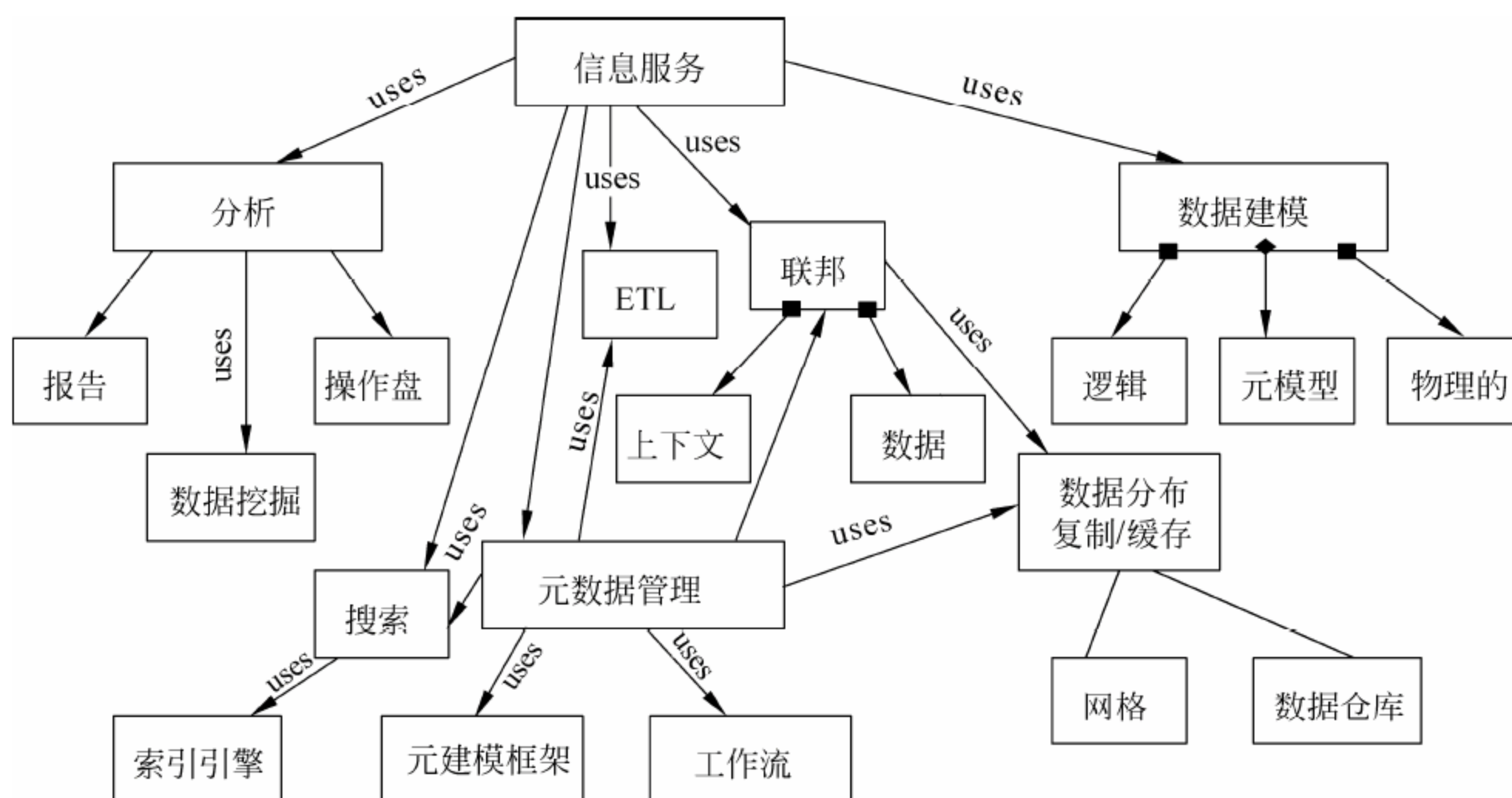
图 3-33 信息服务
