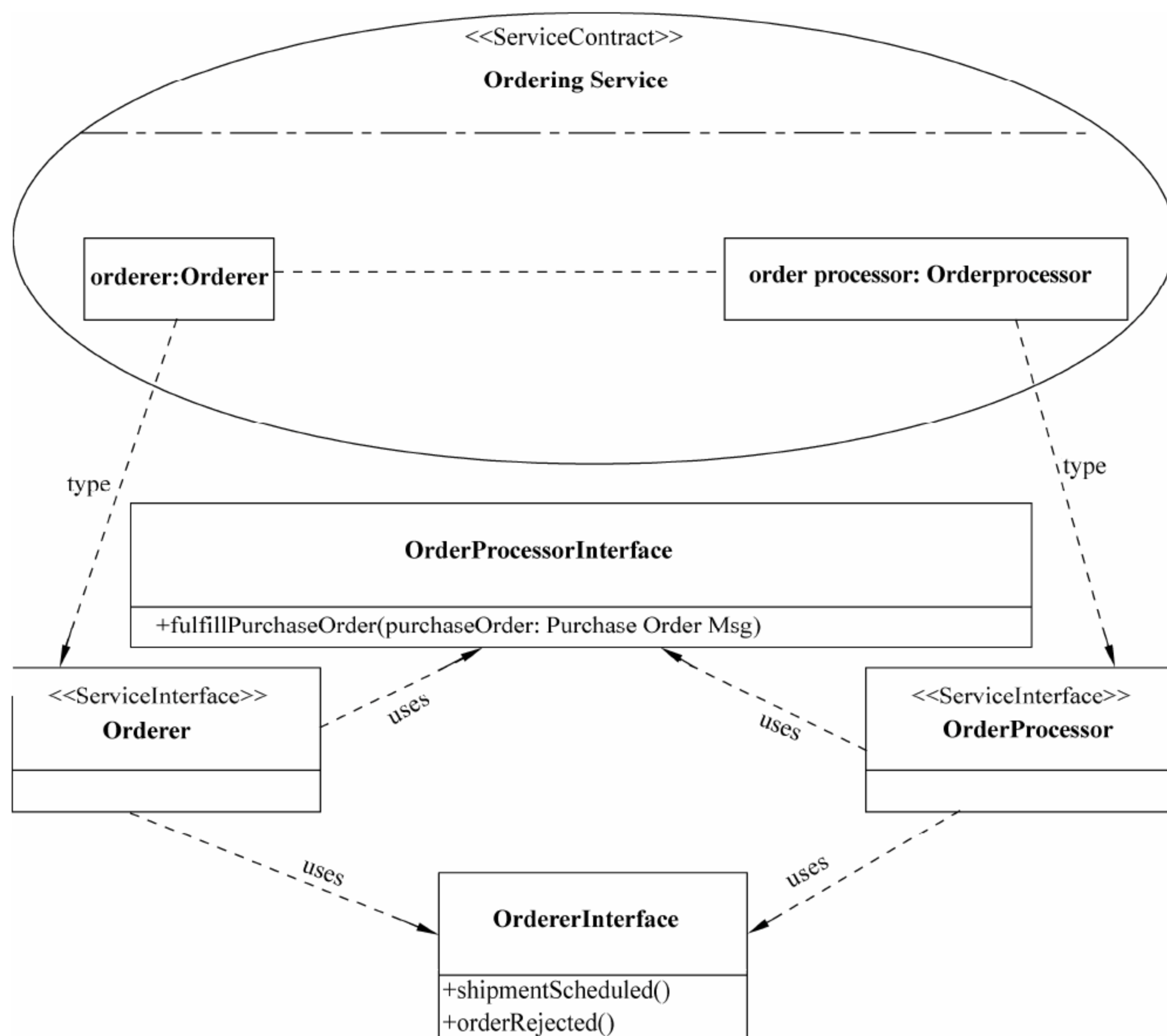
图 3-68 服务接口
