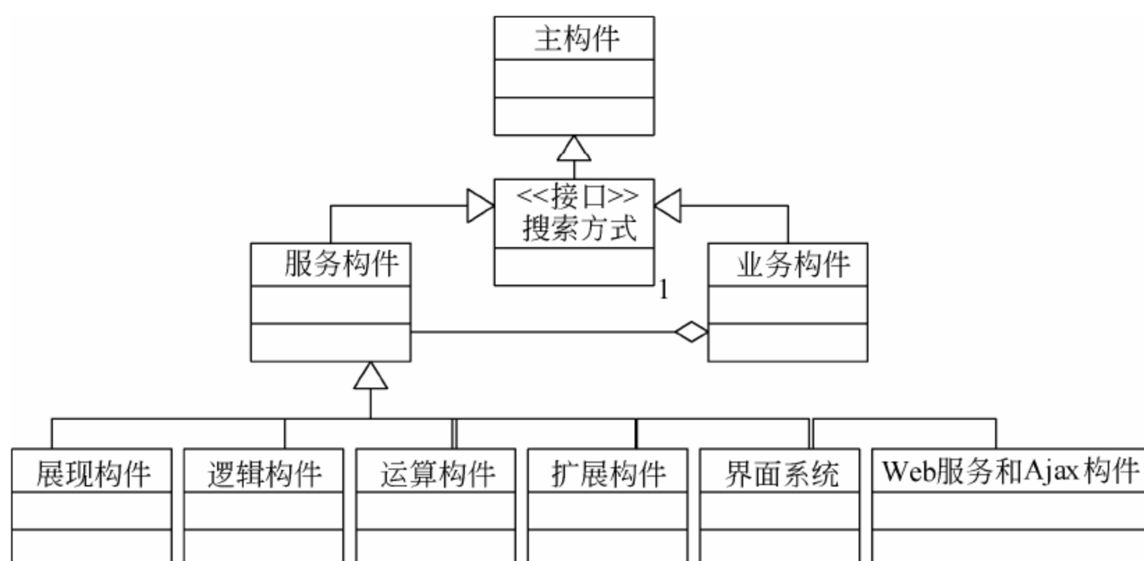
图 2-23 构件类型
