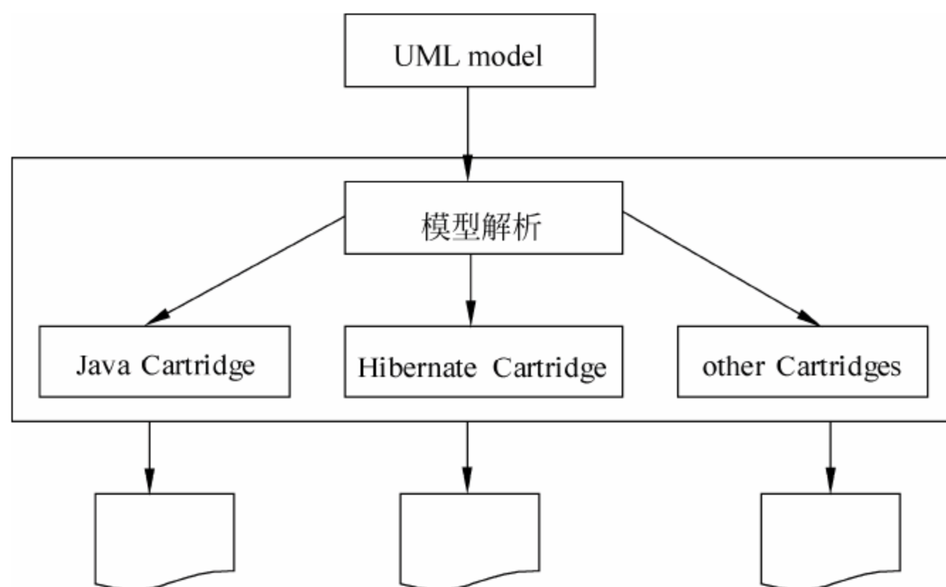
图 3-16 AndroMDA 结构图
