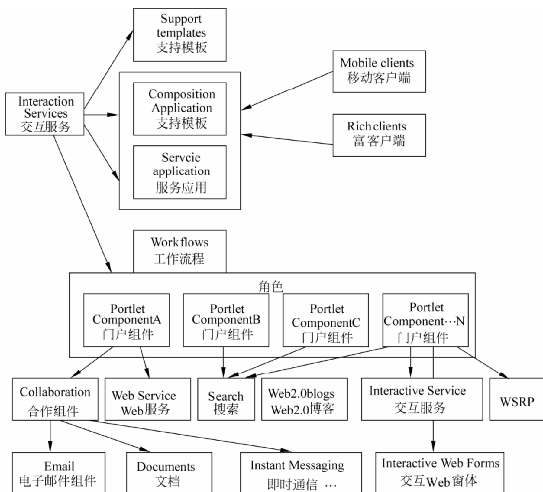
图 3-31 交互服务
