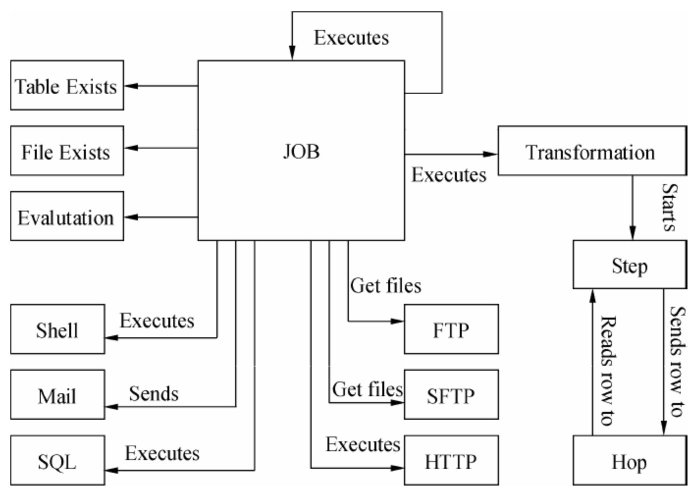
图 6-58 Kettle 结构图
