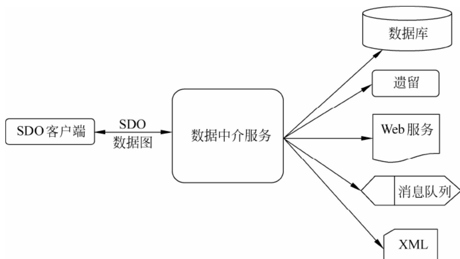
图 5-34 DMS 结构
