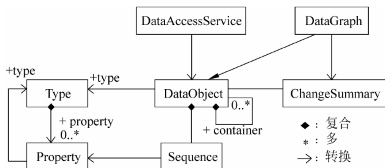
图 5-33 SDO API
