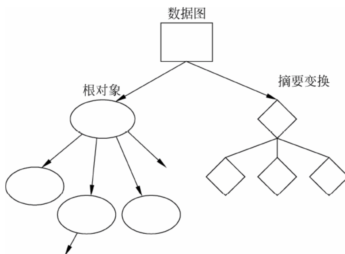
图 5-32 SDO 数据图
