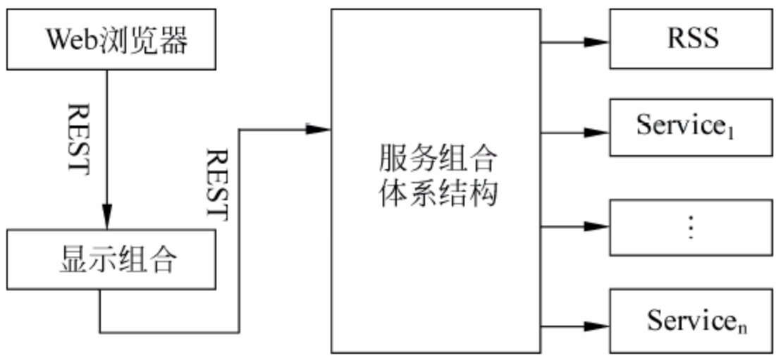
图 5-27 SCA 关系图
