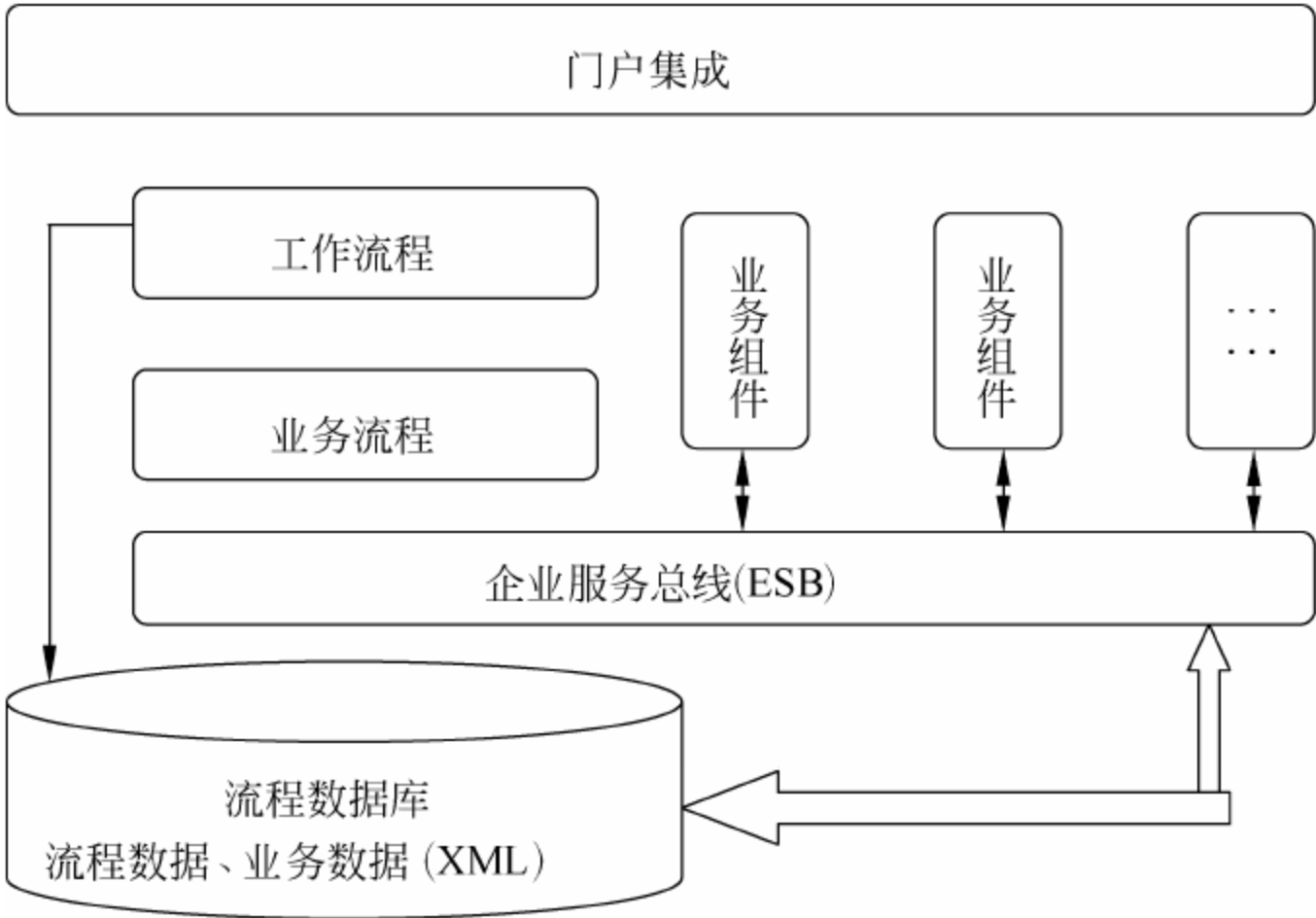
图 3-43 流程整合
