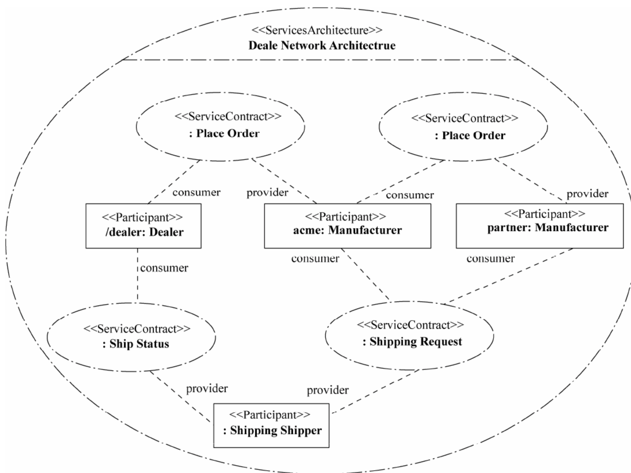
图 3-61 SoaML 联系图
