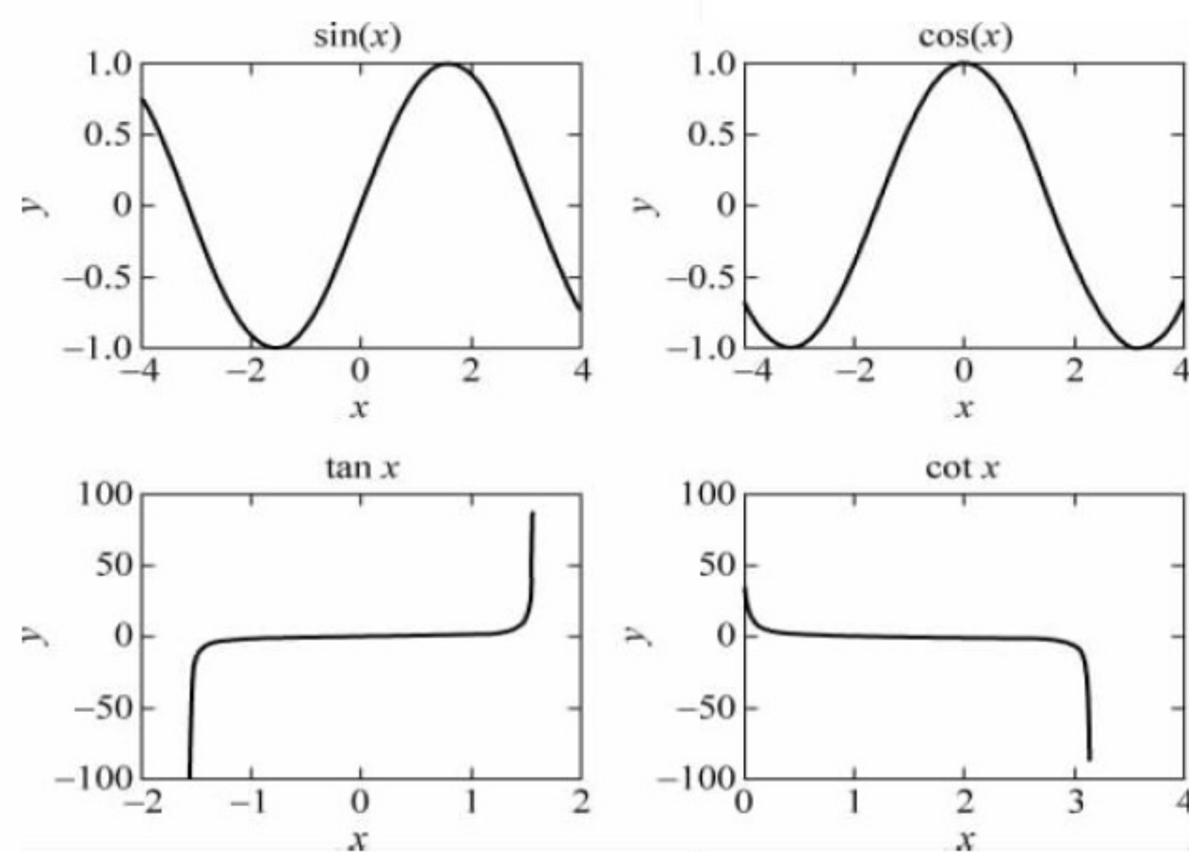
图 3-26 子图
