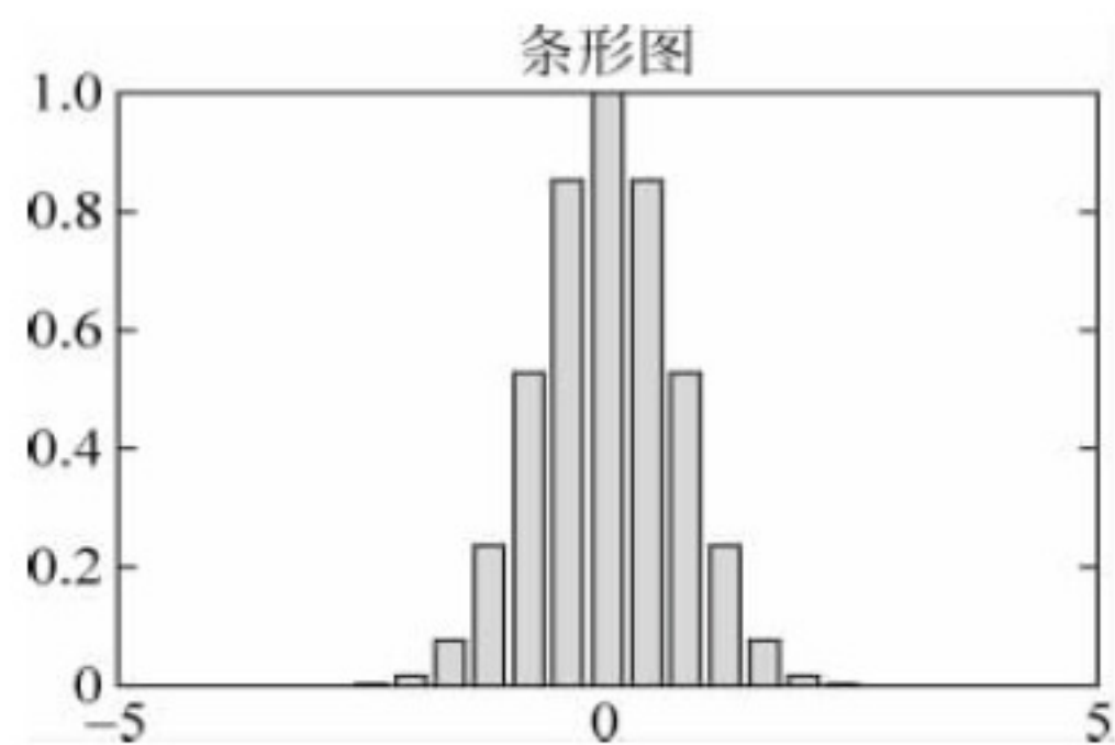
图 3-36 条形图
