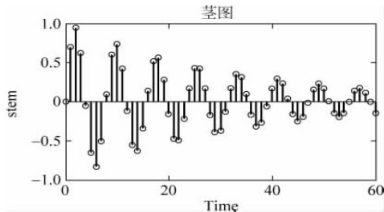
图 3-5 二维的茎图
