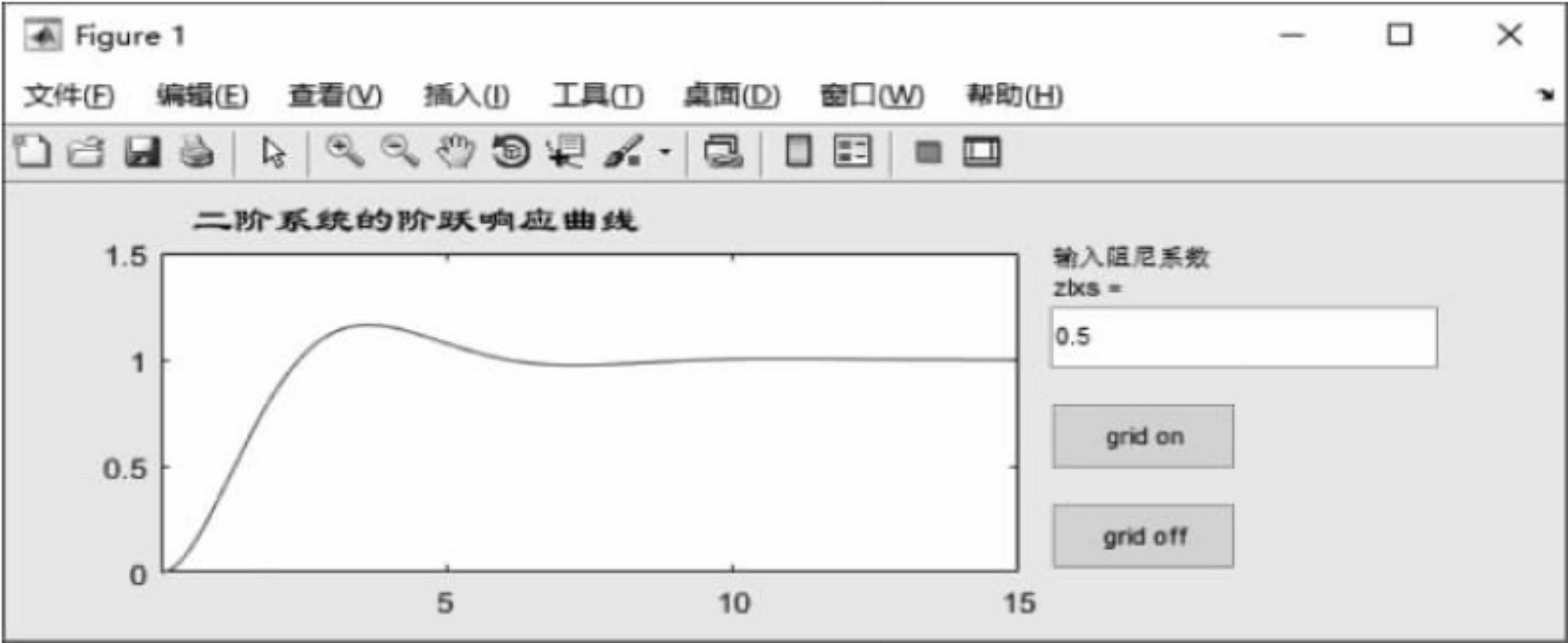
图 4-16 使用该界面
