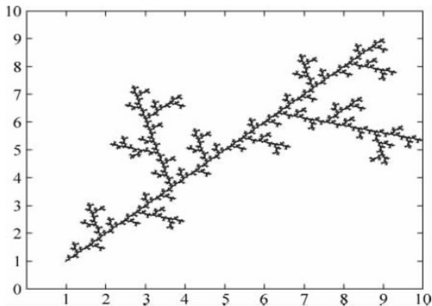
图 17-7 树形图
