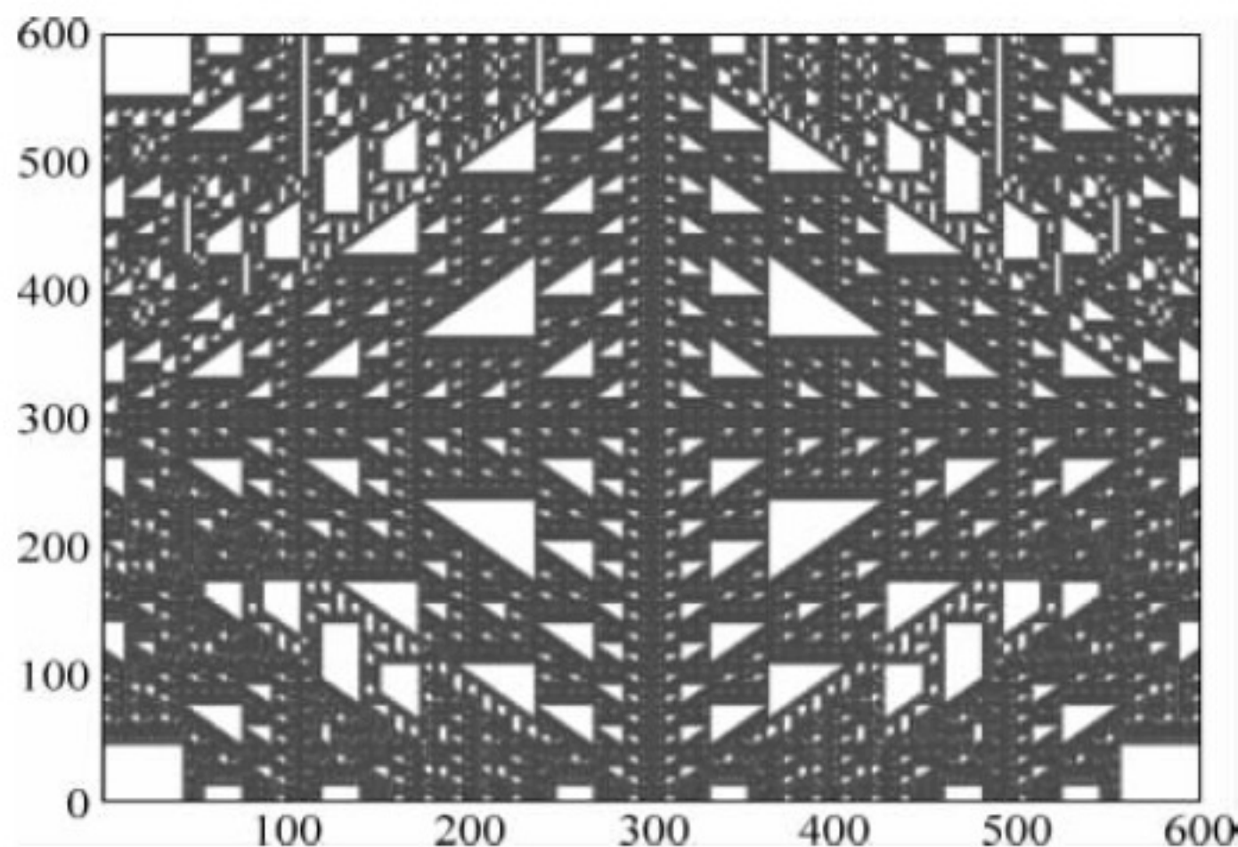
图 17-12 Sierpinski 三角形
