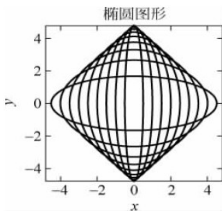
图 3-13 椭圆图形
