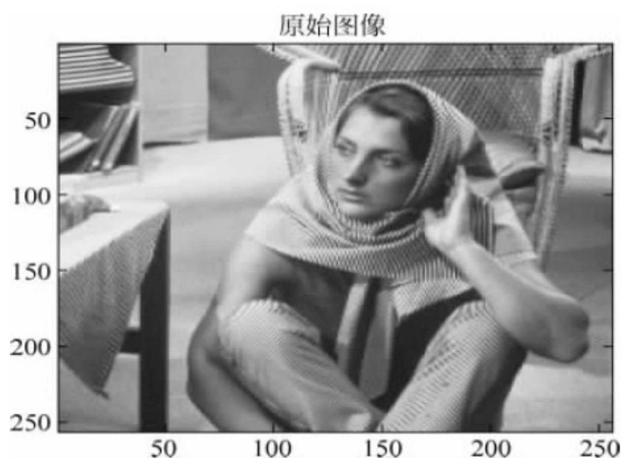
图 15-5 原始图像
