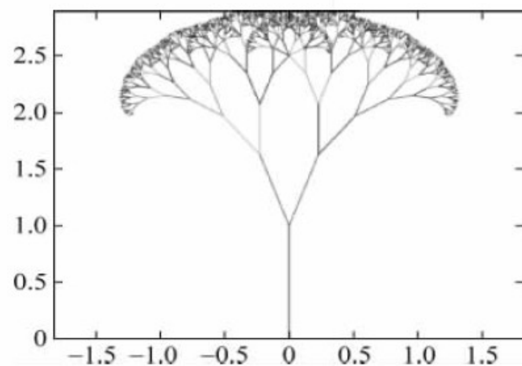
图 17-6 树形图
