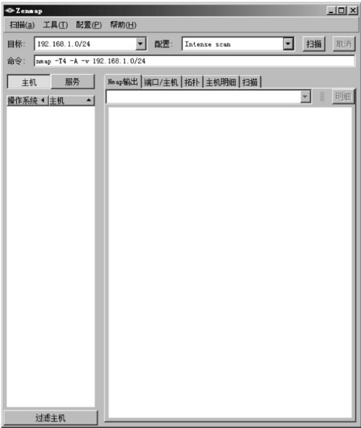
图 5-4 扫描参数设置——检测范围
