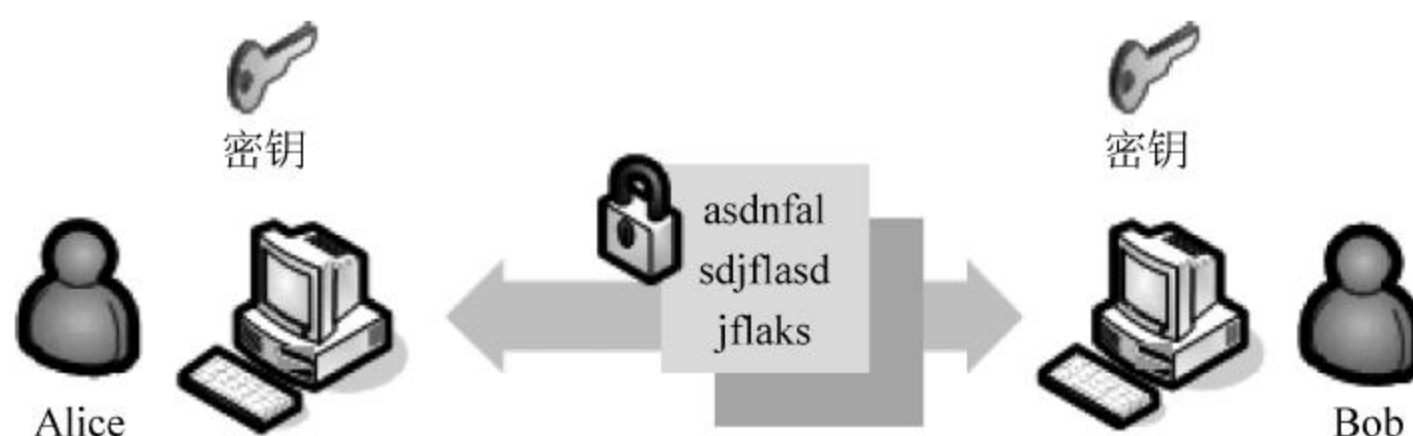
图 3-4 对称密码模型
