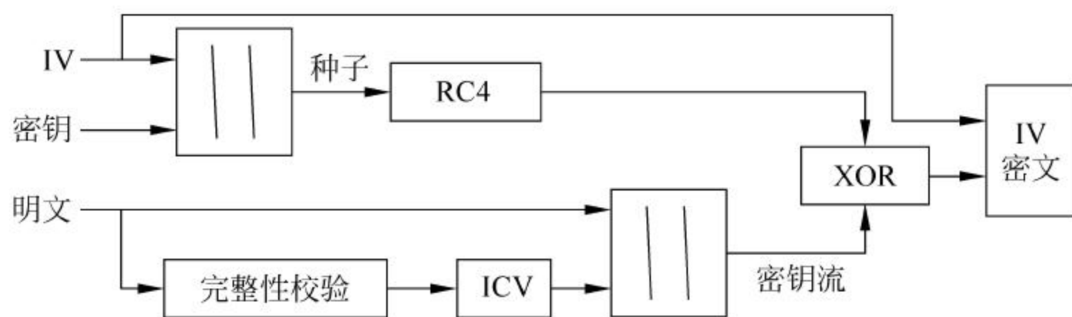
图 9-3 WEP 加密过程
