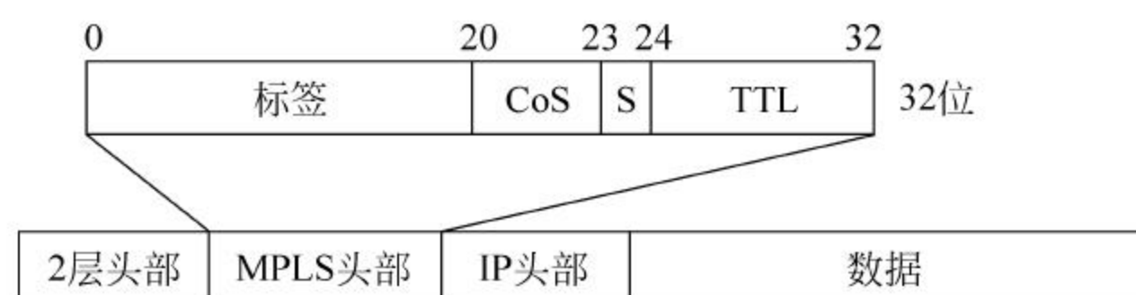
图 8-14 MPLS 协议示意图
