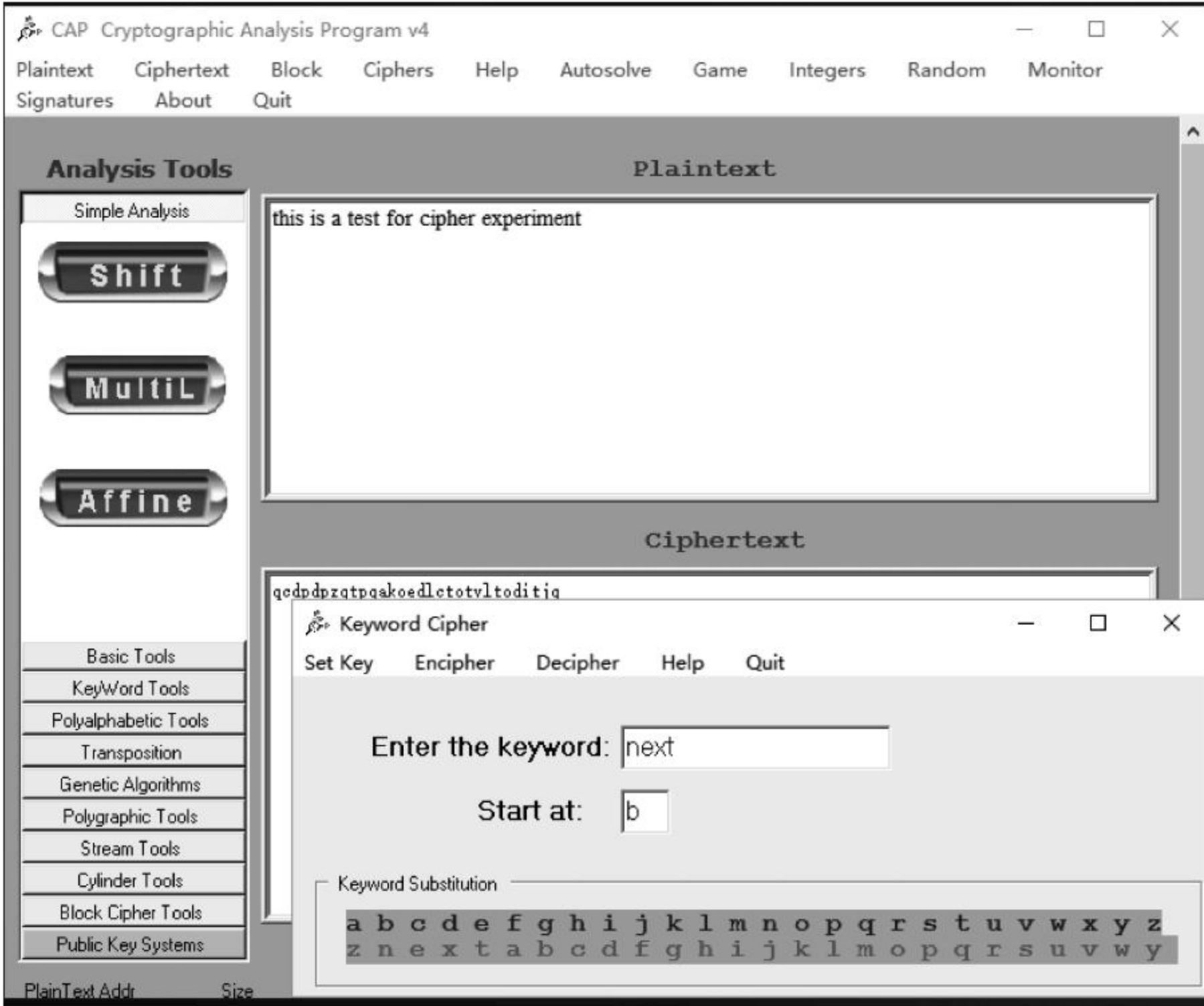
图 3-24 对明文加密
