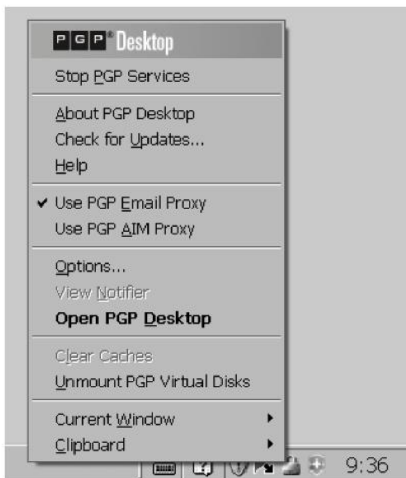
图 3-28 PGP 菜单
