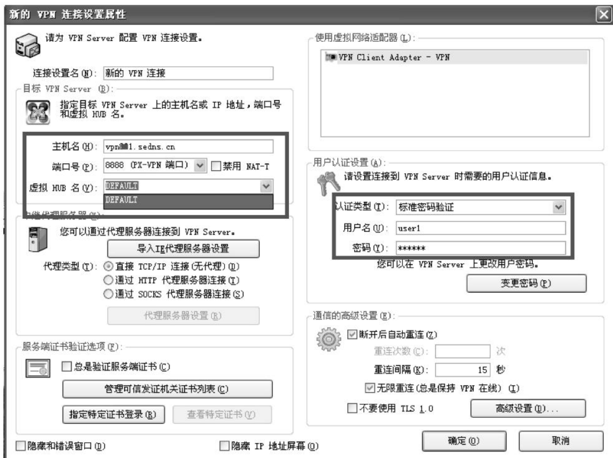
图 8-39 VPN 连接配置界面
