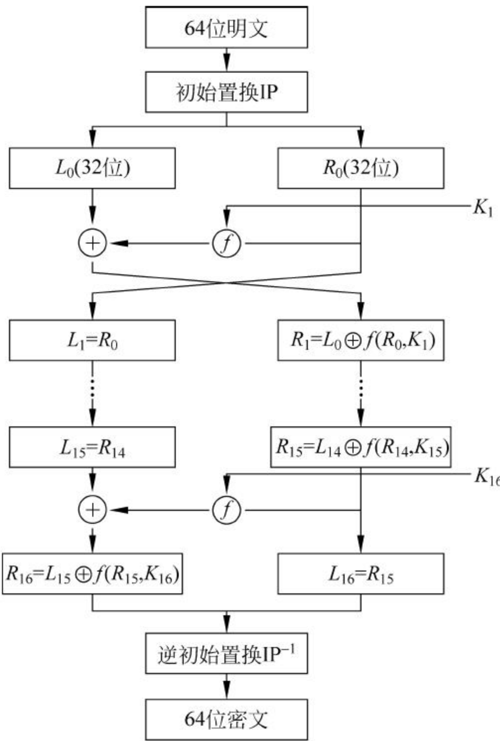
图 3-11 DES 算法的乘积变换
