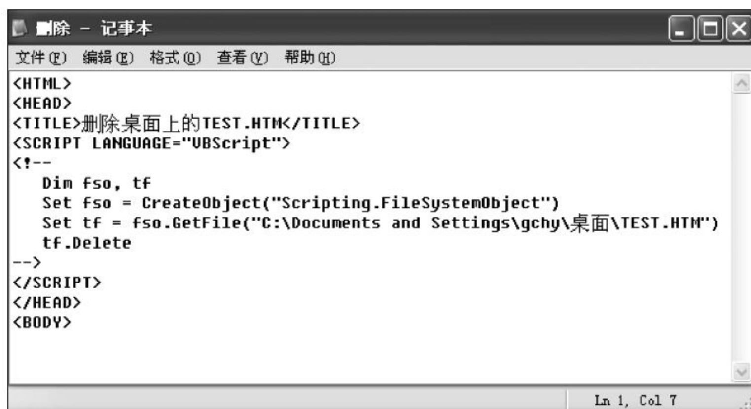
图 11-4 在记事本文件“删除”中输入内容
