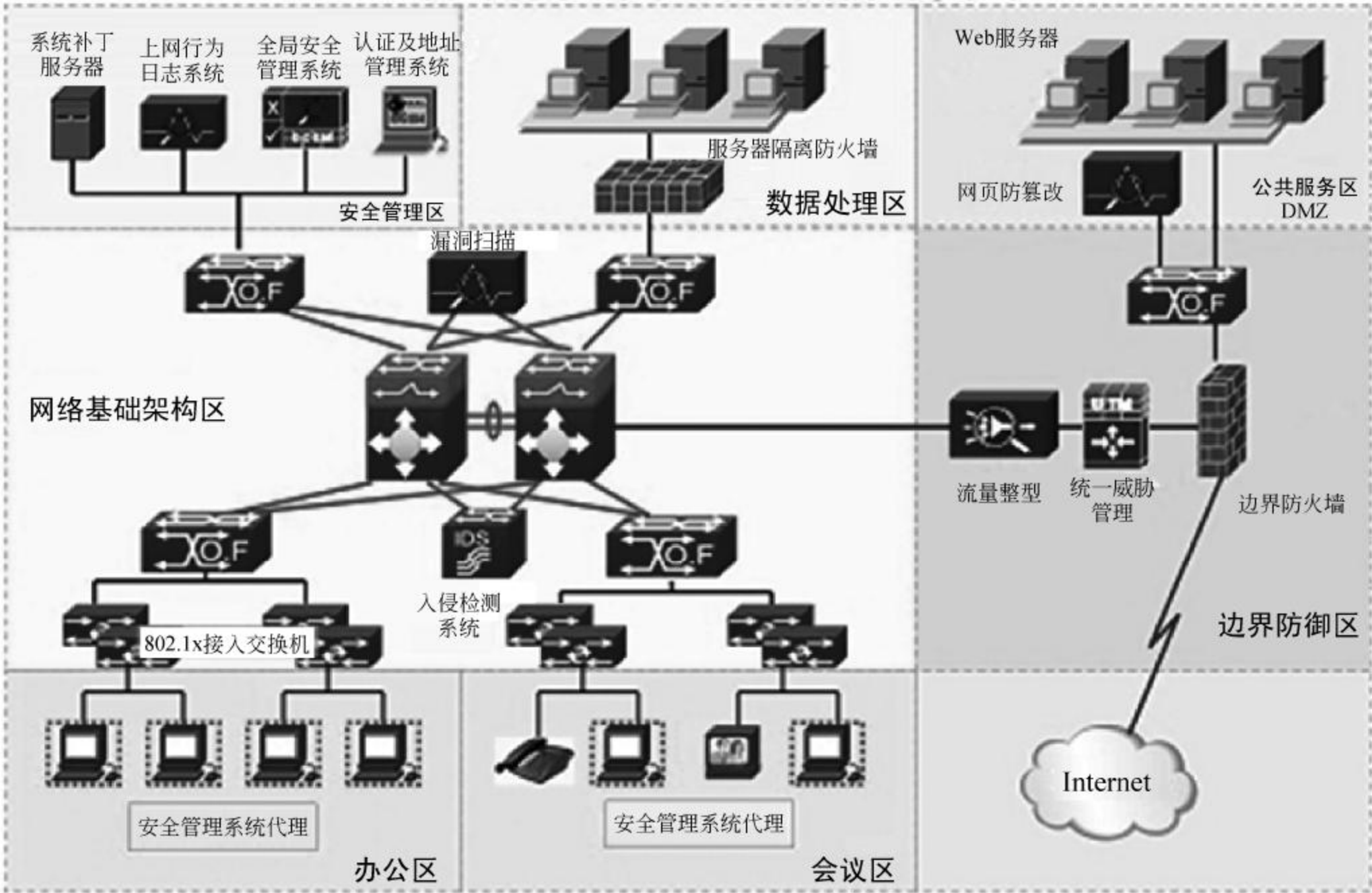
图 13-8 三级电子政务外网的拓扑结构
