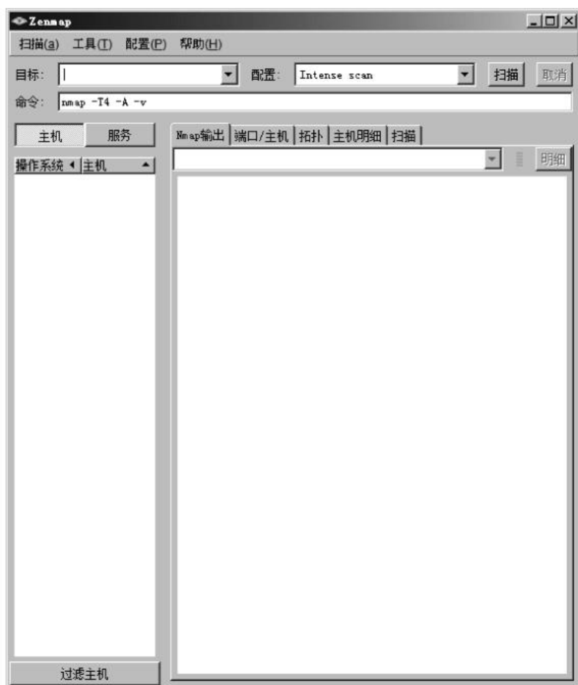
图 5-3 Nmap 主界面
