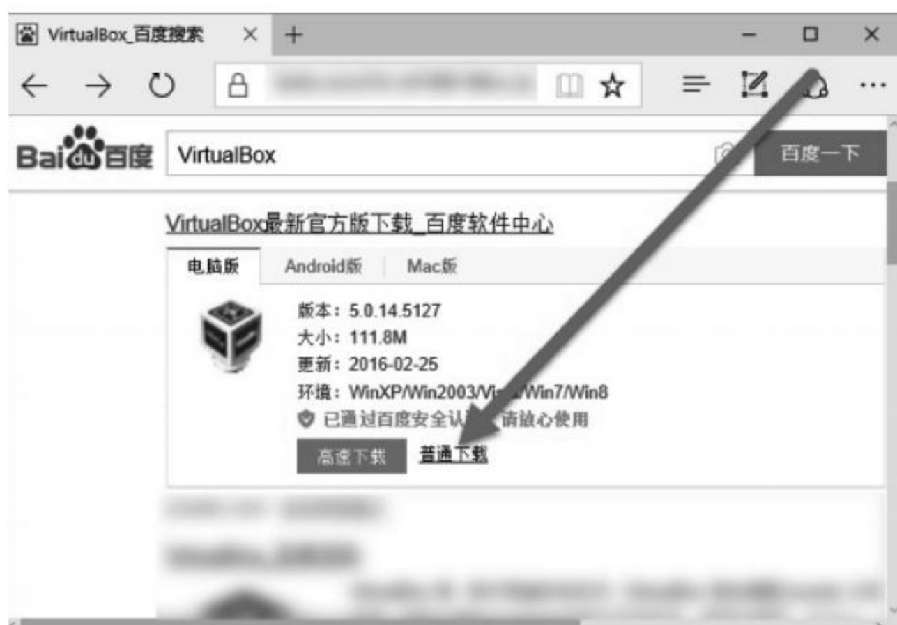
图 1-7 VirtualBox 的下载
