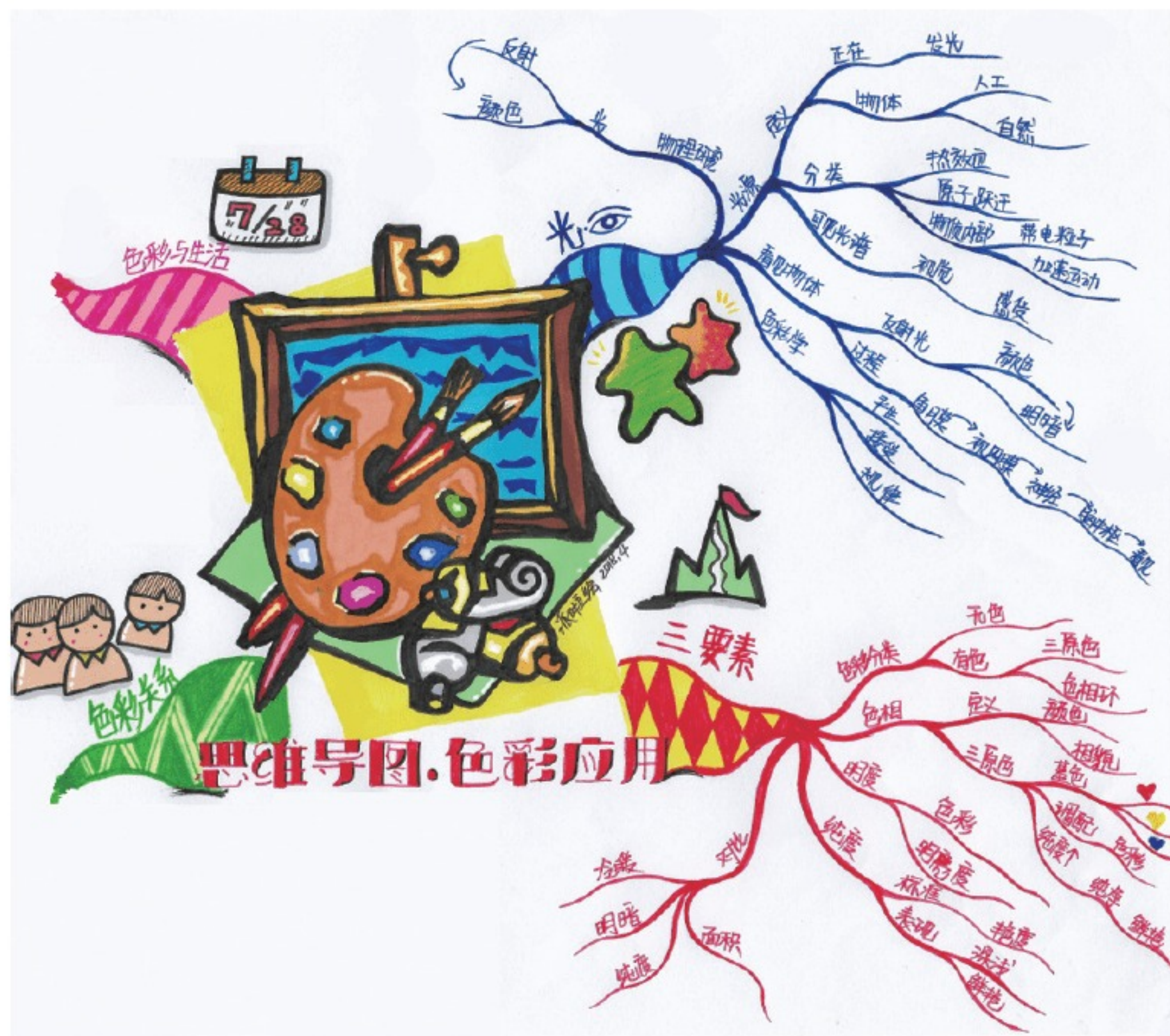
图 3-9 绘制分支图
