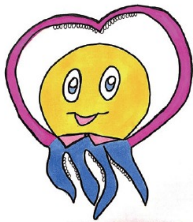
图 5-20 绘制中心图
