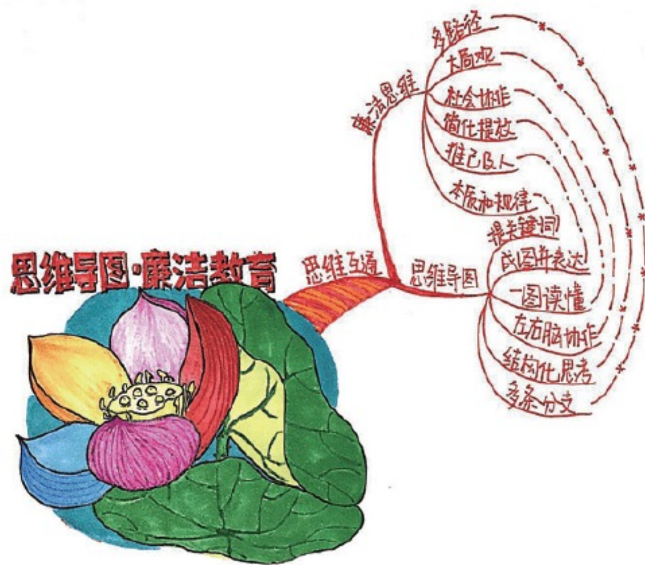
图 2-14 绘制连线
