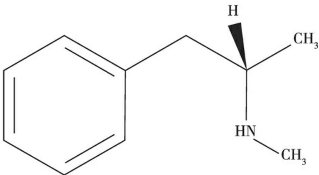
柏飞丁的化学分子式
