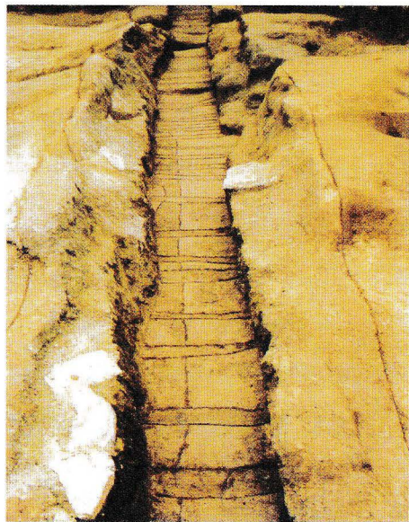
石砌输水管道
