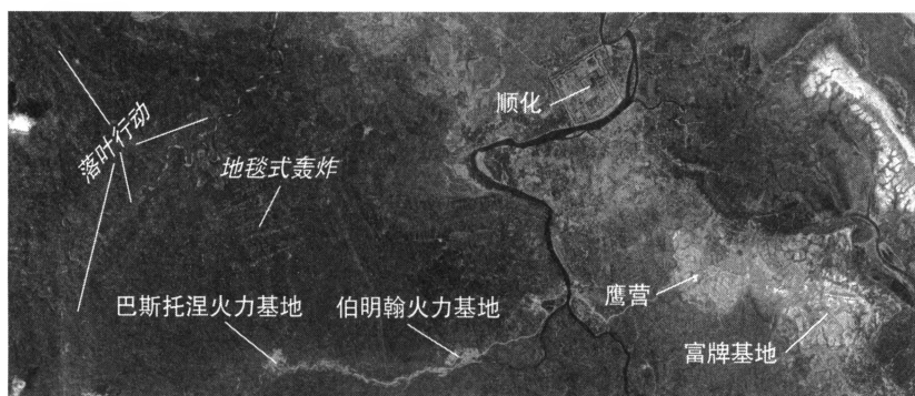
图 5.7 基地区域，1969 年 3 月 20 日。注释由笔者标注
