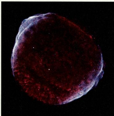
▲ 钱德拉 X 射线望远镜拍摄的 SN 1006 图像
