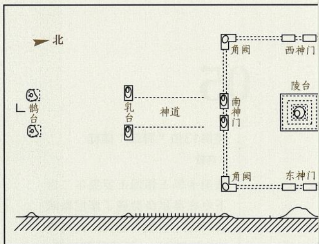
▲ 永定陵上宫平面复原图
