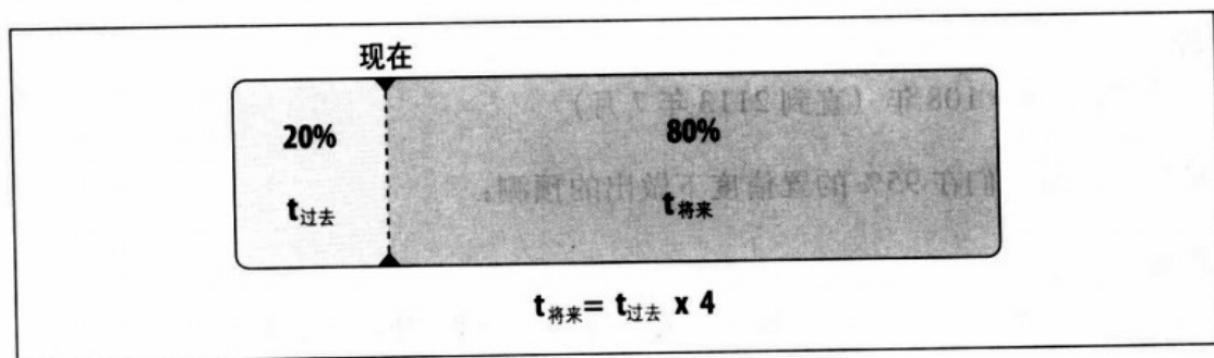
图 5-4: 剩余寿命的最大值 (60% 自信度)
