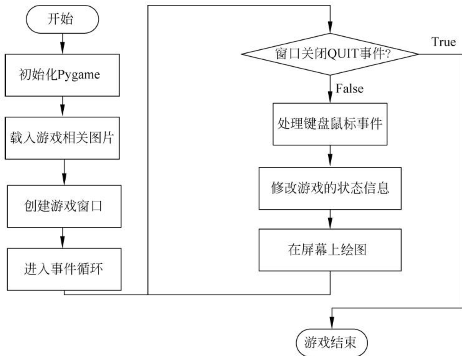
图 12-1 Pygame 开发游戏的主要流程
