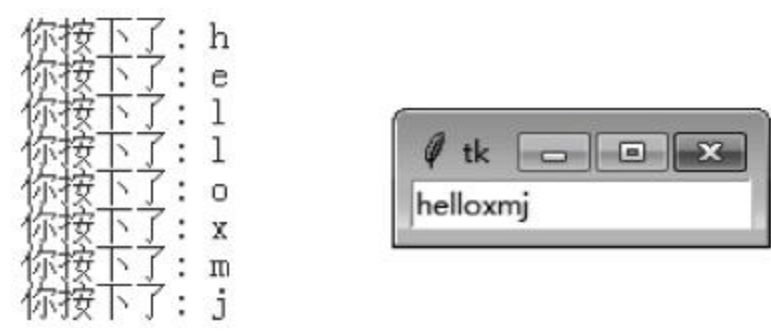
图 7-37 keyPress 键盘事件运行效果
