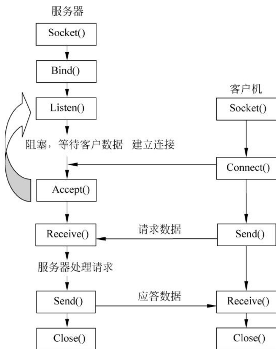
图 9-2 面向连接支持数据流 TCP 的时序图
