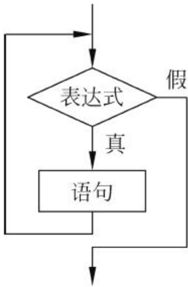
图 3-4 while 语句的流程图
