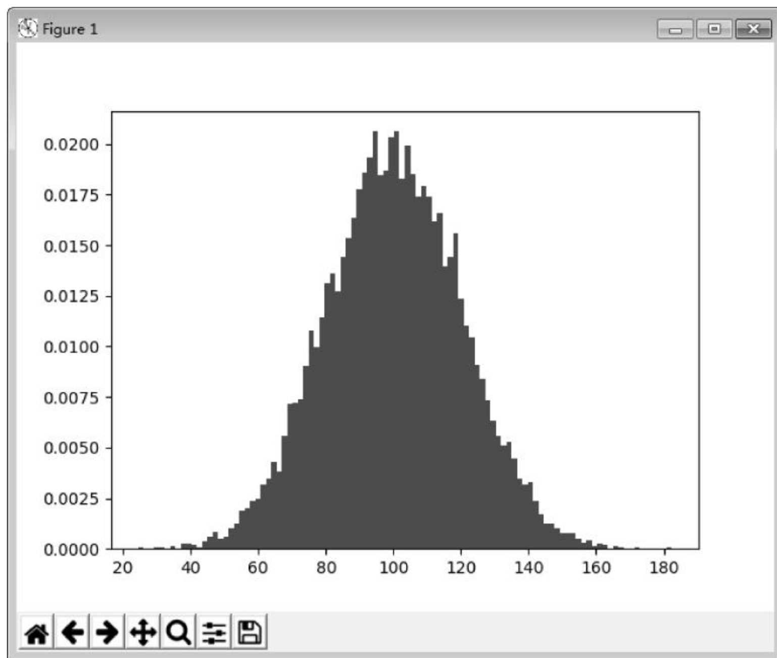
图 14-5 直方图实例
