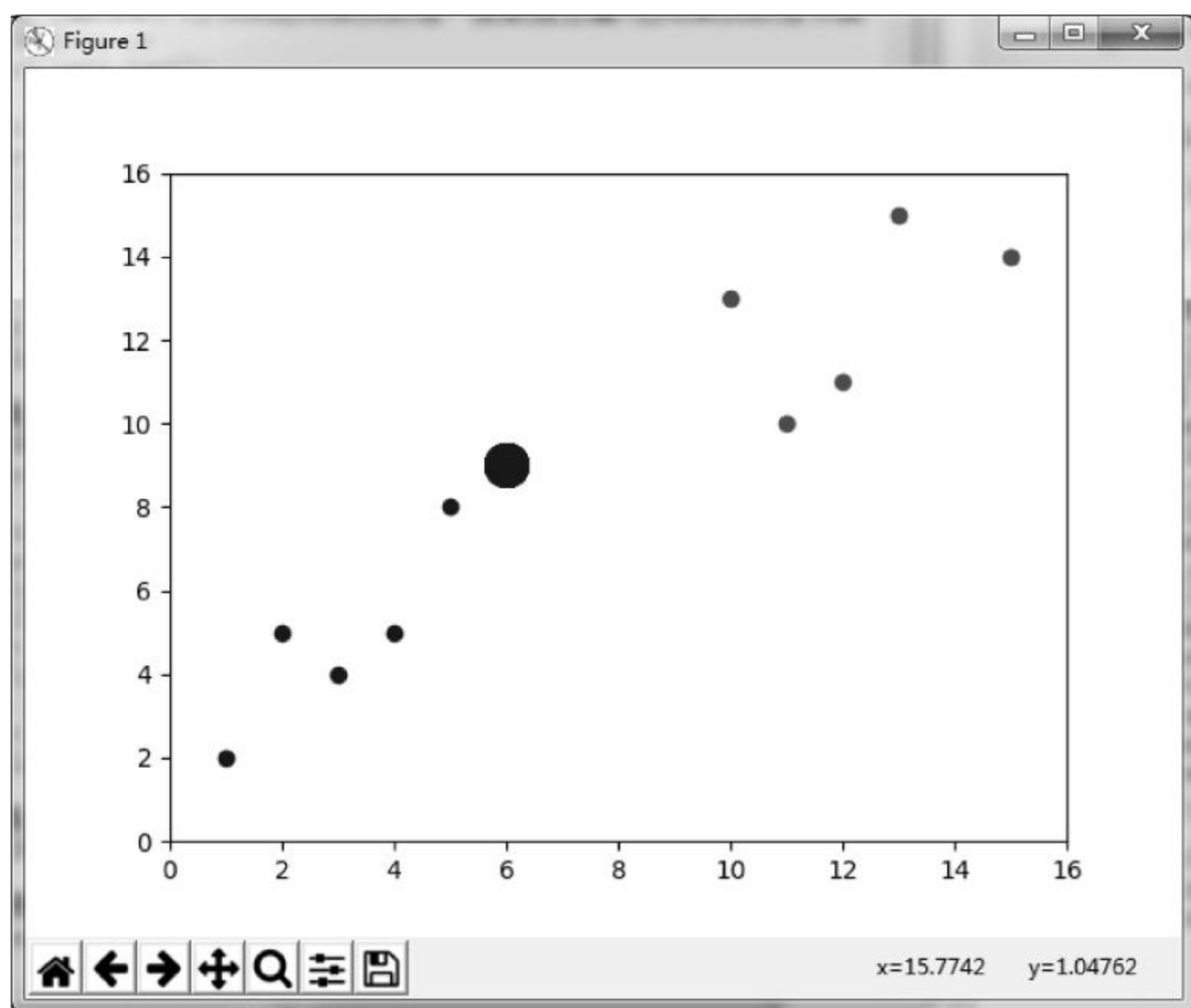
图 16-3 分类结果
