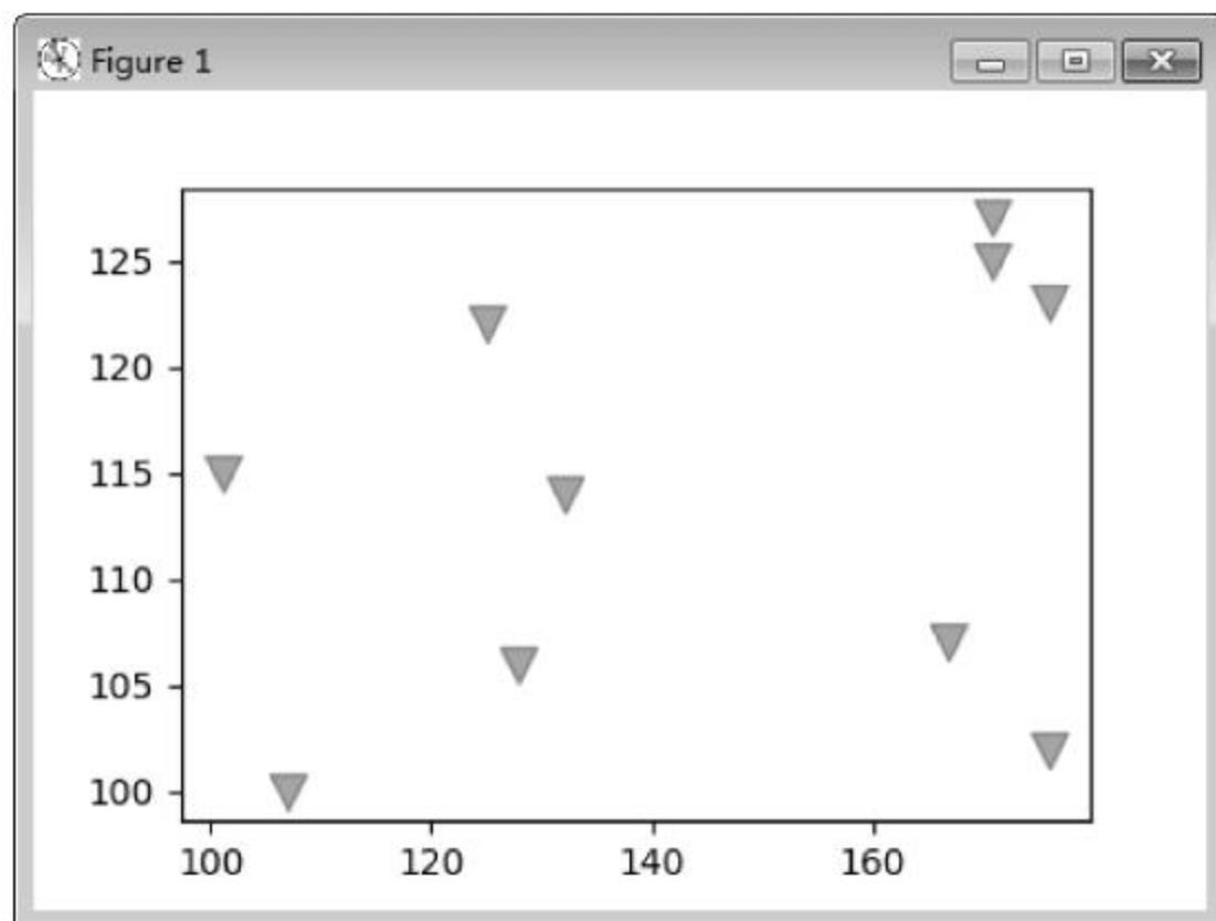
图 14-8 散点图实例
