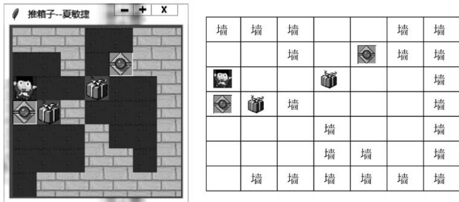
图 5-4 推箱子游戏
