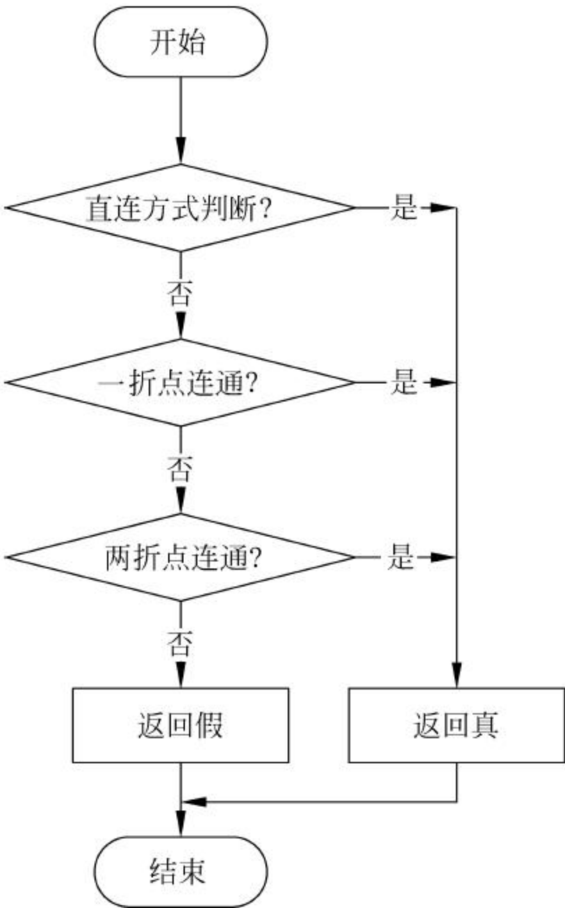
图 10-4 流程图
