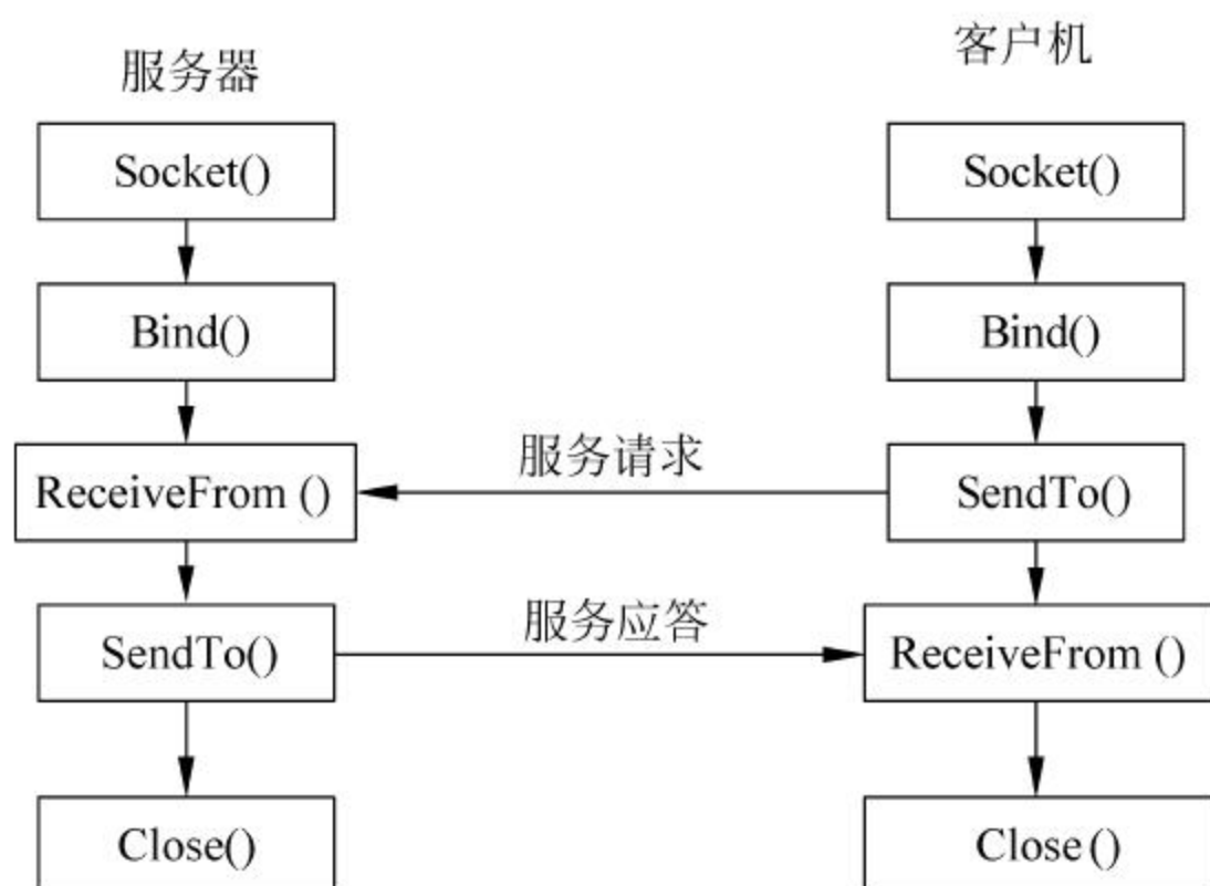
图 9-3 无连接数据报 UDP 的时序图
