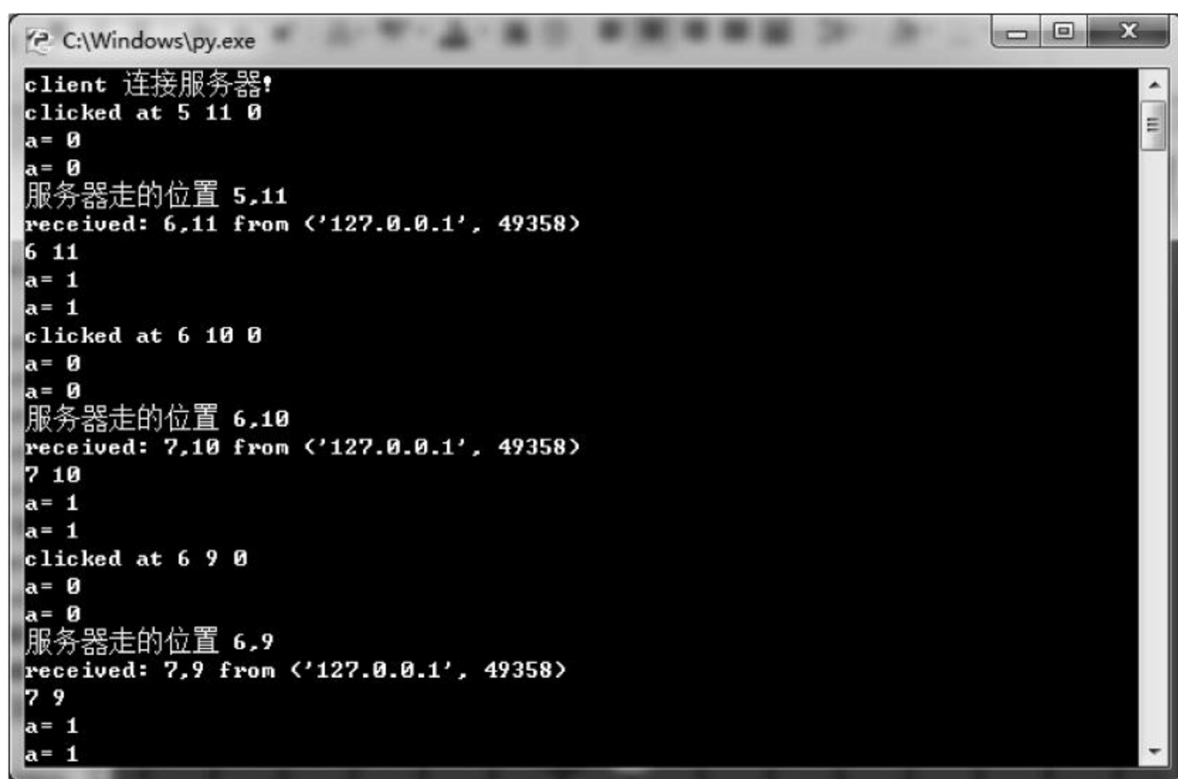
图 9-10 走棋过程打印的输出信息
