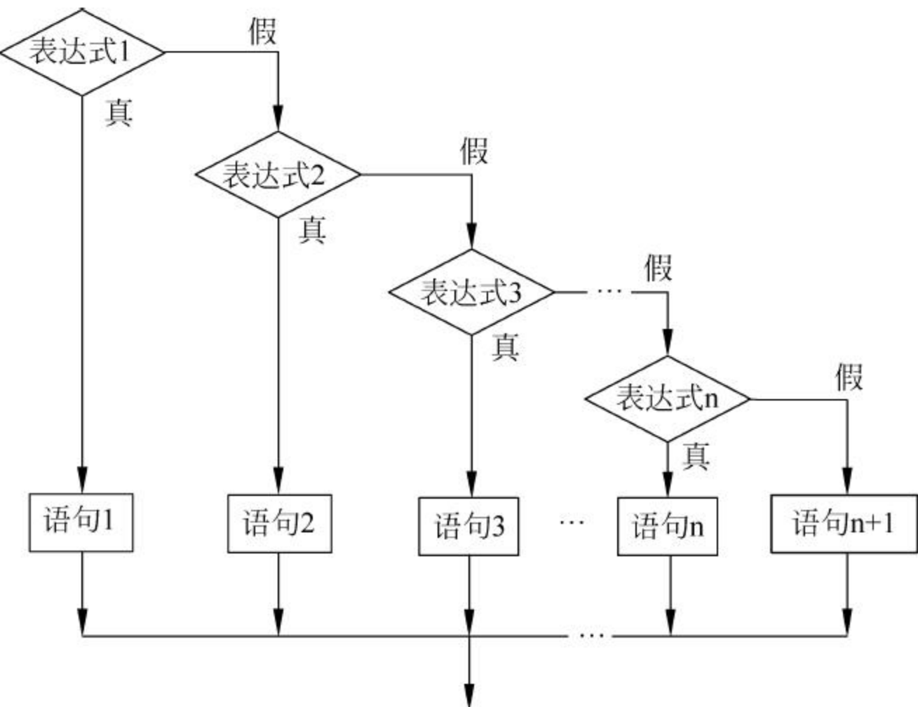
图 3-3 if...elif...else 语句的流程图
