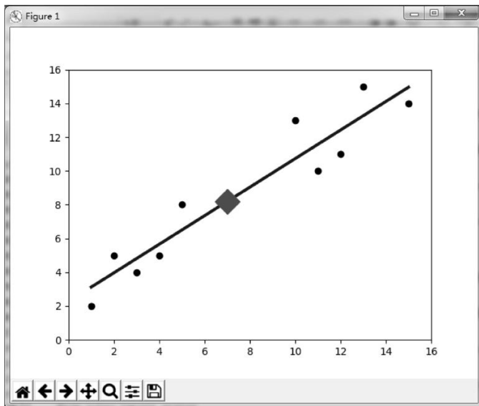
图 16-4 预测点采用菱形标出
