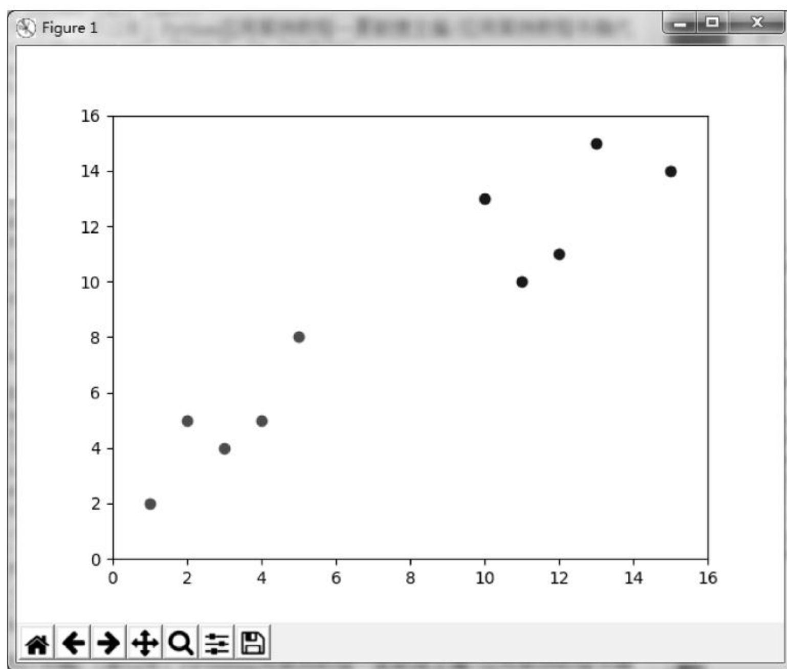
图 16-2 聚类结果
