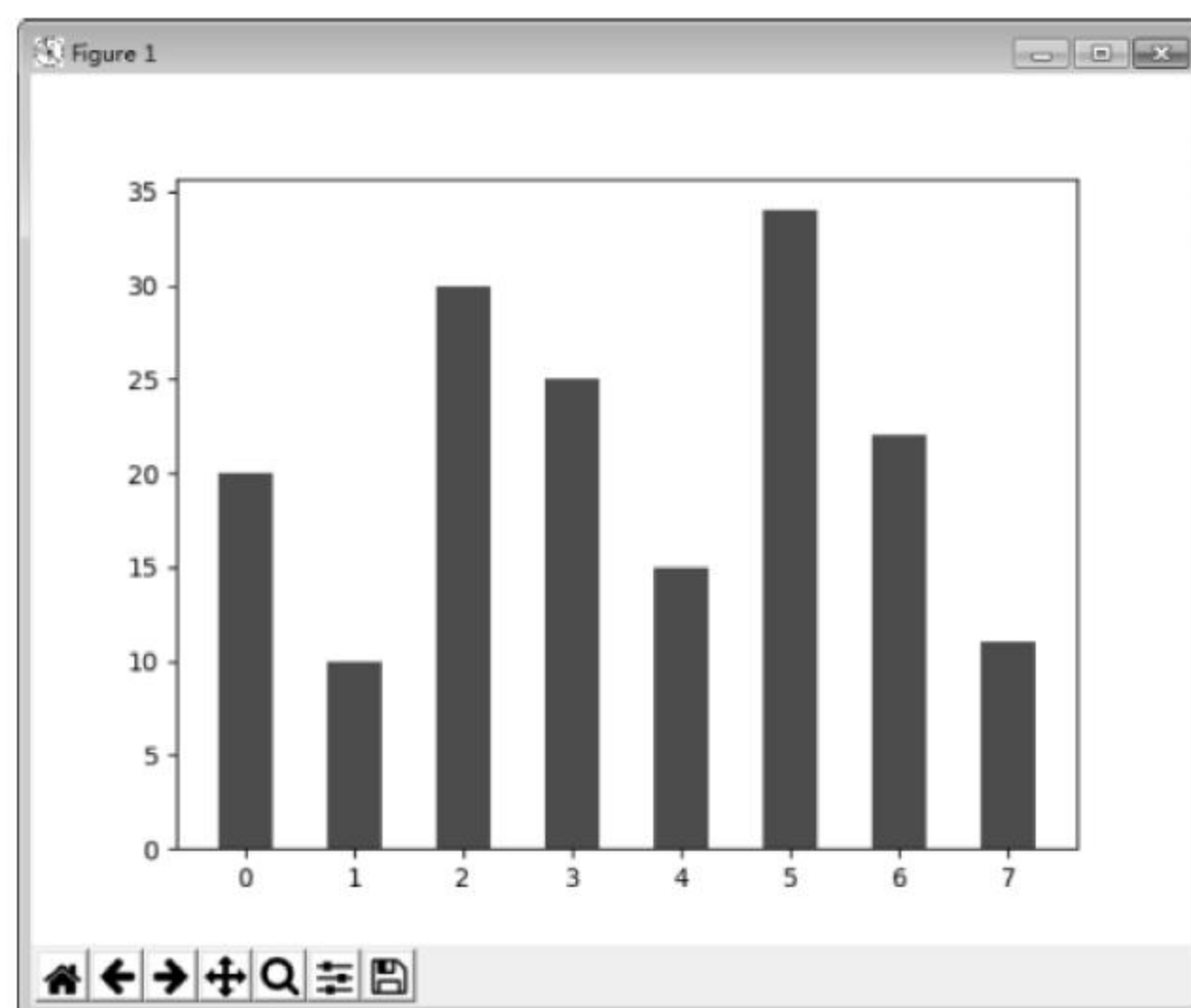
图 14-6 条形图实例
