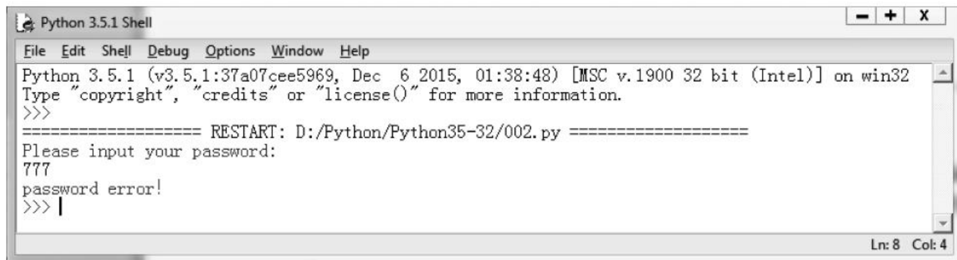
图 1-5 运行界面
