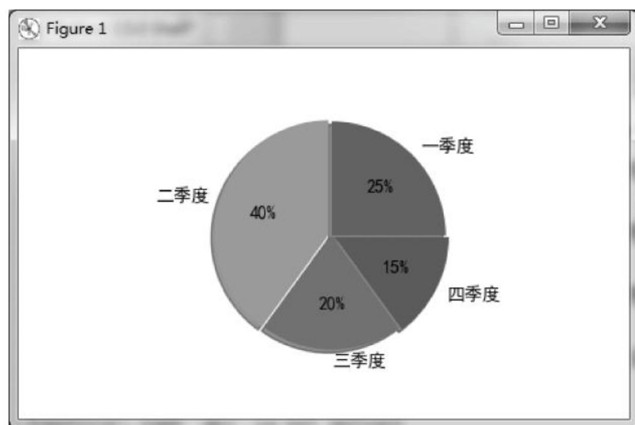
图 14-9 饼状图实例
