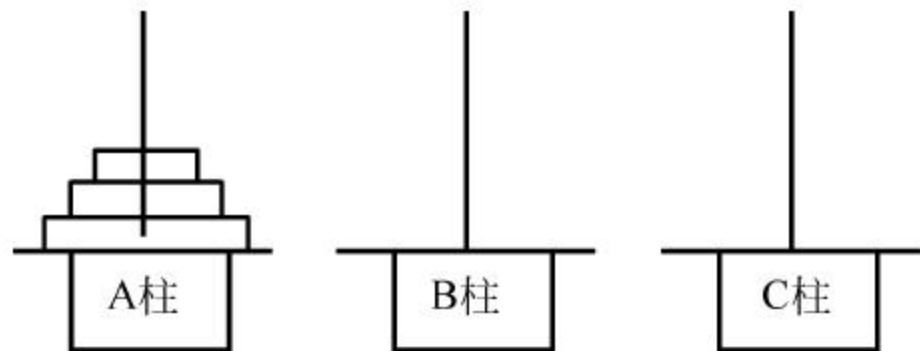
图 4-5 汉诺塔
