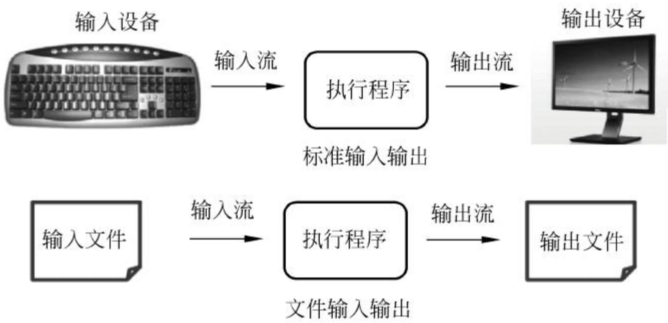
图 5-2 输入输出流
