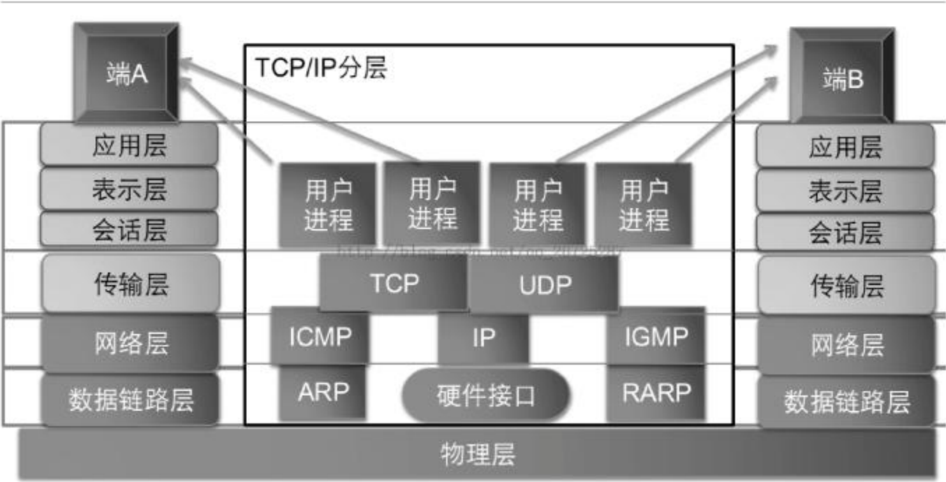
图 9-1 互联网协议
