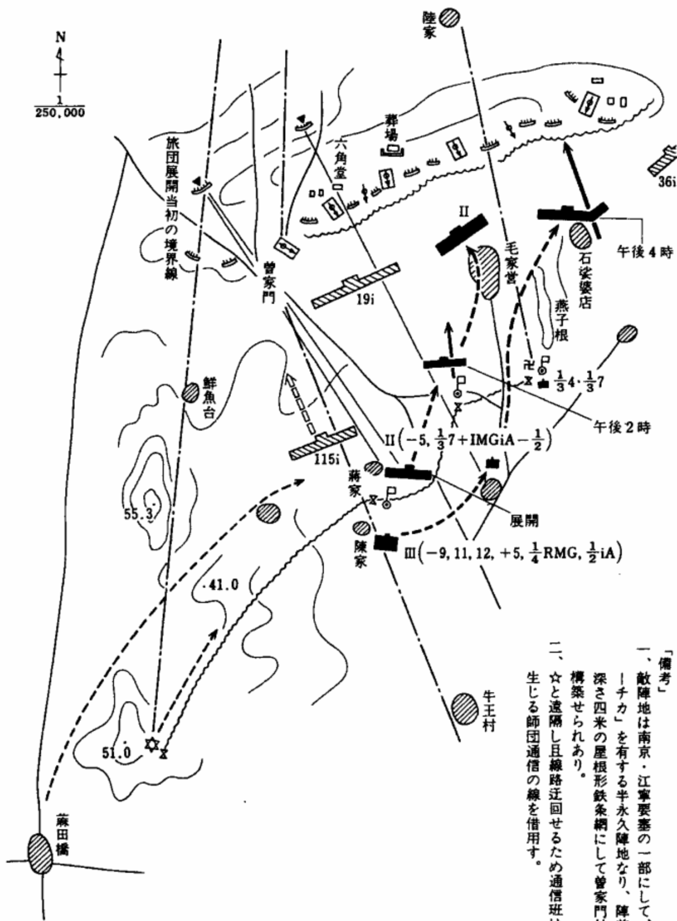
曾家門東方高地攻撃戦經過要図 (昭和12年12月10日10.00—同日18.00)
