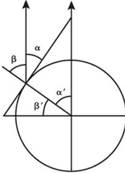
插图8 利用北极星的地平高度测定纬度
