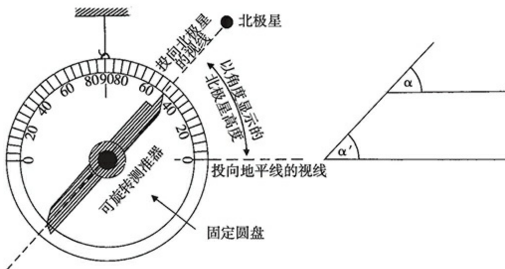
插图11 用等高仪测北极星
