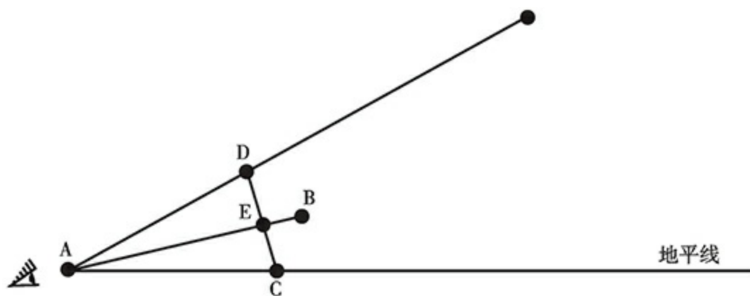
插图12 用十字测天仪（Jakobsstab，或称“十字杆”“直角仪”等）测定太阳高度
