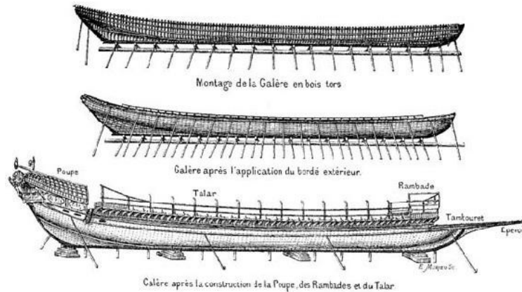
建造桨帆船的步骤
