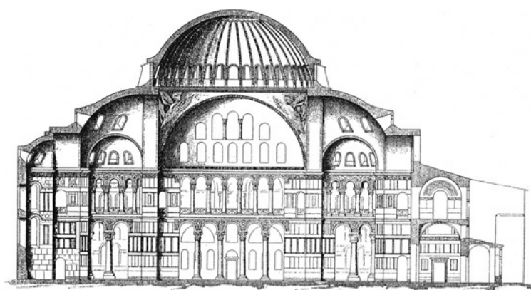
圣索菲亚大教堂截面图
