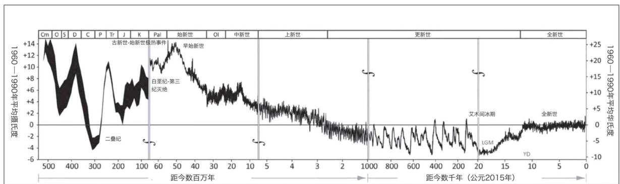
图6.1 气候变化史是基于冰芯等相关材料推断的气候数据重建的。纵观地球的历史，气候不断发生变化。然而，当今气候变化有三个独特之处。第一是变化速度。现在地球变暖的速度远超数百万年前的任何一个时期。第二则是变暖幅度。上一次如此大幅度的气候升温现象发生在4000多万年前始新世，而据预测下一个世纪人类就会面临同样幅度的气候升温现象。第三如图中最右侧所示，自从农业产生以来，人类所经历的气候异
