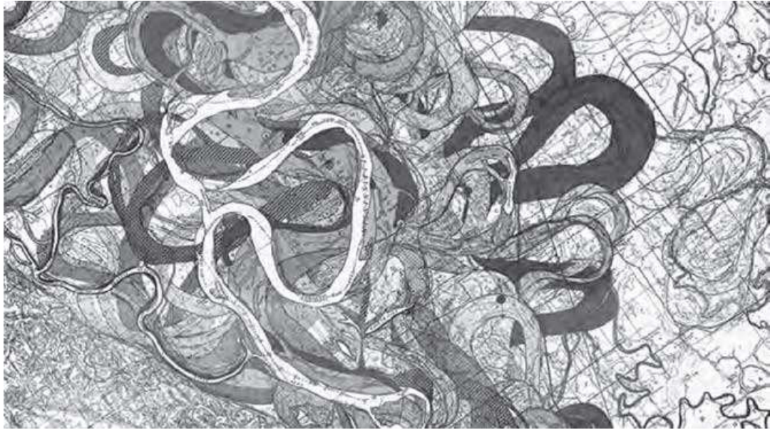
图10.2 密西西比河和它在被河堤冲刷和包围之前的流动轨迹。随着时间的推移，它一直在不停地运动和进化。该地图由来自美国陆军工程兵团的哈罗德·N.菲斯克于1944年制作出版，用于密西西比河下游冲积河谷的地质调查。
