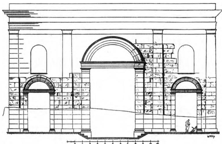
东门的东立面
