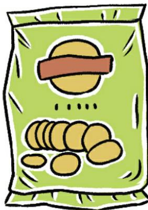
氮气填充
