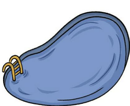
余氯 ( \text{Cl}_2 ) 指示剂 (游泳池)
