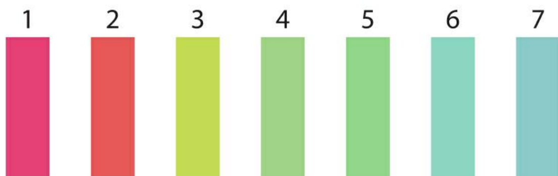
pH 比色卡
