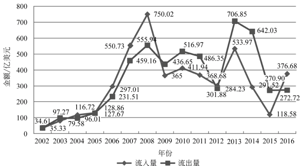
图 11-11 俄罗斯对外直接投资流量对比(2002—2016)
