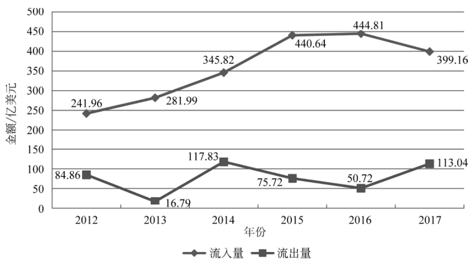
图 11-12 印度对外直接投资流量对比(2011—2017)
