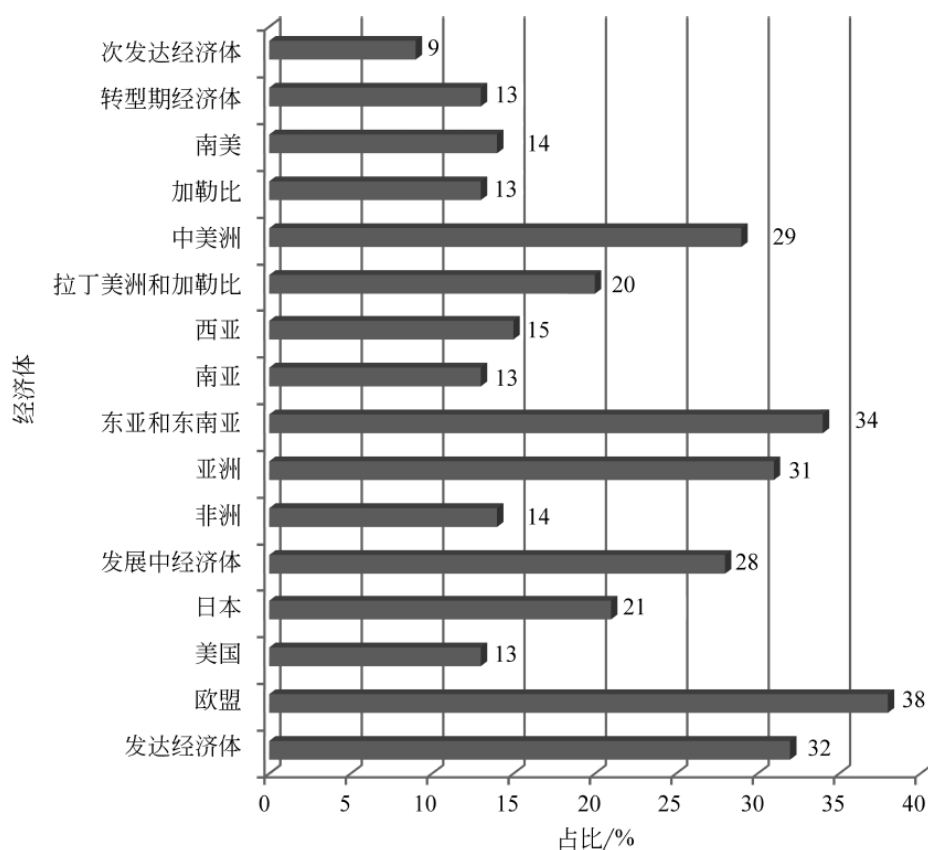
图 10-9 2017 年 FVA 在各经济体出口中的份额
