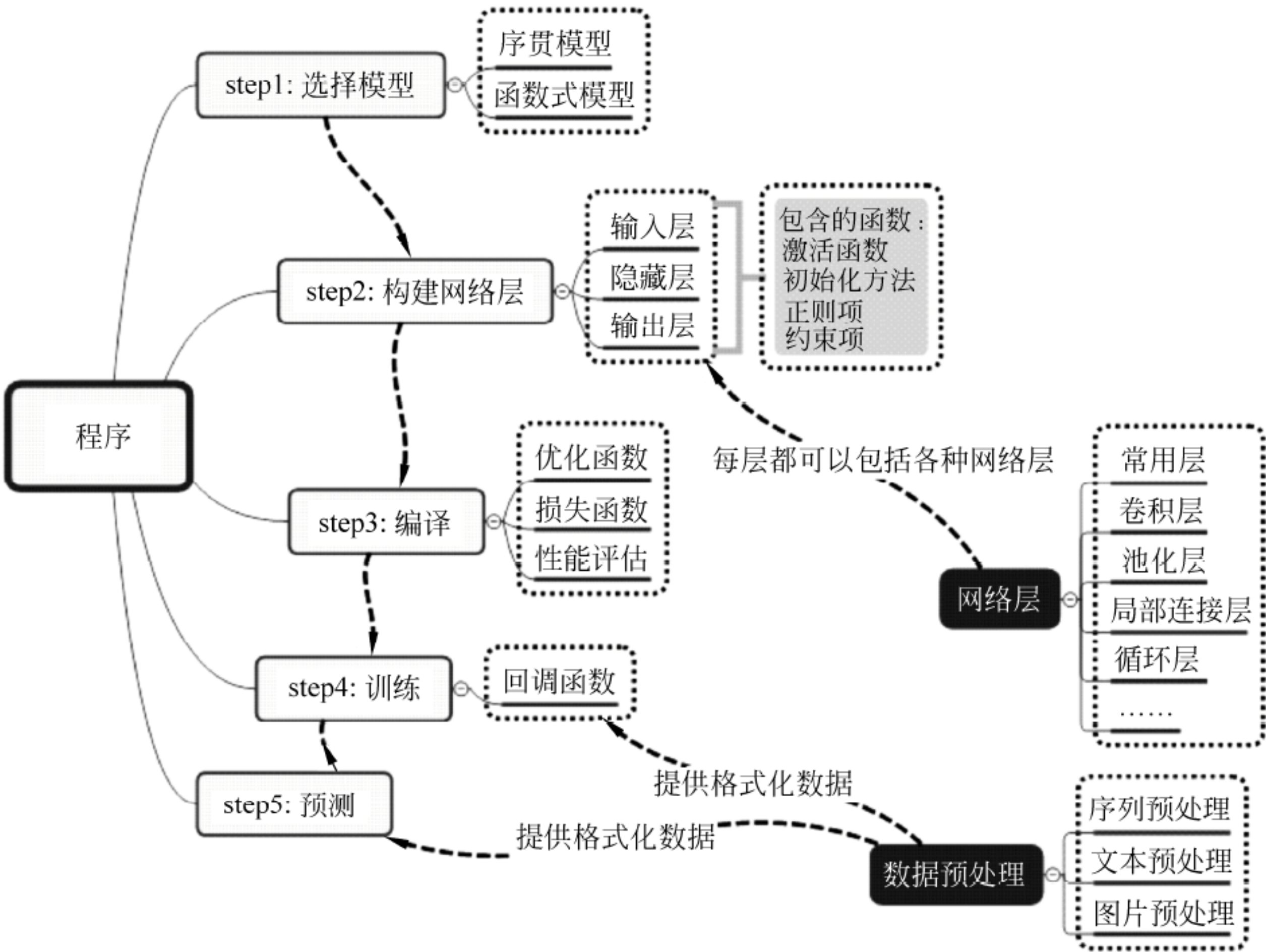
图 19-12 用 Keras 搭建神经网络
