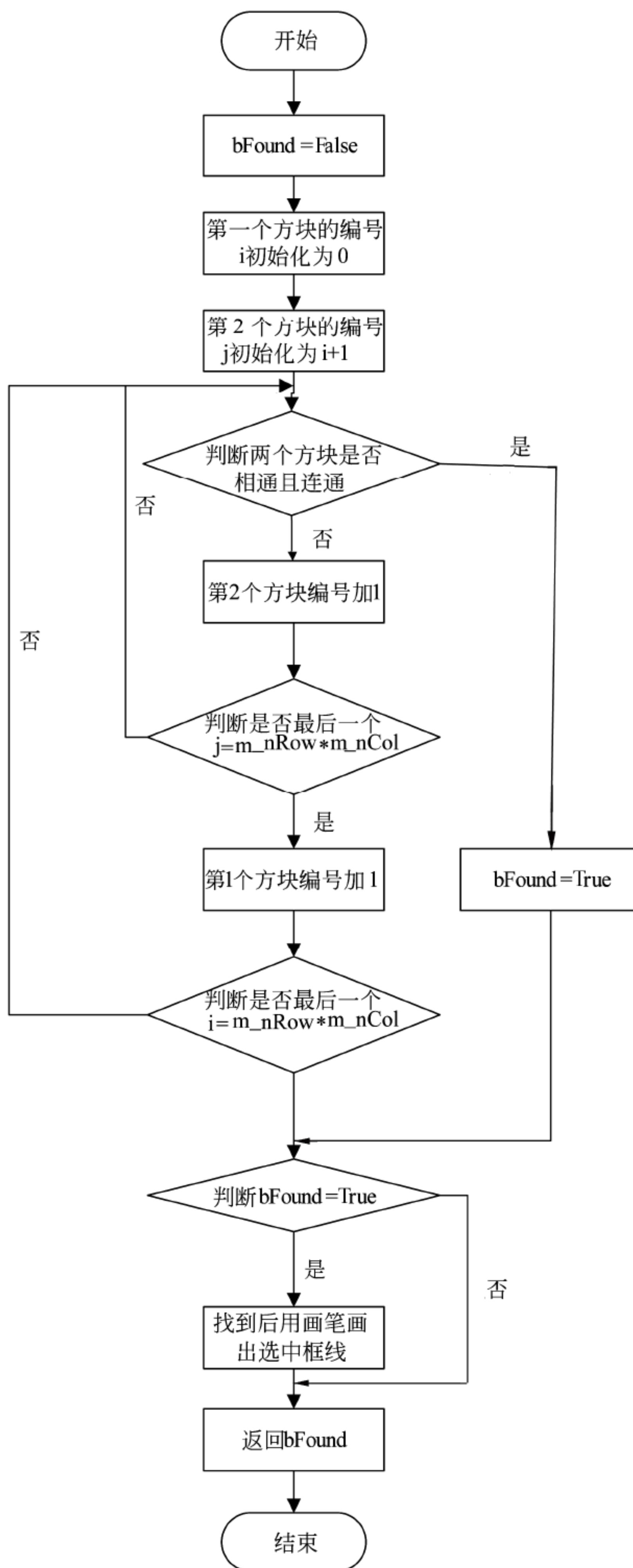
图 10-8 智能查找匹配方块的流程图
