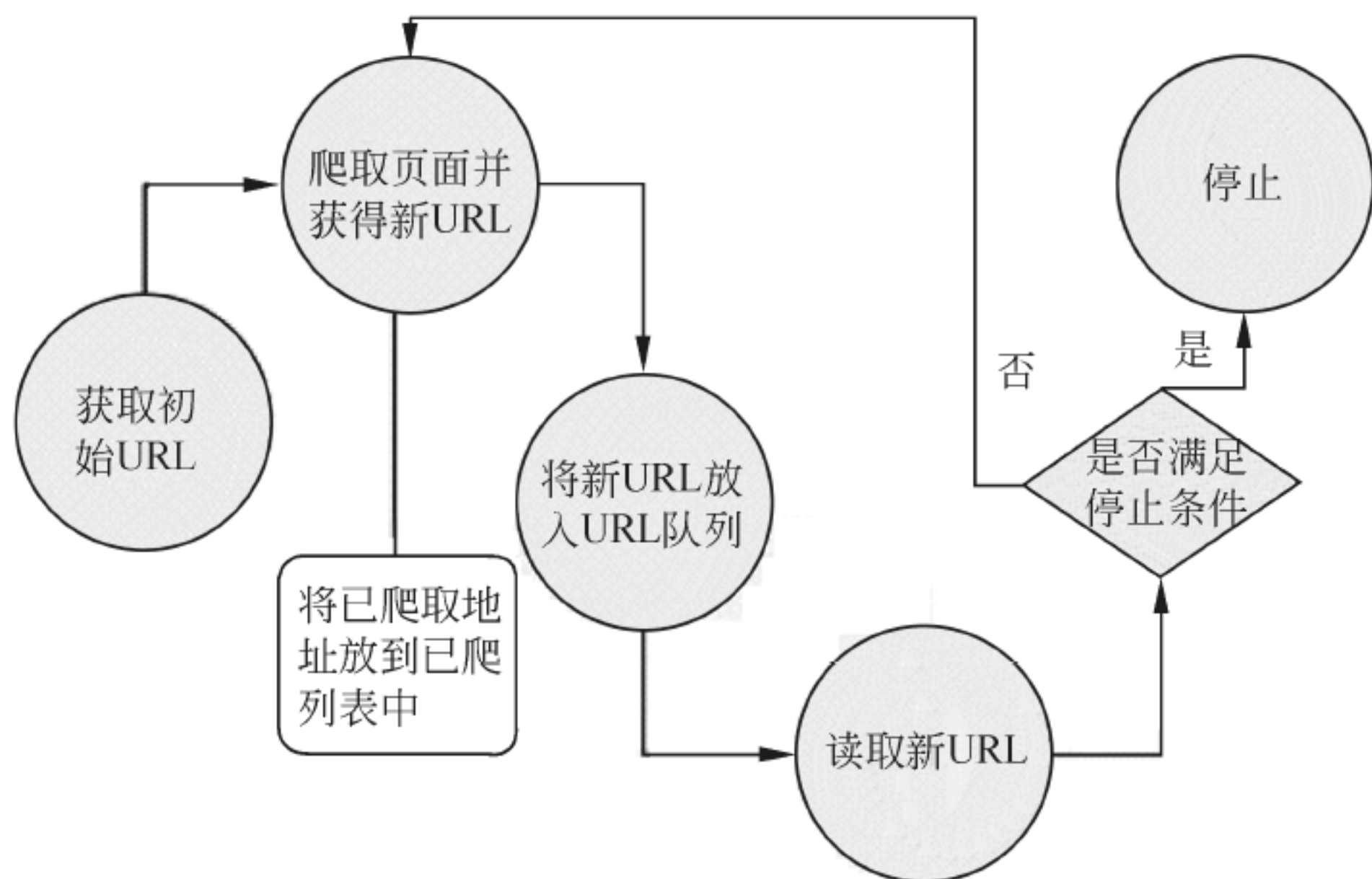
图 5-4 网络爬虫的实现原理及过程
