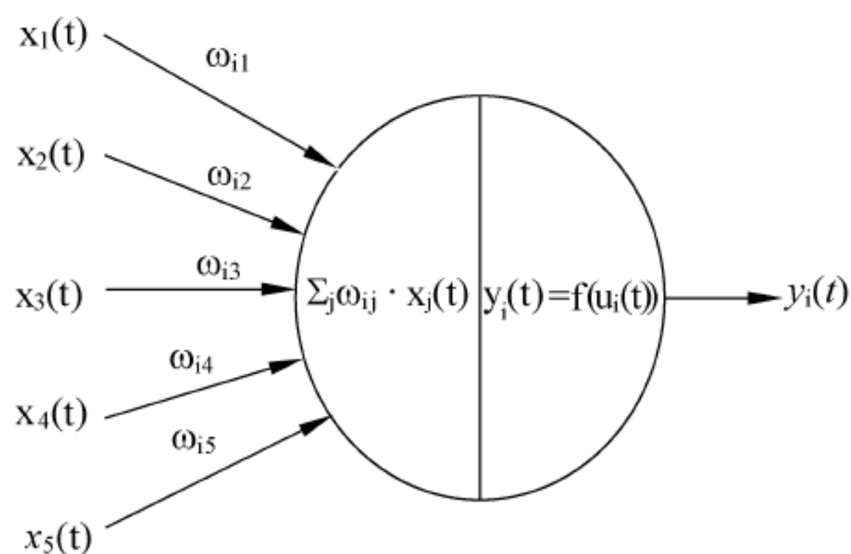
图 19-3 人工神经网络
