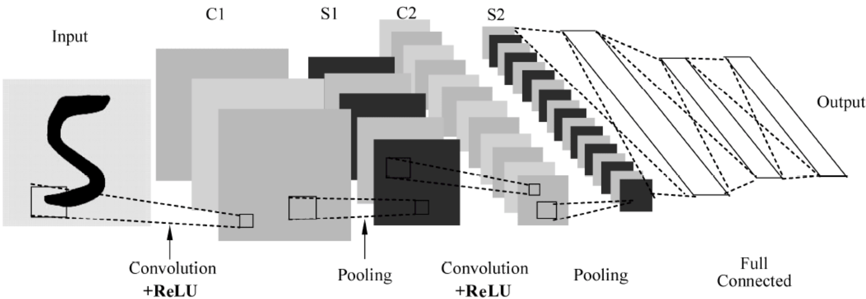
图 19-11 一个典型的 CNN 网络结构
