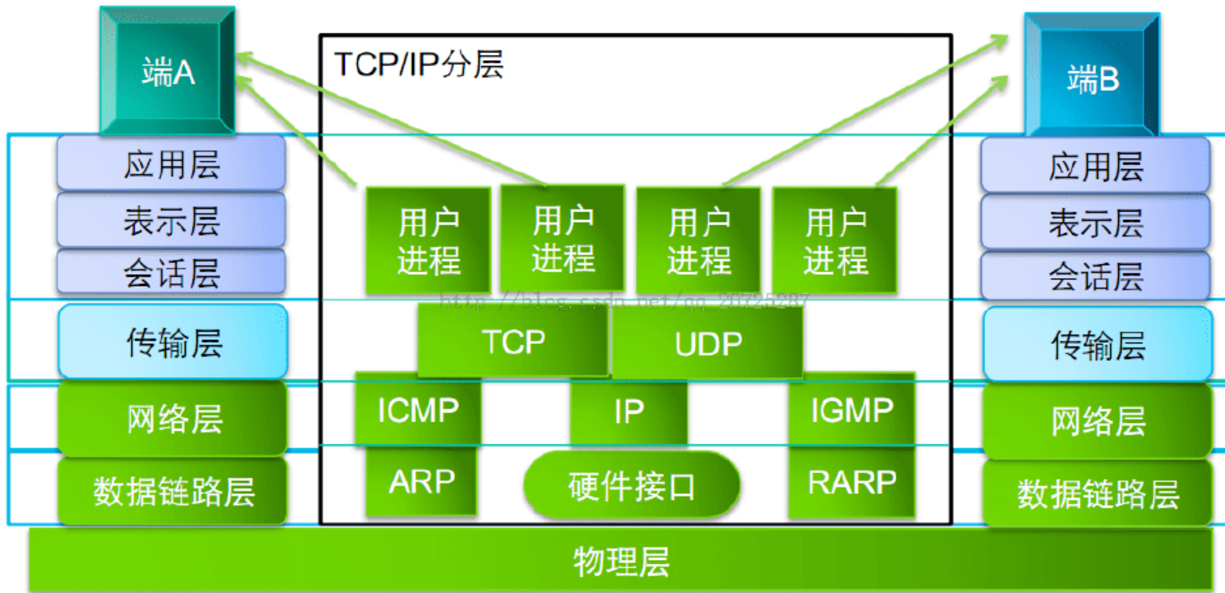
图 13-2 互联网协议
