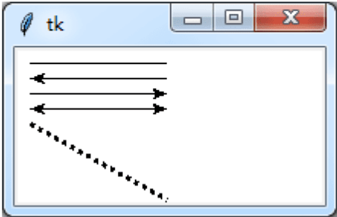
图 10-10 创建线条
