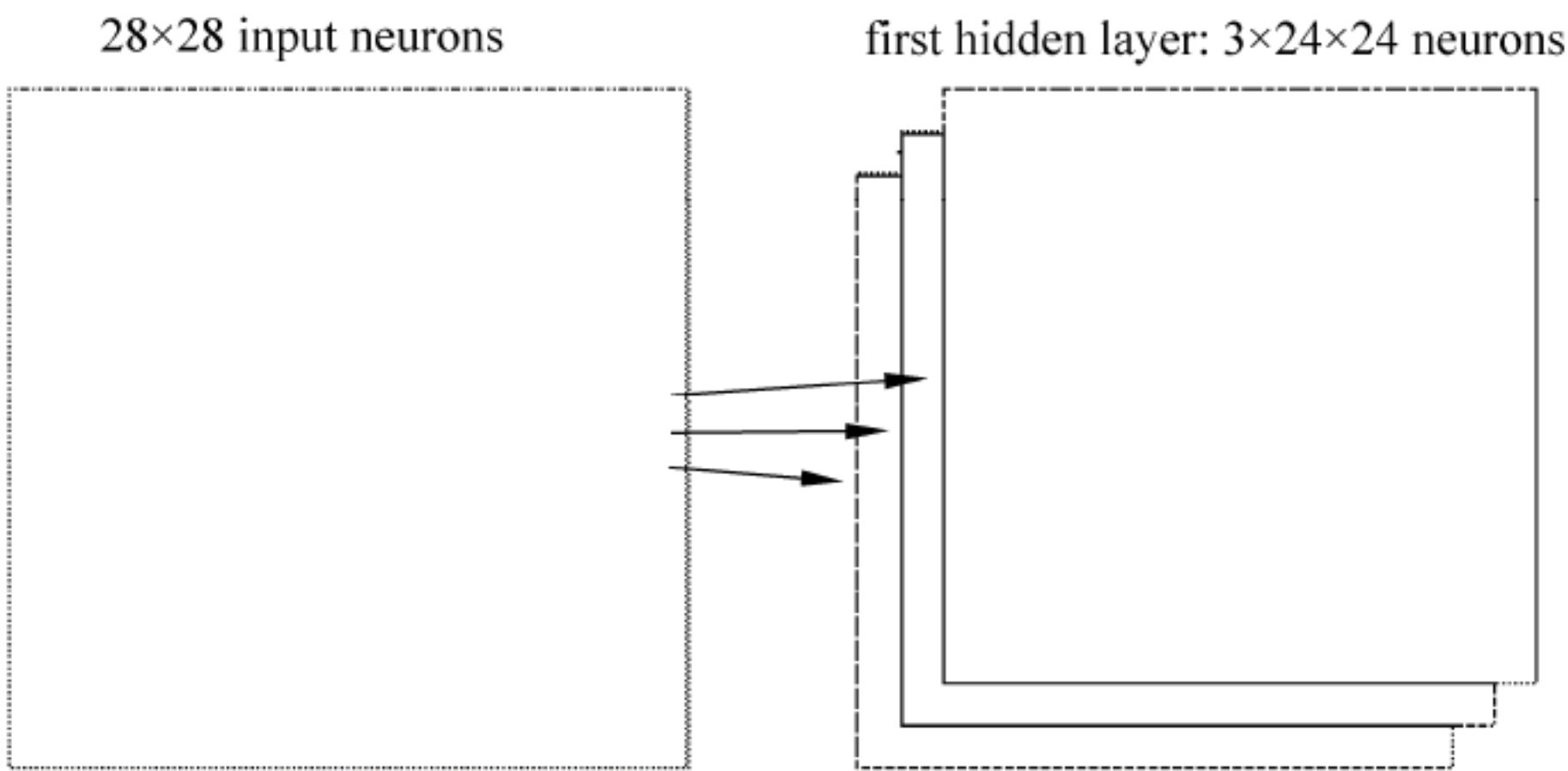
图 19-7 多个卷积核
