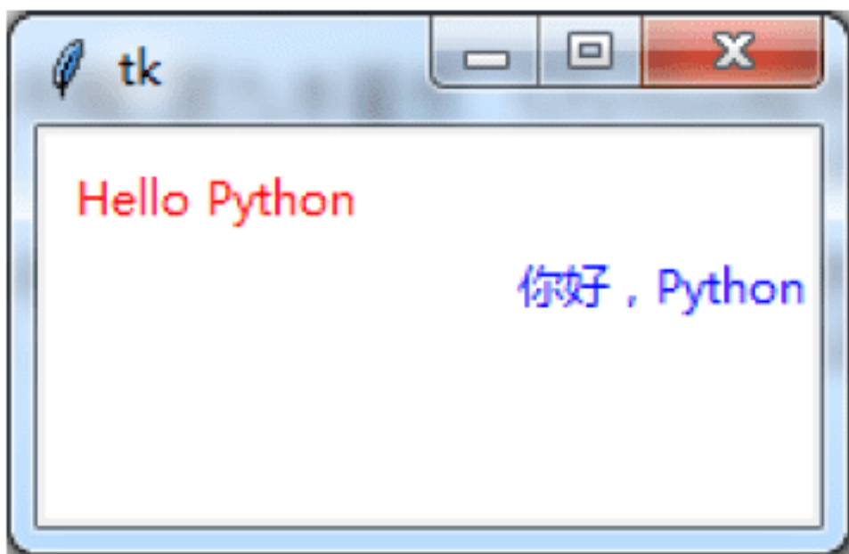
图 10-14 创建文本
