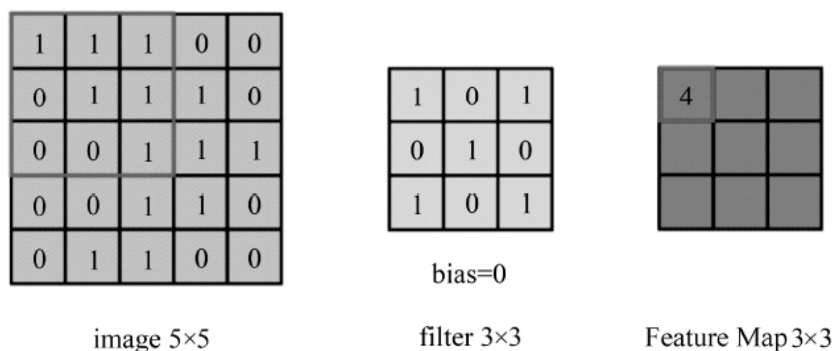
图 19-5 卷积原理图 1
