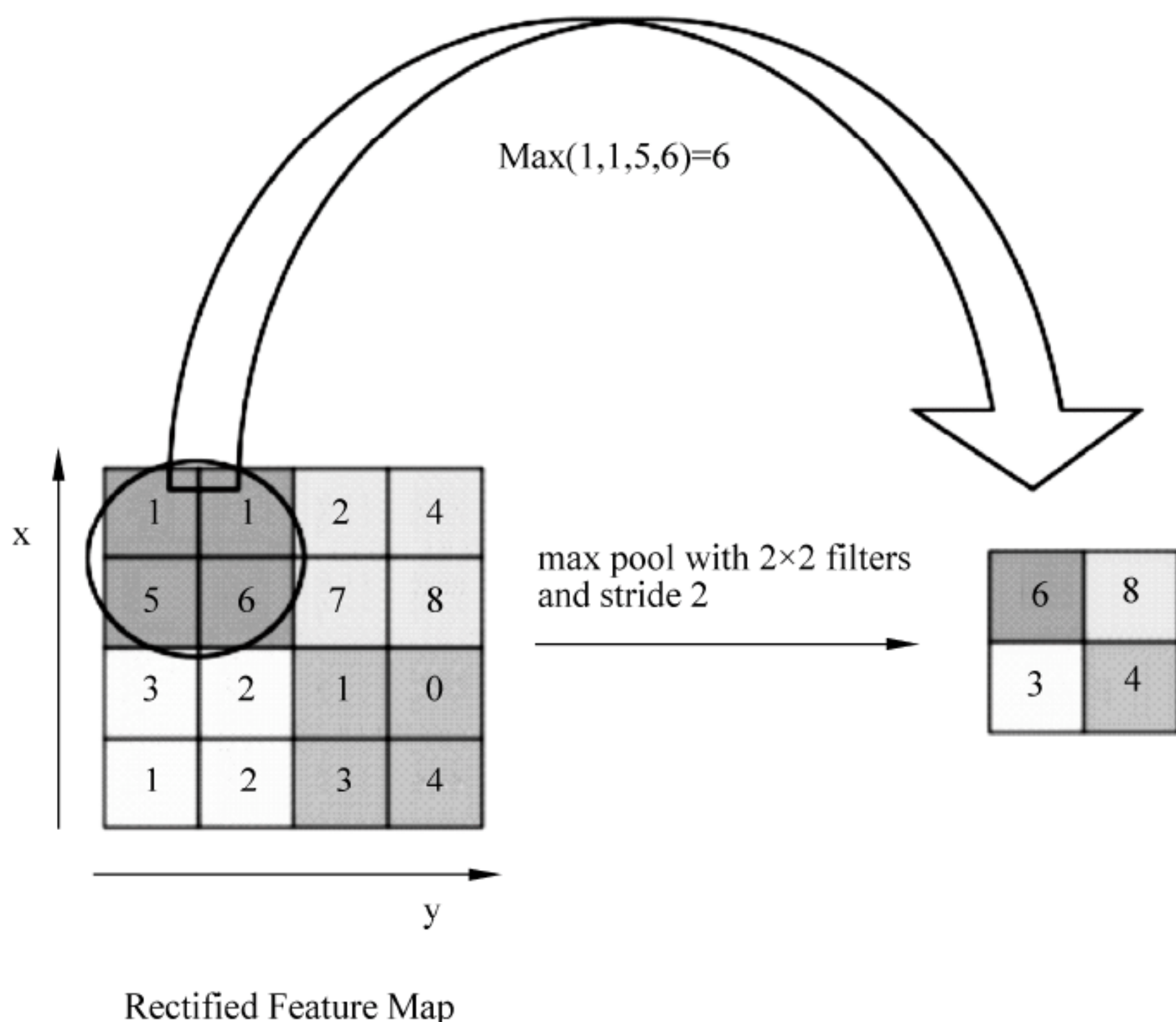
图 19-8 池化
