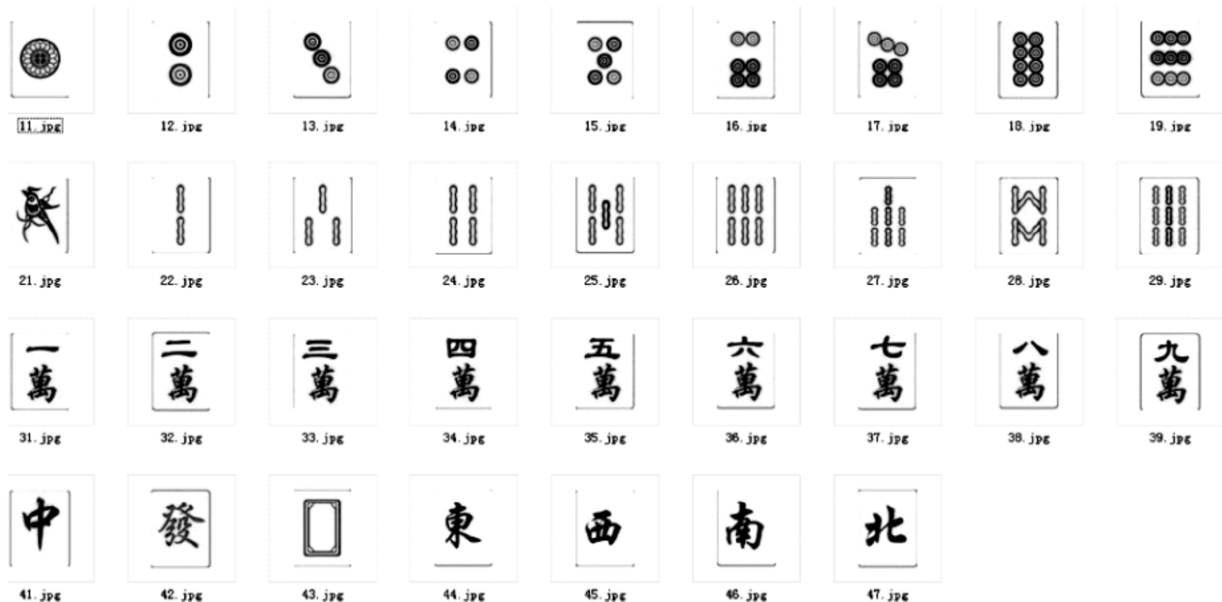
图 12-2 素材图片
