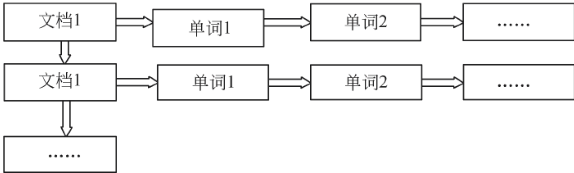
图 5-2 正排表结构示意图
