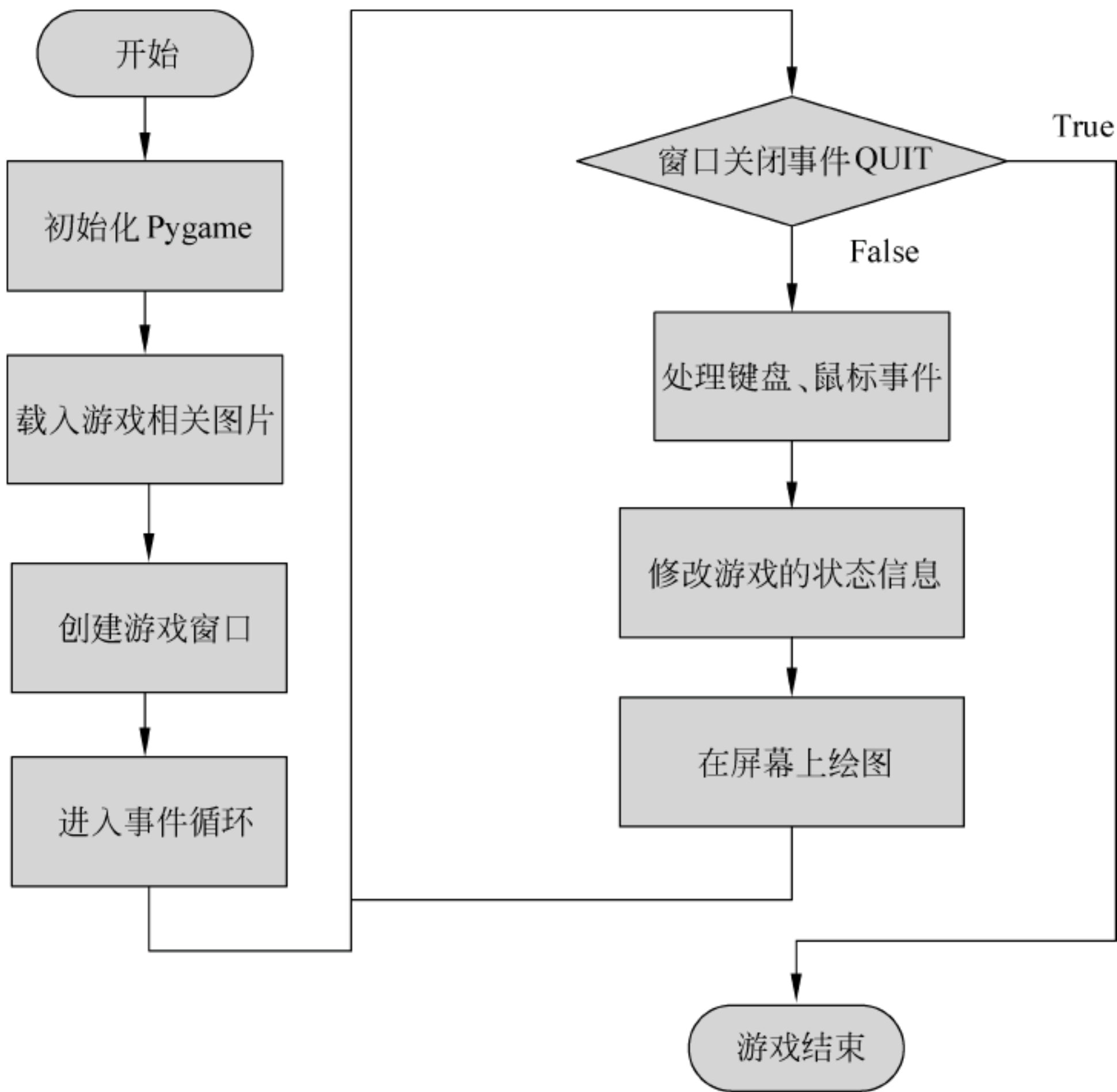
图 17-1 Pygame 开发游戏的主要流程
