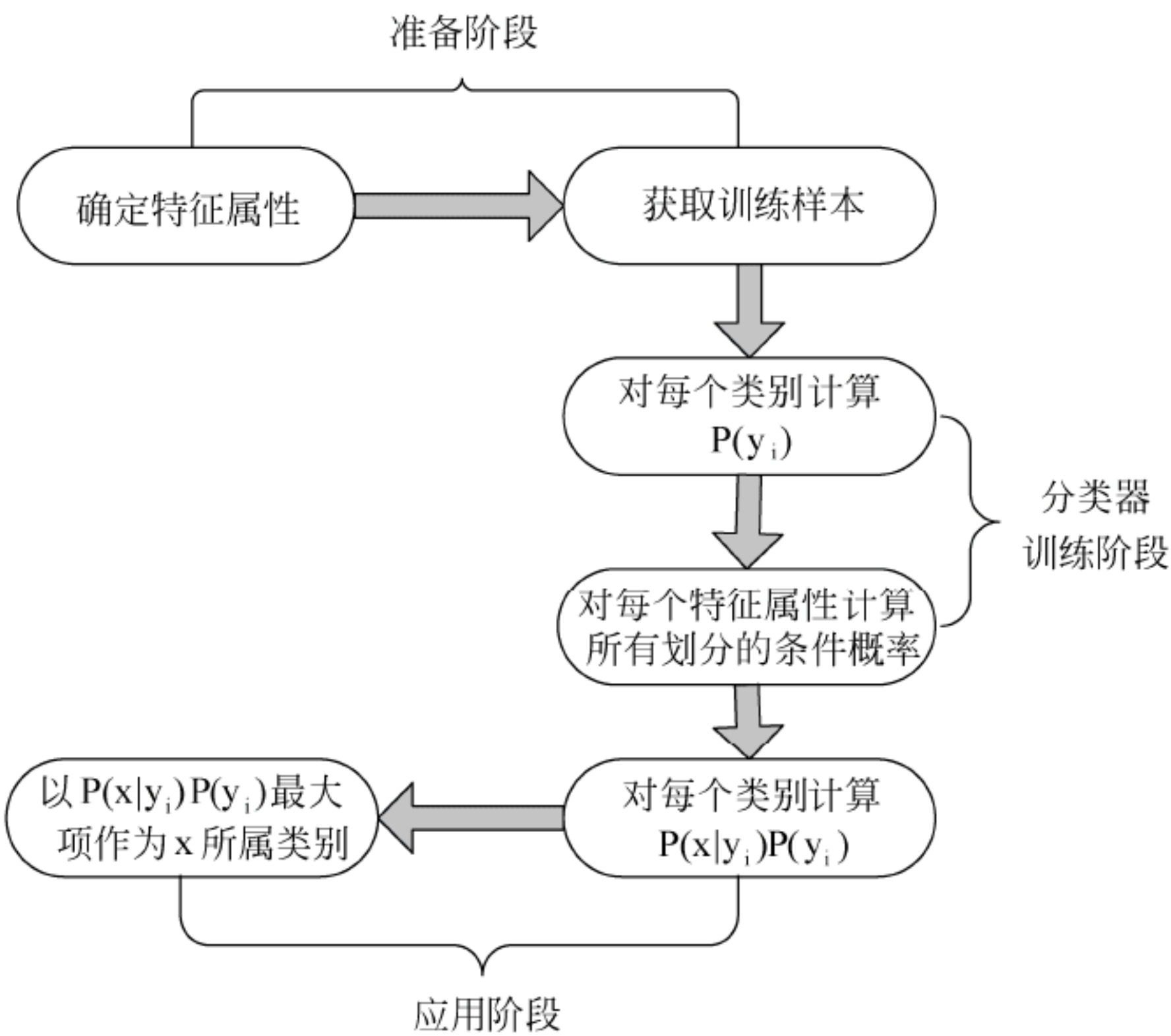
图 18-3 朴素贝叶斯分类流程
