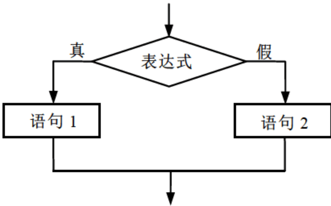
图 1-2 if...else 语句的流程图
