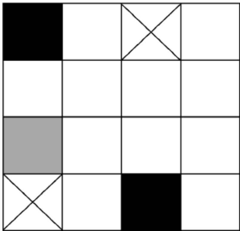
图 10-5 一个折点连通示意图
