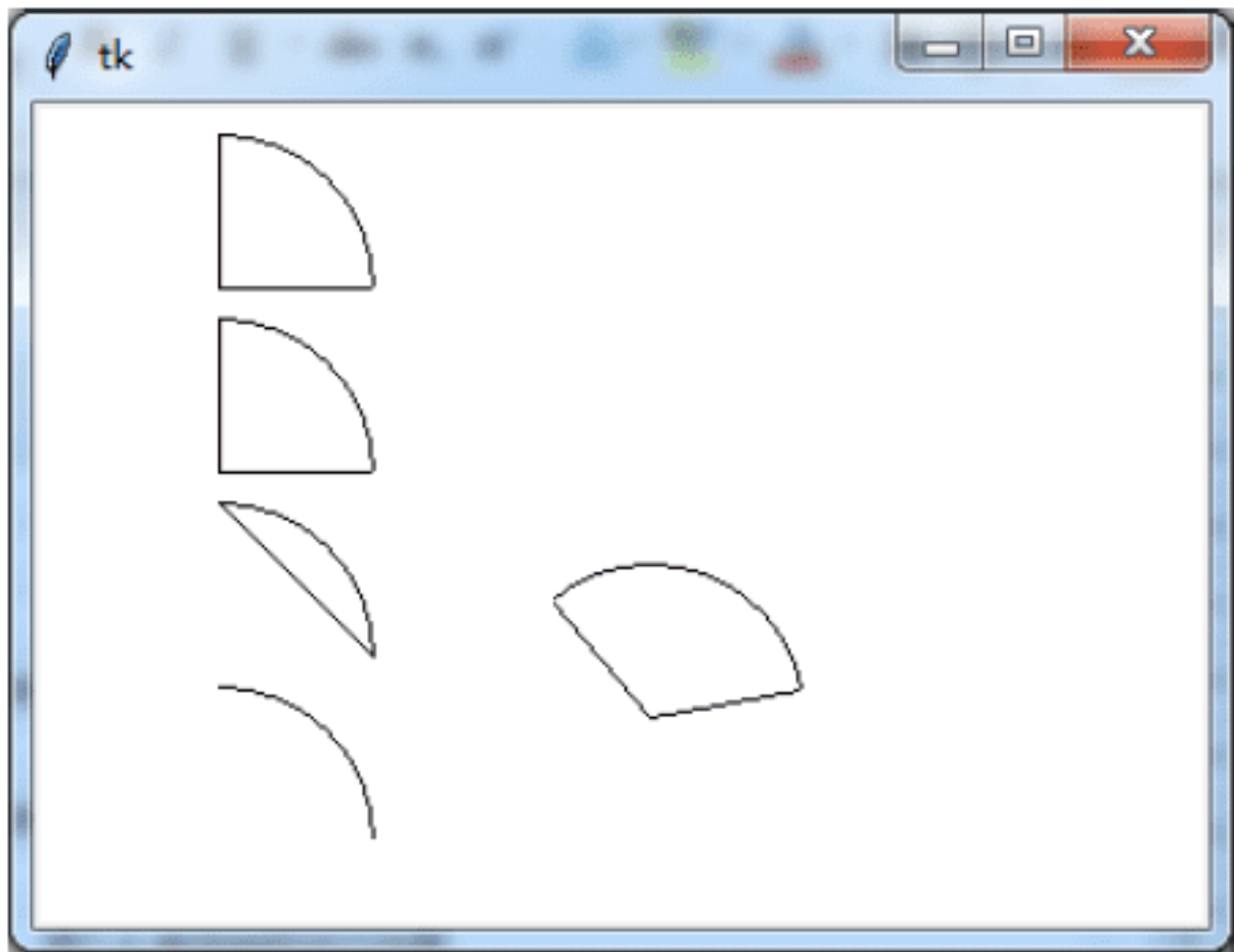
图 10-9 创建圆弧
