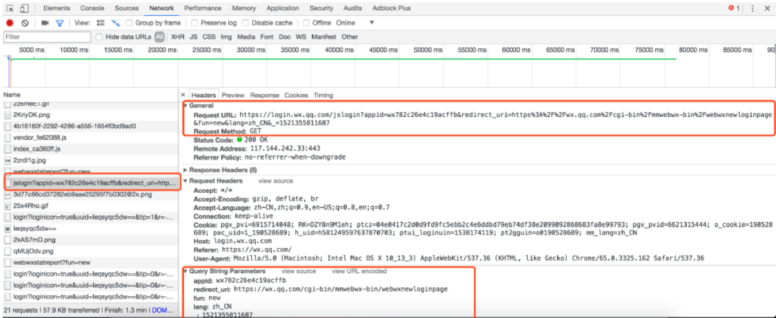
图 8-3 分析 URL
