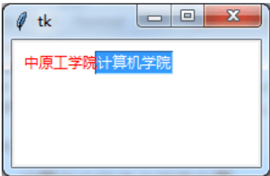
图 10-15 选中文本
