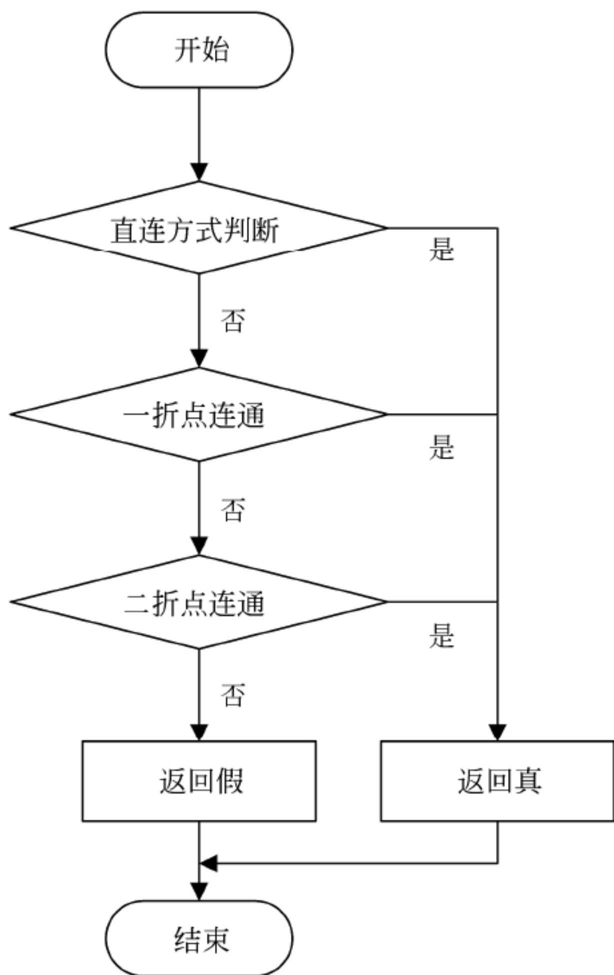
图 10-4 流程图
