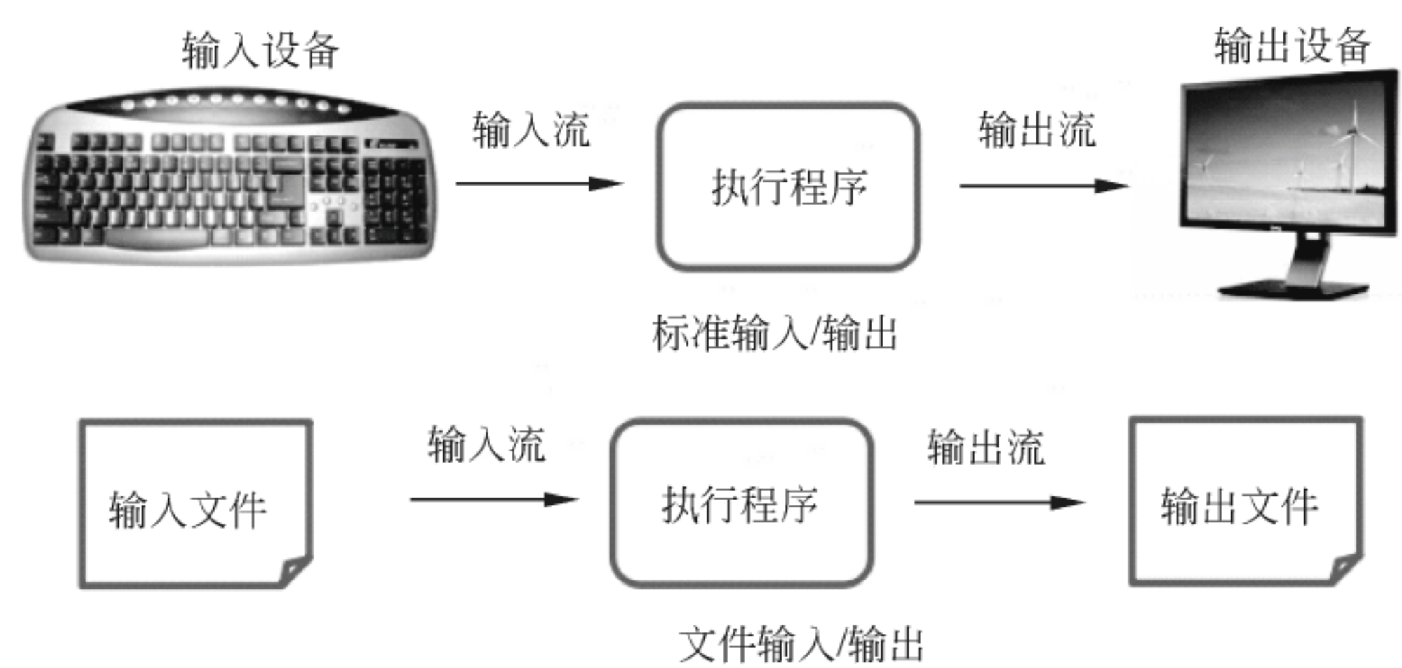
图 1-22 输入/输出流
