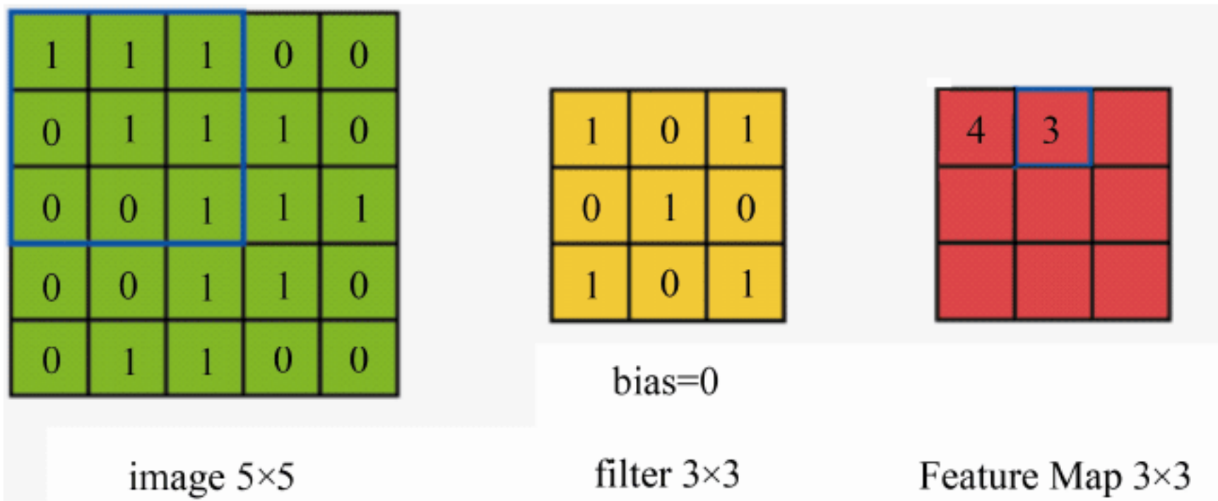
图 19-6 卷积原理图 2
