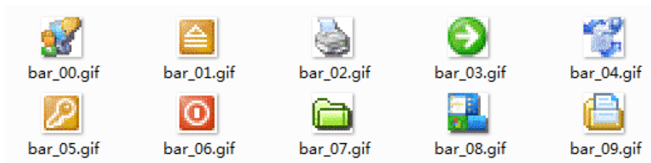
图 10-2 图标方块
