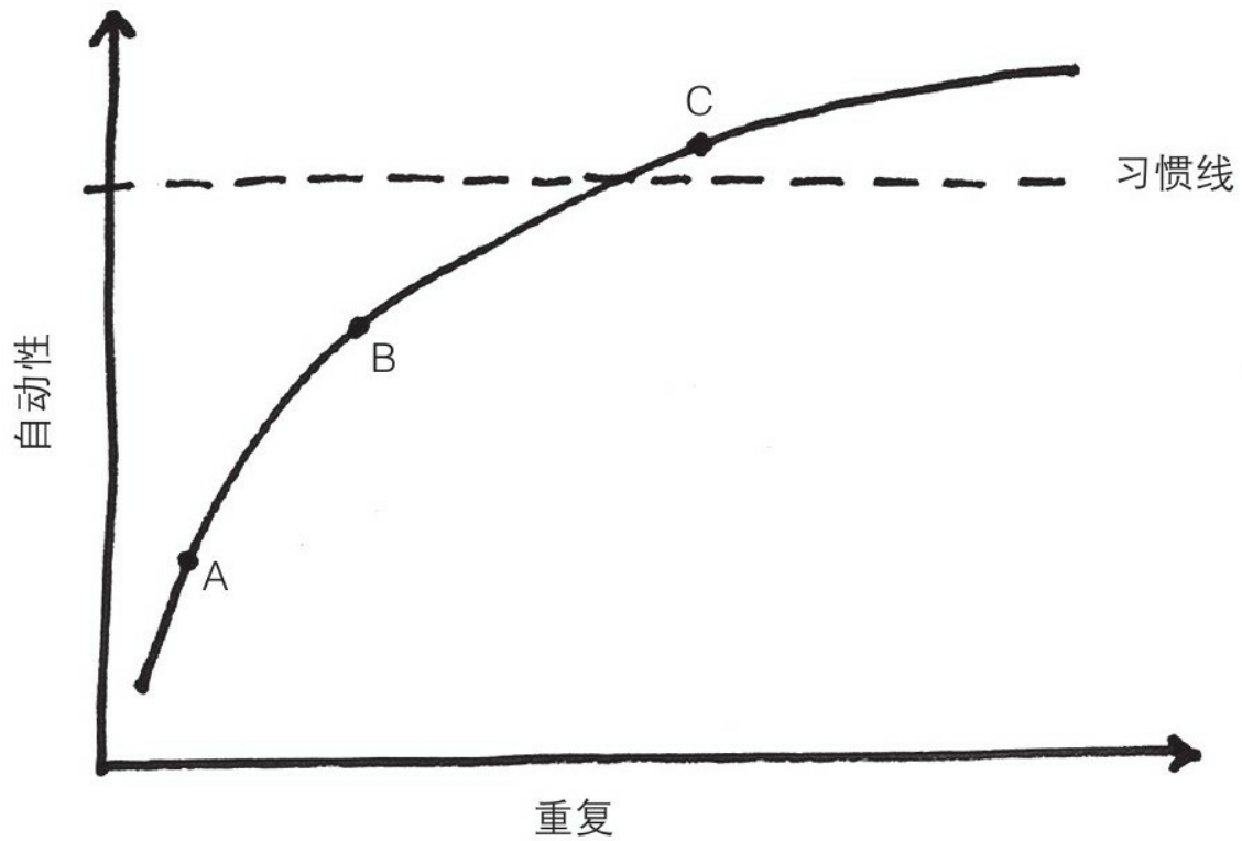
图11：在开始时（A点），一个习惯动作需要极大的努力和专注才能完成。在重复几次后（B点），它变得容易了一些，但是仍然需要有意为之。经过足够的练习（C点），习惯成自然，无须有意为之。超越这个界限，即习惯线之后，就可以不假思索地自动完成这个动作，就此形成了一种习惯
