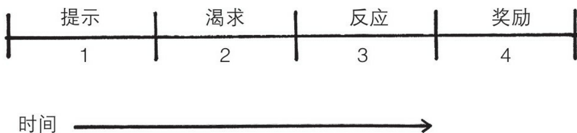
图5：所有习惯的形成都会经历相同顺序的四个阶段：提示、渴求、反应和奖励
