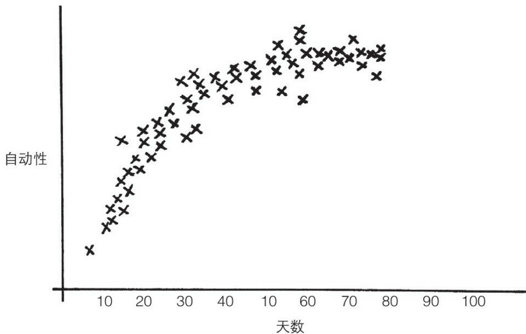
图12：这个图表显示了一个人养成了每天早餐后步行十分钟的习惯。请注意，随着重复次数的增加，自动化程度也会增加，直到行为尽可能简单和自动化
