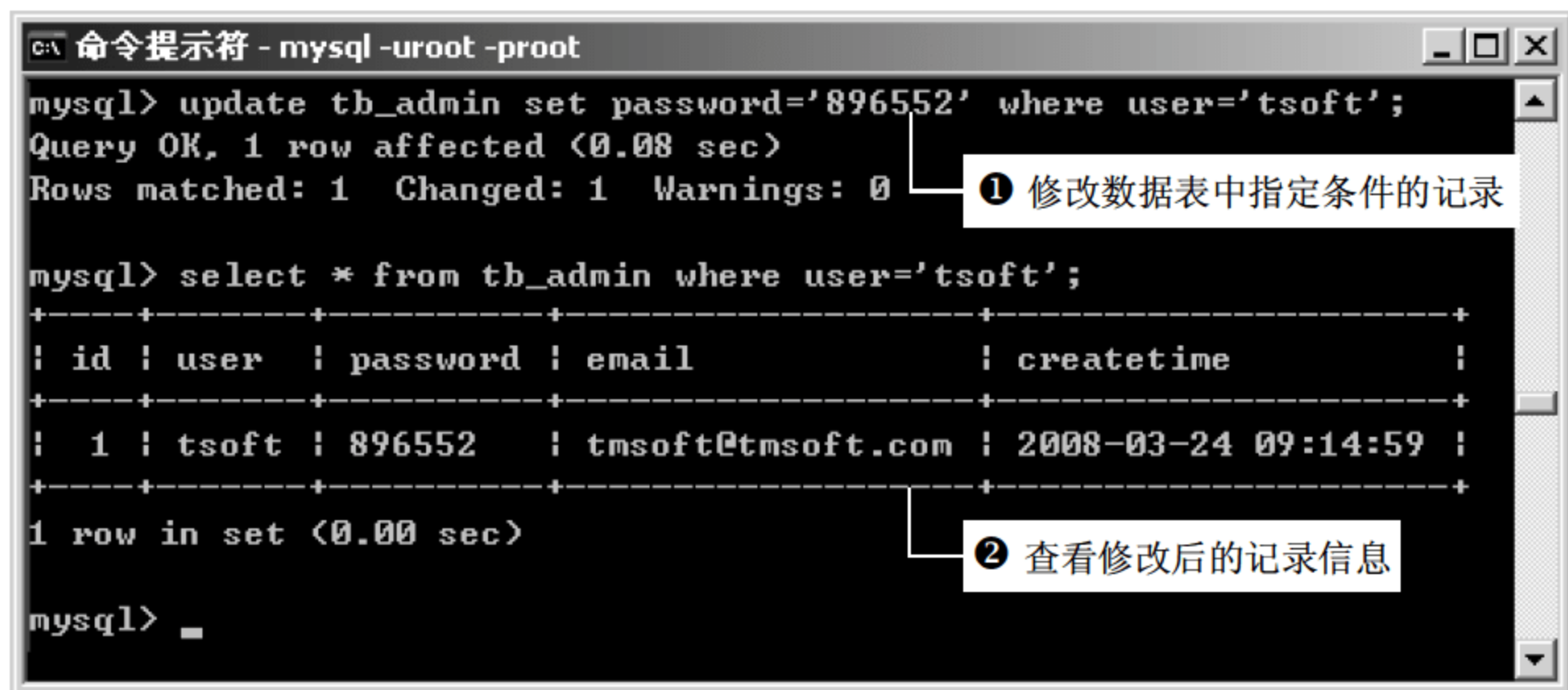
图 16.22 修改指定条件的记录
