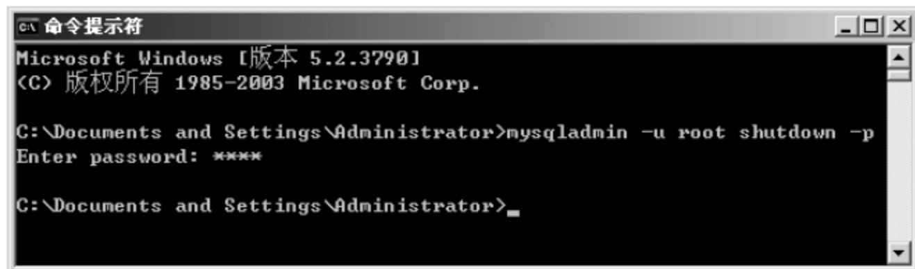
图 16.8 使用 mysqladmin 命令停止 MySQL 服务器
