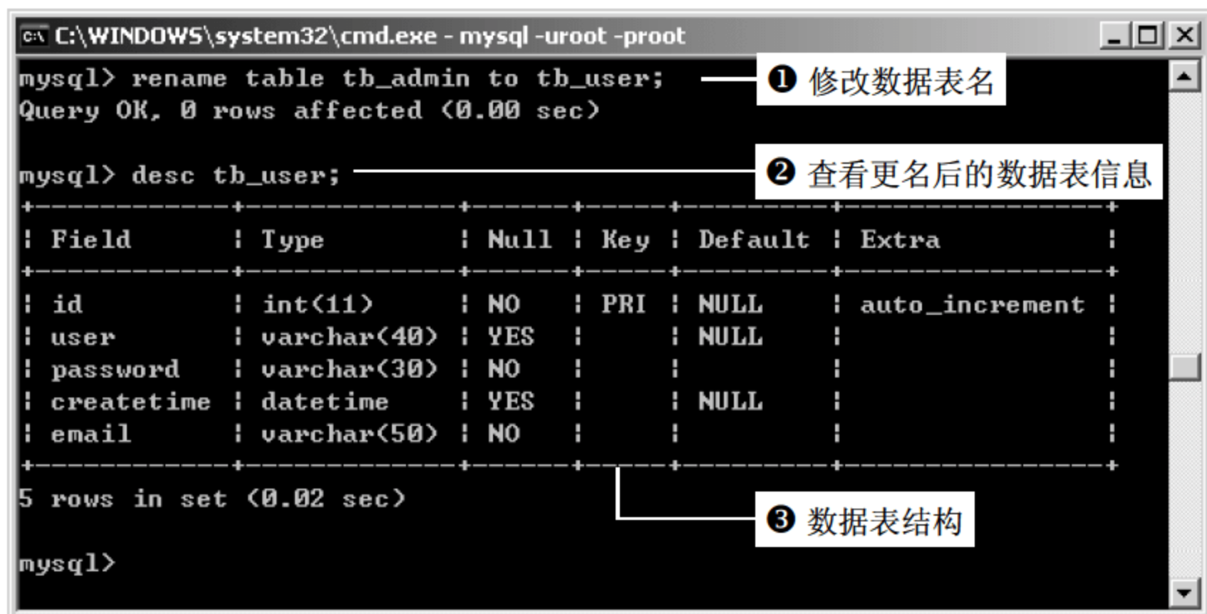
图 16.17 对数据表进行更名
