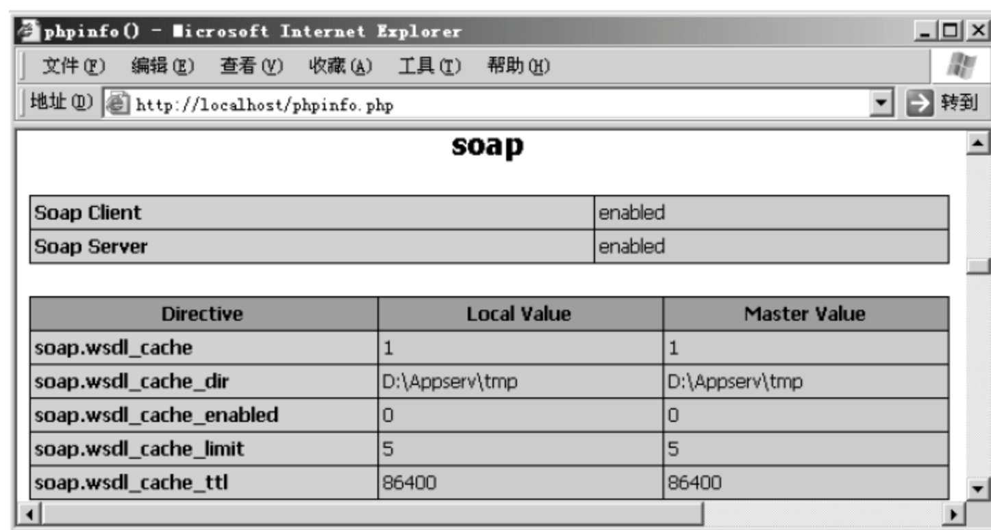
图 25.1 phpinfo.php 中关于 SOAP 的信息
