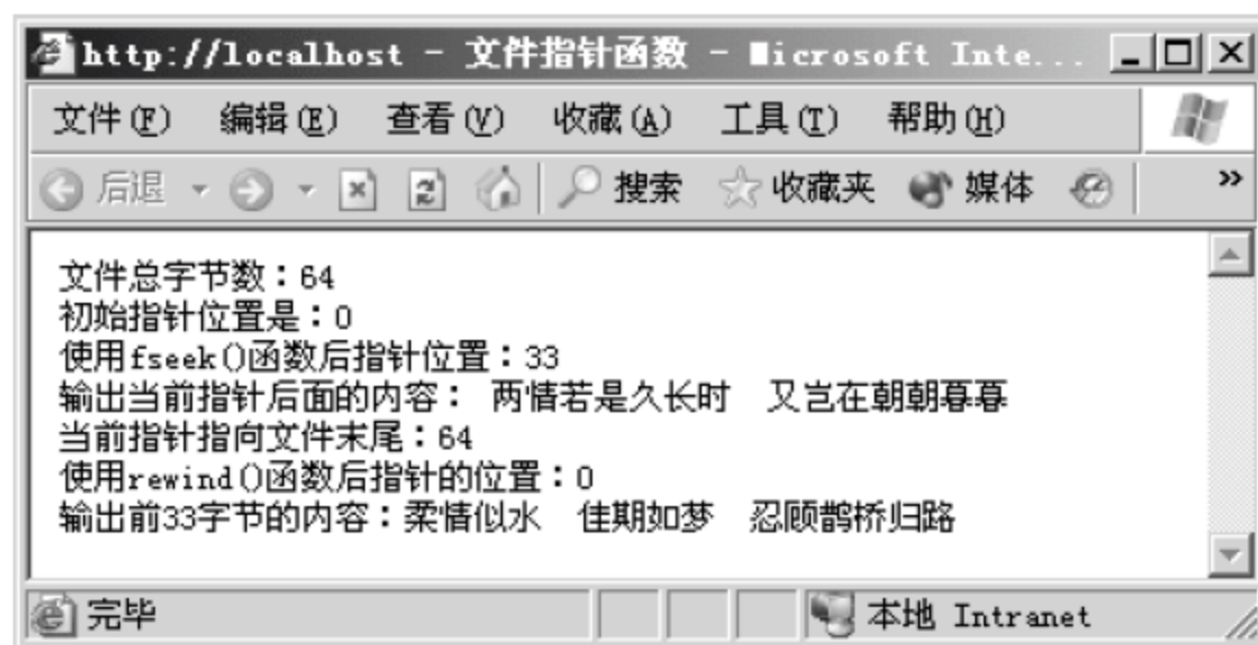
图 13.7 文件指针函数
