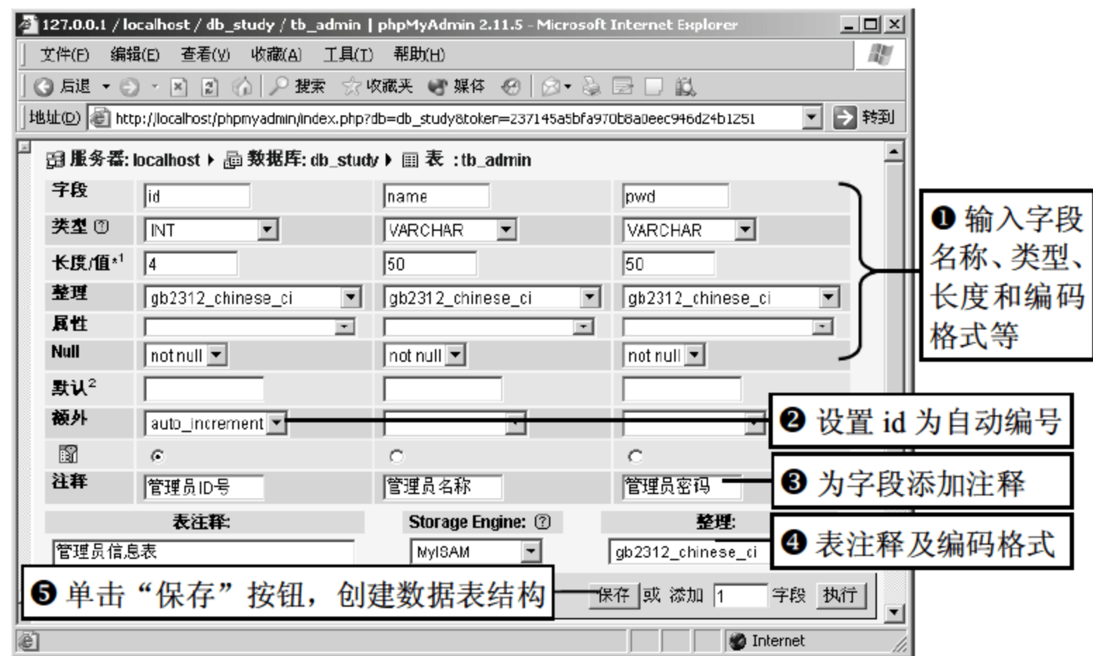
图 17.9 创建数据表结构
