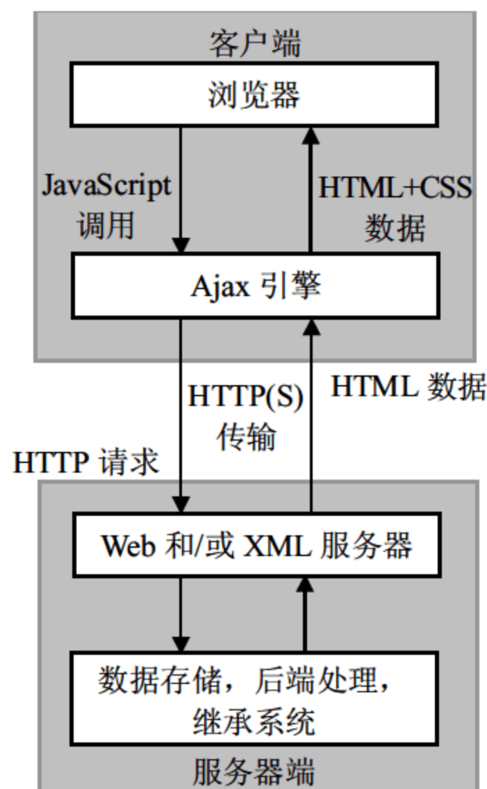
图 24.2 Ajax 的开发模式
