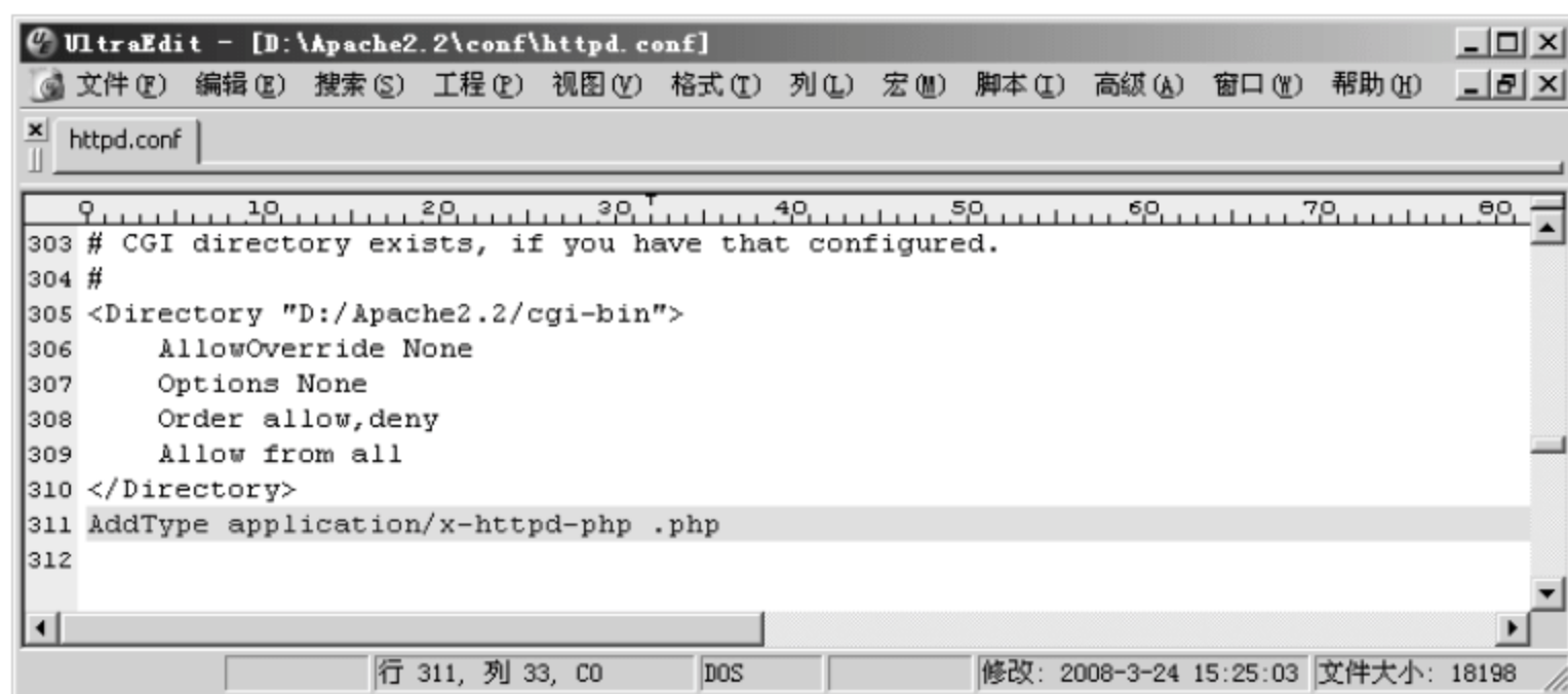
图 2.19 添加 PHP 扩展识别
