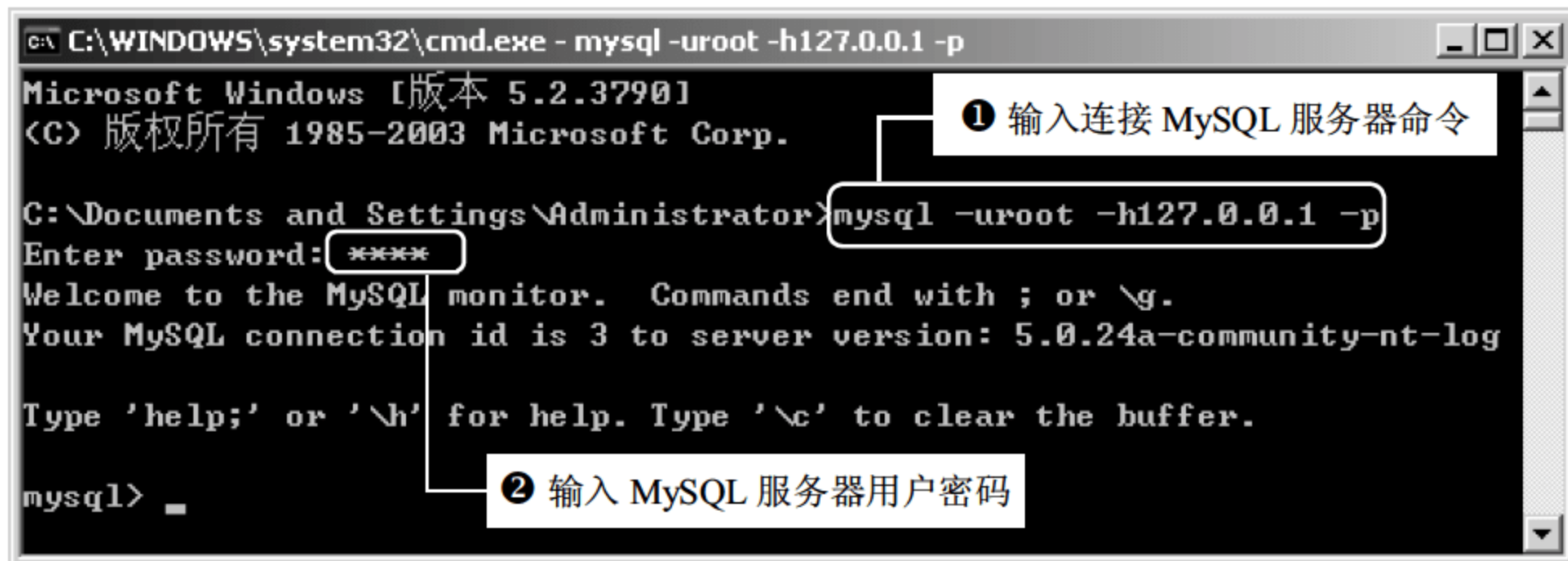
图 16.3 连接 MySQL 服务器
