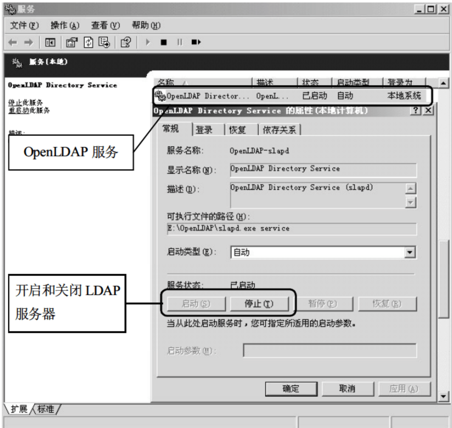
图 23.3 开启和关闭 OpenLDAP 服务
