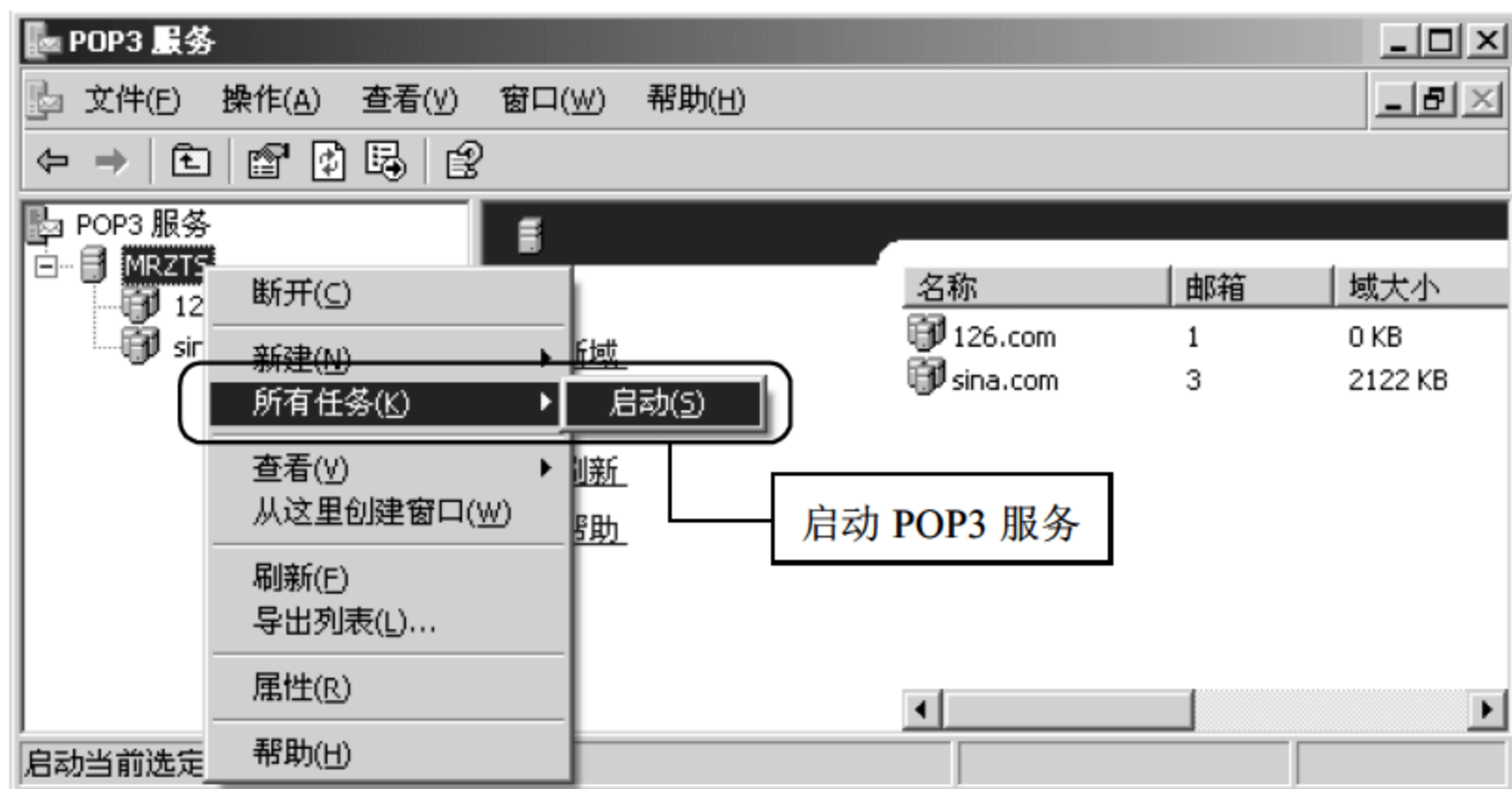
图 21.19 启动 POP3 服务
