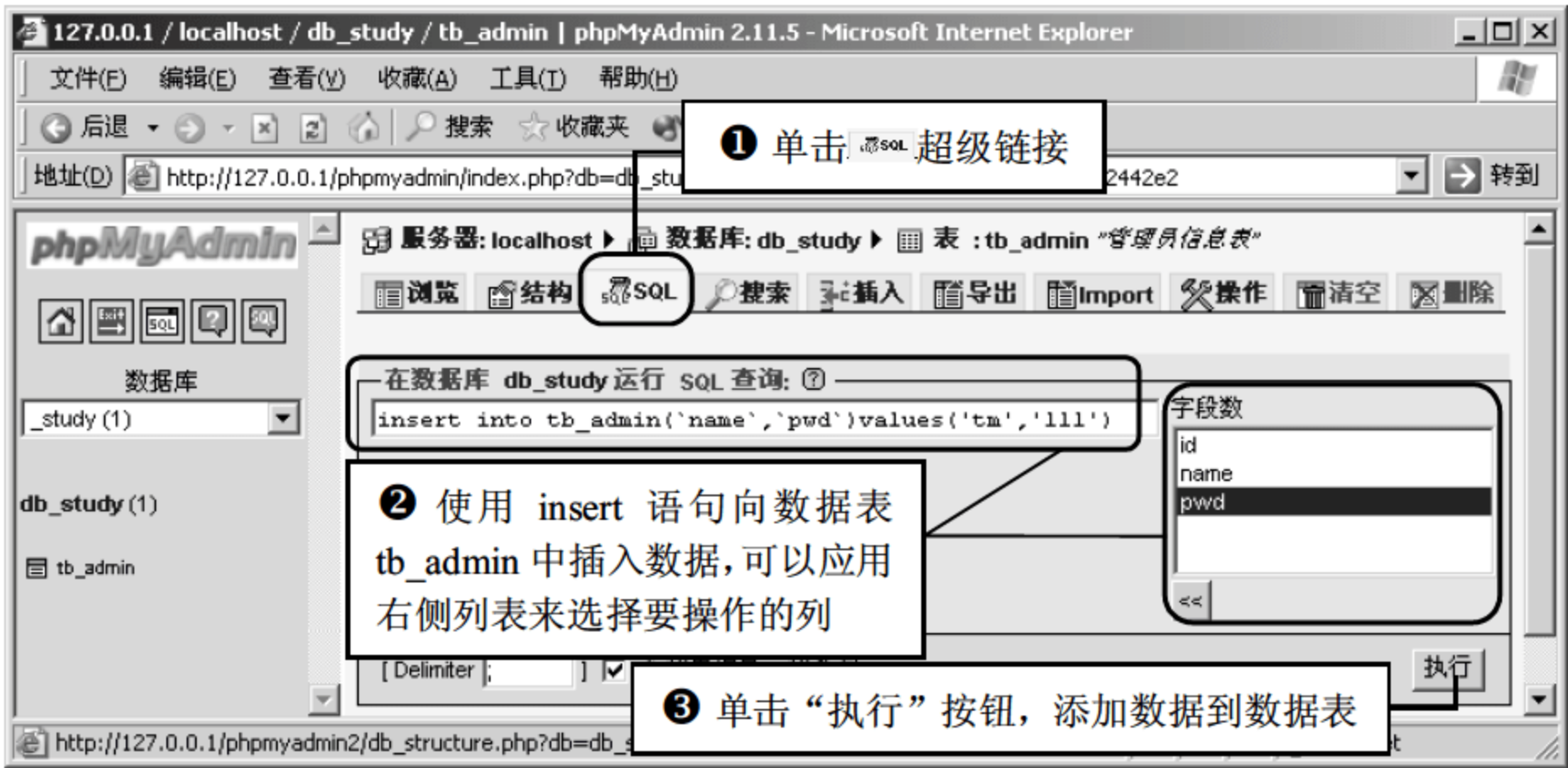
图 17.12 使用 SQL 语句向数据表中插入数据
