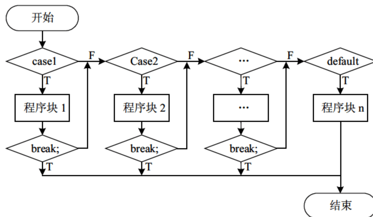
图 4.5 switch 语句流程控制图
