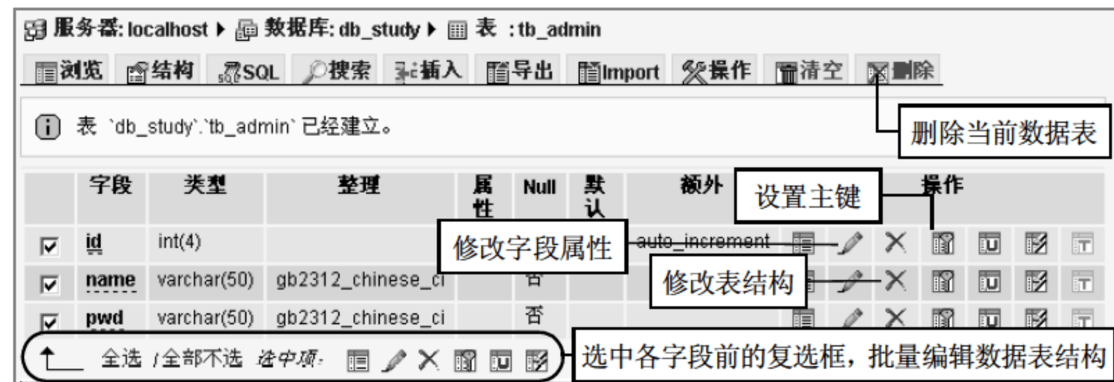
图 17.11 修改数据表结构
