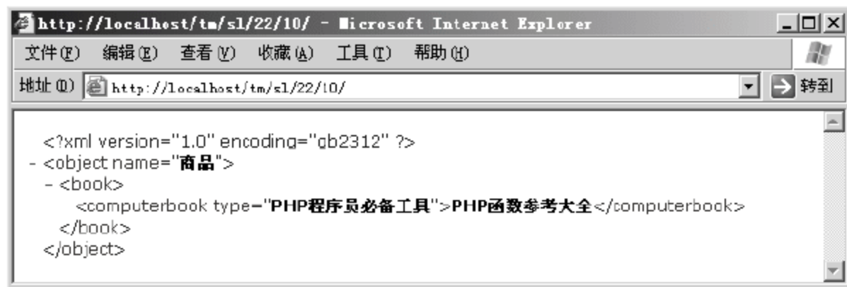
图 22.6 保存 SimpleXML 对象
