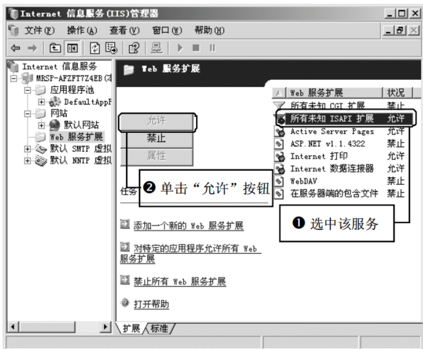
图 2.27 开启 ISAPI 扩展
