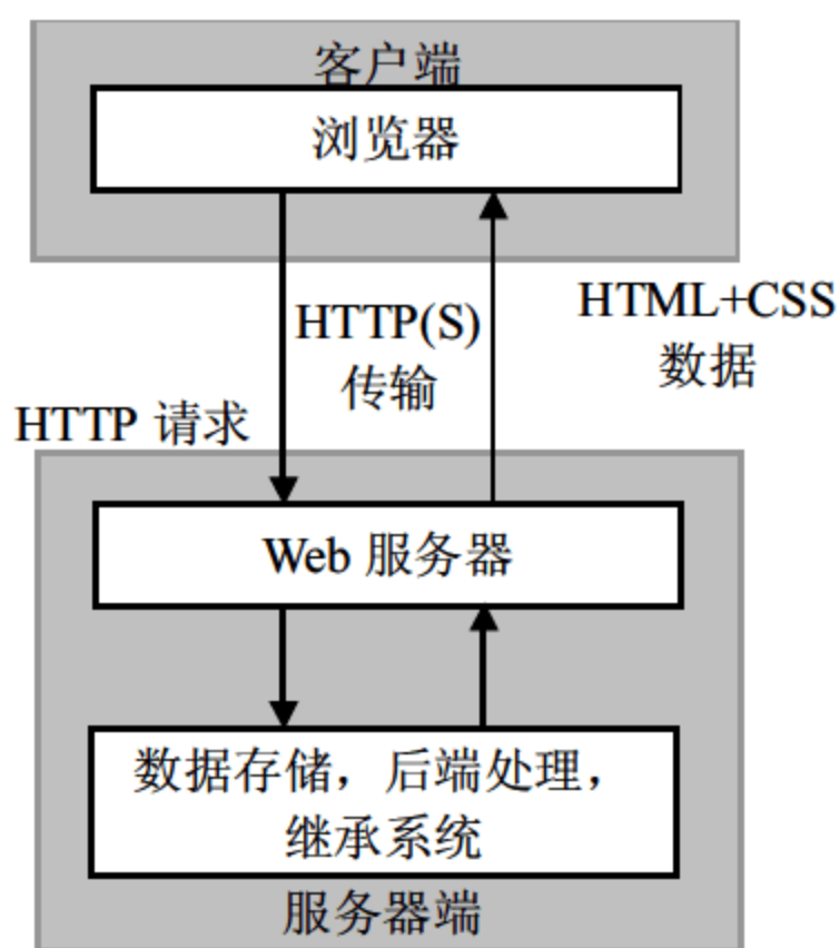
图 24.1 传统的 Web 开发模式
