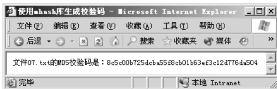
图 15.7 使用 Mhash 库生成校验码
