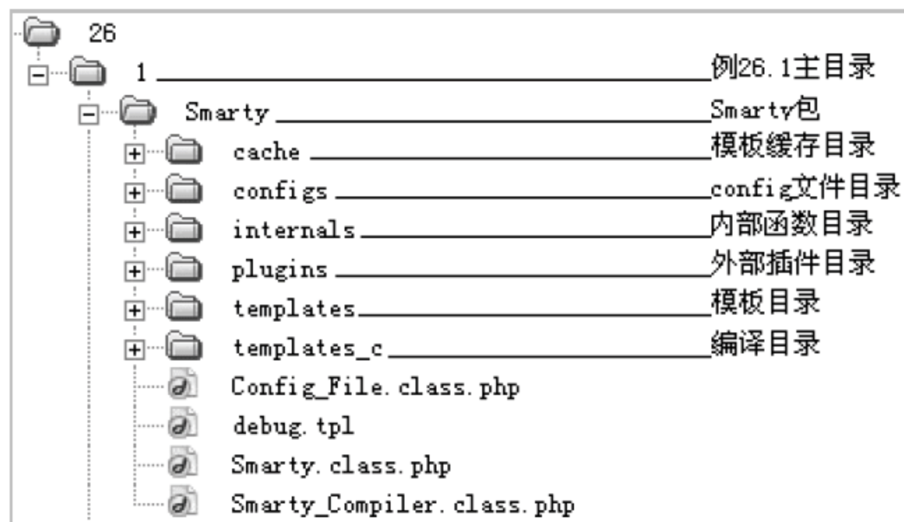
图 26.1 Smarty 包的目录结构
