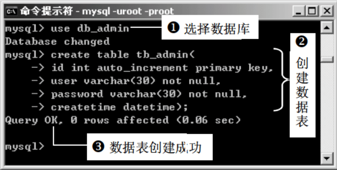
图 16.13 创建 MySQL 数据库
