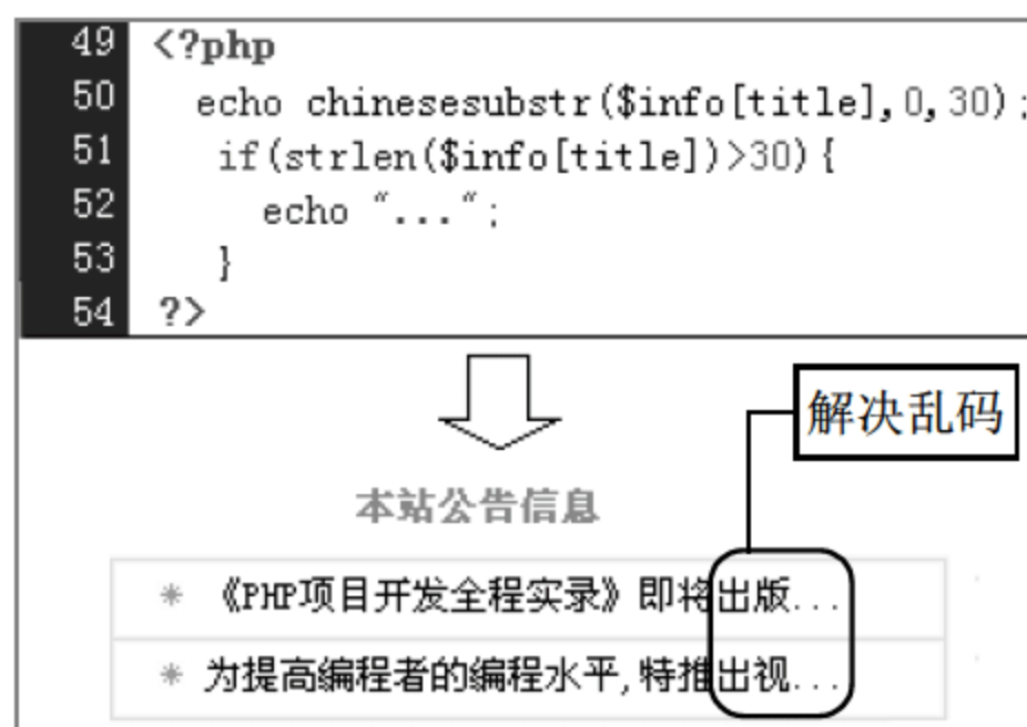
图 18.12 使用自定义 chinesesubstr()函数解决截取字符串乱码
