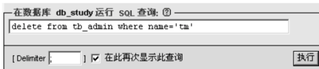
图 17.18 添加删除指定数据信息的 SQL 语句
