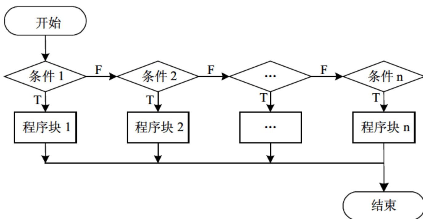
图 4.4 elseif 语句的流程控制图
