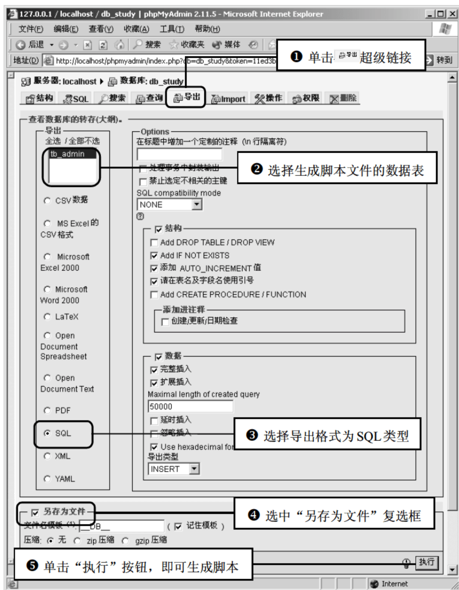
图 17.23 生成 mysql 脚本文件设置界面
