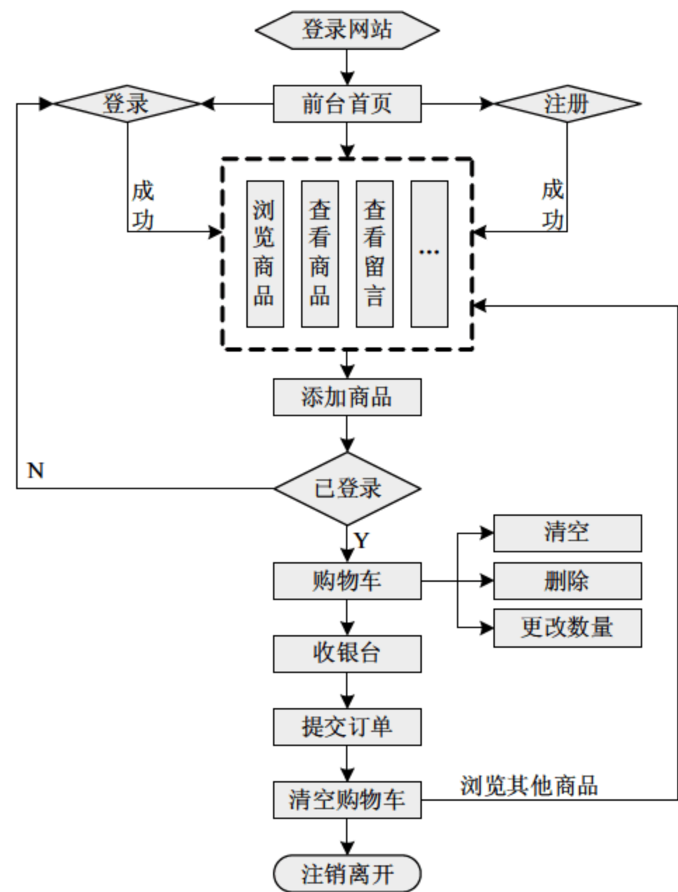
图 27.3 系统流程图
