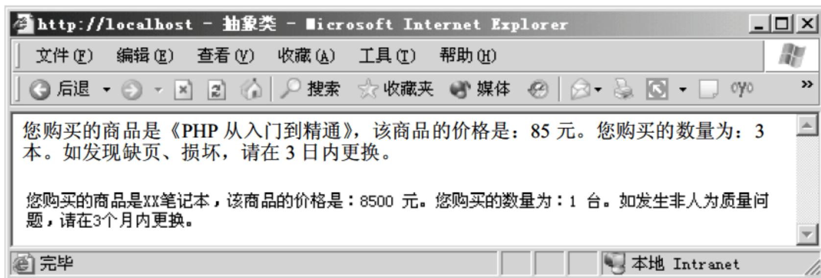
图 14.5 抽象类
