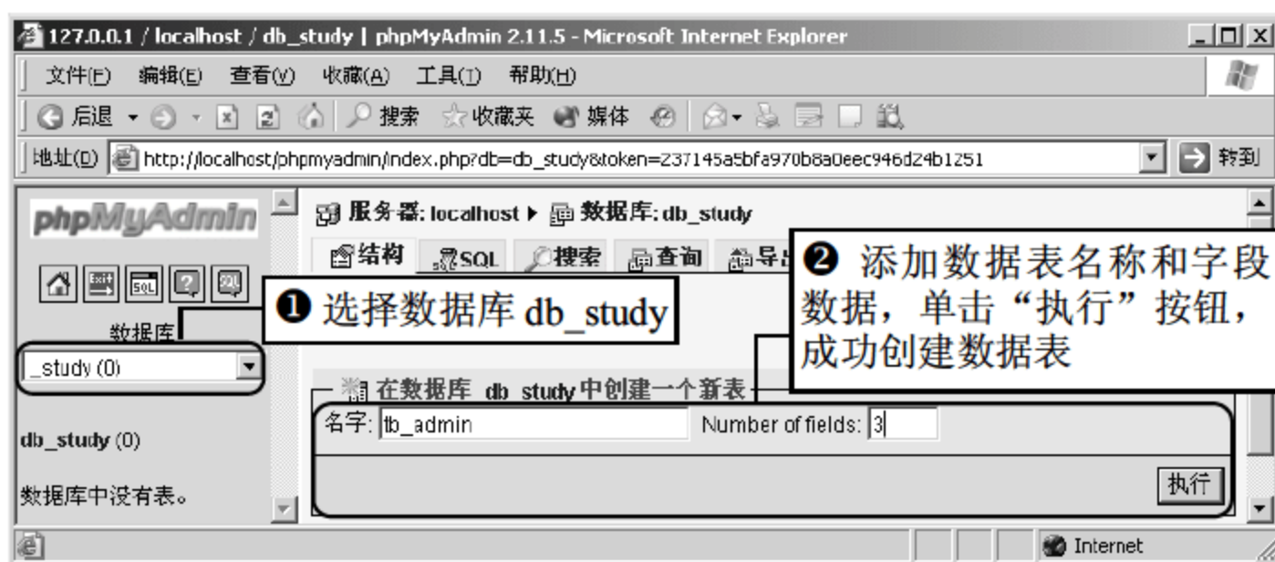
图 17.8 创建数据表
