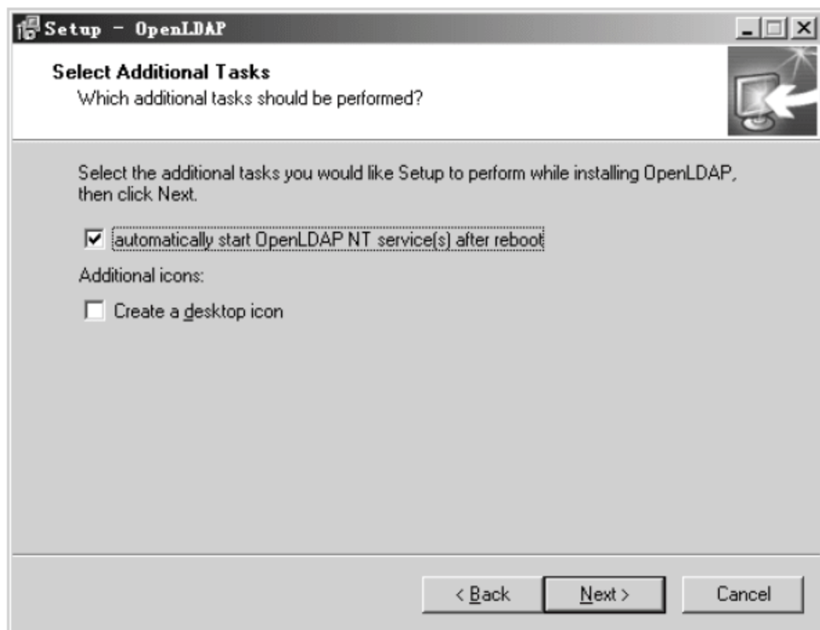
图 23.2 选择启动项
