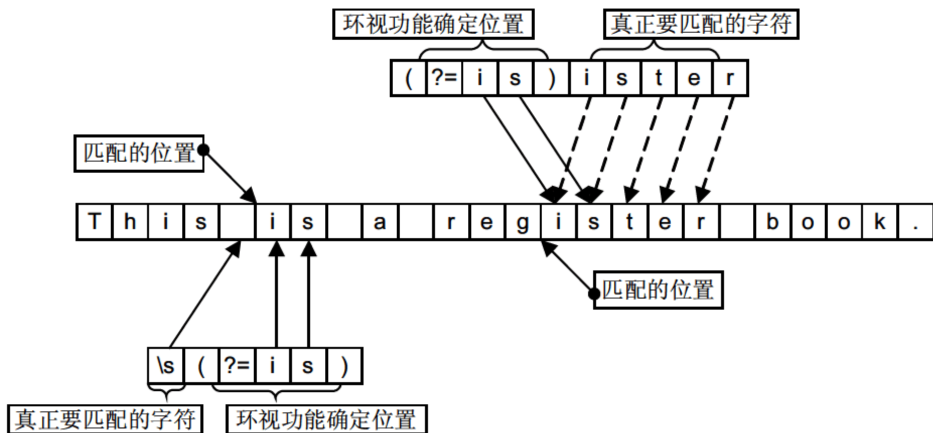
图 6.1 顺序环视
