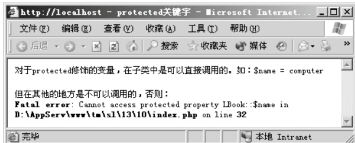
图 14.3 protected 关键字
