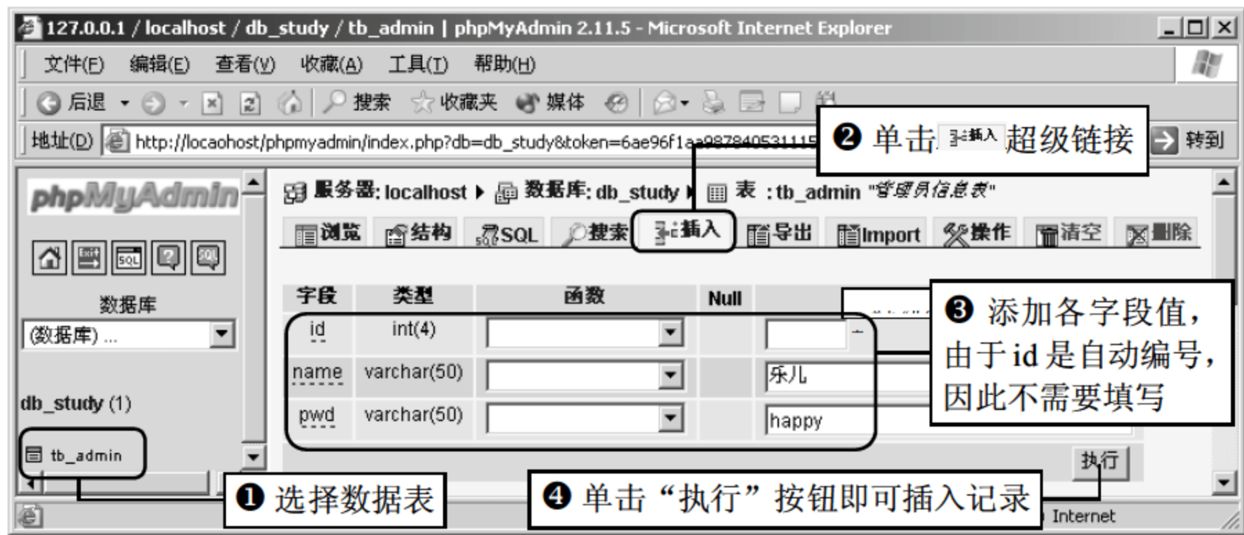
图 17.20 插入数据
