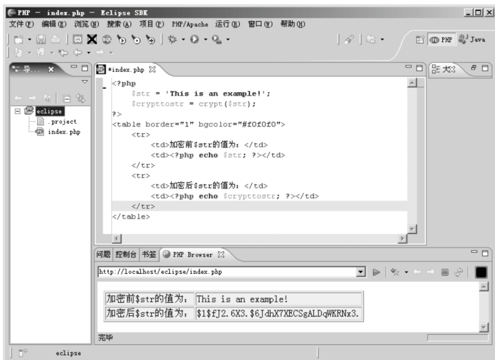
图 2.30 Eclipse3.2
