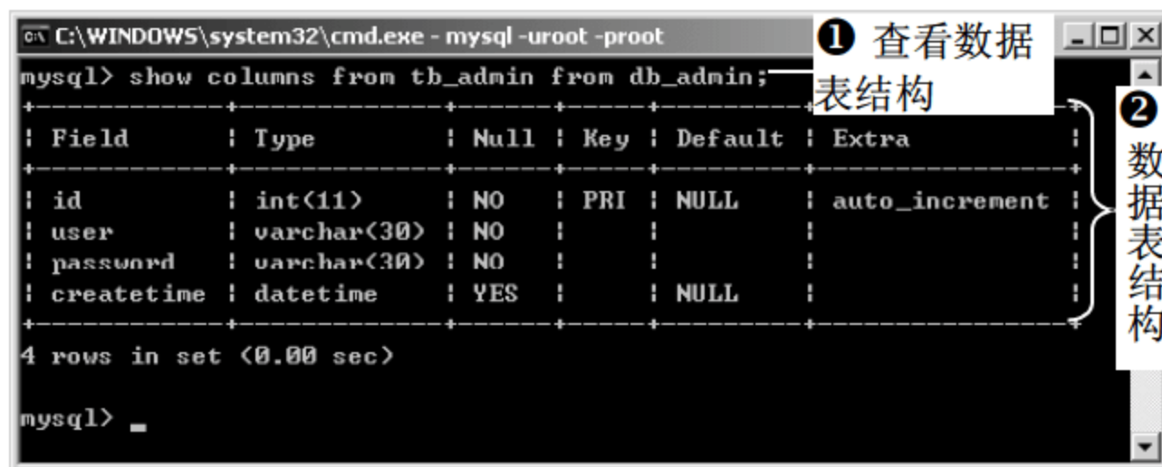
图 16.14 查看表结构
