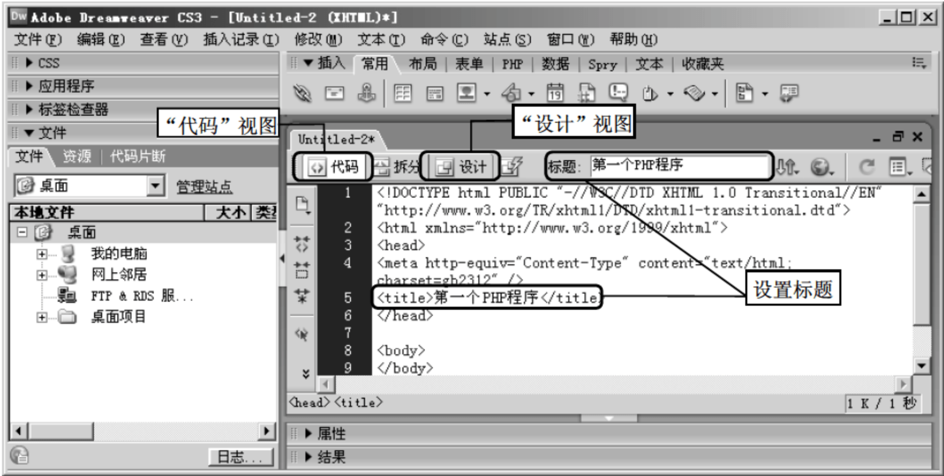
图 2.36 为标题命名
