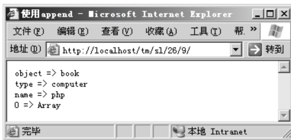
图 26.10 使用 append
