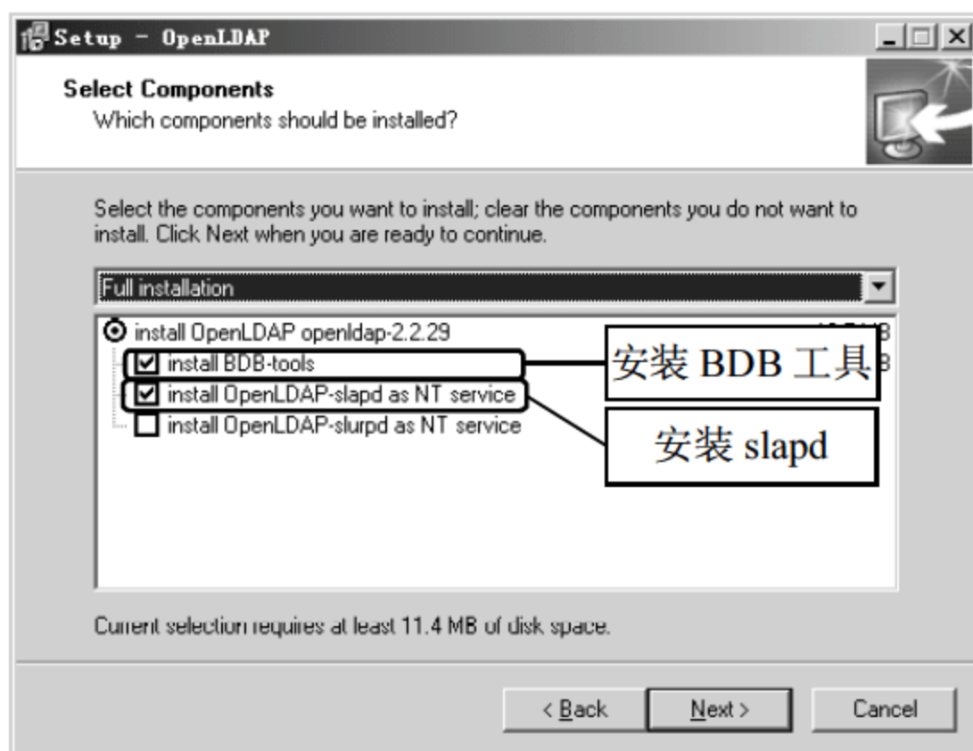
图 23.1 选择组件
