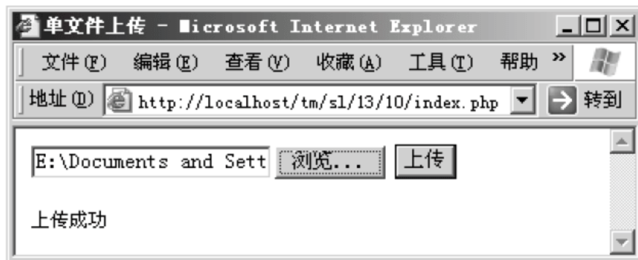
图 13.9 单文件上传
