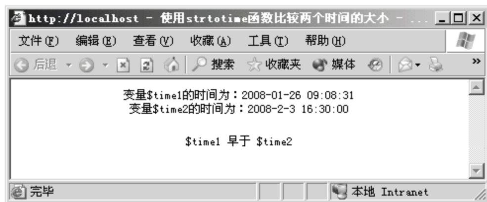
图 10.8 使用 strtotime() 函数比较两个时间的大小
