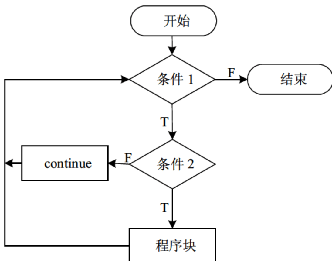
图 4.15 continue 流程控制图
