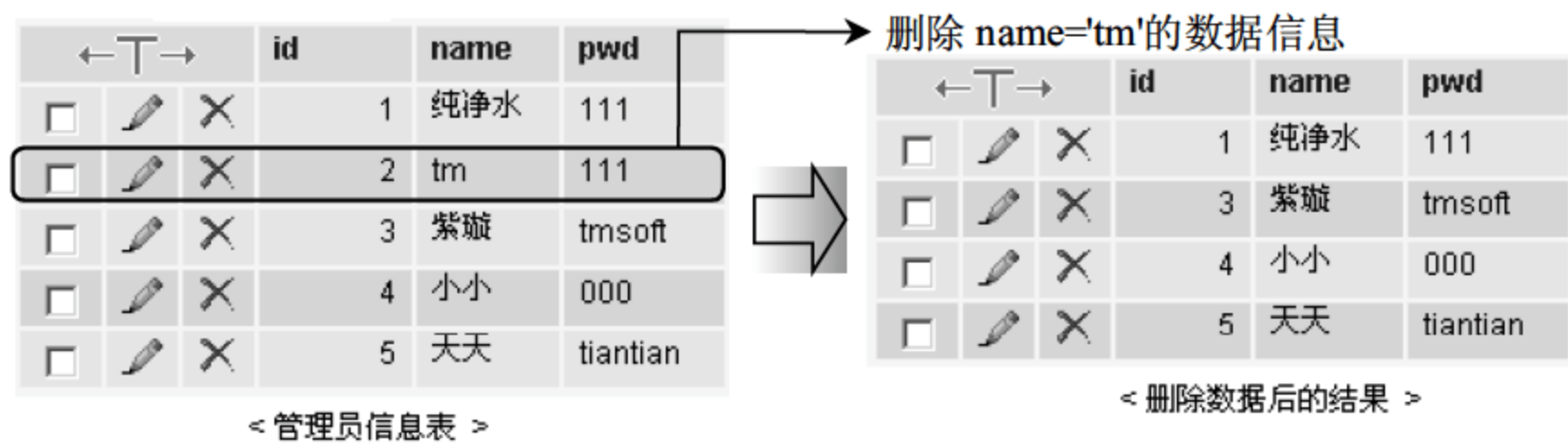
图 17.19 删除指定条件的数据信息的实现过程
