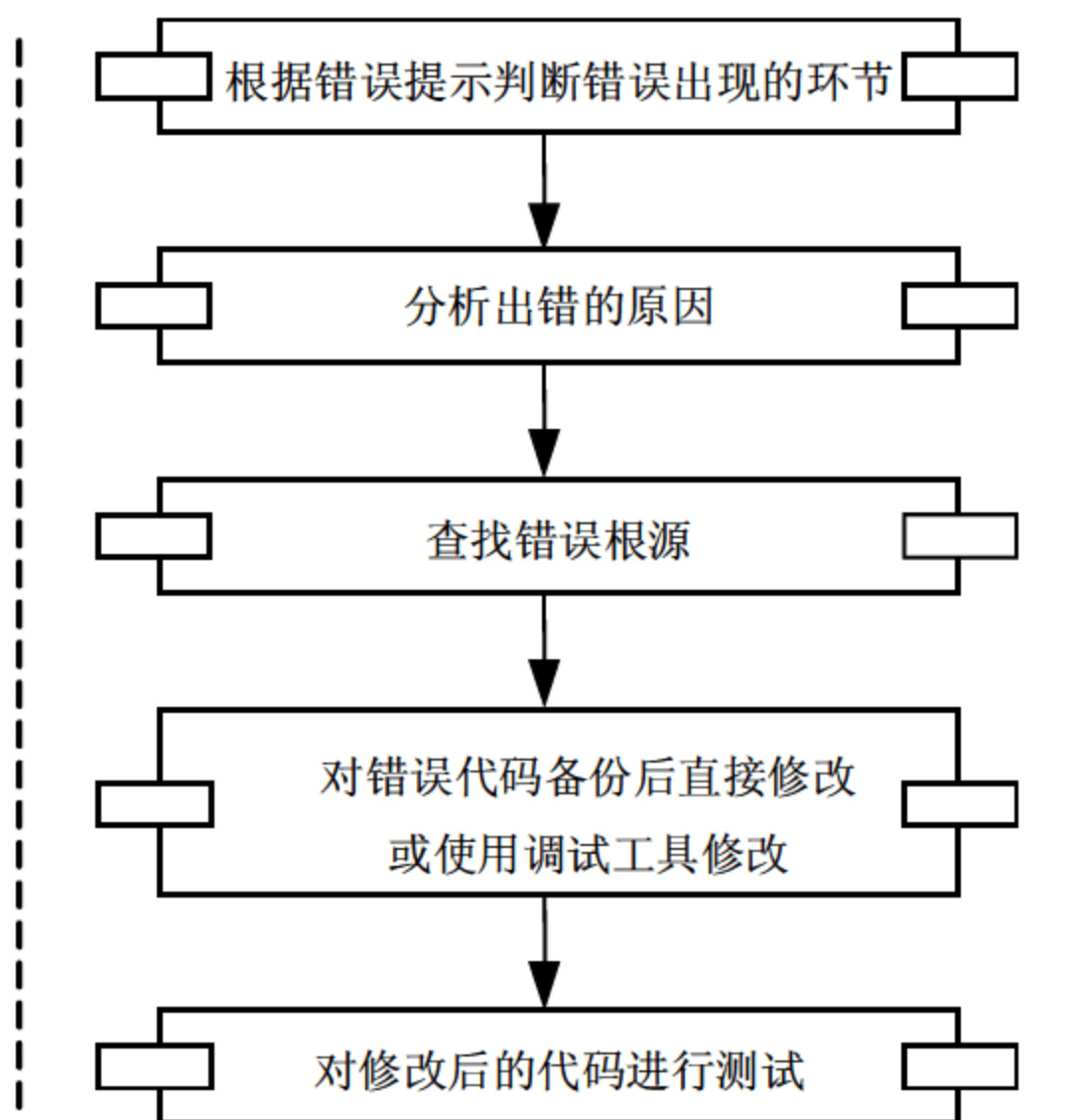
图 20.1 基本调试流程
