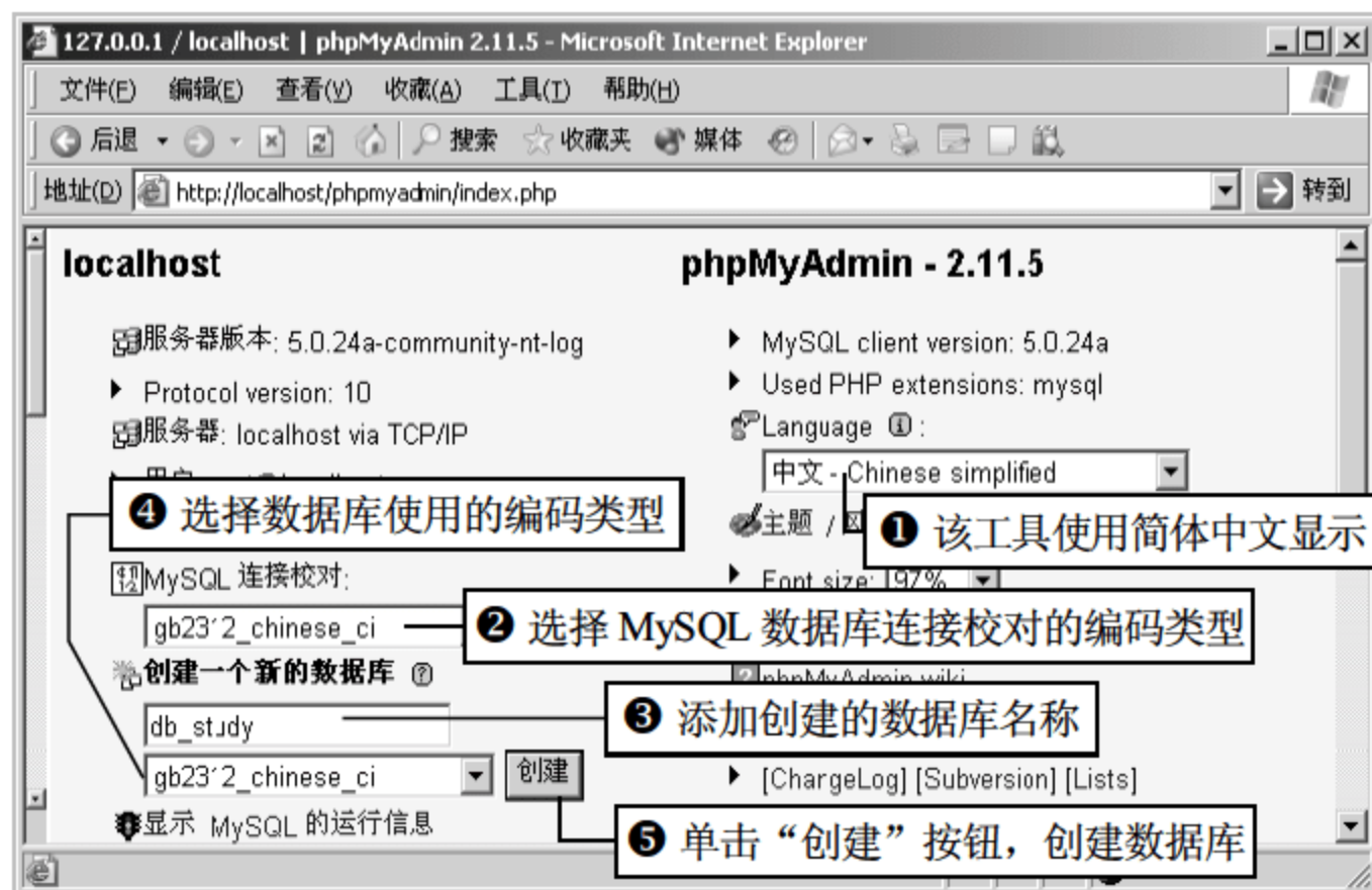
图 17.5 phpMyAdmin 管理主界面
