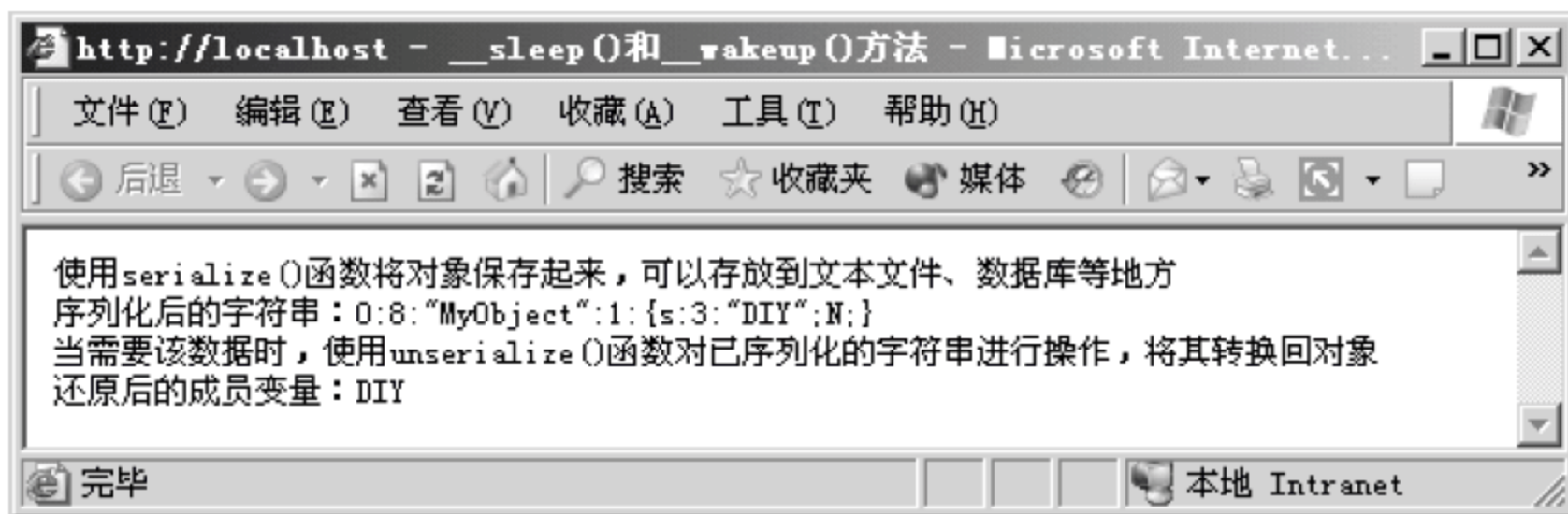
图 14.10 __sleep()和__wakeup()方法
