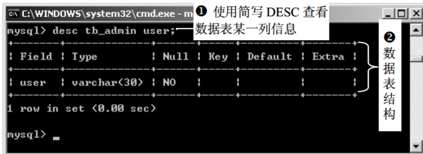
图 16.15 查看表的某一列信息
