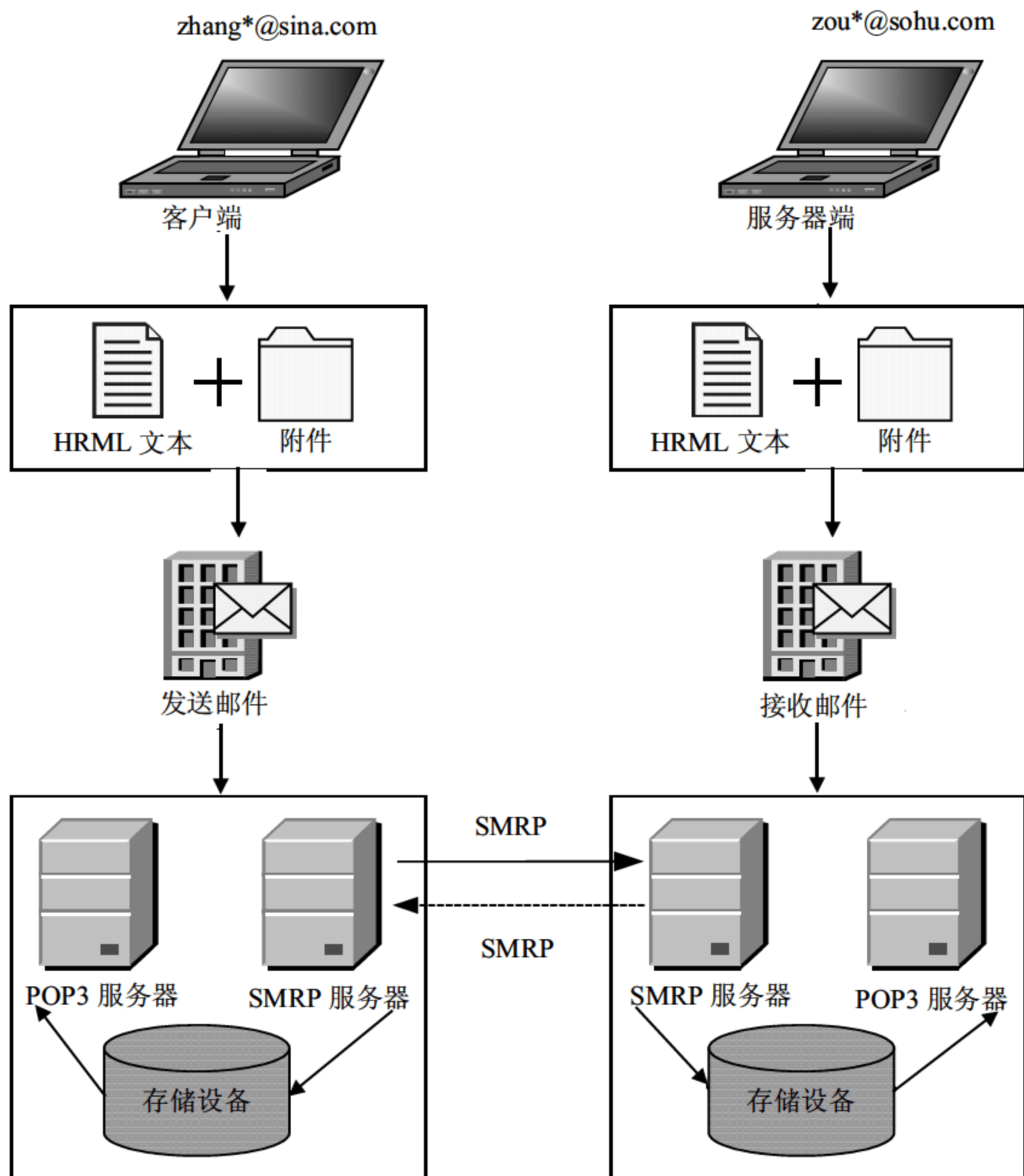
图 21.1 电子邮件的工作原理图
