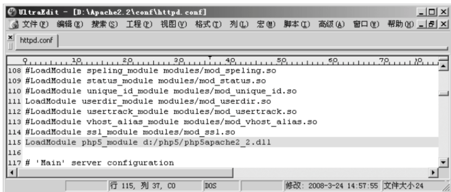
图 2.18 加载 dll 文件
