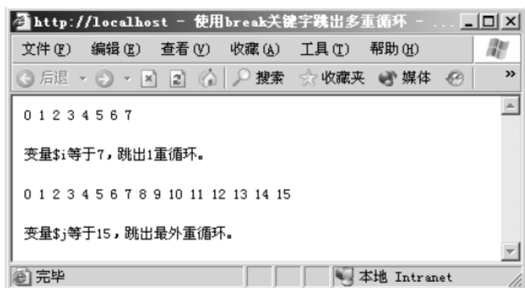
图 4.14 使用 break 关键字跳出多重循环
