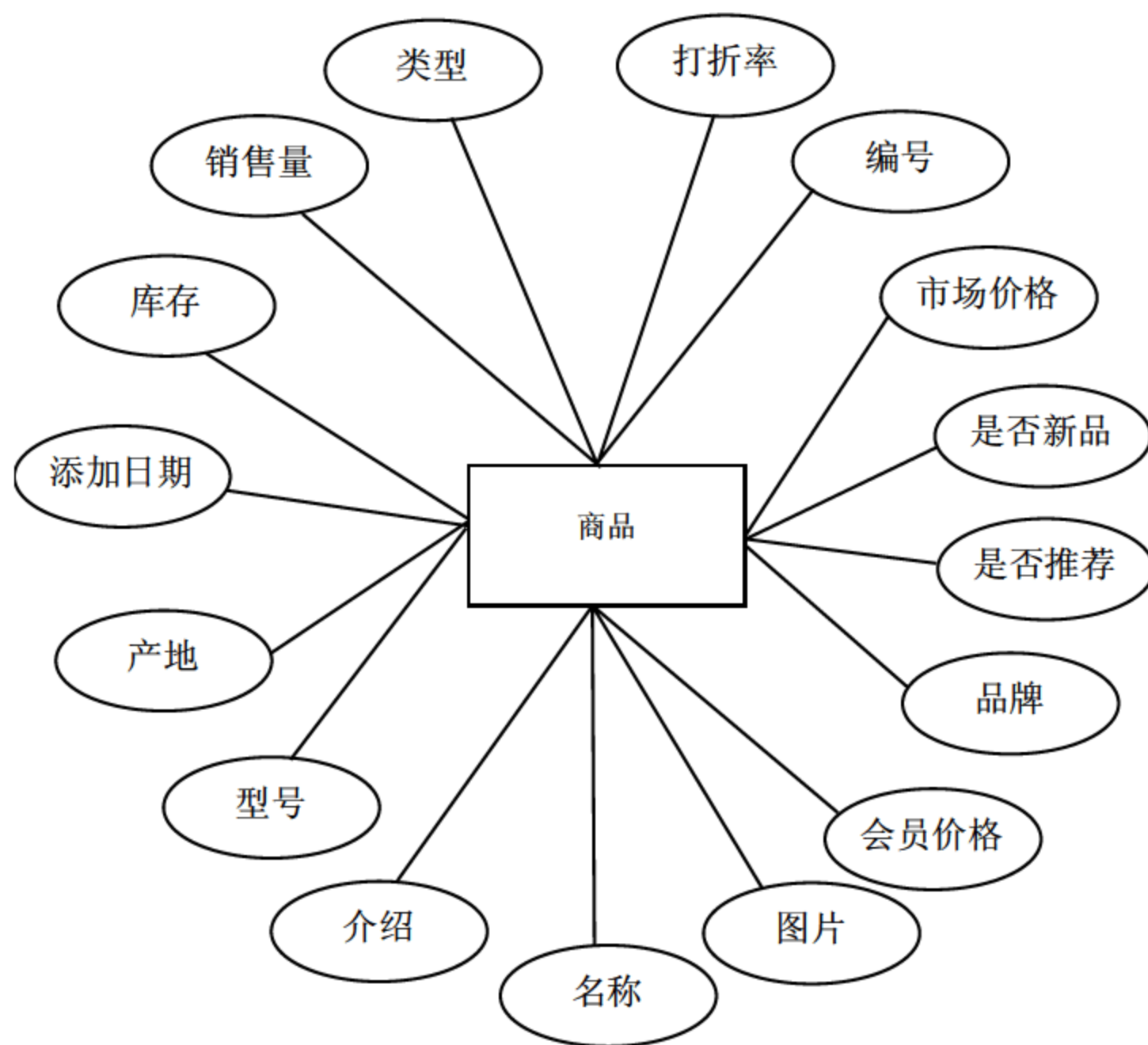
图 27.5 商品信息实体 E-R 图
