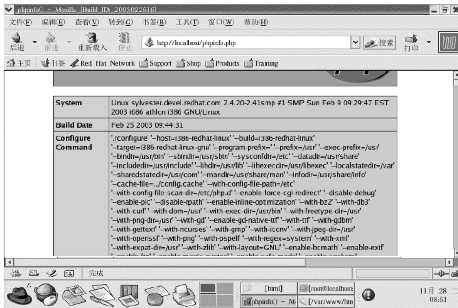
图 2.29 phpinfo 信息
