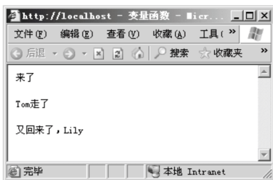
图 3.15 变量函数
