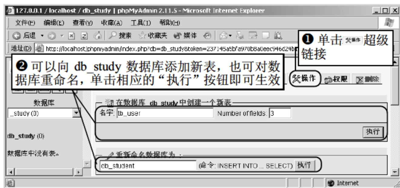
图 17.7 修改数据库
