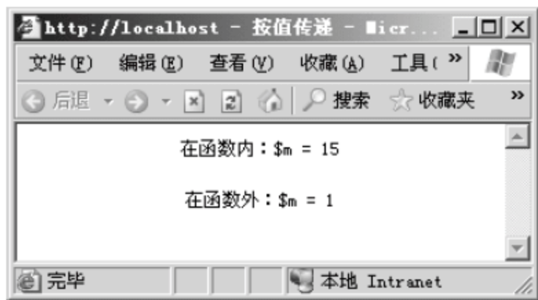
图 3.13 按值传递
