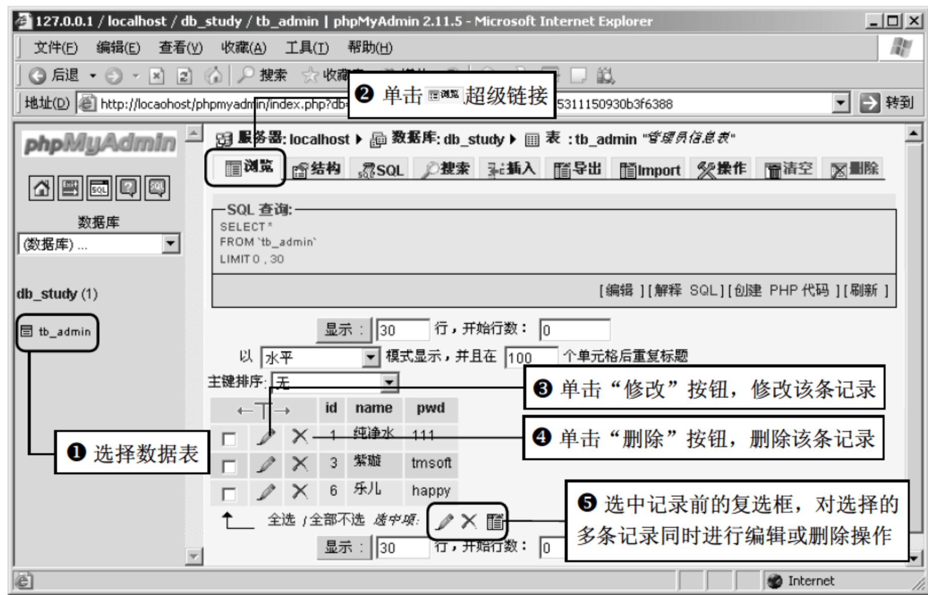
图 17.21 浏览数据
