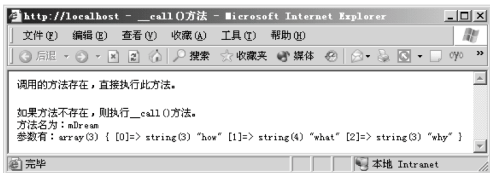
图 14.9 __call()方法
