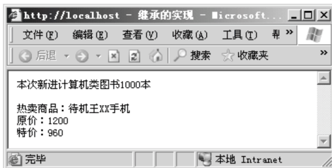
图 14.1 继承的实现
