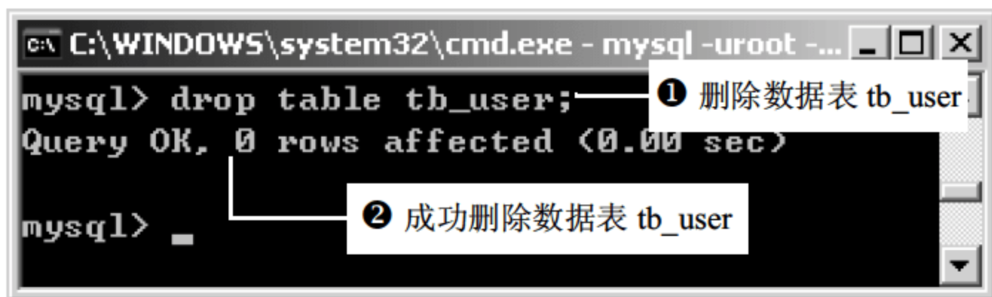
图 16.18 删除数据表
