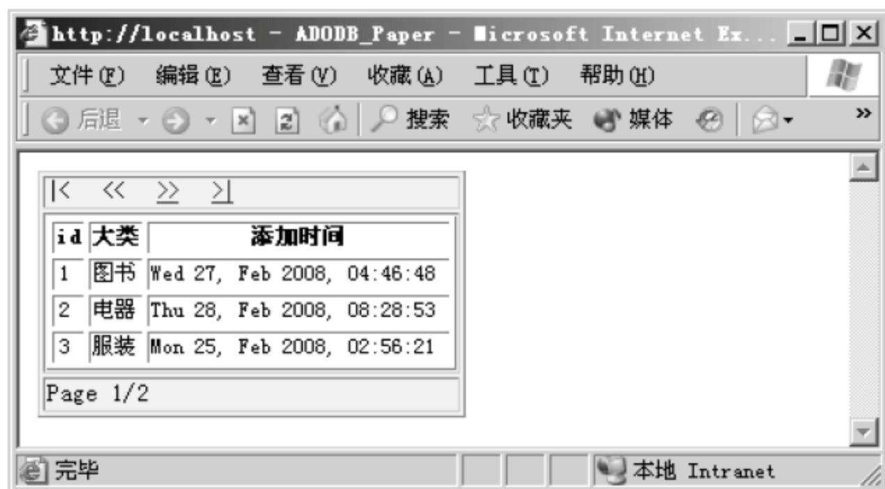
图 19.3 ADODB_Pager
