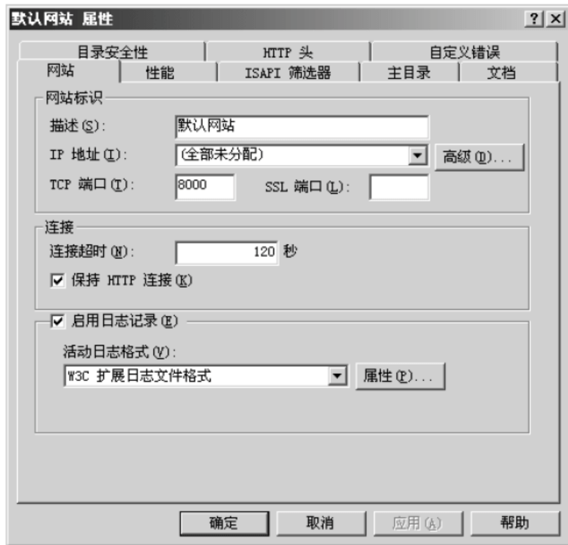
图 2.22 “网站”选项卡
