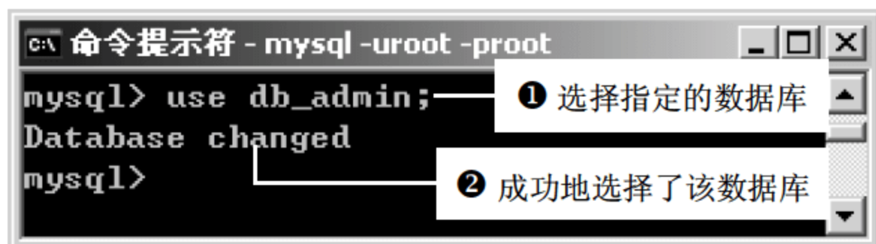
图 16.11 选择数据库
