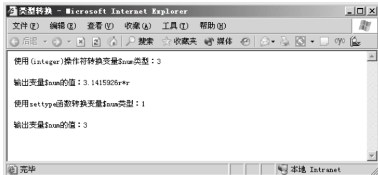
图 3.6 类型转换
