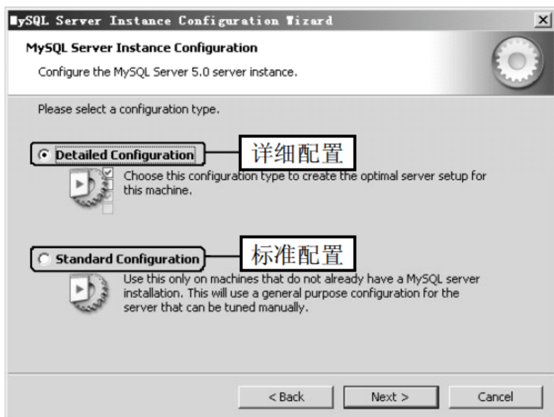
图 2.10 MySQL 界面
