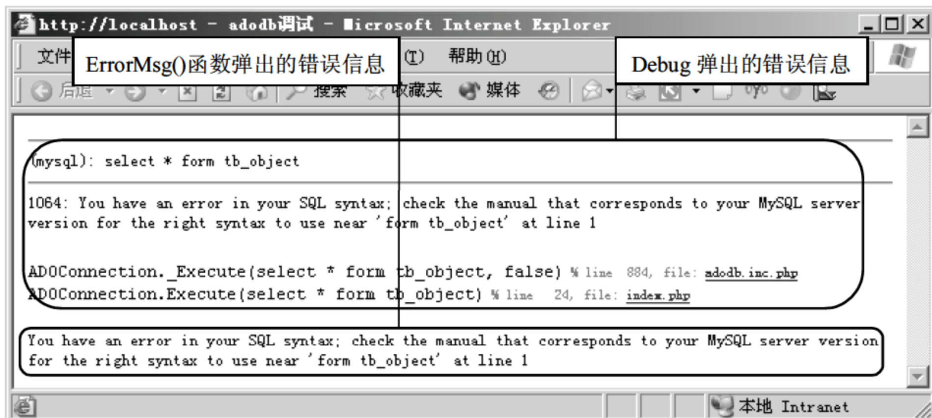
图 19.4 ADODB 调试
