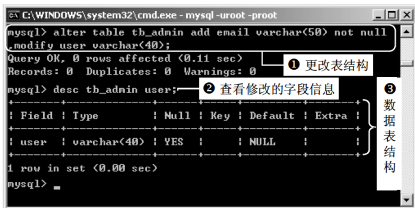
图 16.16 修改表结构
