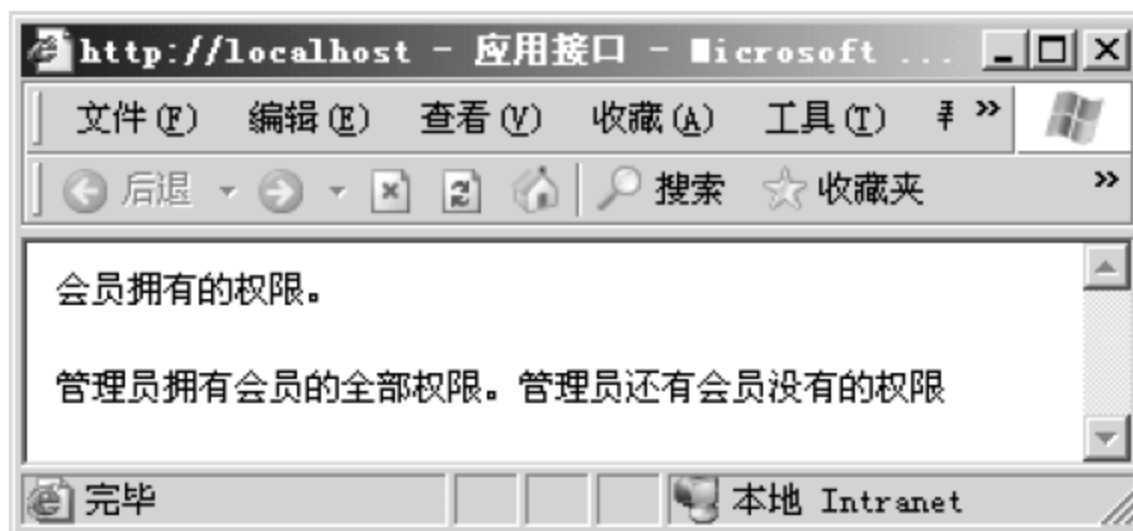
图 14.6 应用接口
