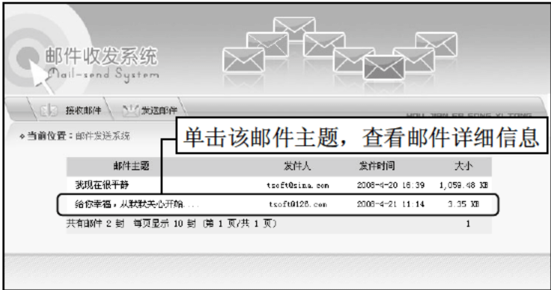
图 21.20 邮件列表
