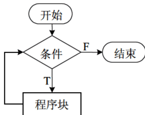
图 4.7 while 语句流程控制图
