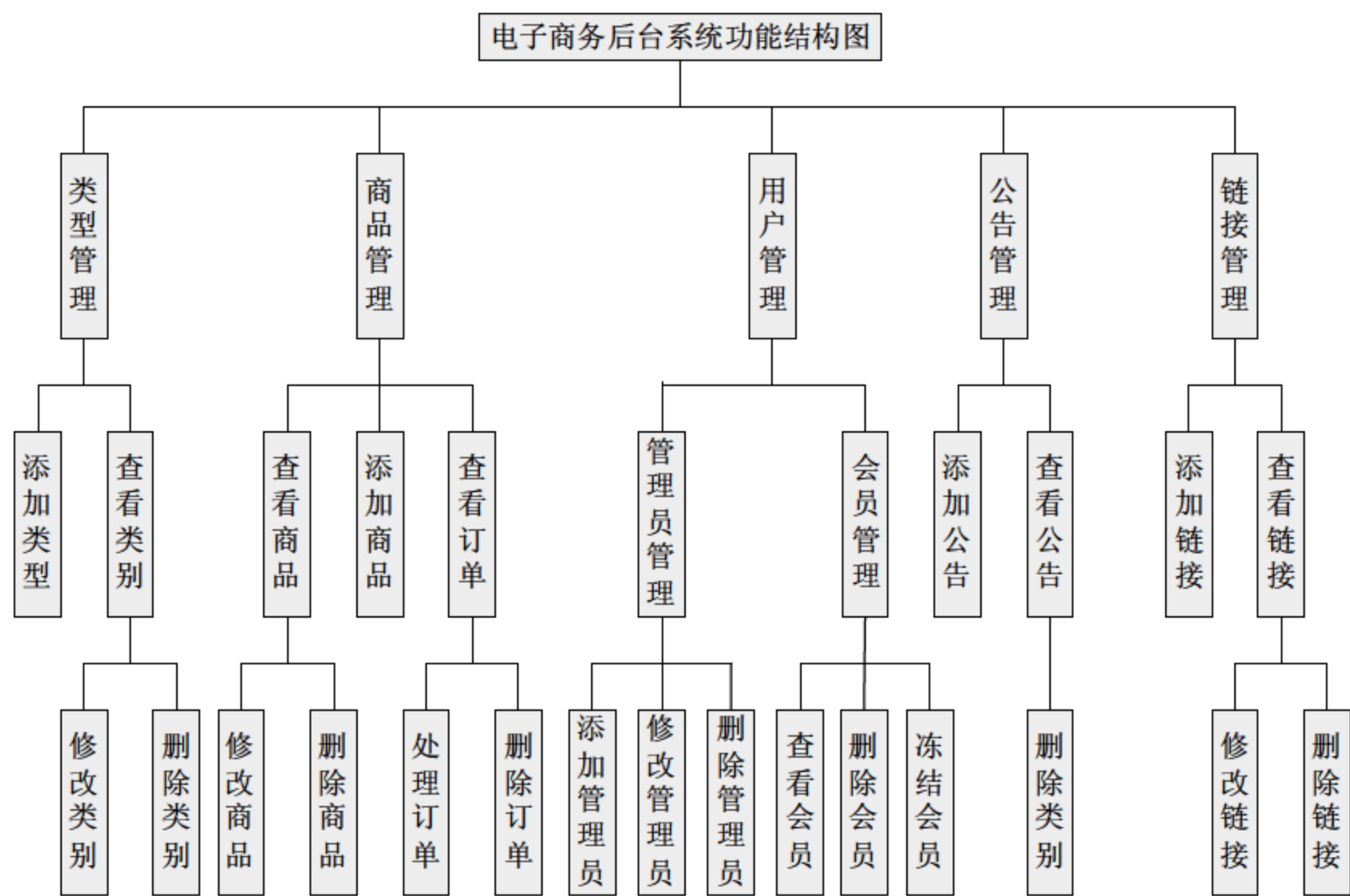
图 27.2 电子商务后台系统功能结构图
