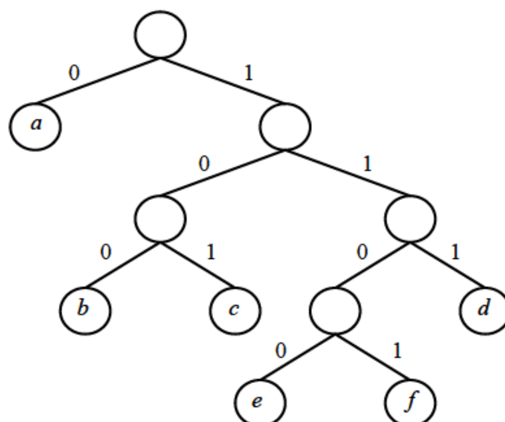
图 5.11 二元前缀码与对应的二叉树
