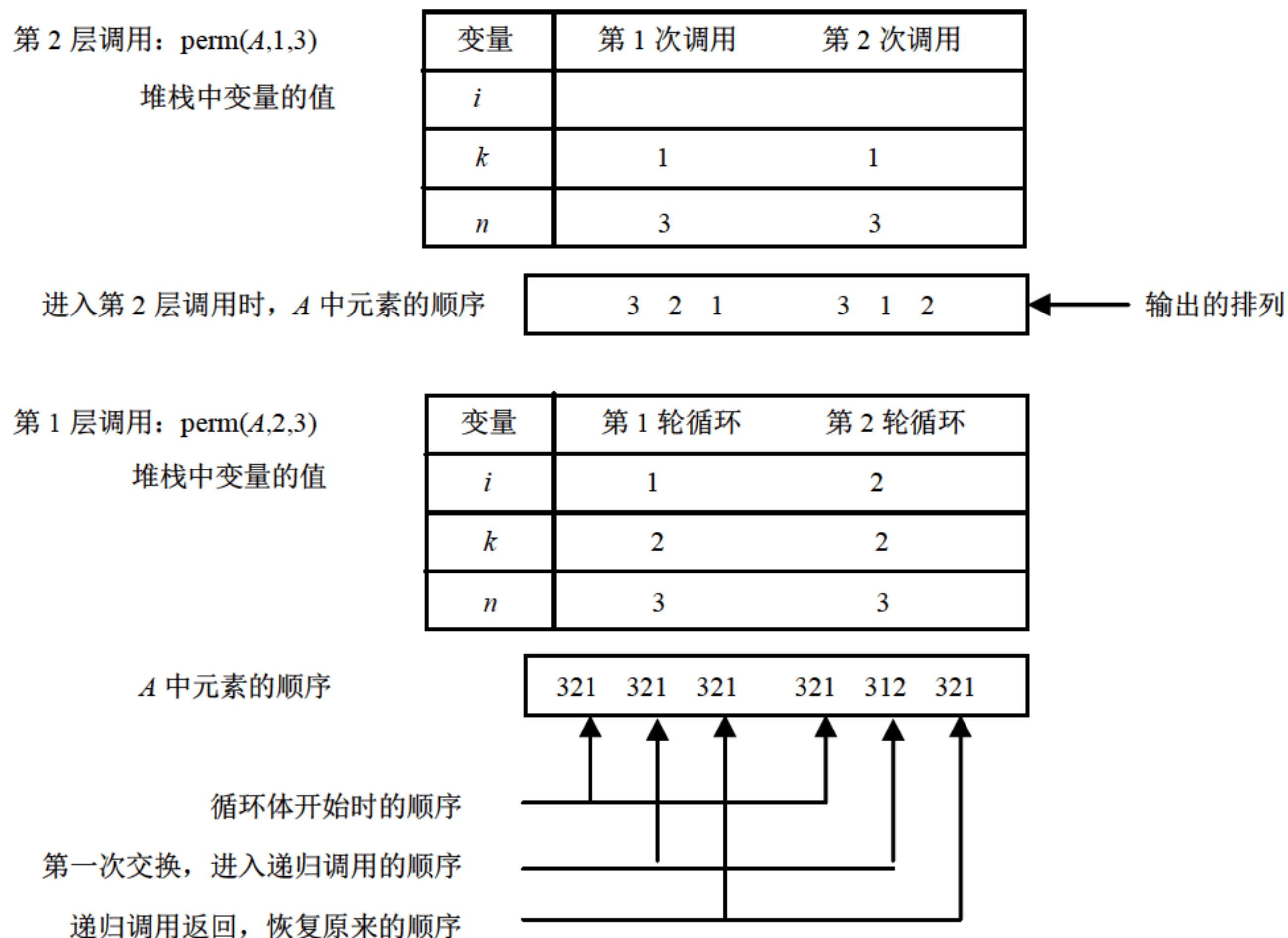
(c) 第3轮循环体的执行情况
