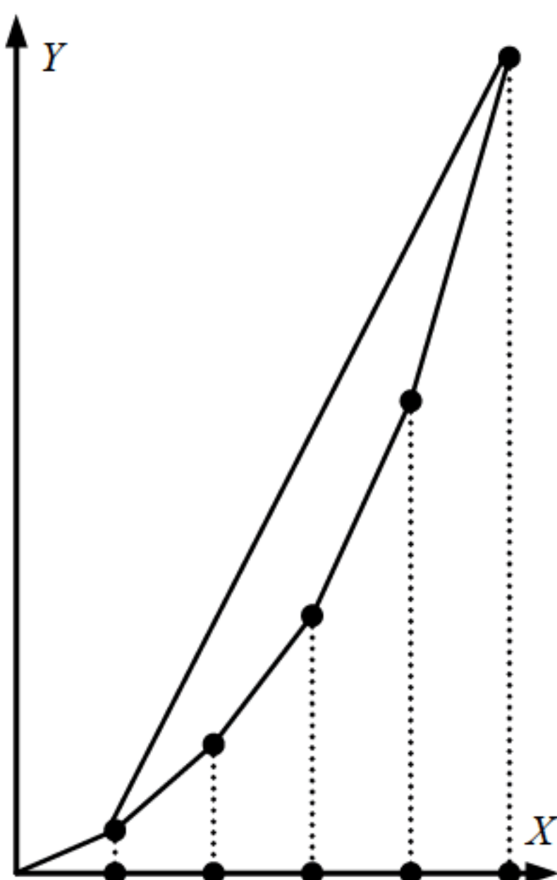
图 14.4 把排序问题归约为凸壳问题
