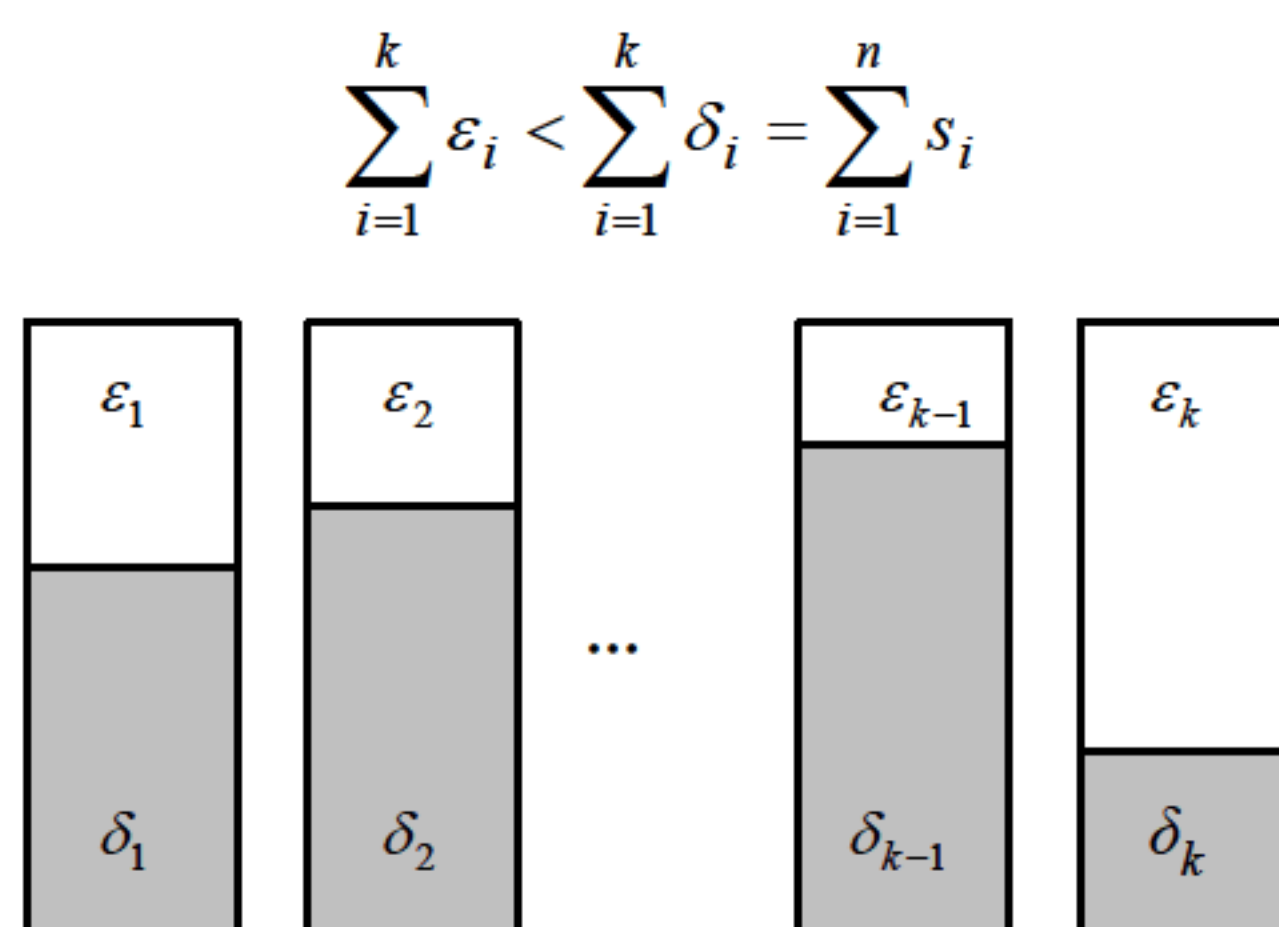
图 15.1 FF 算法的箱子装入情况
