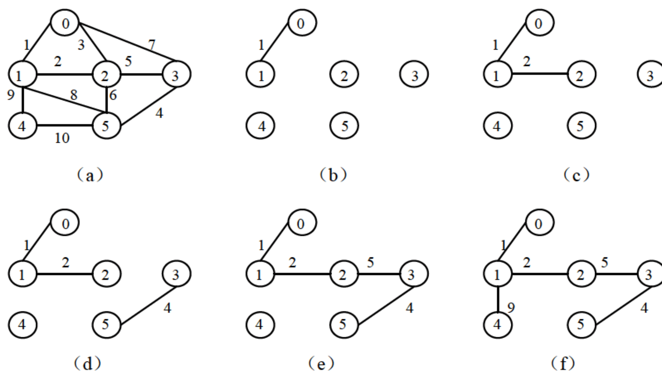
图 5.8 Kruskal 算法的执行过程
