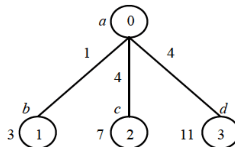
图 8.4 图 8.3 搜索树的第一层分支结点
