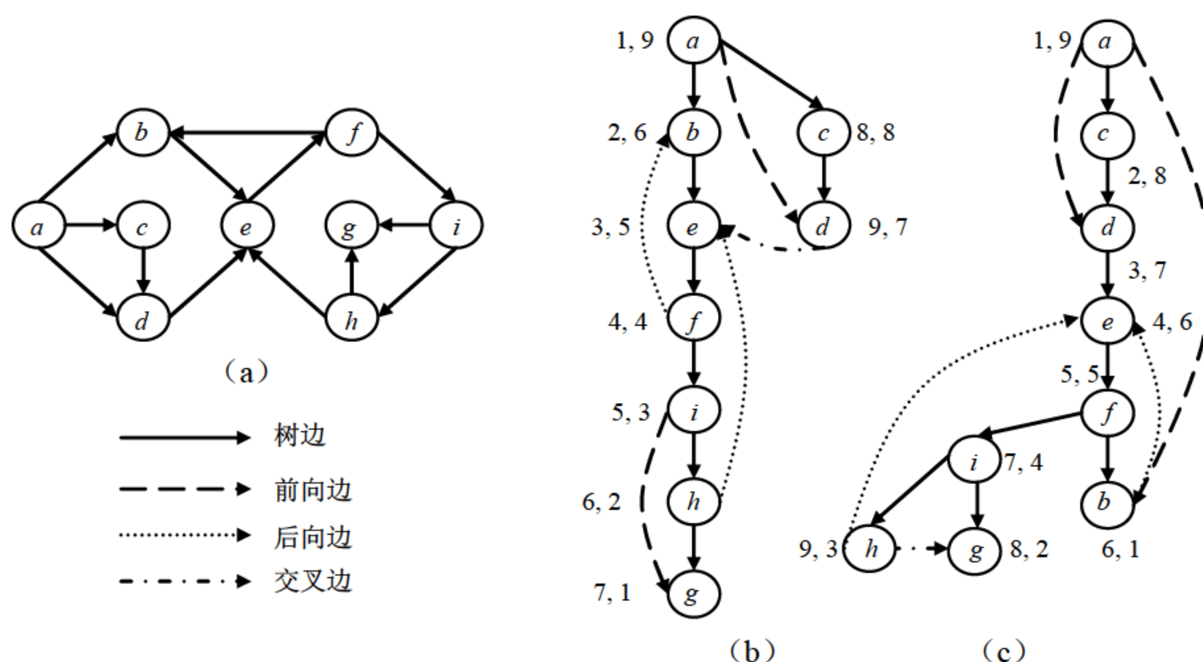
图 10.2 有向图的深度优先搜索遍历的例子
