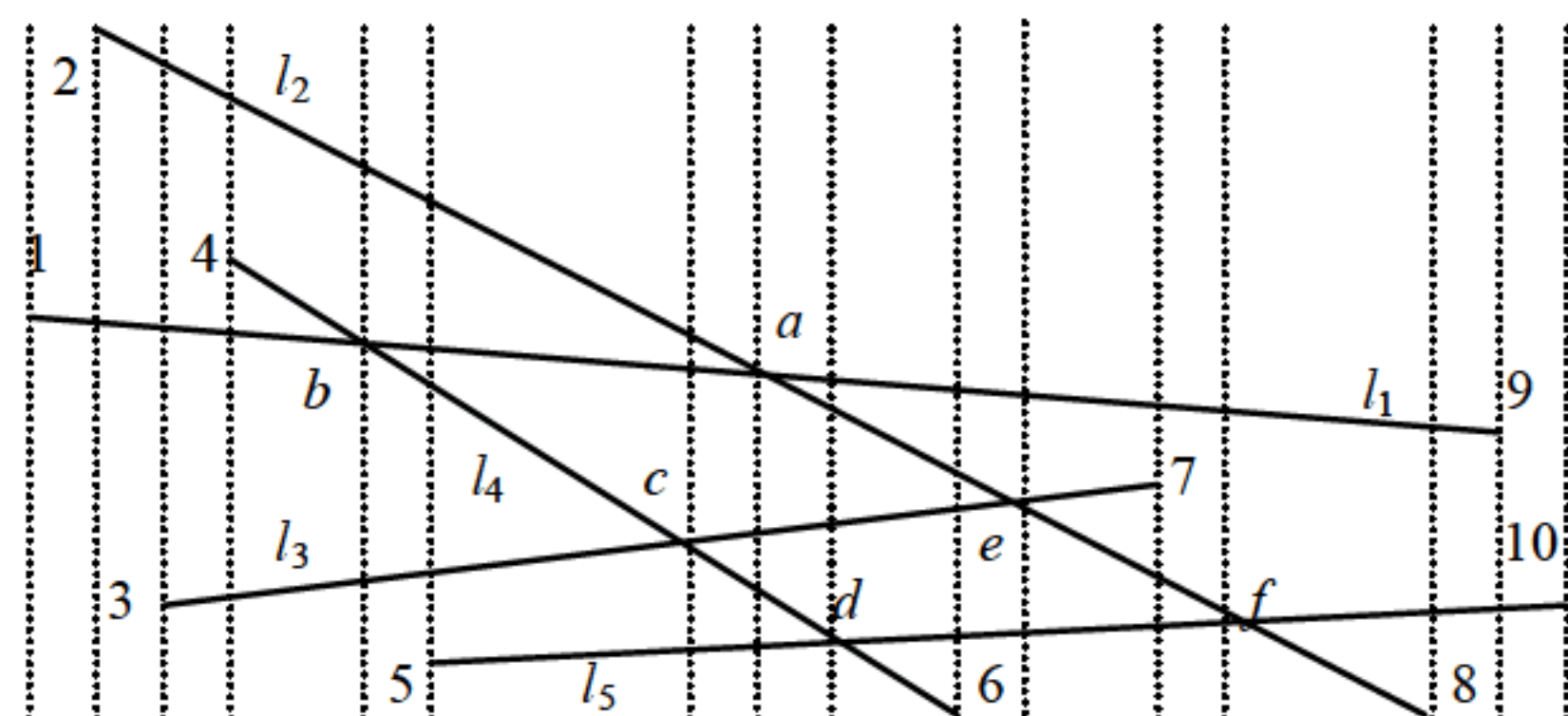
图 11.6 寻找线段交点的过程
