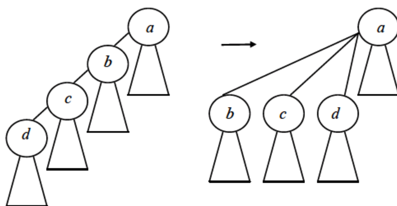
图 3.9 路径压缩
