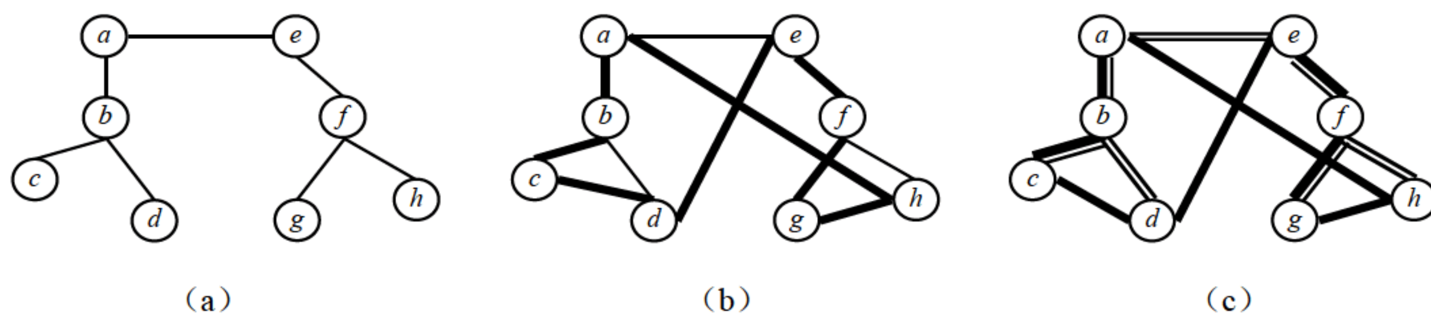
图 15.3 最小生成树探索算法的执行过程和近似比率的说明
