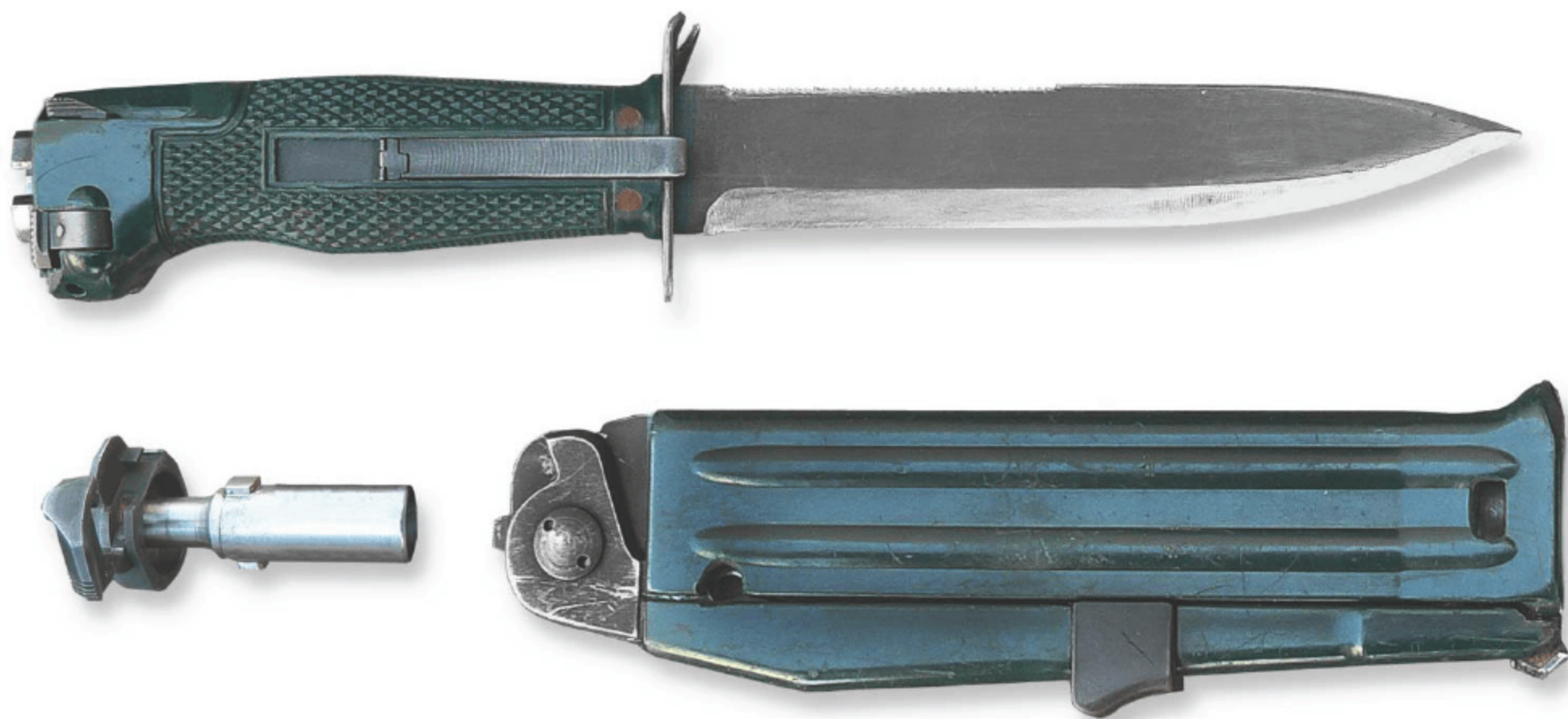
NRS-2 侦察匕首
