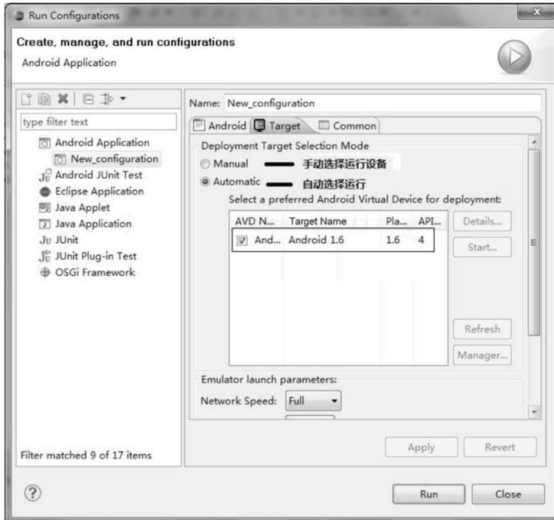
图 2-9 Run 配置—运行设备设置页面
