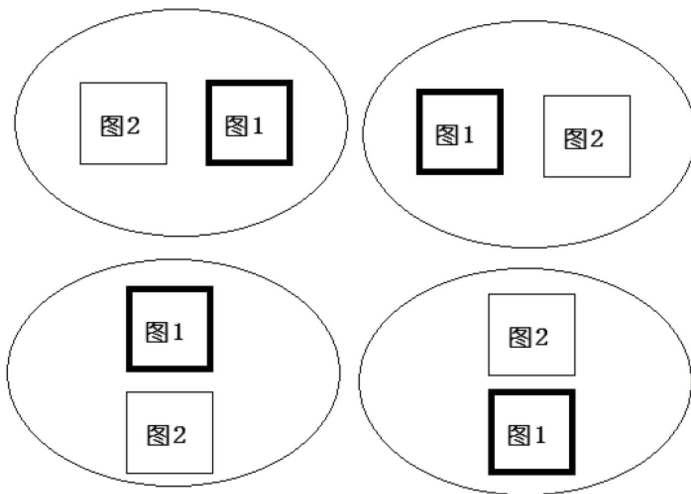
图 4-47 矩形不发生碰撞的四种情况
