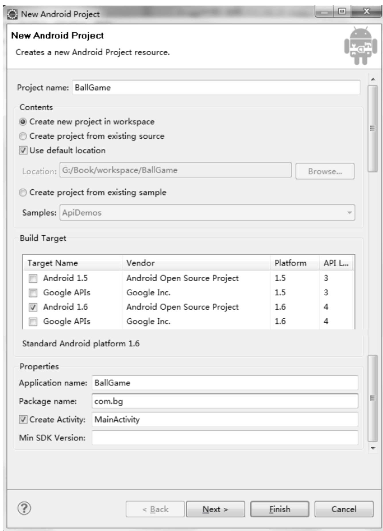
图 8-5 新建项目“BallGame”
