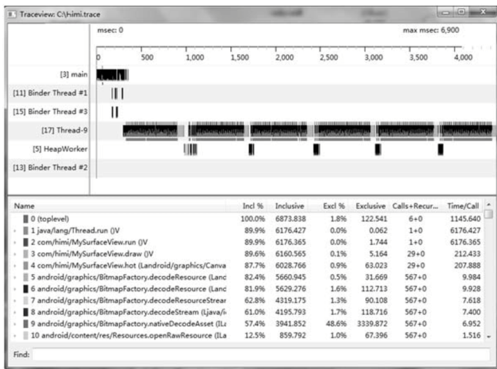
图 6-14 TraceView 效率检视工具
