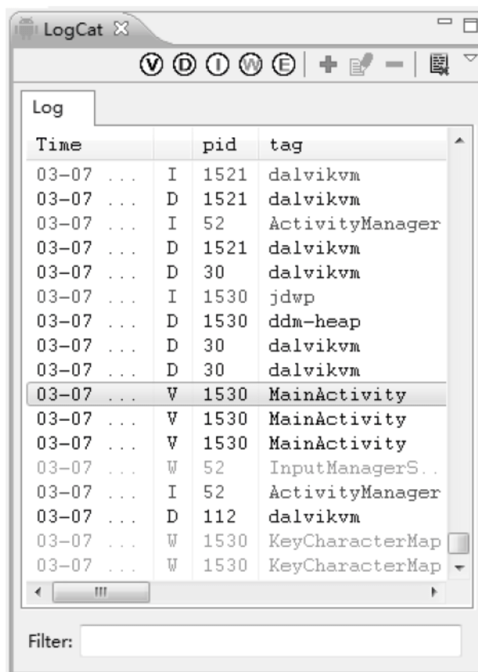
图 2-38 LogCat 视图
