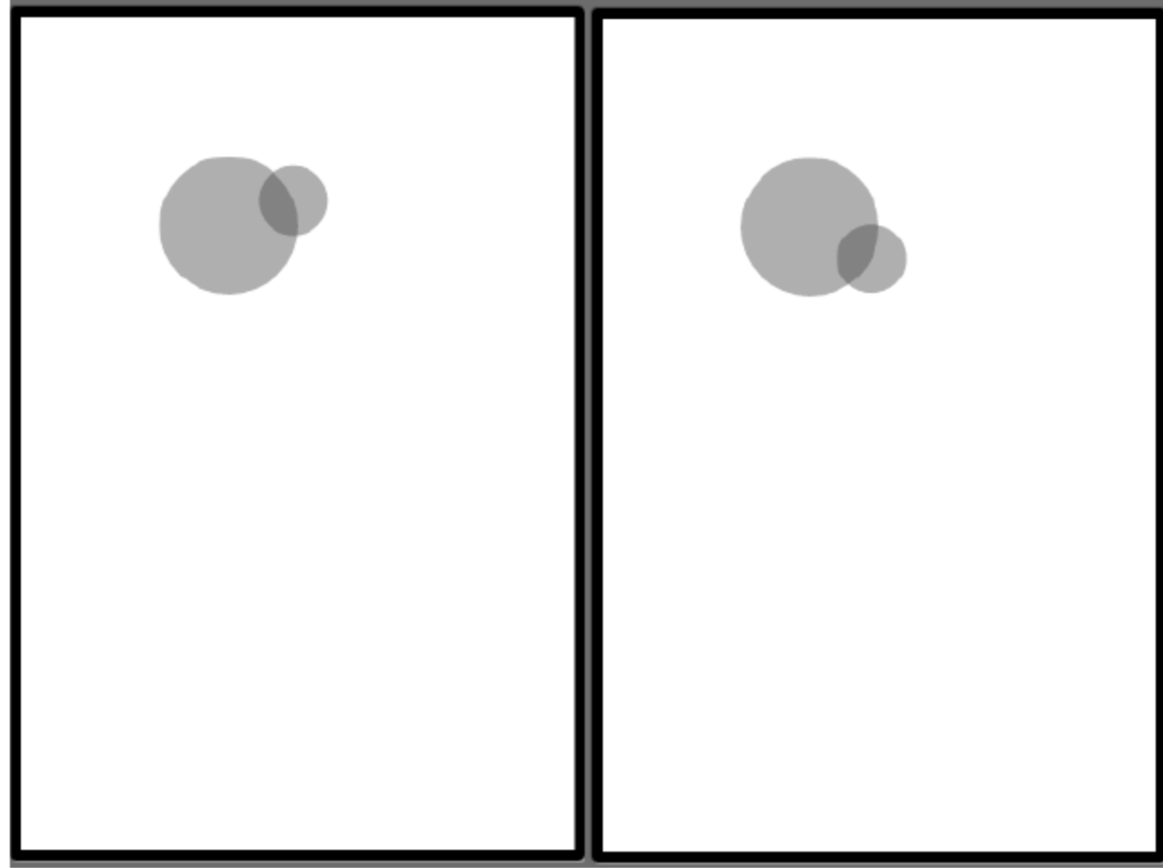
图 6-2 圆周运动
