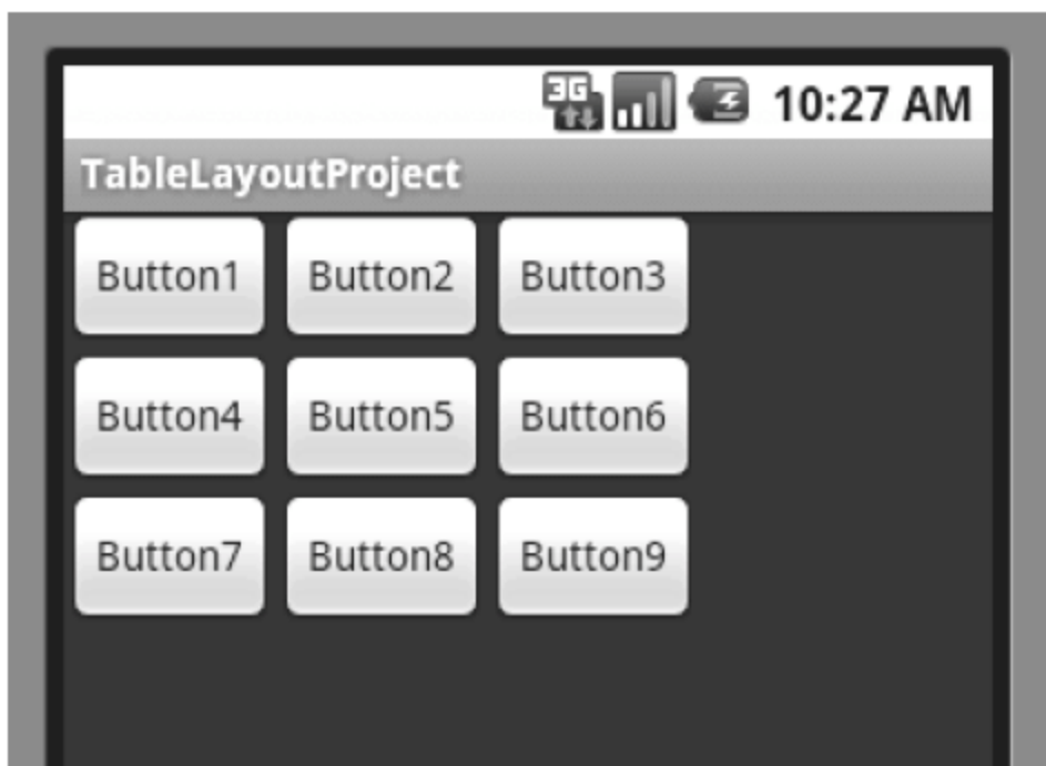
图 3-12 android:shrinkColumns="2"的布局
