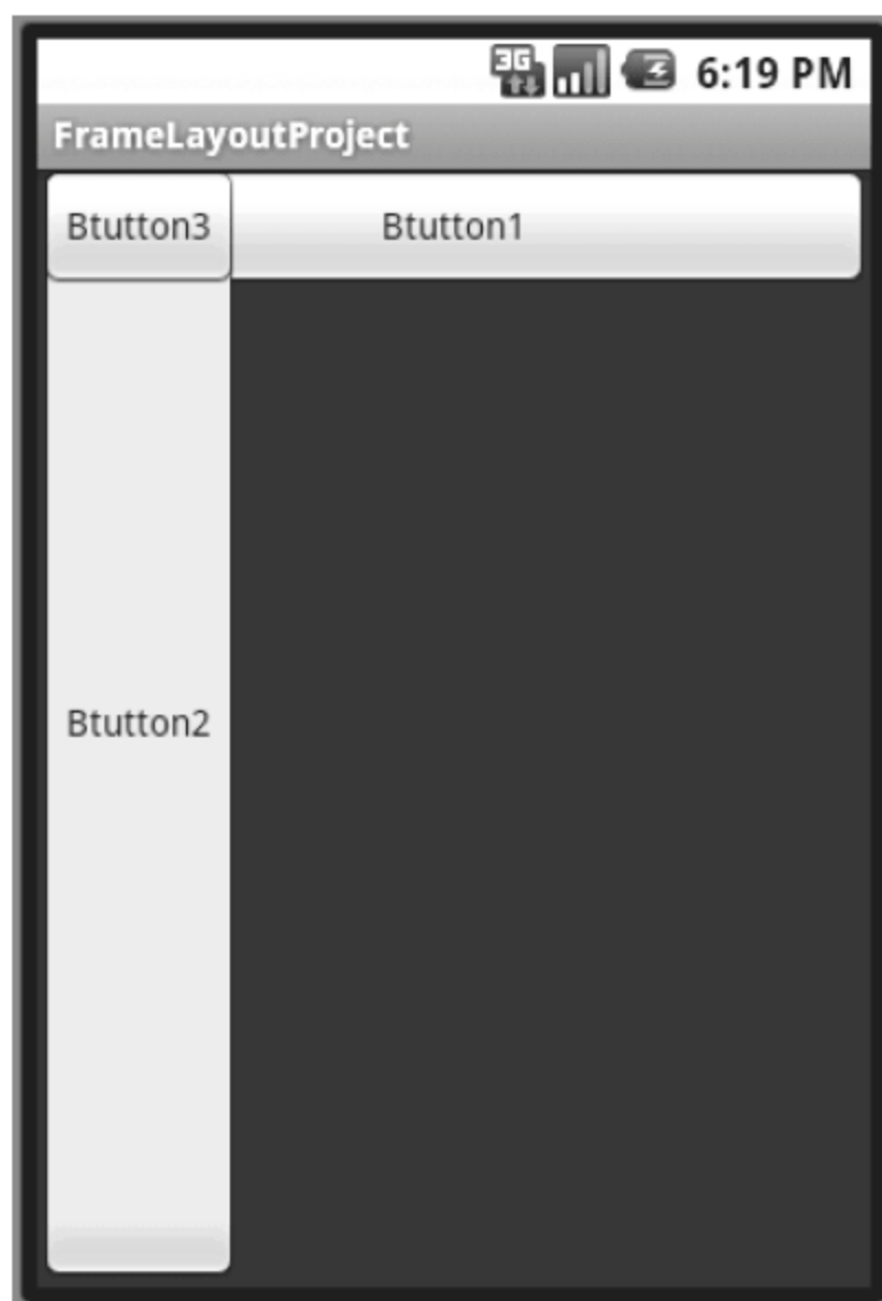
图 3-20 单帧布局
