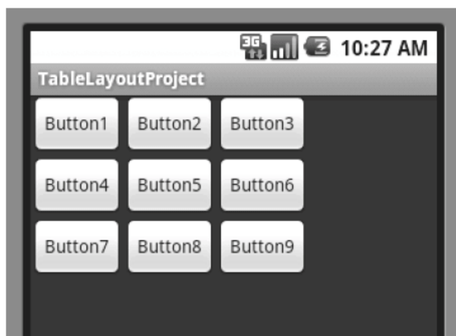
图 3-11 表格布局
