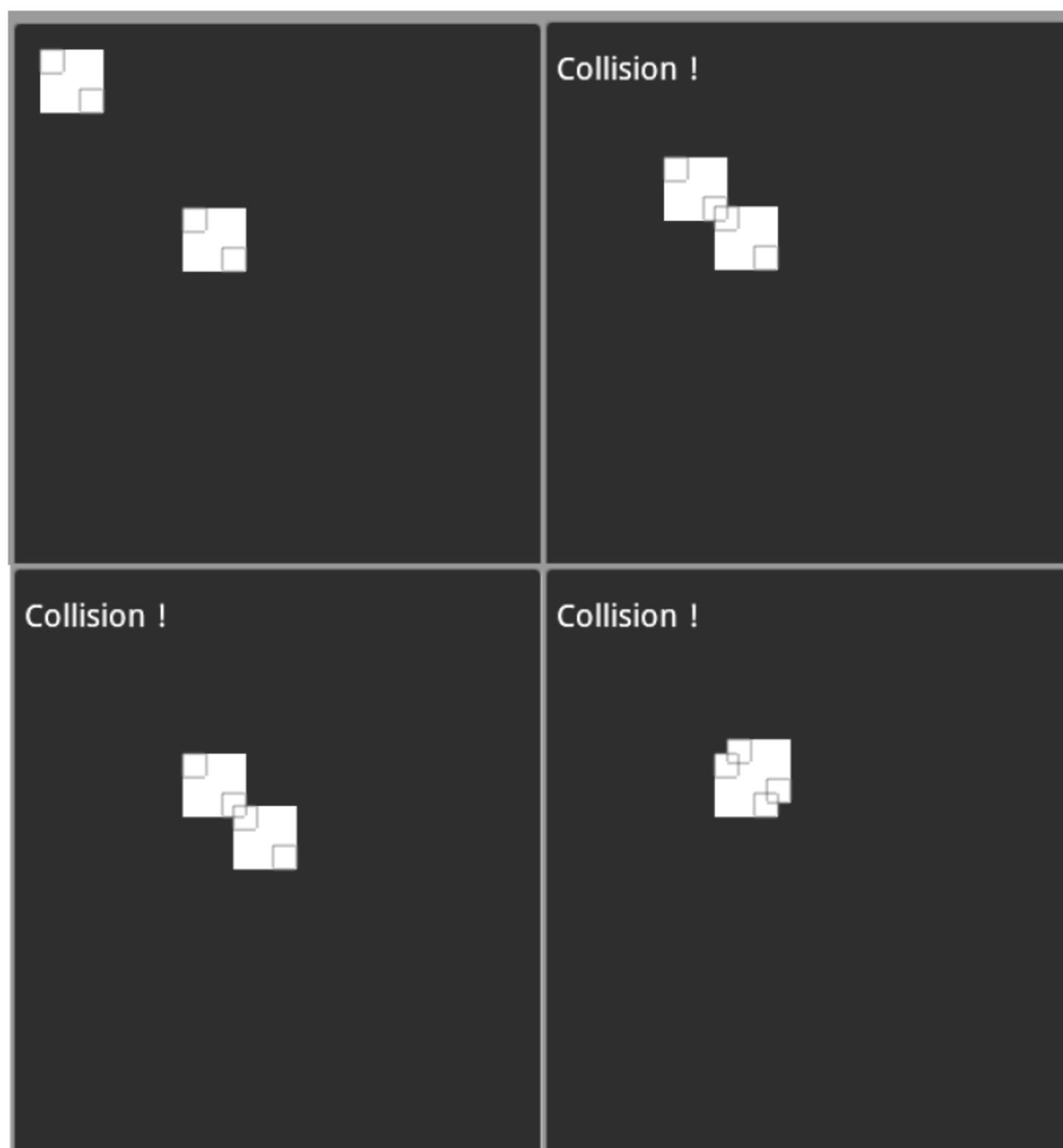
图 4-53 多矩形碰撞
