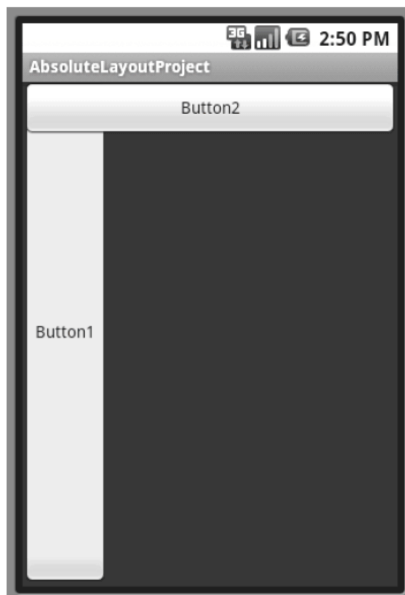
图 3-18 绝对布局
