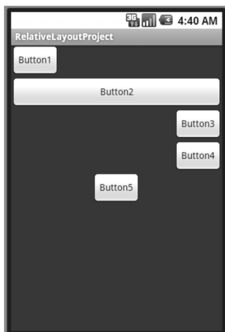
图 3-8 相对布局
