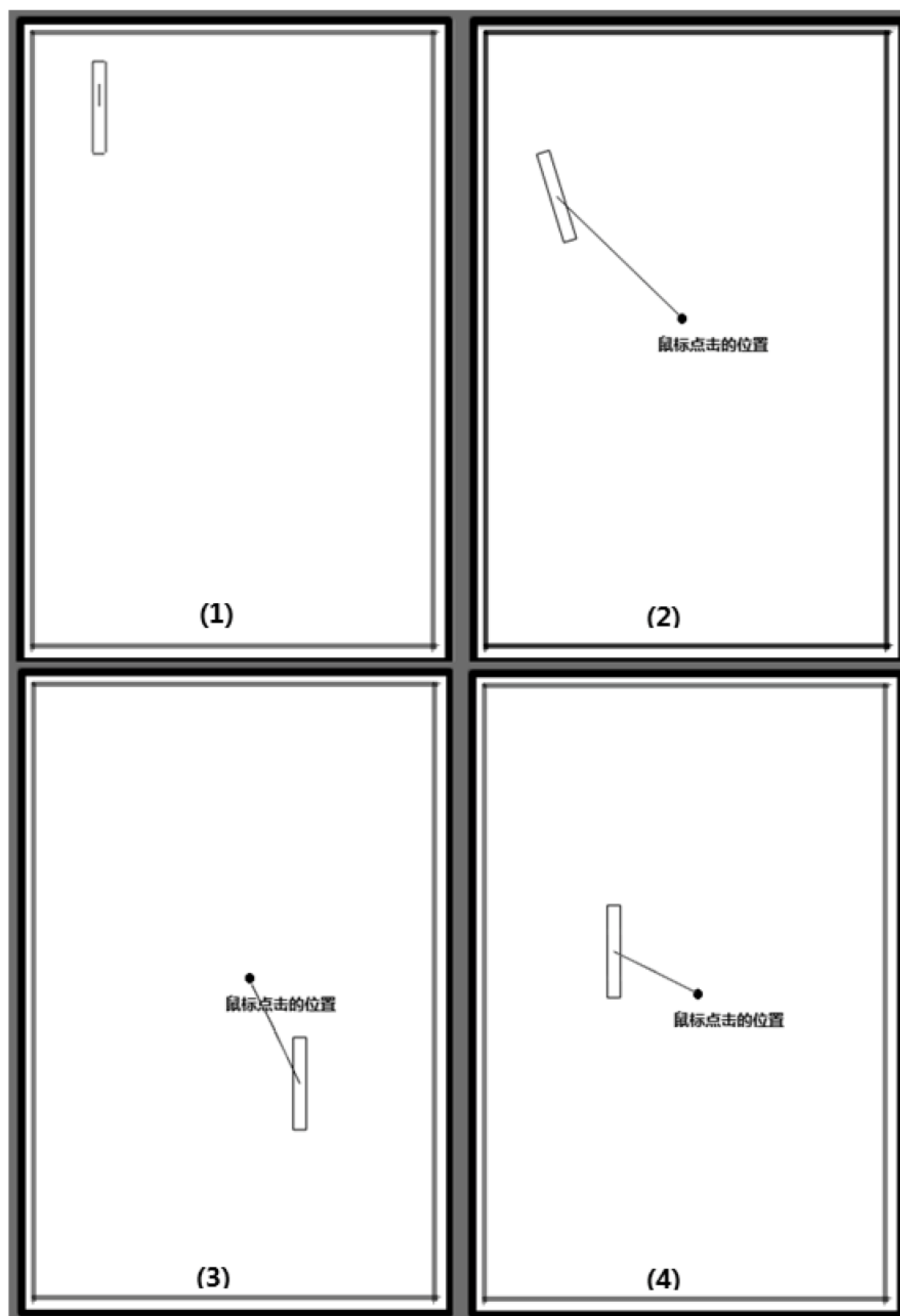
图 7-23 鼠标关节
