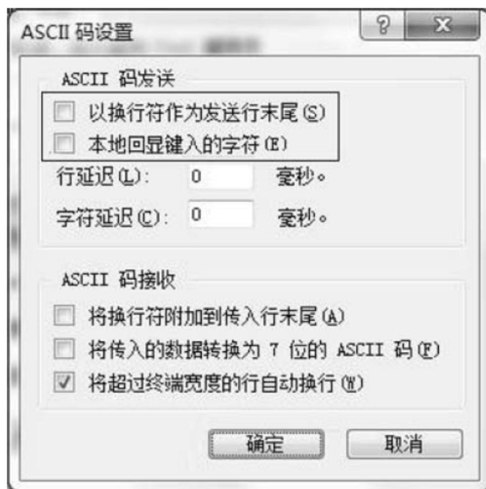
图 6-22 配置截图 7
