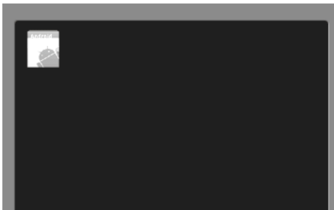
图 4-14 绘制位图
