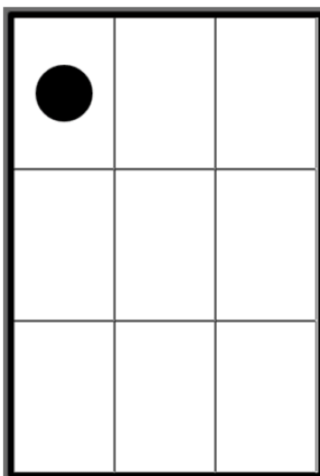
图 4-59 项目截图
