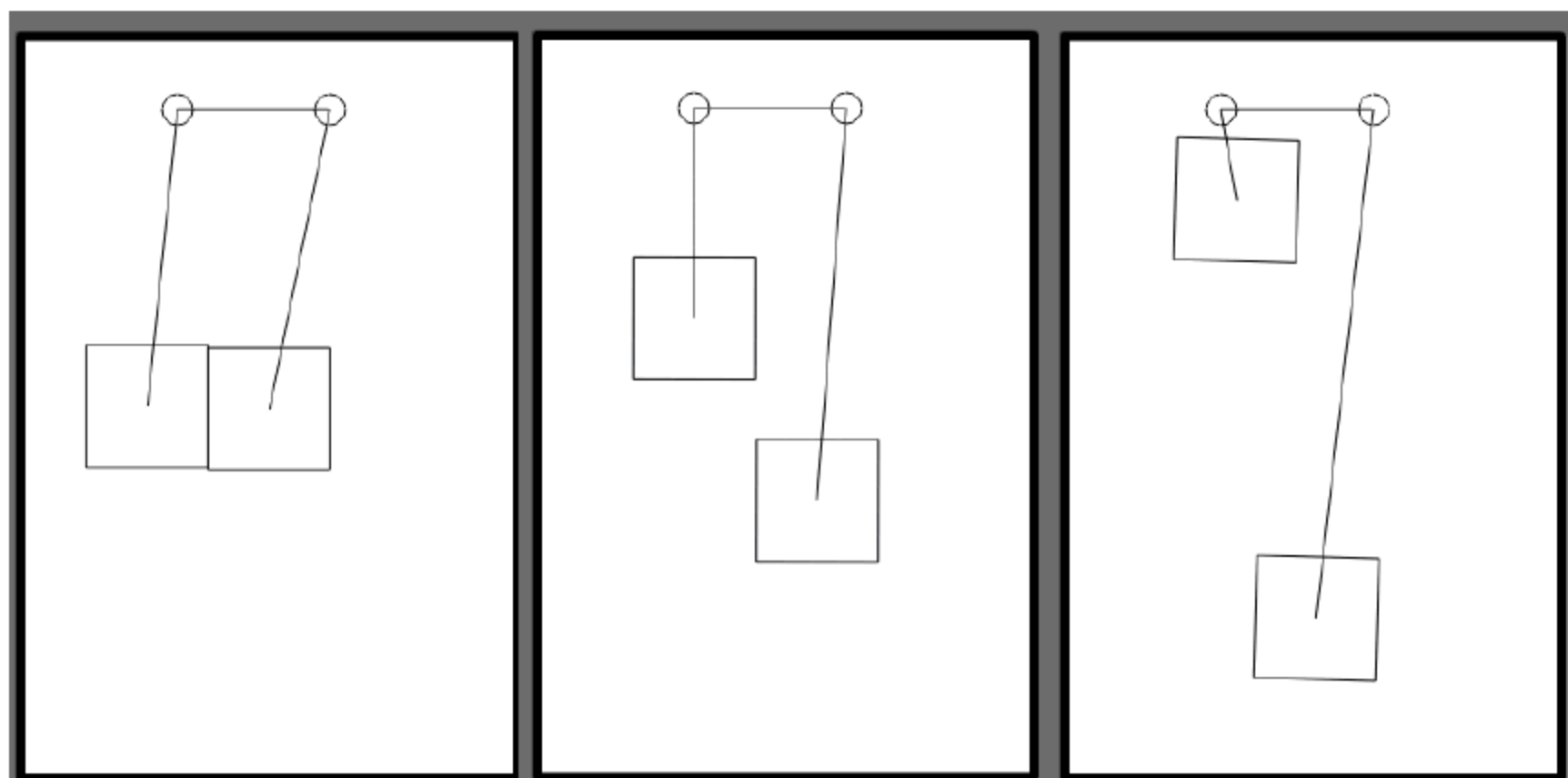
图 7-18 滑轮关节
