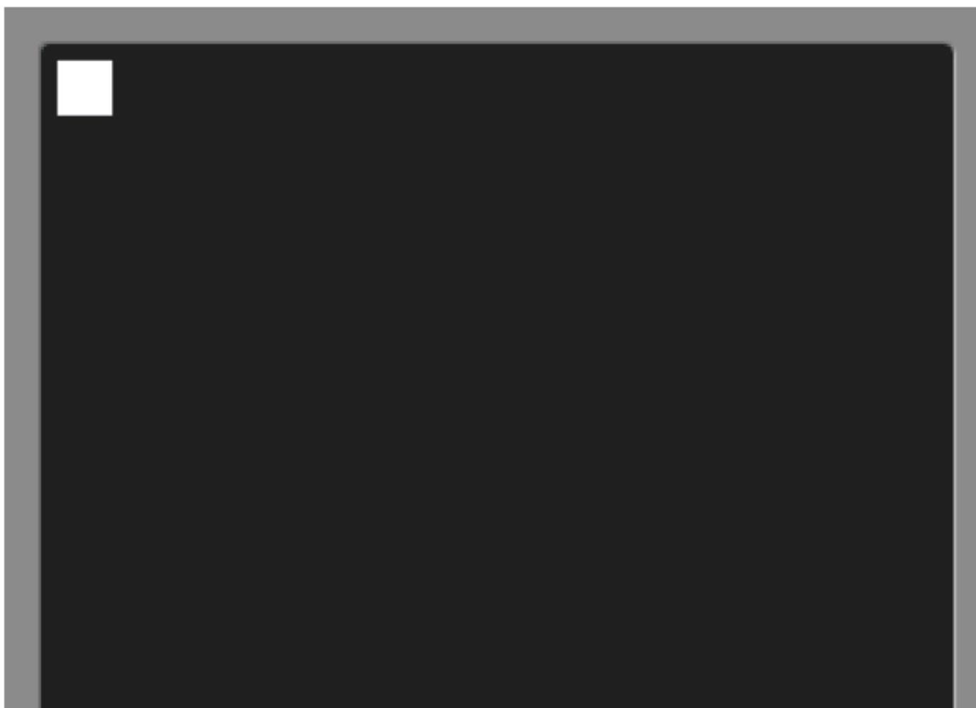
图 4-24 剪切区域
