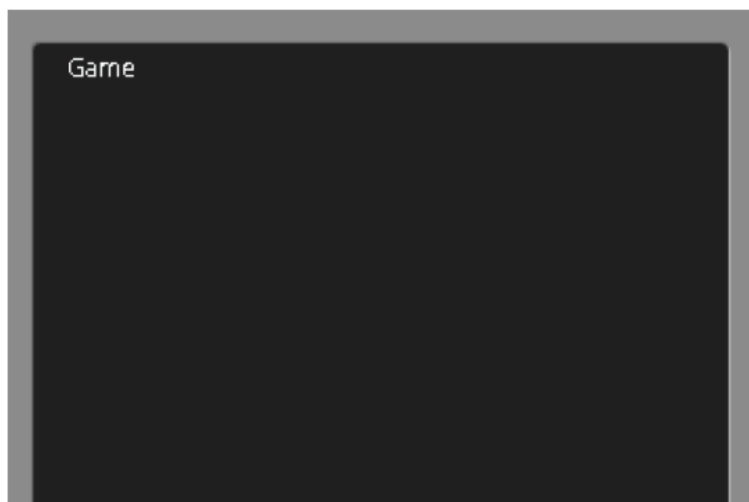
图 4-9 SurfaceView 视图
