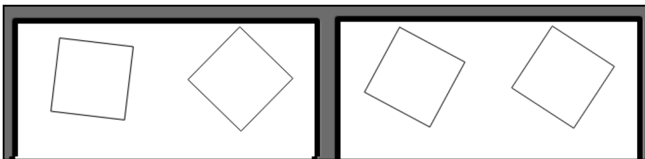
图 7-17 齿轮关节
