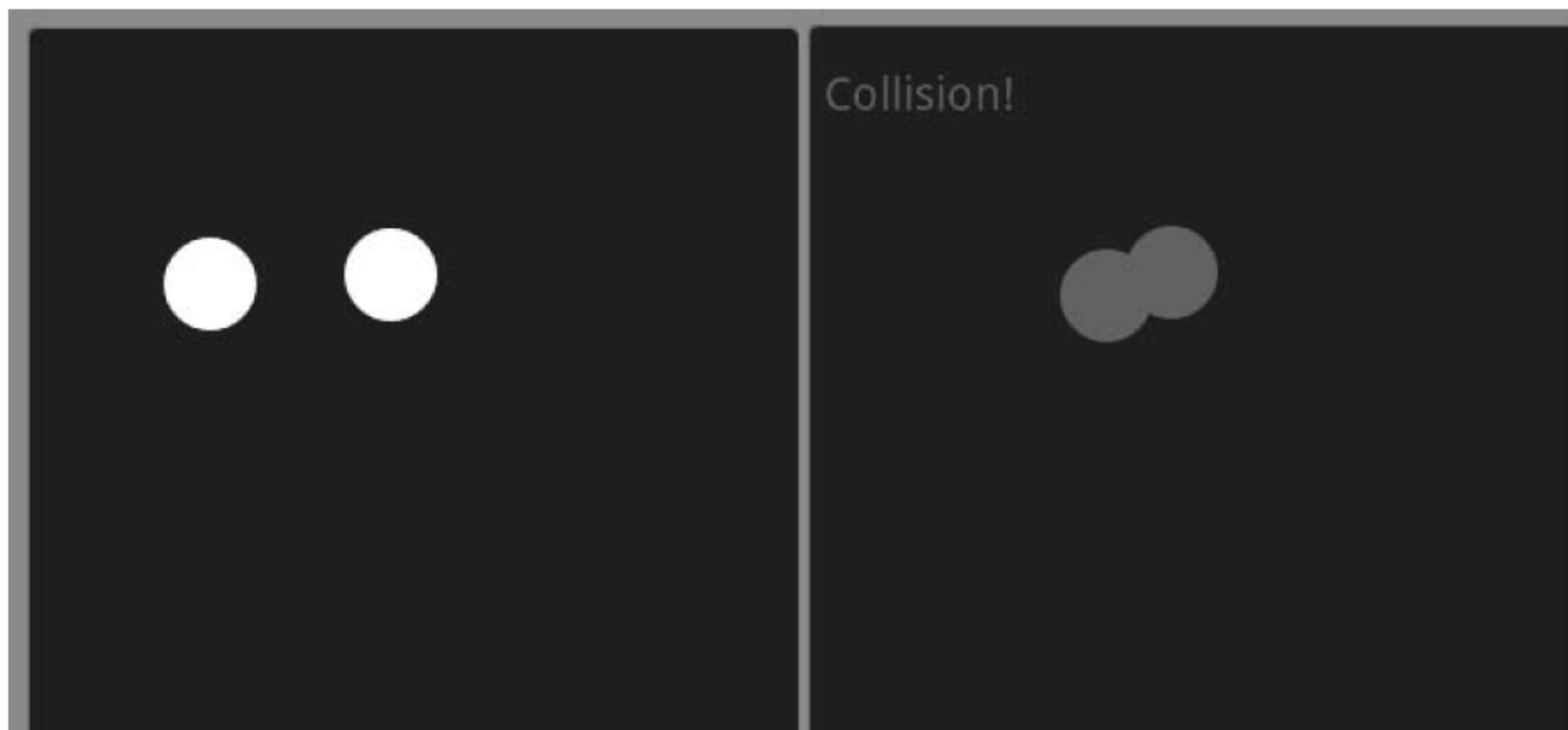
图 4-49 圆形碰撞
