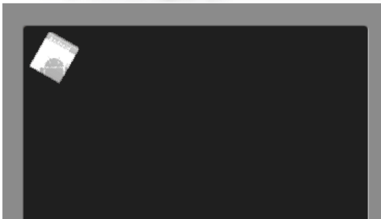
图 4-15 旋转画布
