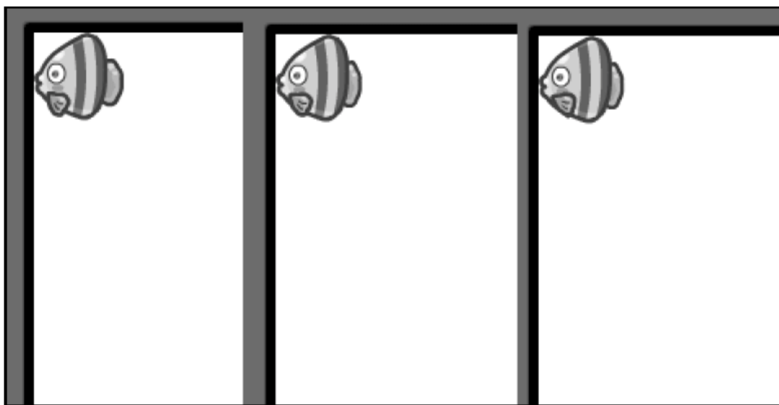
图 4-38 帧动画
