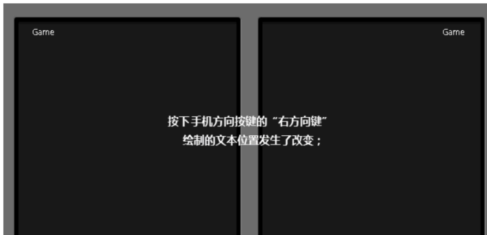
图 4-7 按键监听
