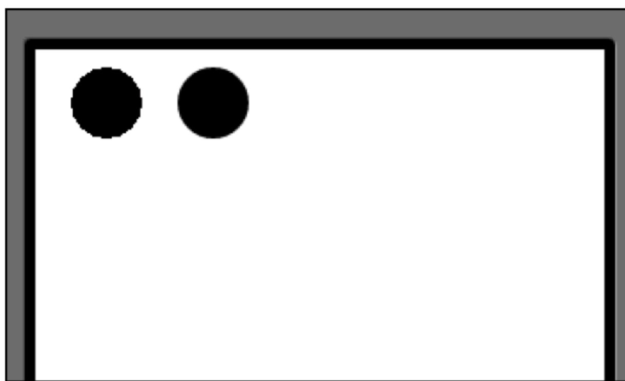
图 4-12 画笔无锯齿
