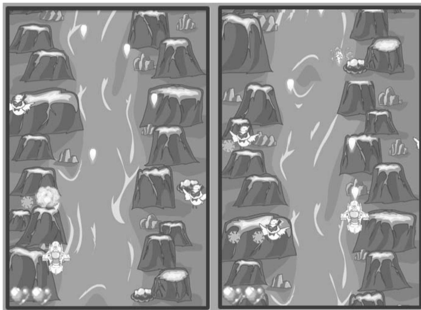
图 5-7 爆炸效果
