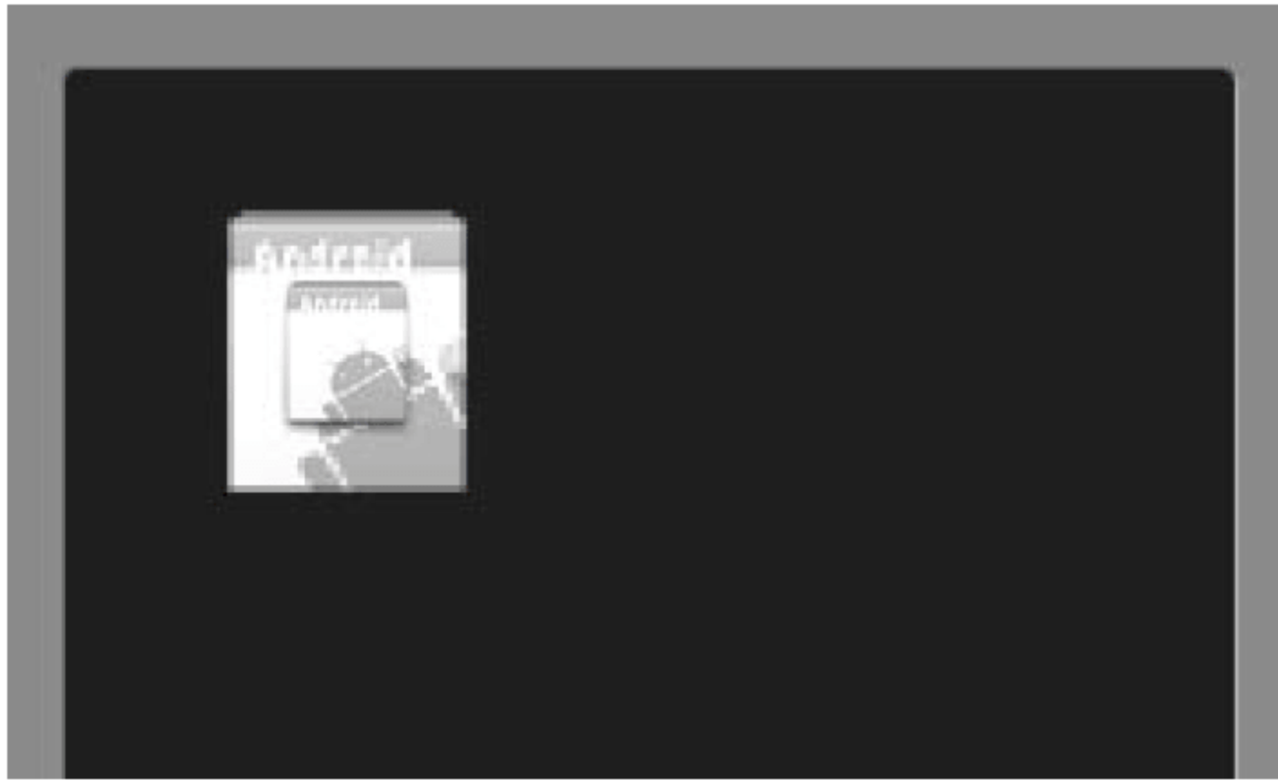
图 4-19 画布的缩放
