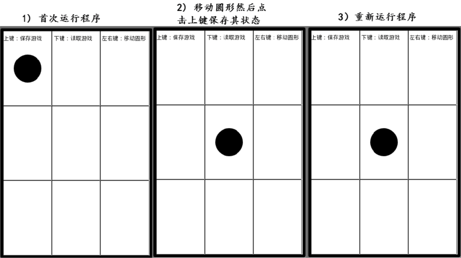
图 4-60 SharedPreferences 存储
