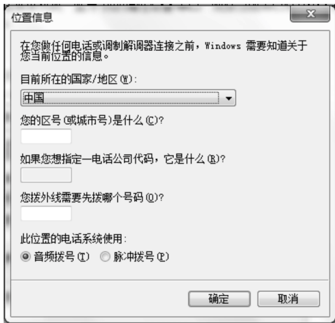
图 6-16 配置截图 1
