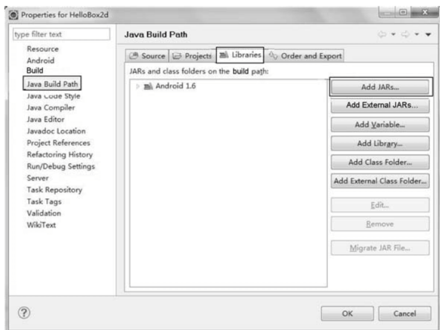
图 7-2 项目配置
