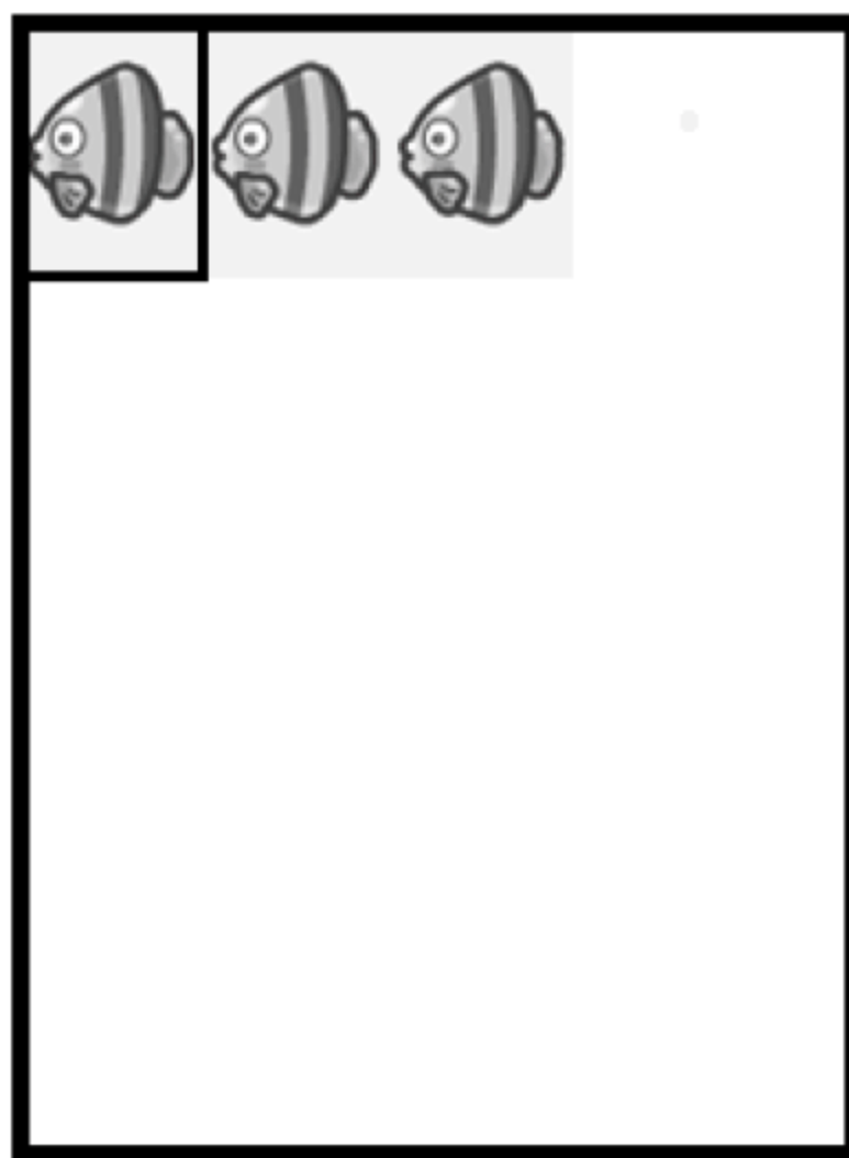
图 4-39 演示效果图 1
