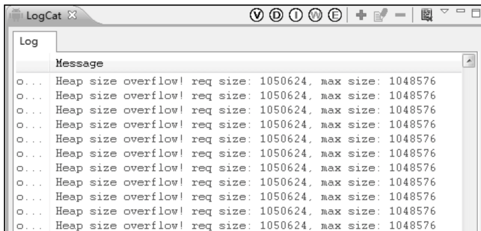
图 4-58 异常截图
