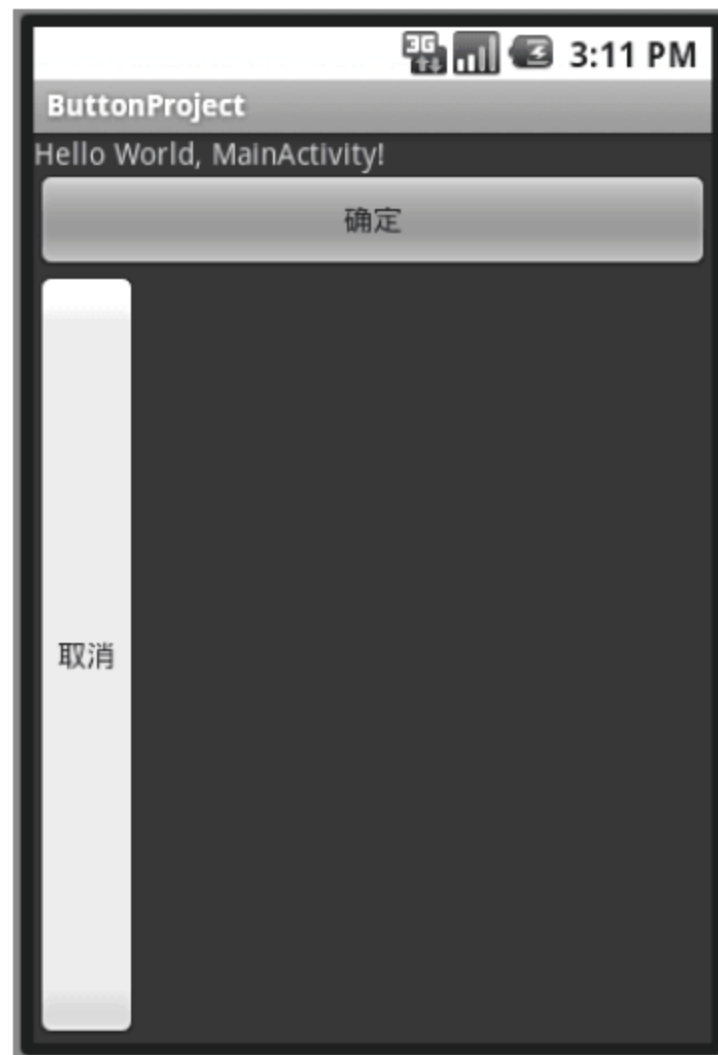
图 3-1 两个 Button
