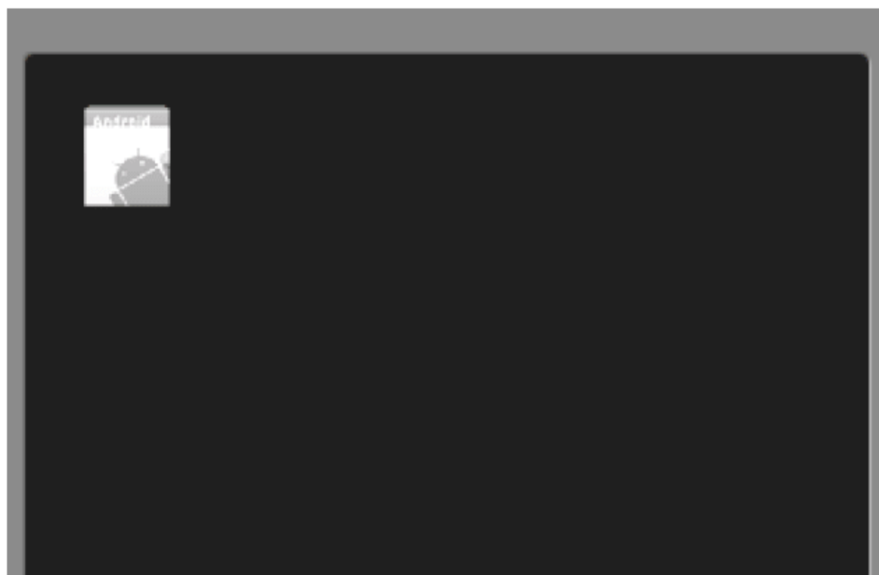
图 4-18 平移画布
