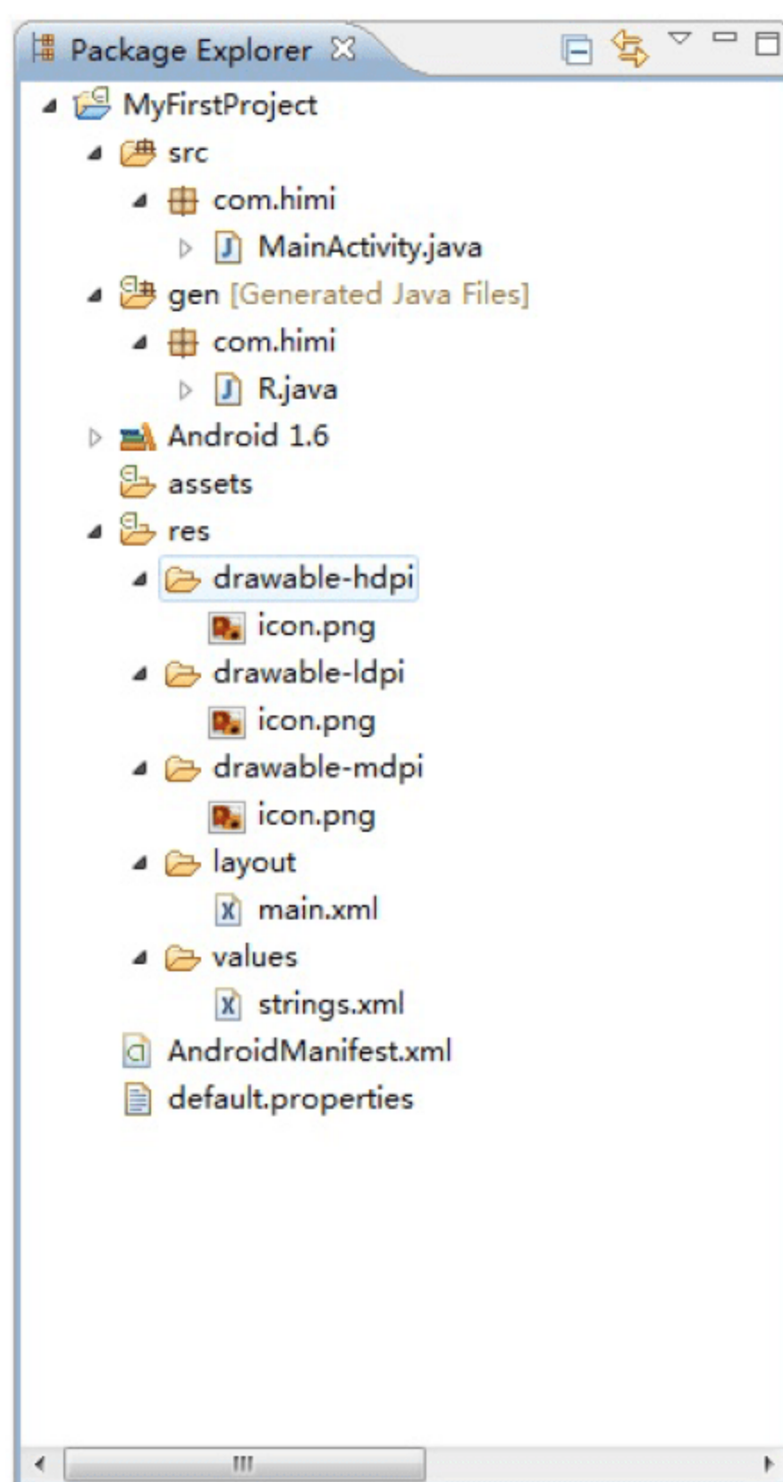
图 2-3 项目结构
