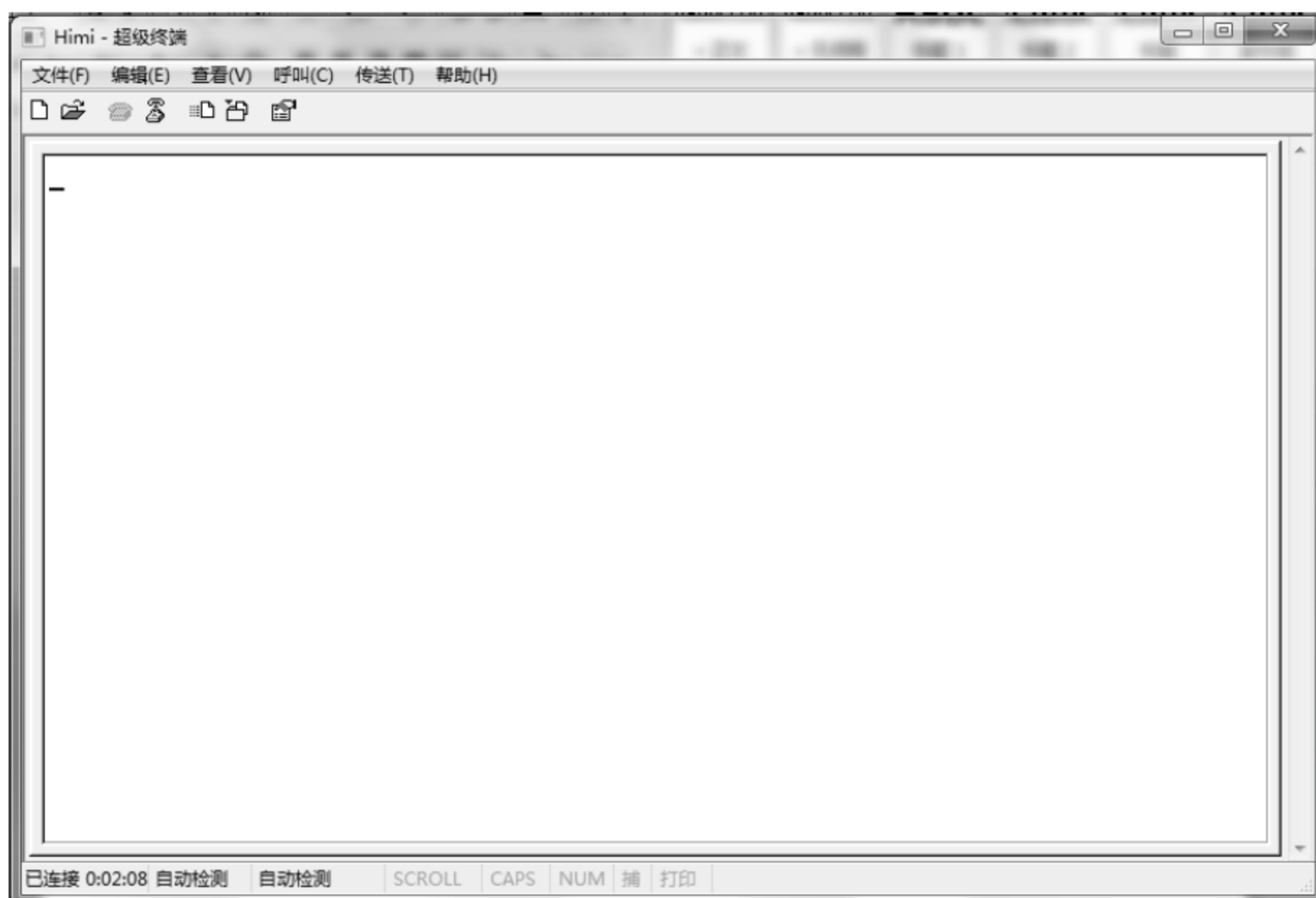
图 6-20 配置截图 5
