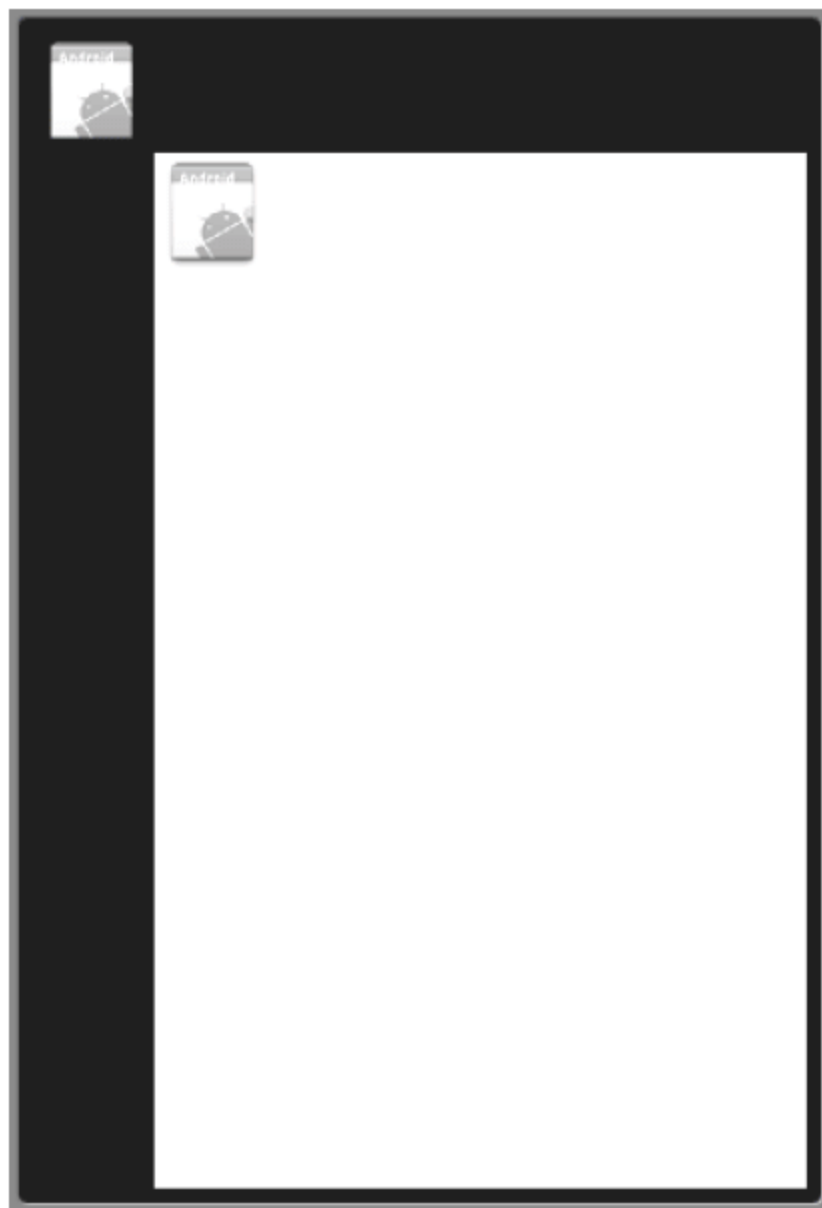
图 6-12 截屏效果图
