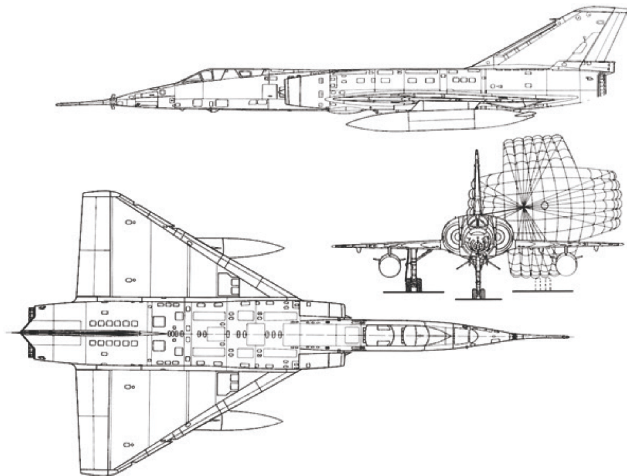
“幻影Ⅳ”轰炸机三视图
