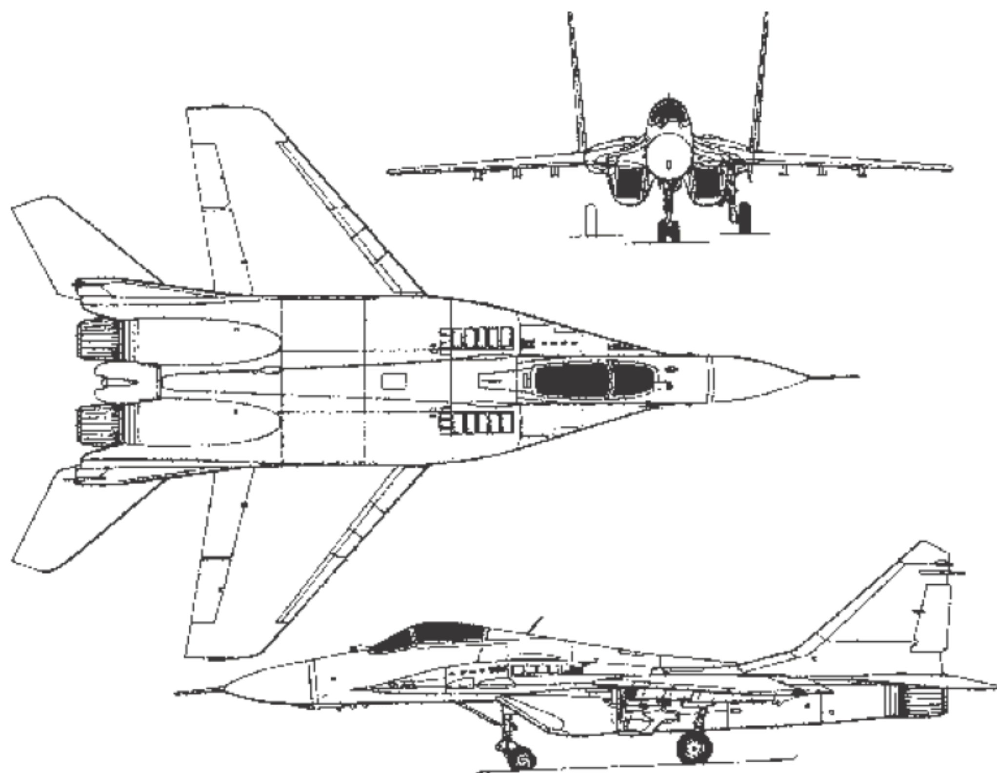
米格 -29 战斗机三视图
