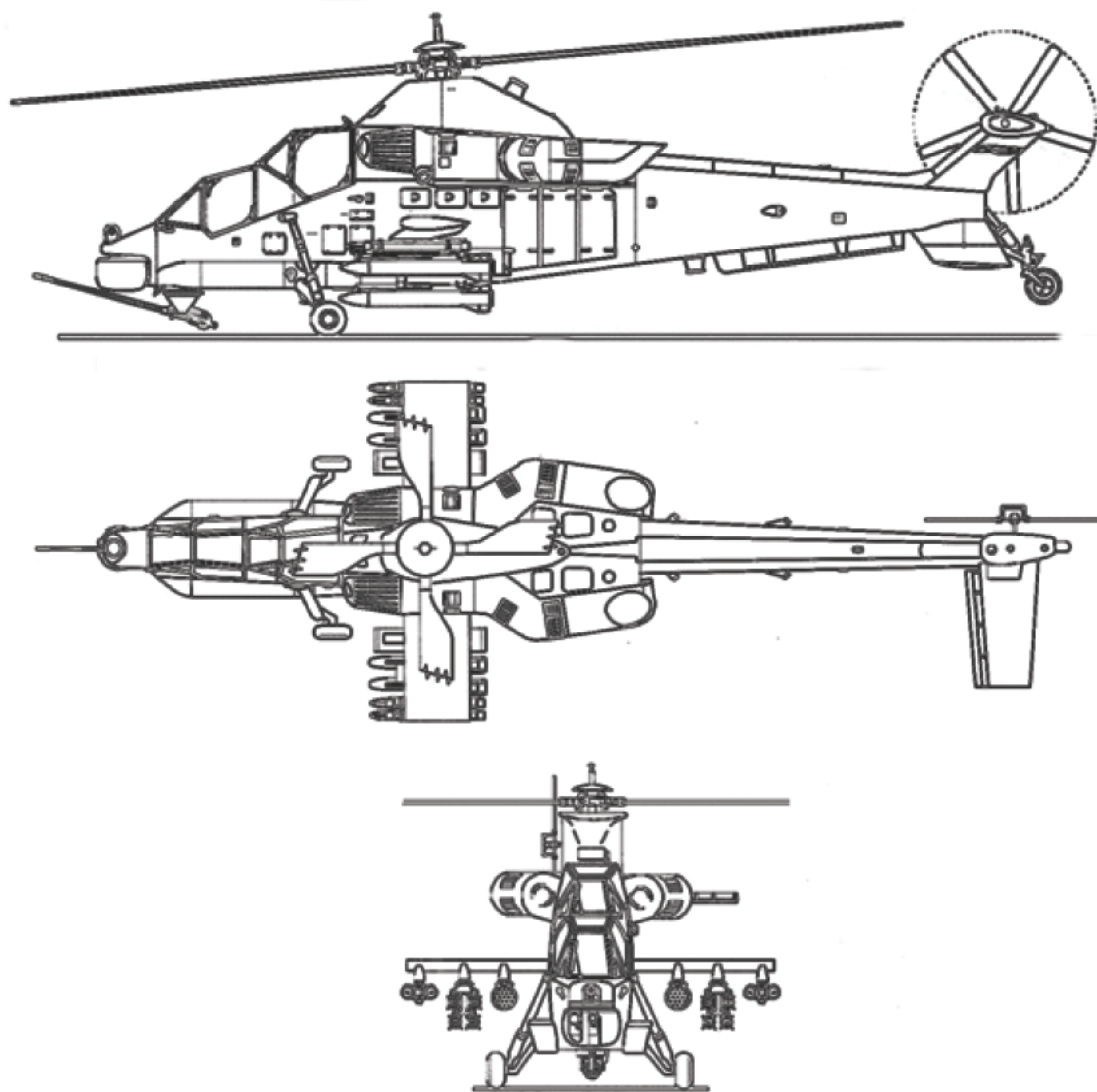
CSH-2 直升机三视图
