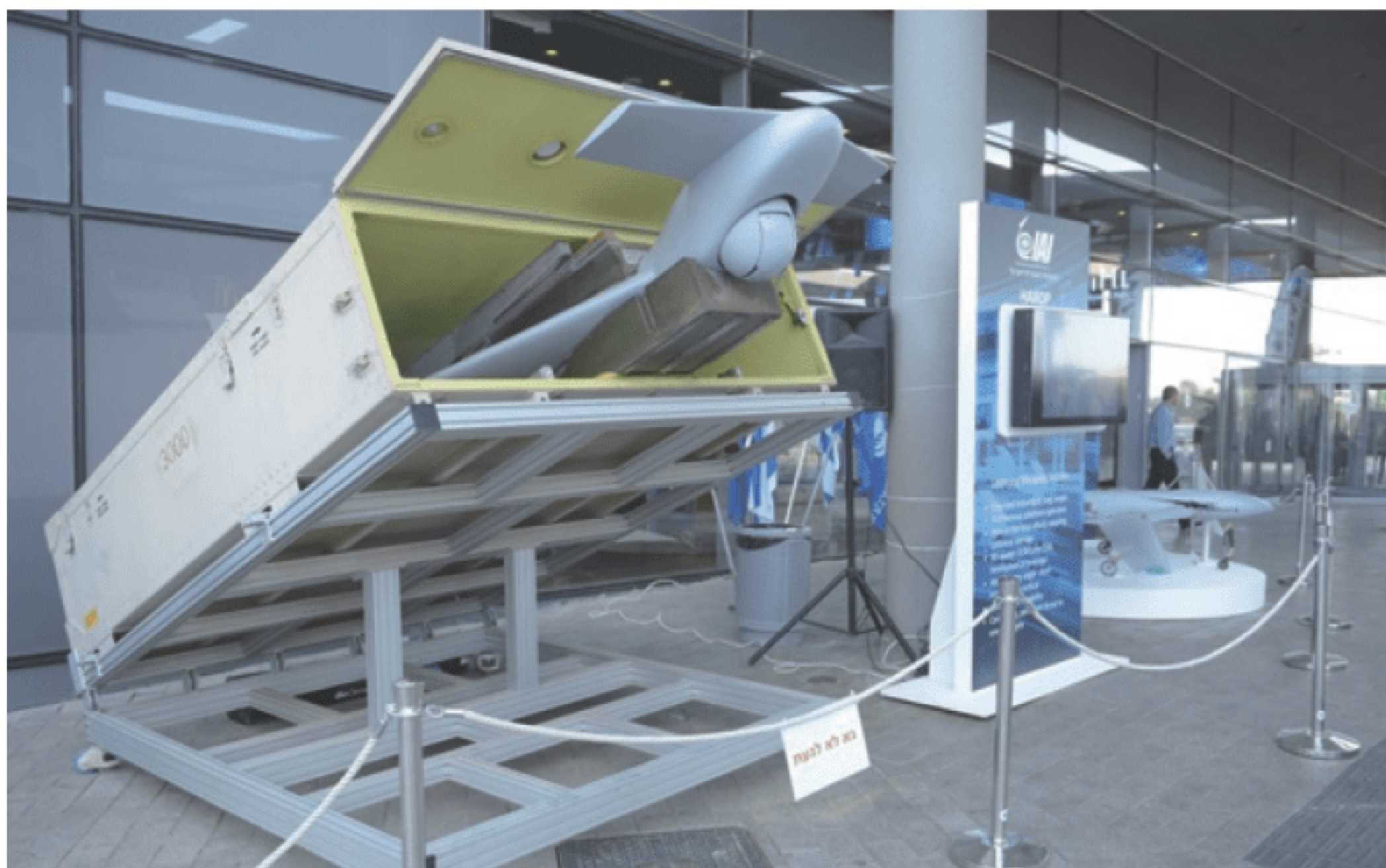
“哈洛普”无人机及发射装置
