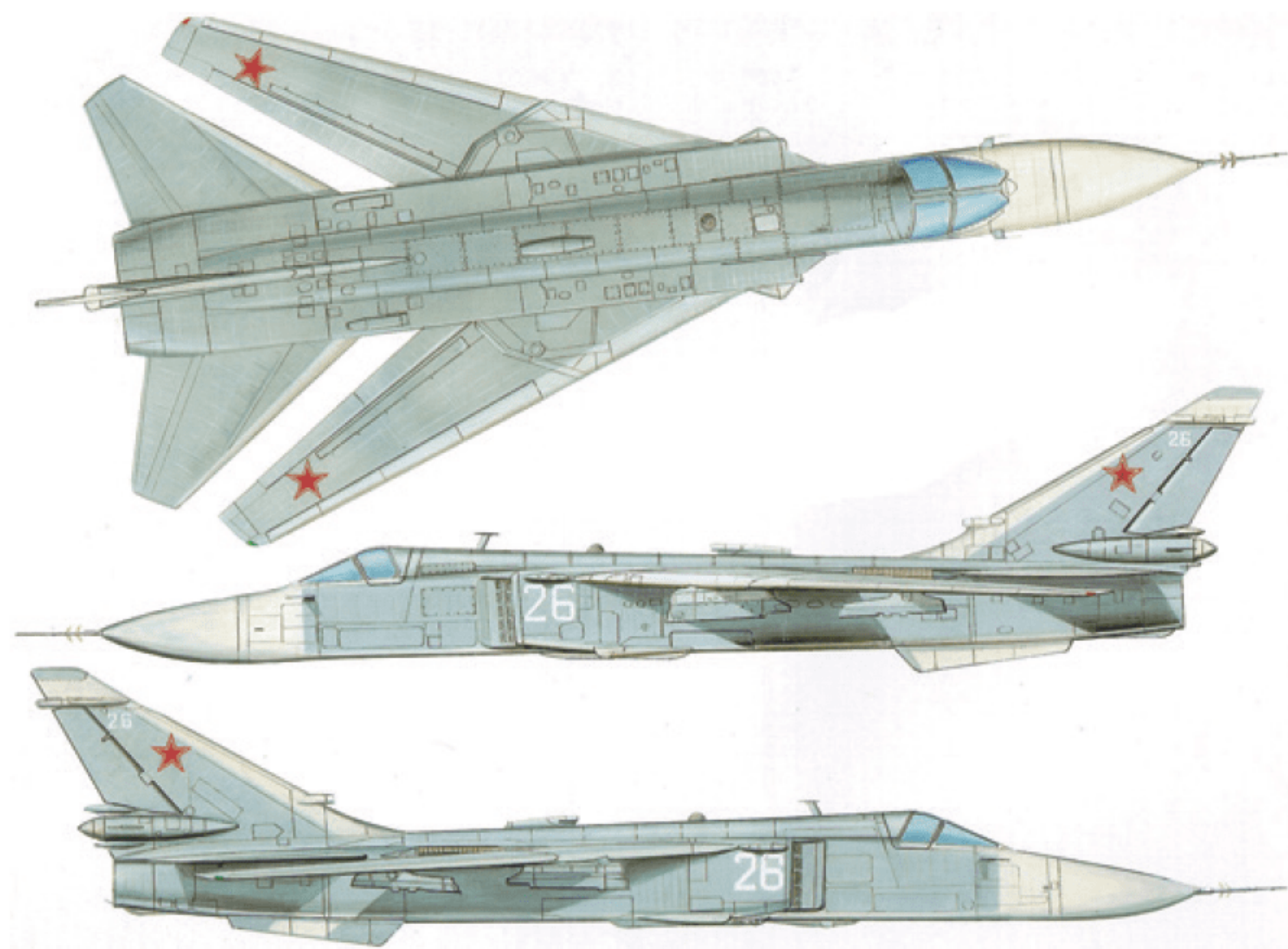
苏-24 战斗轰炸机三视图
