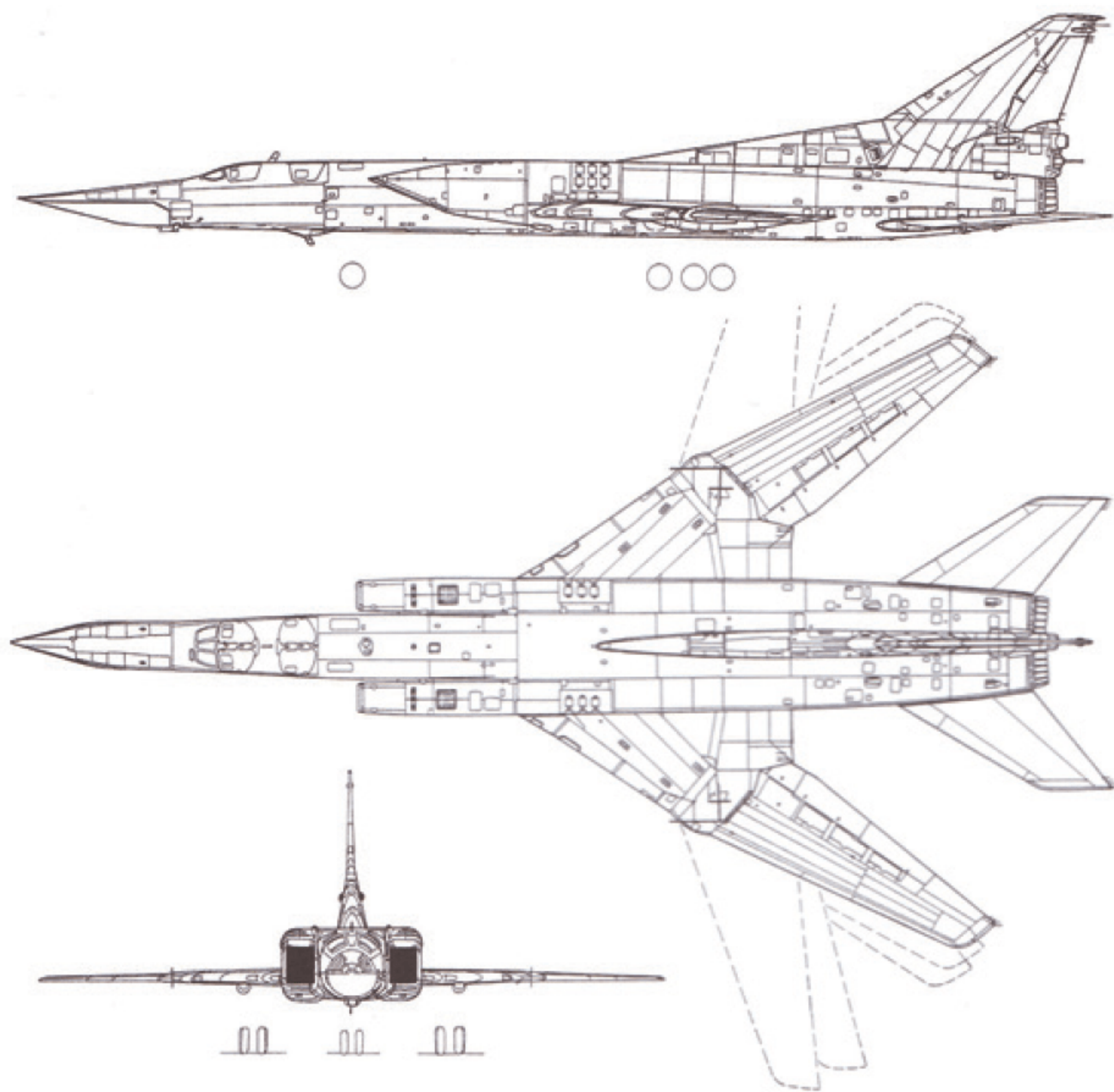
图 -22M 轰炸机三视图
