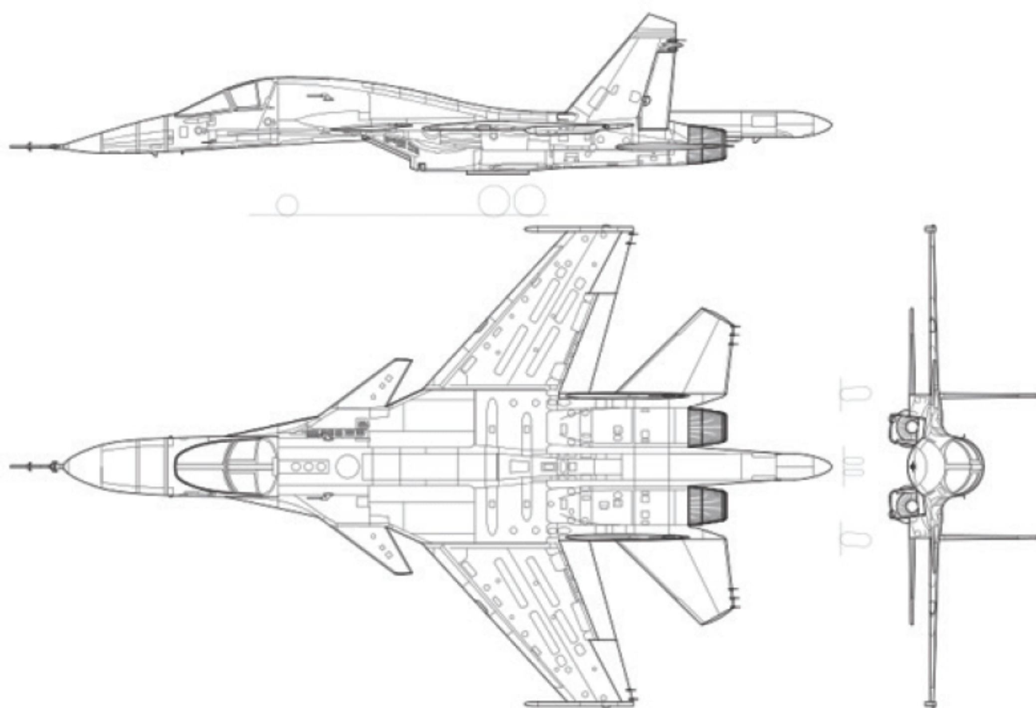
苏-34 战斗轰炸机三视图
