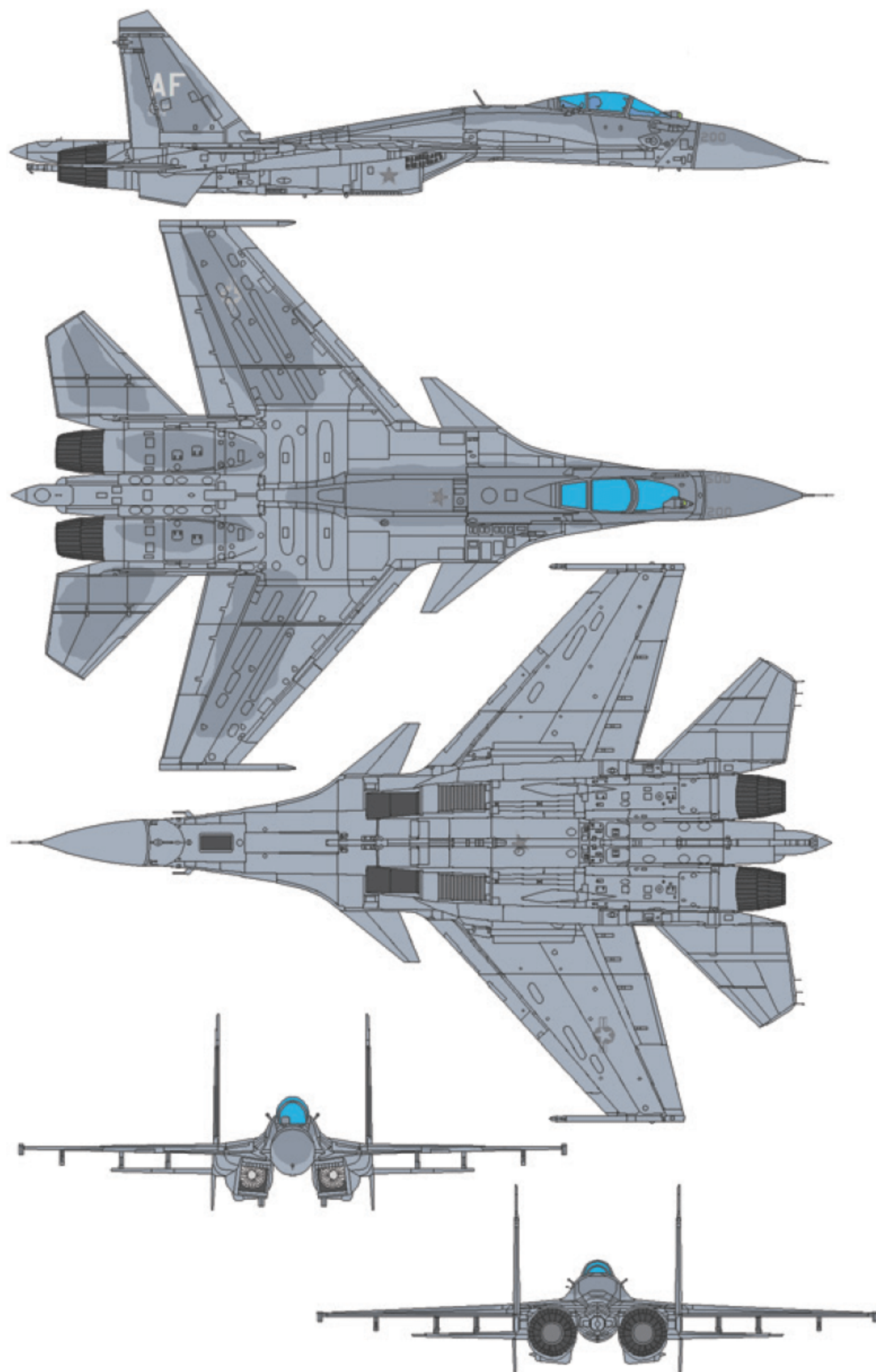
苏-33 战斗机结构图
