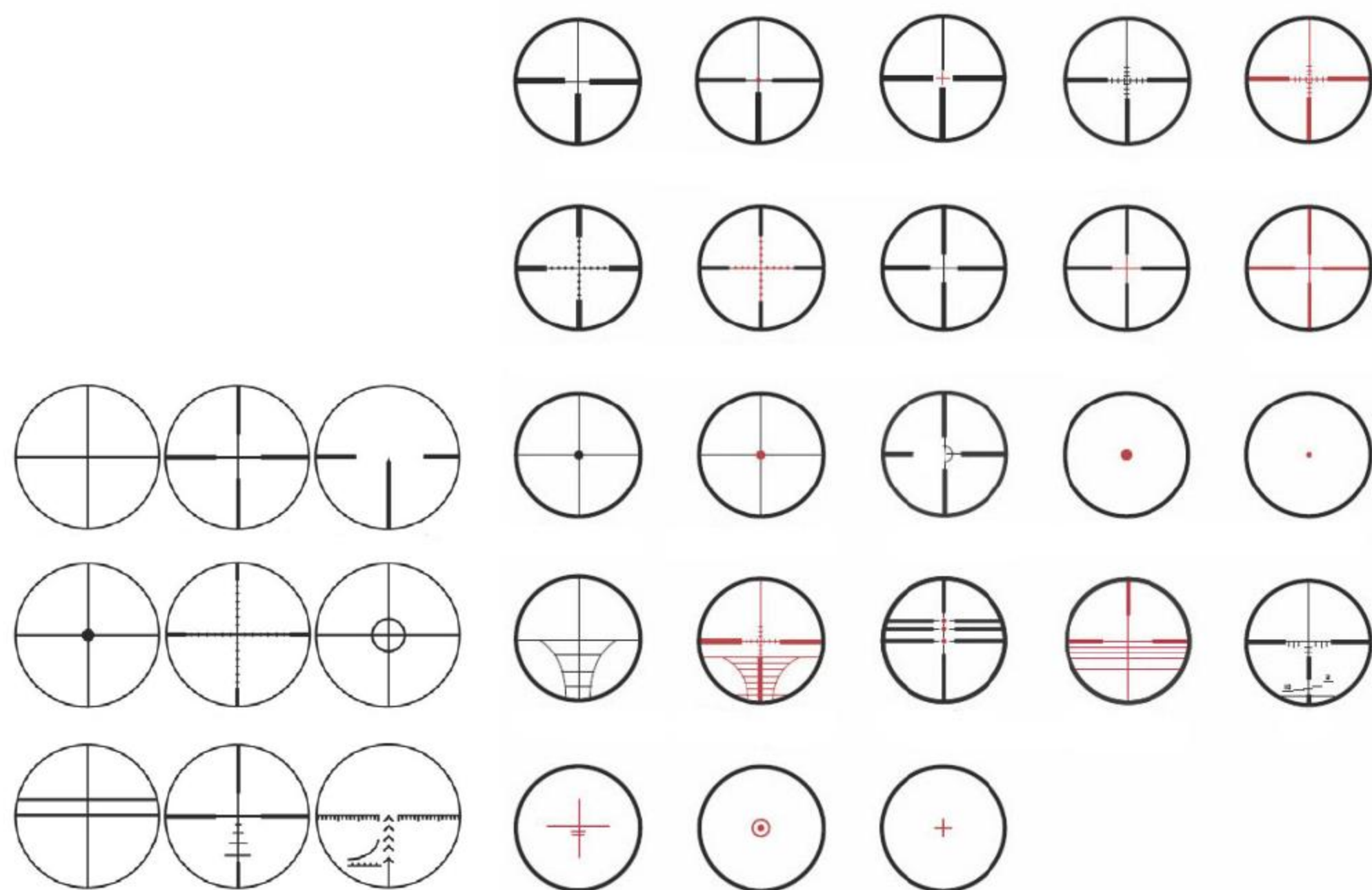
常见瞄准镜分划
