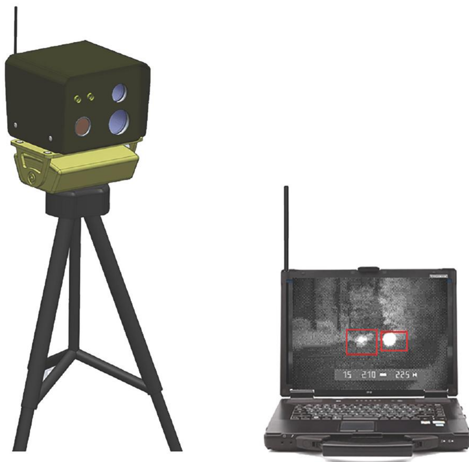
法国激光工业公司研制的狙击手探测系统
