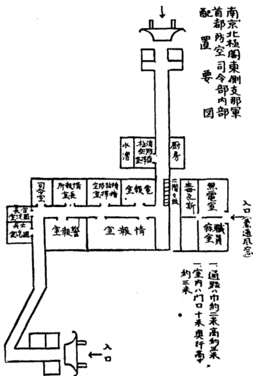
首都防空司令部配置要图
