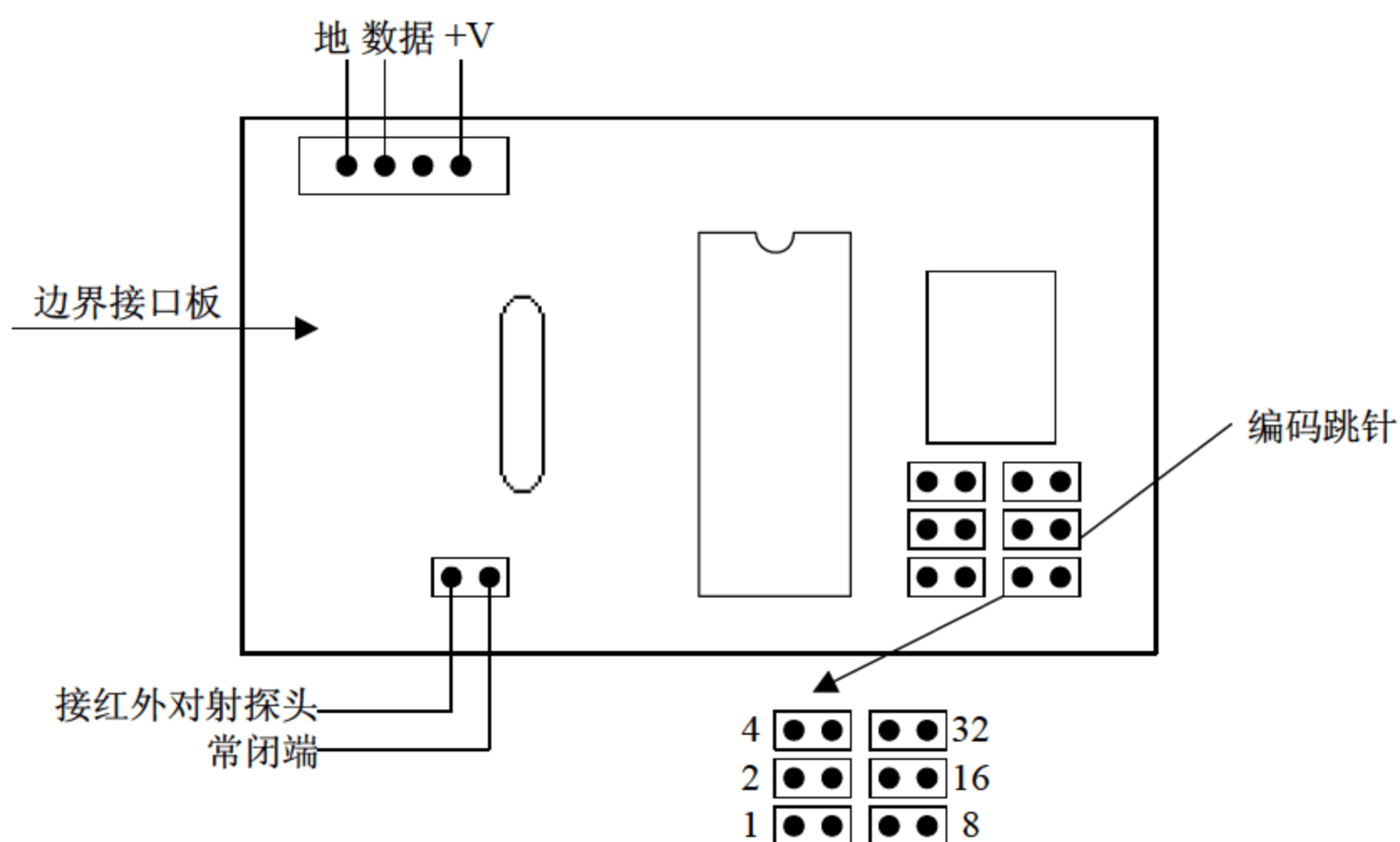
图 5-5 边界接口板示意图
