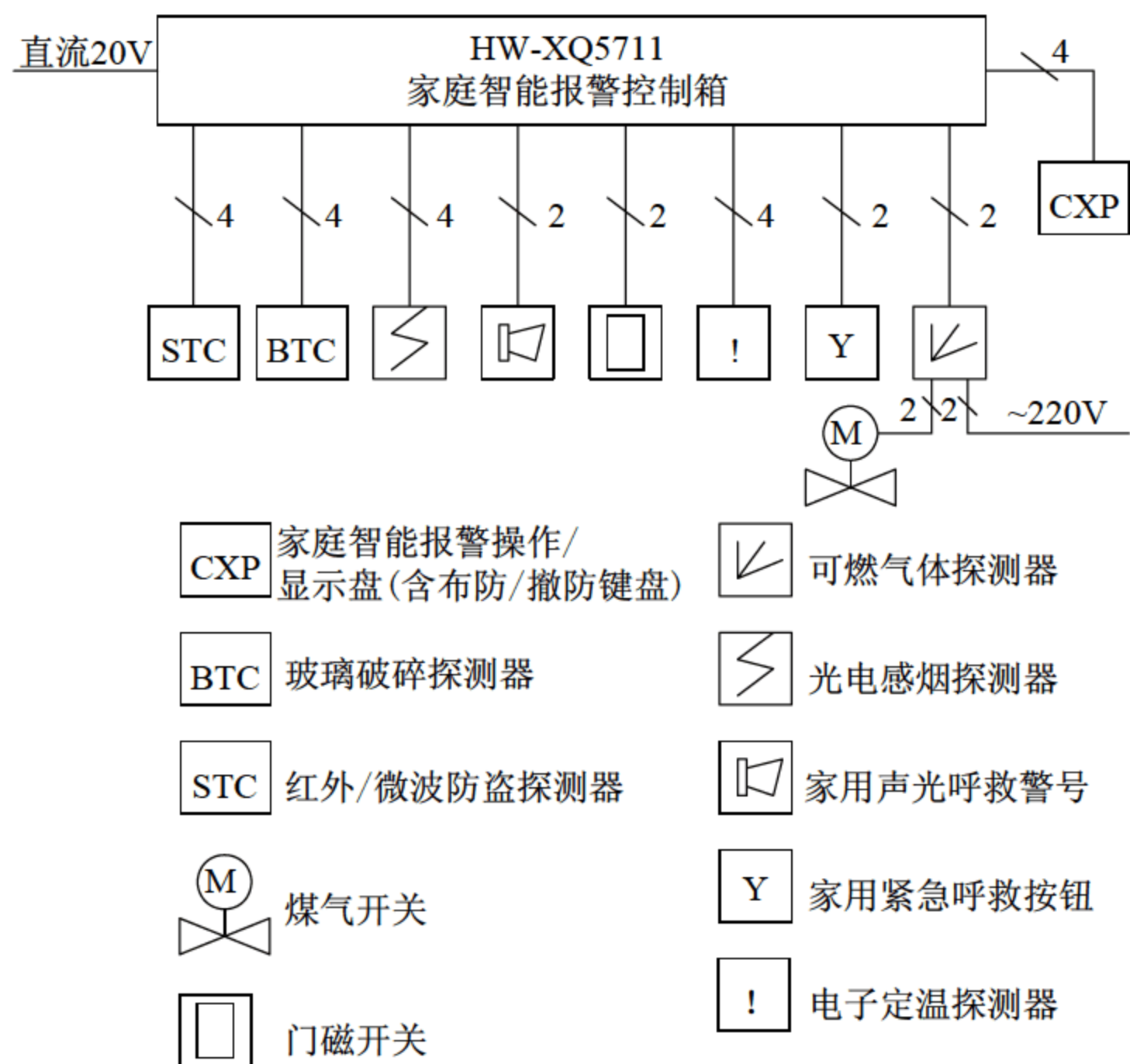
图 9-1 一个典型的家庭报警控制箱
