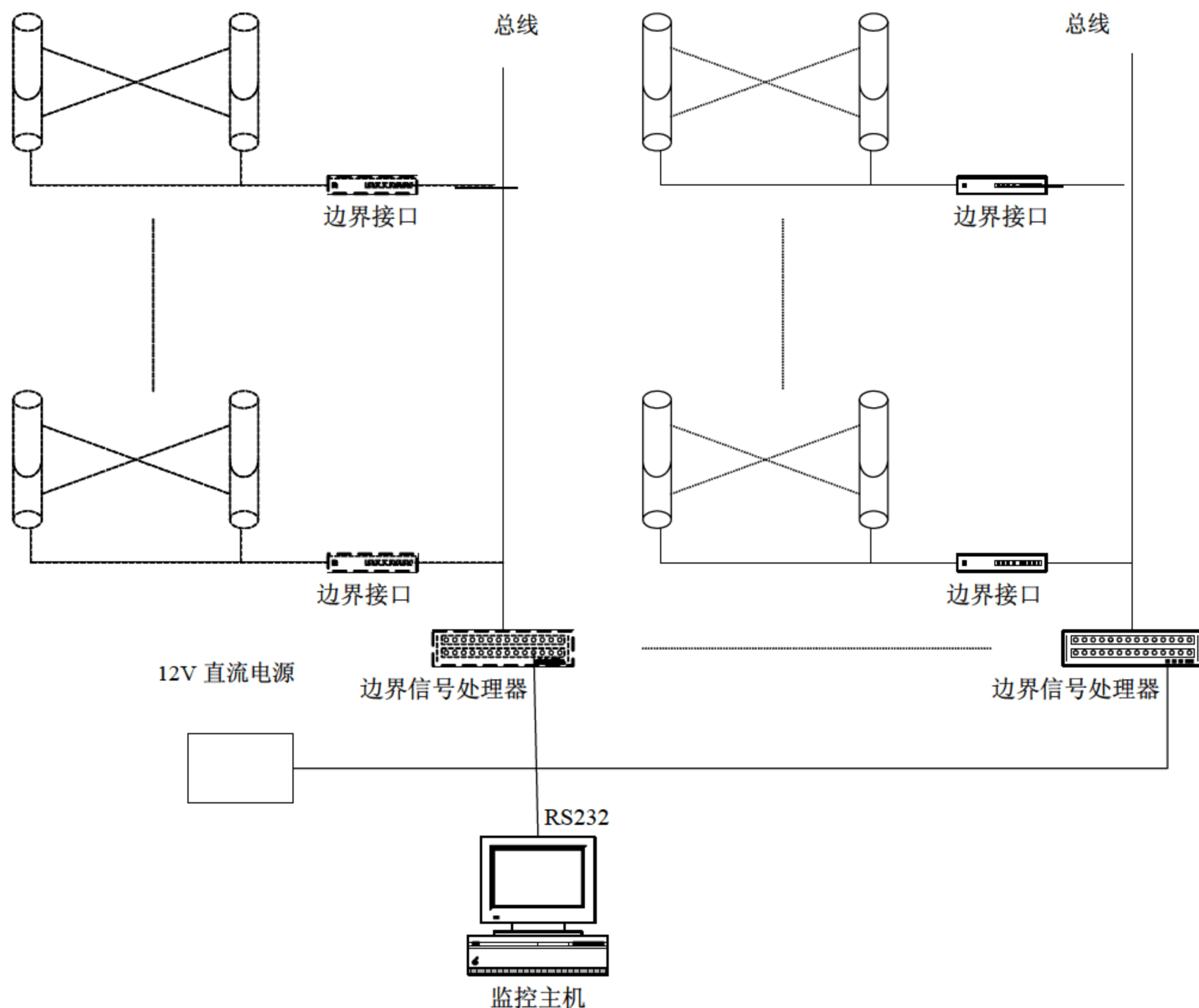
图 1-10 红外对射探头组成的边界防范子系统结构示意图
