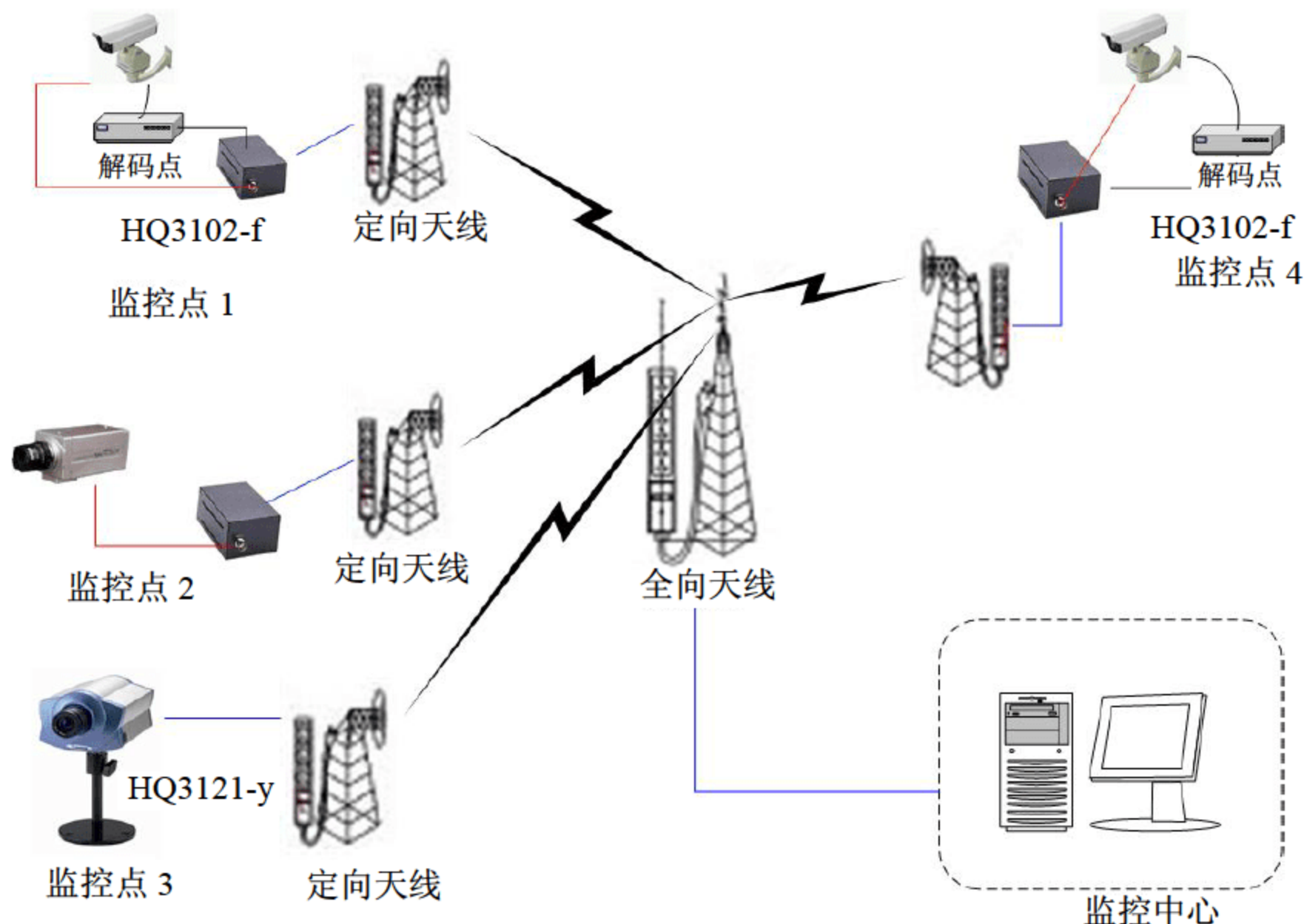
图 10-2 网络拓扑图
