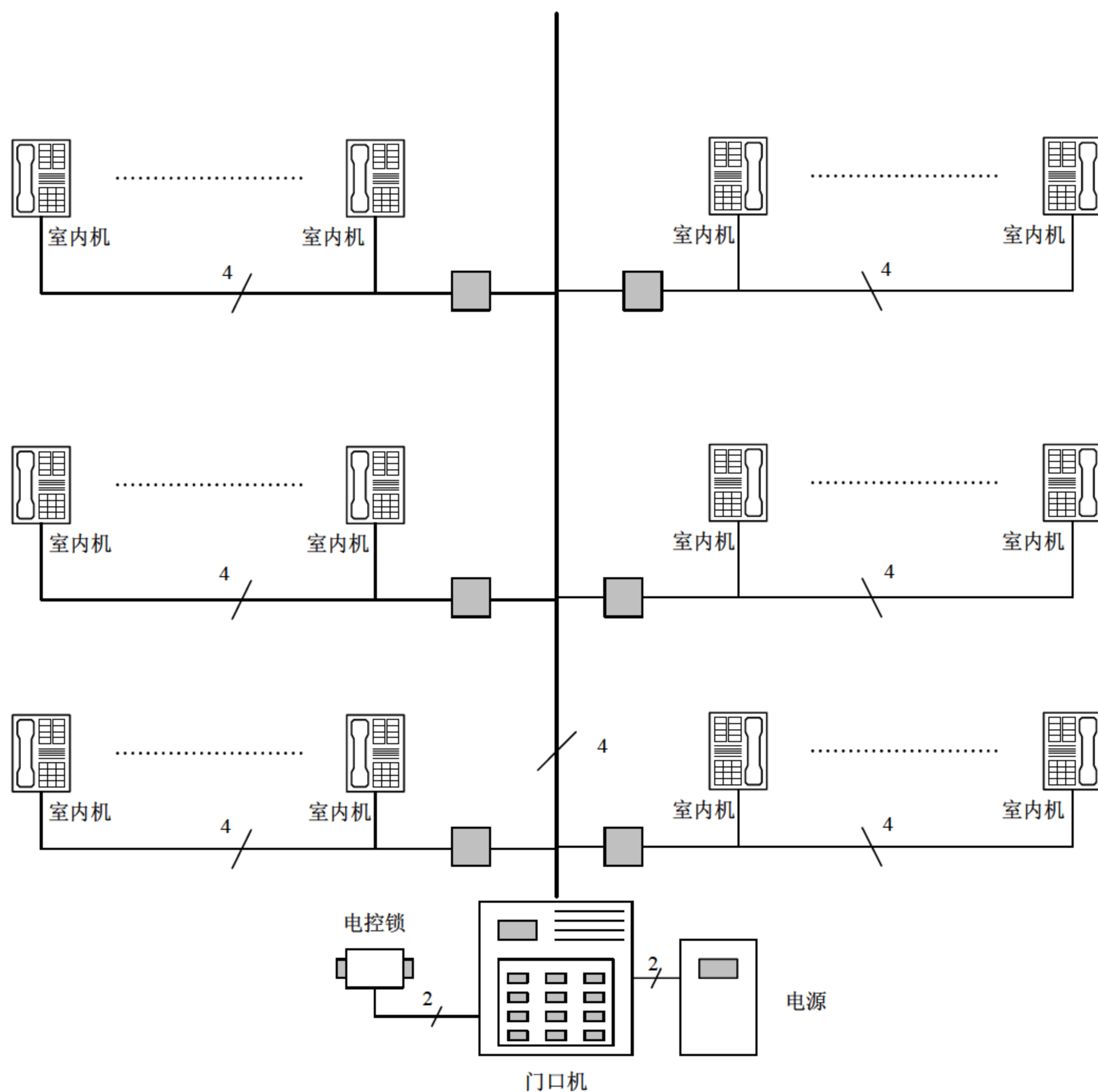
图 8-27 数码式普通对讲系统原理图
