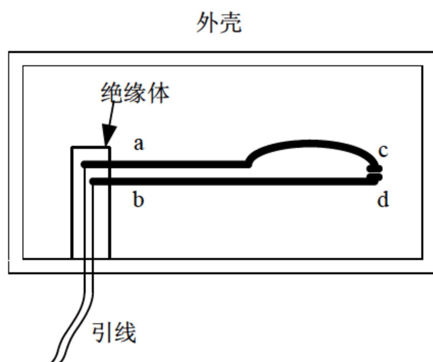
图 9-5 导电簧片式玻璃破碎探测器
