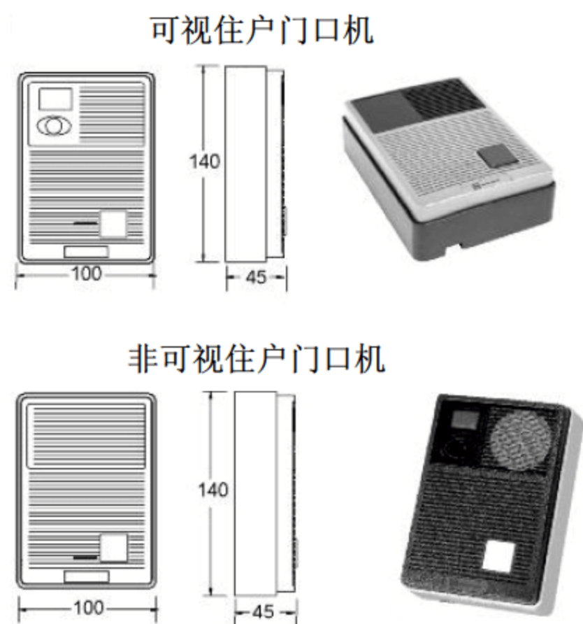
图 8-15 住户门口机
