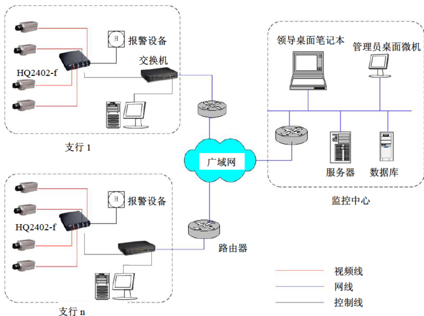
图 6-7 系统拓扑图
