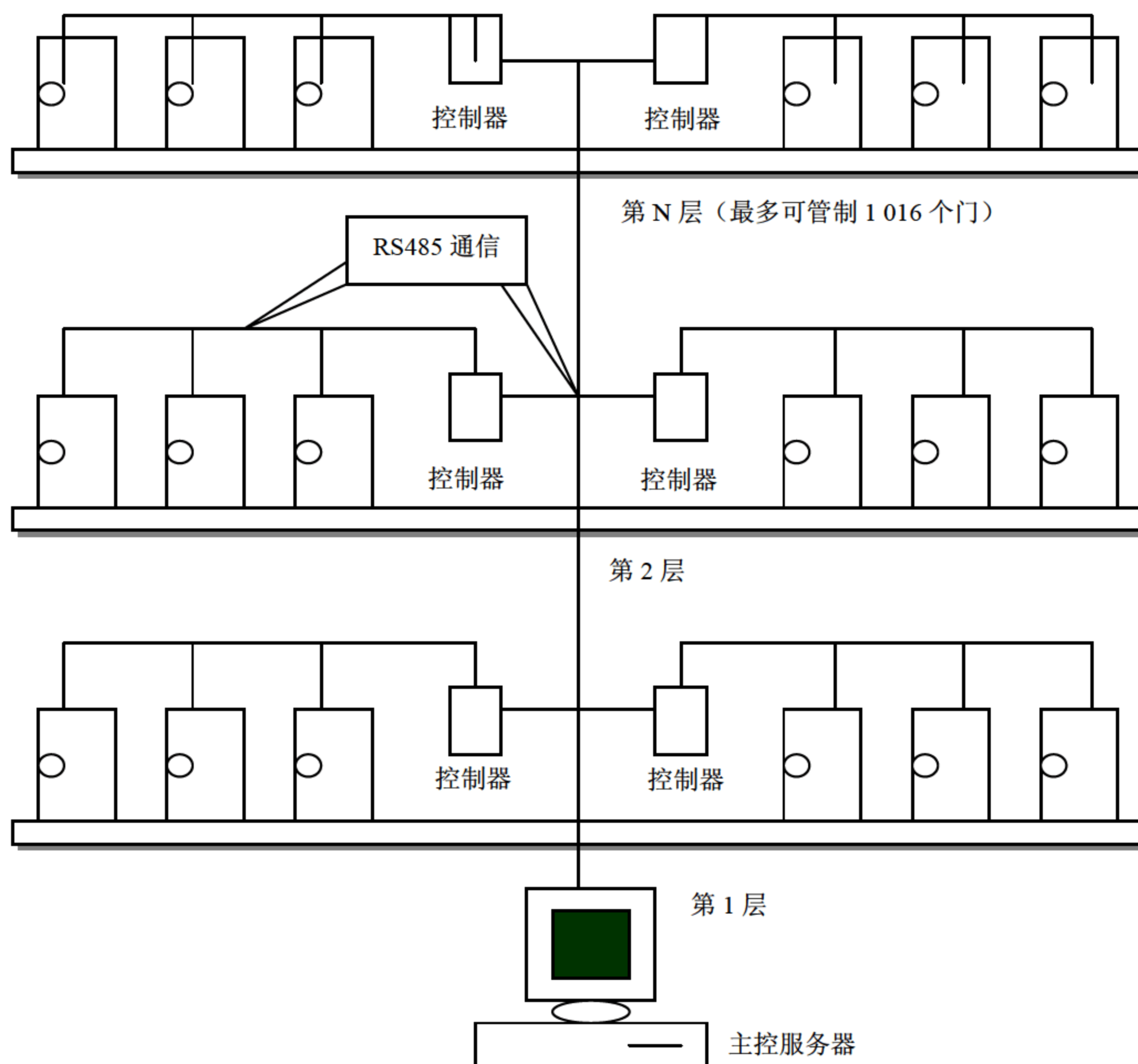
图 4-3 门禁系统网络示意图
