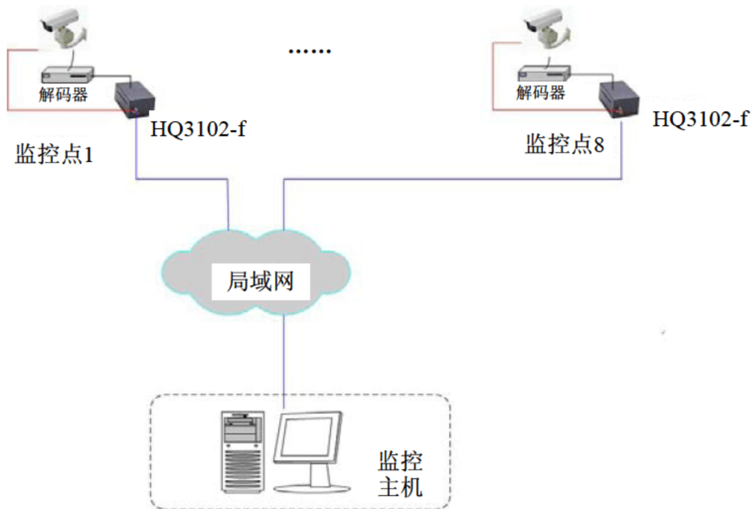
图 6-6 系统结构图
