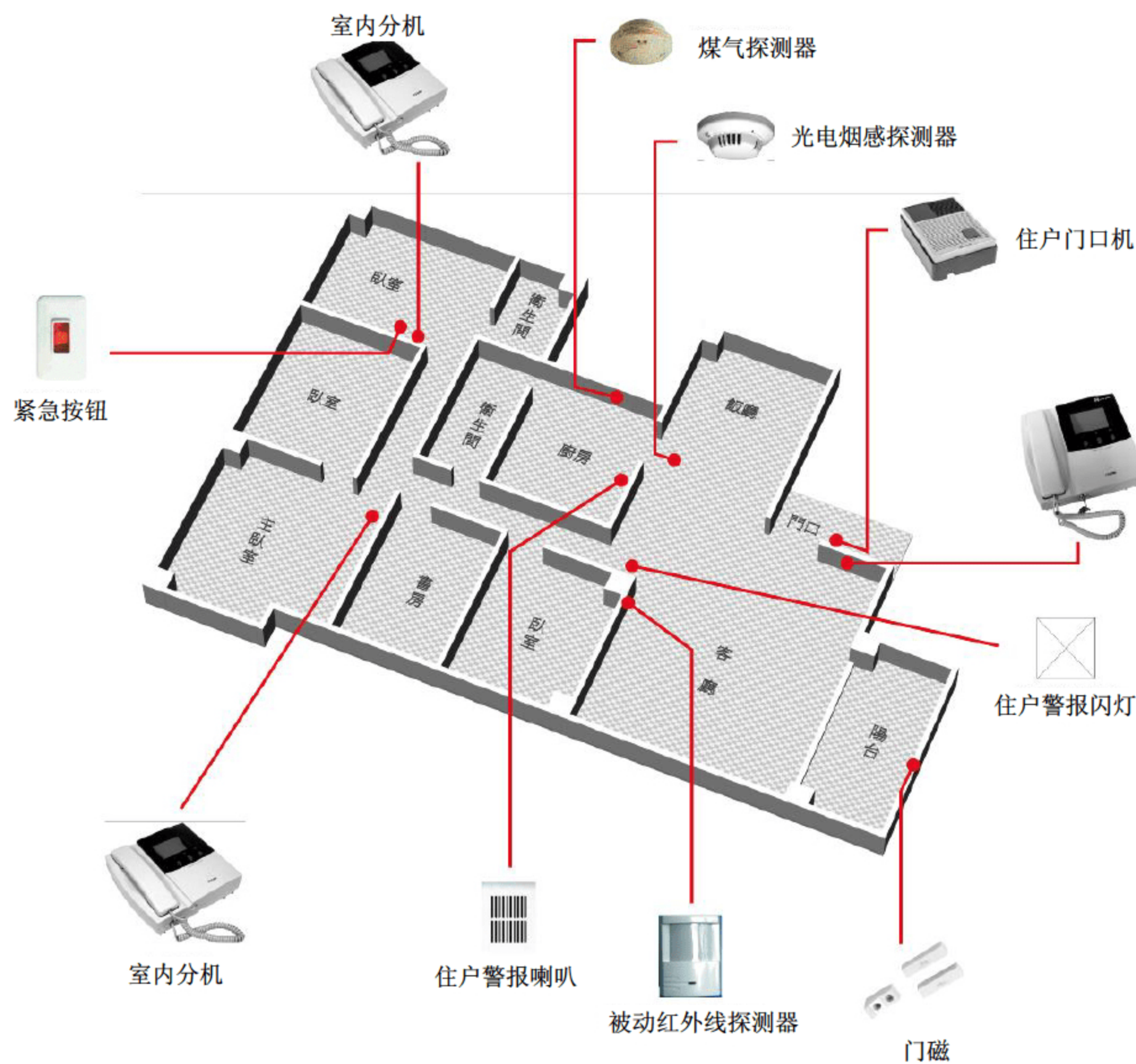
图 8-13 住户配置图（此图仅供参考，实际配置情况以现场施工为准）
