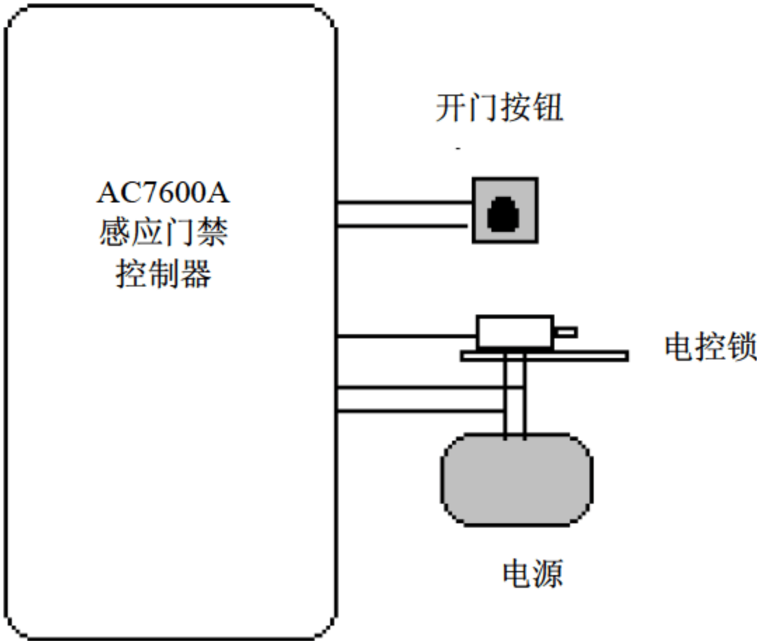
图 4-6 AC7600A 感应门禁系统示意图
