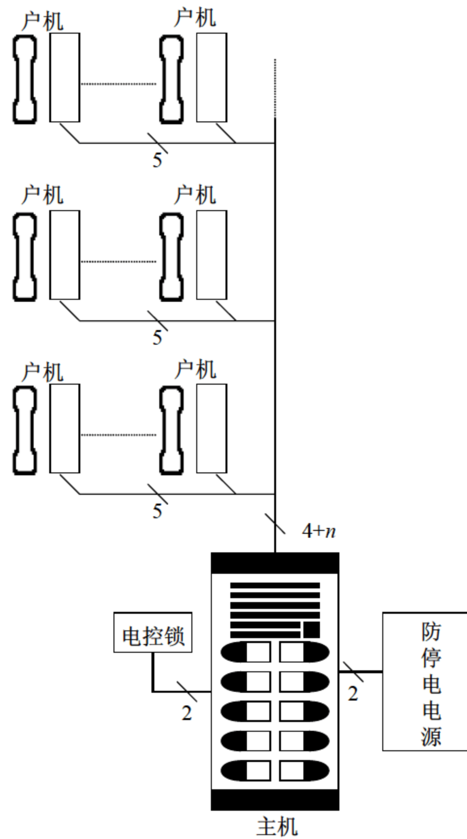
图 8-5 直接式对讲系统结构示意图
