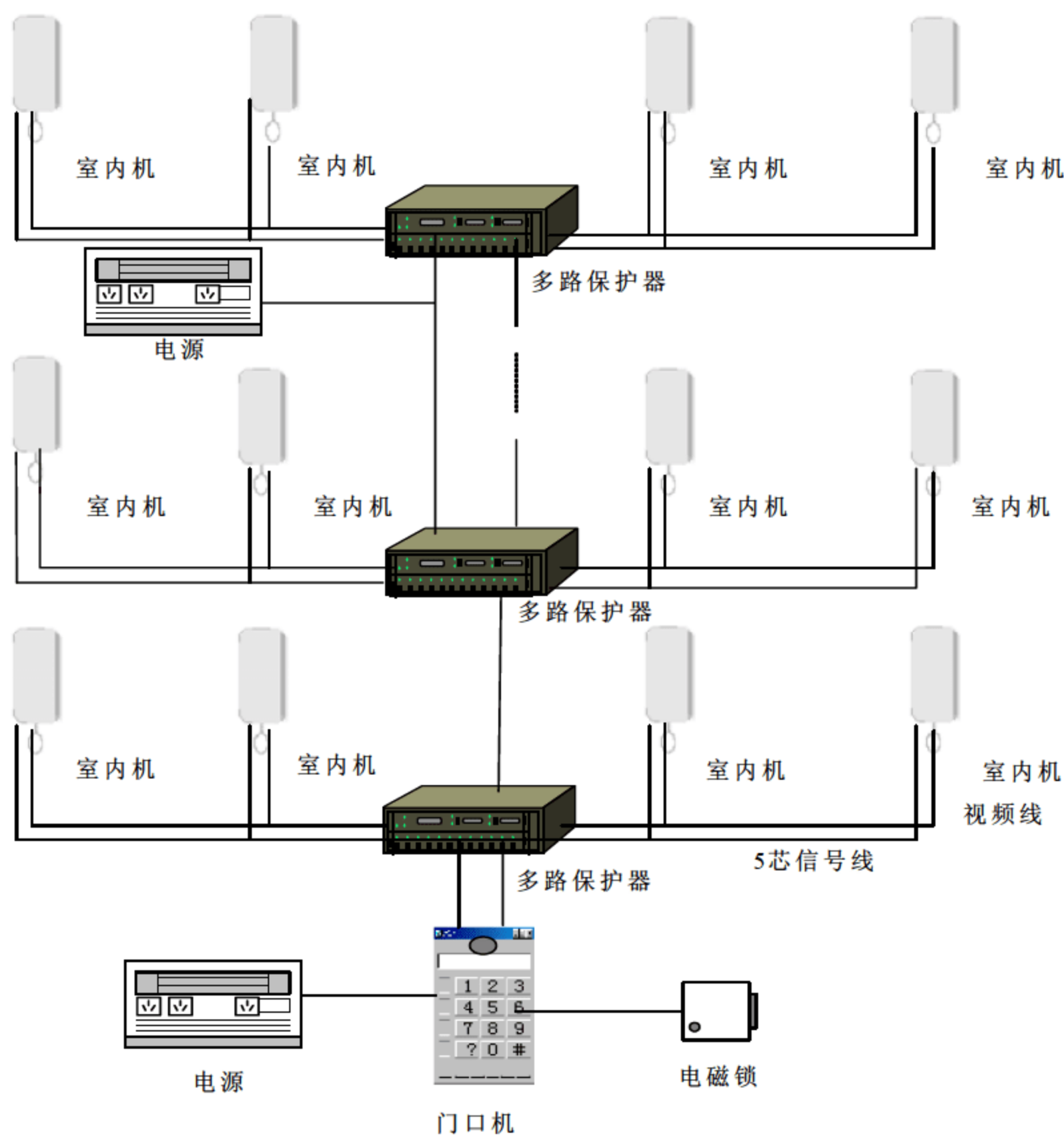
图 8-23 一座高层建筑的可视对讲系统原理图
