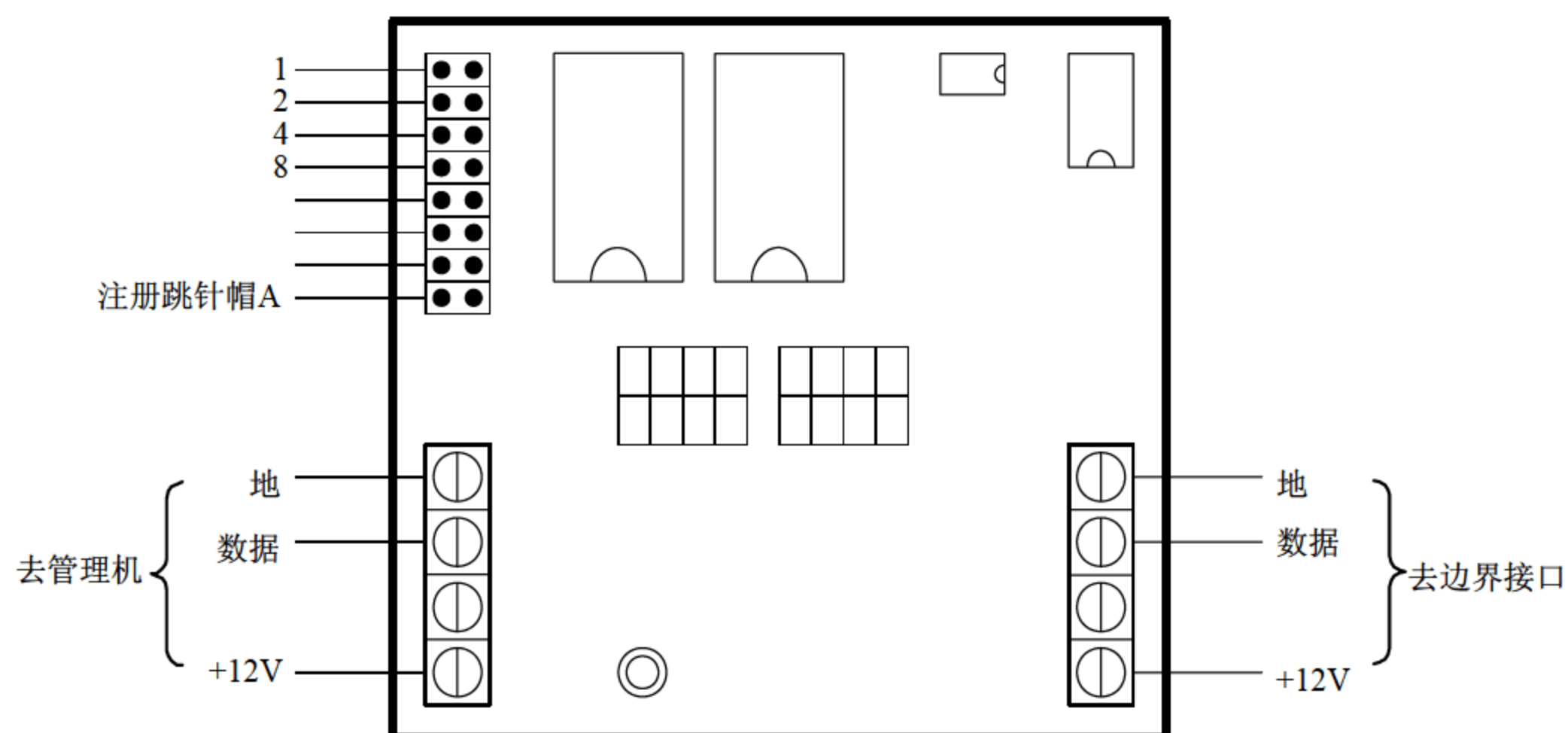
图 5-6 边界信号处理器电路板示意图
