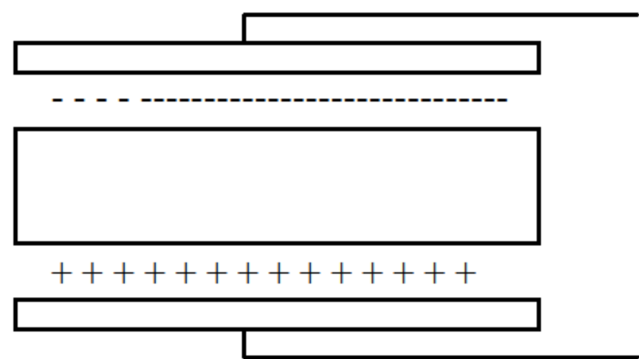
图 9-4 电介质极化现象
