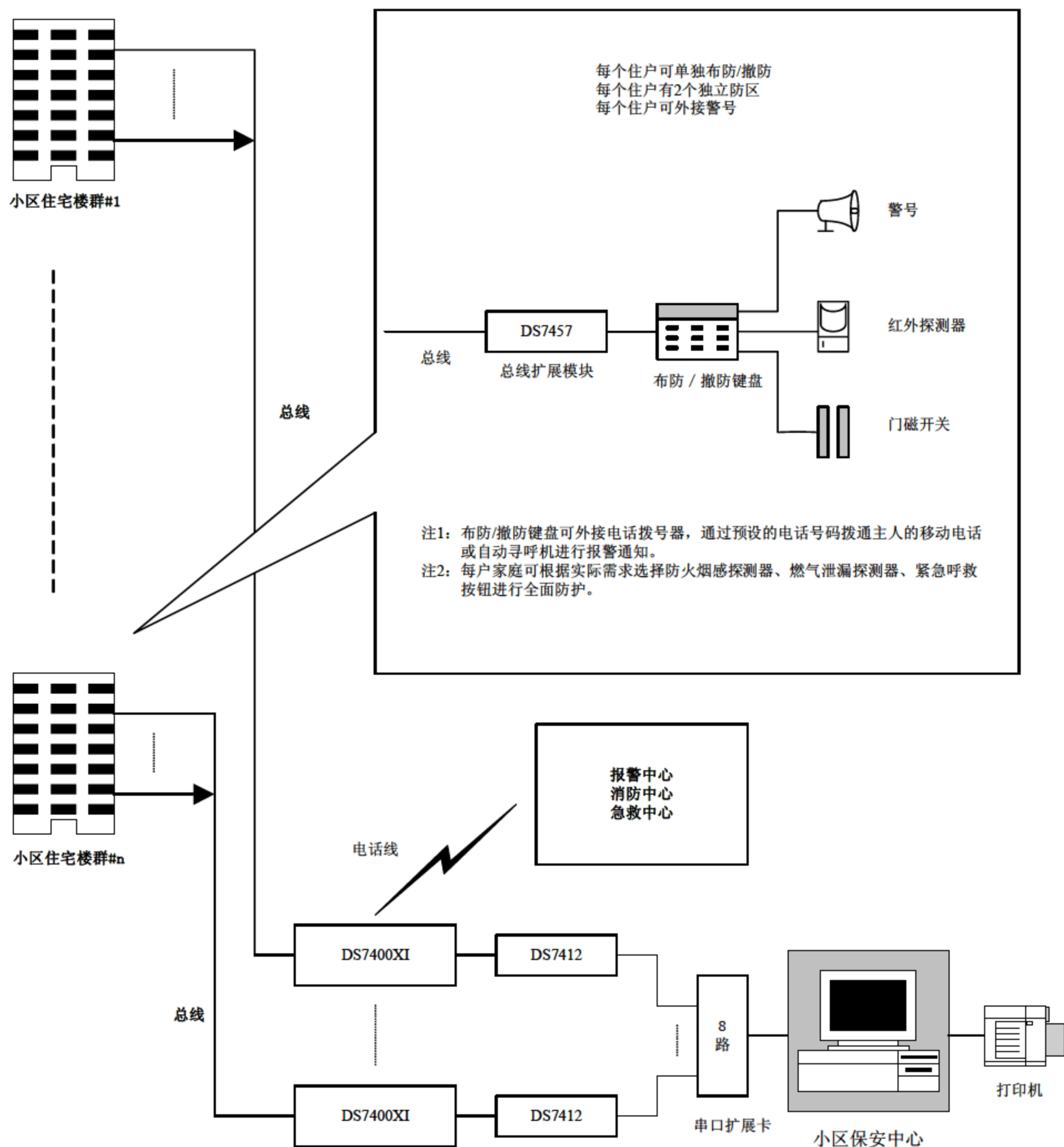
图 3-15 小区防盗报警系统结构及功能
