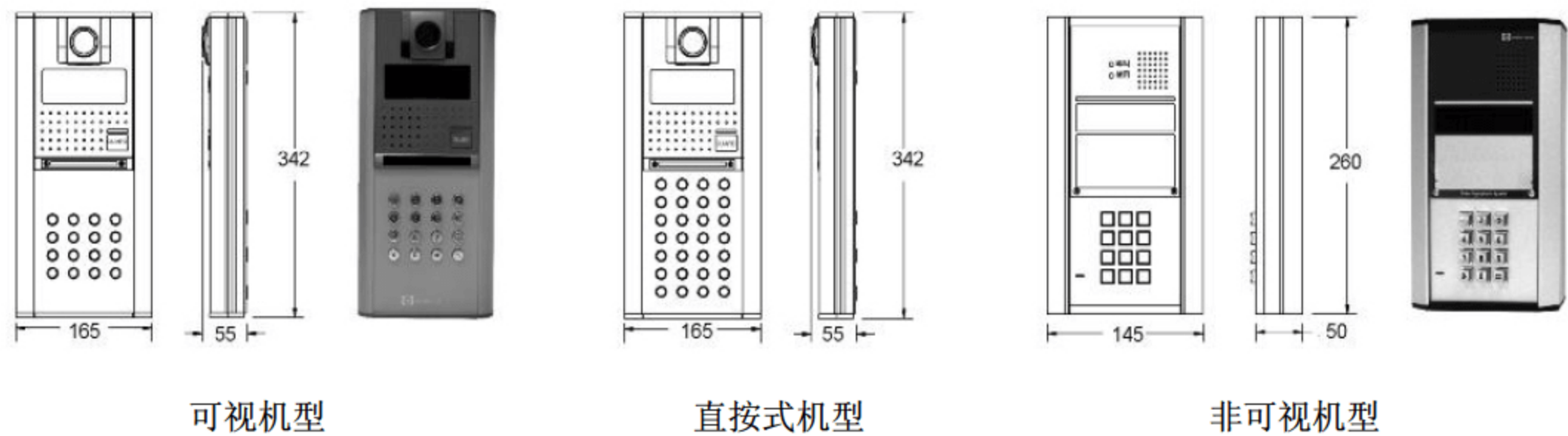
图 8-14 门口机机型
