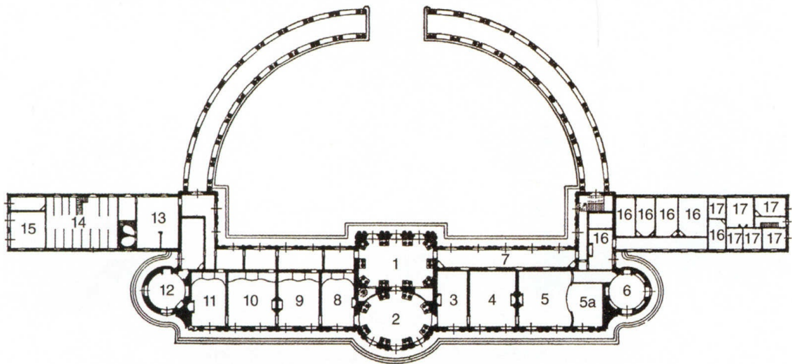
10.无忧宫平面图 (1) 入口大厅, (2) 大理石大厅/正式晚宴餐厅, (3) 前厅 (小餐厅), (4) 音乐室, (5) 书房和卧室, 带有放床的凹室 (5a), (6) 图书馆, (7) 画廊, (8—12) 客房, (13) 厨房, (14) 马厩, (15) 外围建筑, (16)
